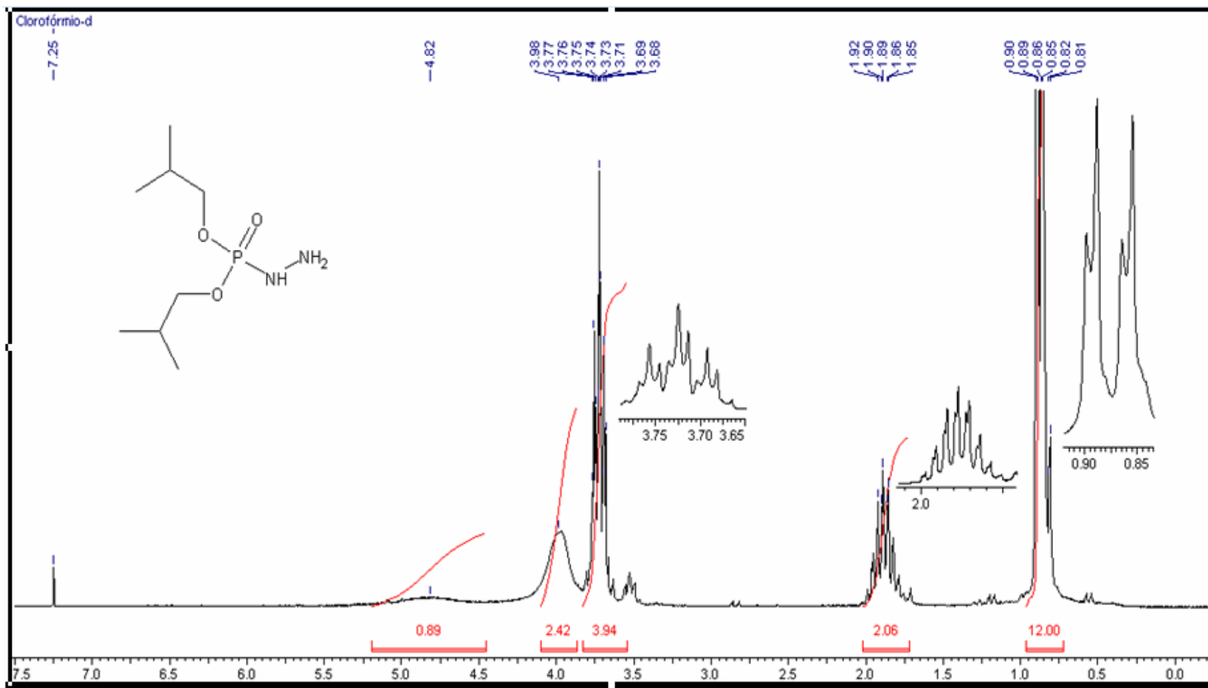
Figura 54: Espectro de RMN- 1 H da diisobutilfosforilidrazina (40).
