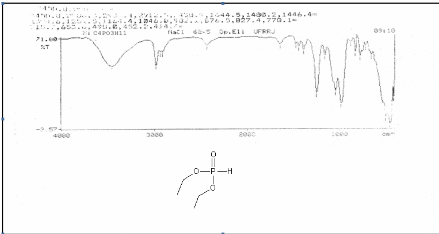
Figura 39: Espectro de infravermelho do fosfonato de dietila (35).
