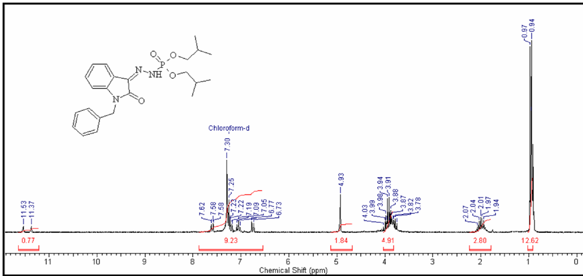
Figura 91: Espectro de RMN- ^1\text{H} ( \text{CDCl}_3 -200MHz) do ácido fosforoidrazídico N' -[1,2-diidro-2-oxo-1-(benzil)-3H-indol-3-ilideno]- éster de diisobutila (4).
