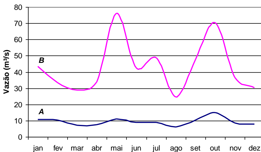
Figura 3.14. Regime anual do Rio das Pedras. A curva A é constituída pelas médias das vazões médias e a curva B , pelas médias das vazões máximas, considerando o período 1985-2005. Fonte: SUDERHSA/ANA.
