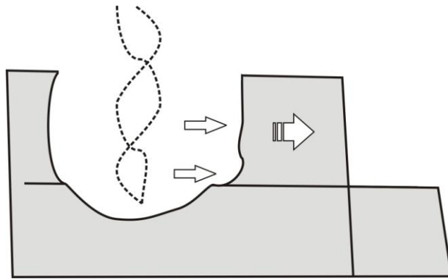
Figura 6.4. Interação entre o processo abrasivo formador de marmitas e o processo de arranque em leito fluvial em basaltos. O fluxo em vórtice (linhas tracejadas) força o arranque do bloco delimitado por fraturas e explora as linhas de fraqueza das fraturas horizontais. Na medida em que a feição abrasiva aumenta os blocos laterais tornam-se mais facilmente arrancáveis. Com isso as dimensões das marmitas são condicionadas pelo espaçamento das fraturas.
