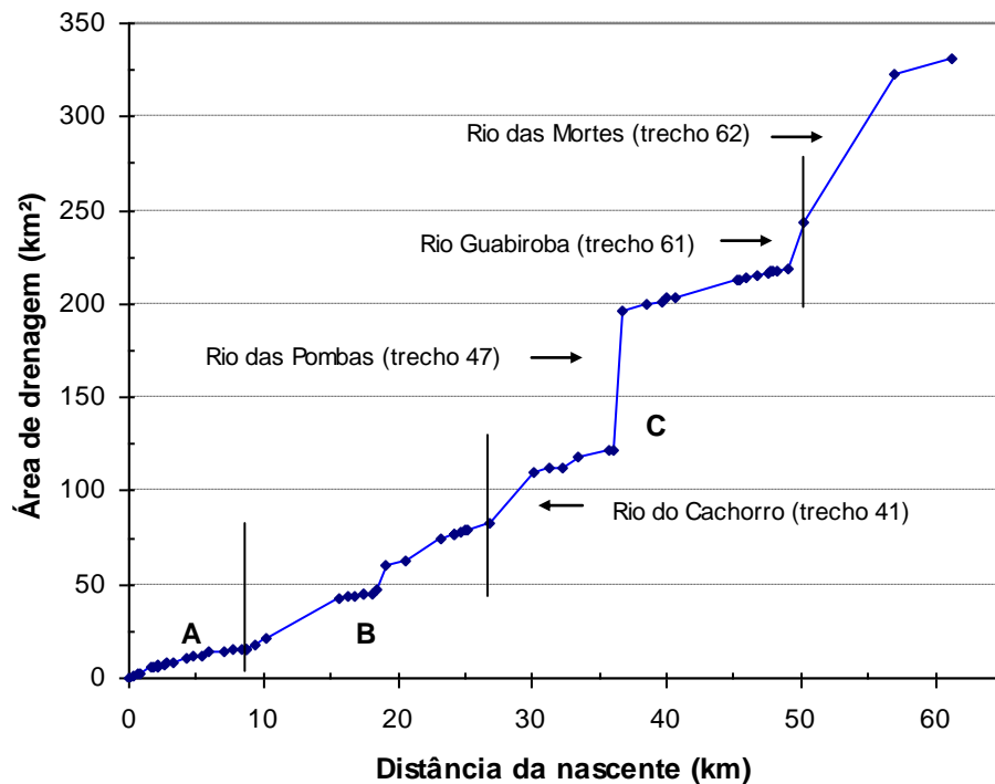
Figura 5.6. Aumento da área drenada em função do aumento da distância da nascente. As setas indicam os maiores incrementos, que ocorrem devido à inserção dos principais afluentes. As letras A, B e C designam os compartimentos do perfil longitudinal, delimitados por barras verticais, cujas declividades apresentam comportamentos gerais distintos, conforme identificados na Figura 5.3. Ver discussão no texto.
