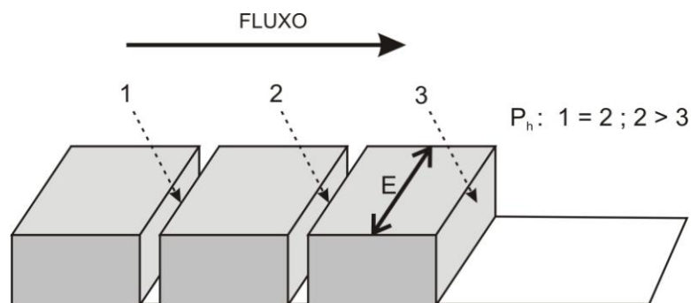
Figura 10.5. Idealização das condições de pressão hidrostática atuantes em uma ruptura de declive em meio fraturado, conforme conclusões de Dubinski (2008). O deslocamento dos blocos (arranque) ocorre devido principalmente ao diferencial de pressão hidrostática ( P_h ) existente no bloco frontal da ruptura. Quanto maior for o bloco, isto é, quanto maior o espaçamento das fraturas ( E ), maior será o diferencial de pressão entre a face do bloco voltada para montante e a face voltada para jusante, facilitando o arranque.
