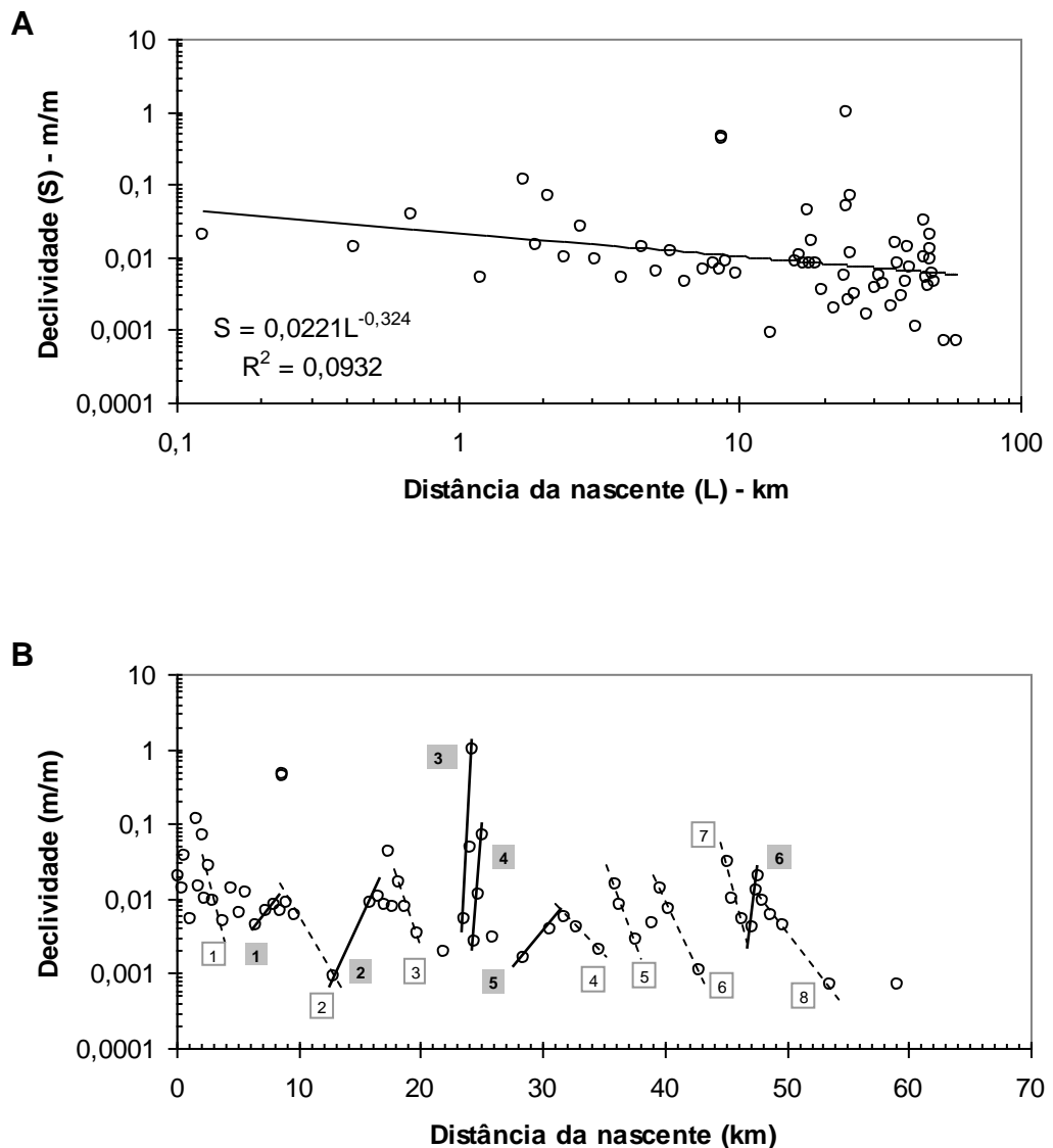
Figura 5.4. Relação entre declive e distância da nascente no Rio das Pedras, plotadas em escalas bi-logarítmica (A) e mono-logarítmica (B). Em A foi ajustada uma reta de regressão pela qual se descreve o perfil em termos de rugosidade pelo coeficiente de determinação ( R^2 ), conforme Shepherd (1985). Em B estão identificados os segmentos côncavos (linhas tracejadas) e convexos (linhas cheias) do perfil, numerados sequencialmente. Dados no Anexo C.
