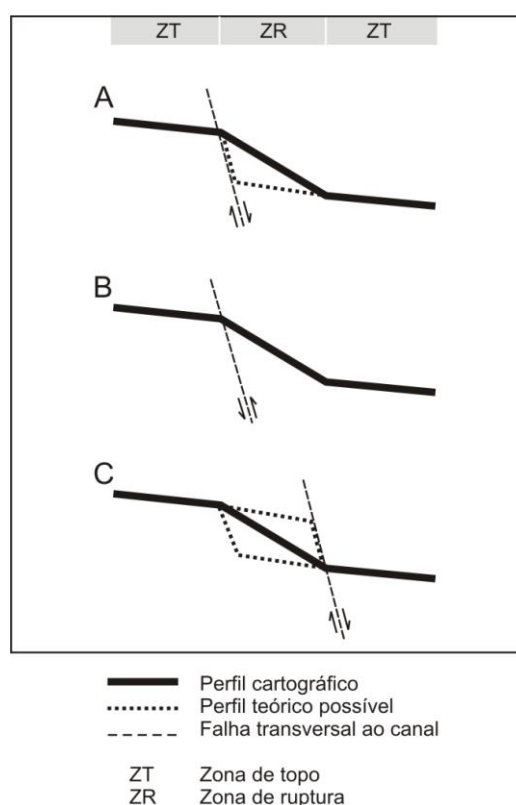
Figura 9.1. Representação esquemática da interação entre falhas transversais ao canal e os declives do perfil longitudinal. Nos três casos (A, B e C) o primeiro trecho pode ser também uma zona de ruptura de baixa declividade relativa, constituindo com o trecho seguinte um segmento convexo. Em A e B a falha coincide com o início da zona de ruptura, sendo do tipo normal no primeiro caso e inversa no segundo; em C a falha é normal, mas está situada no final da zona de ruptura.
