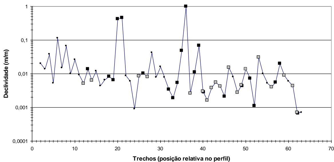
Figura 6.2. Declividade dos trechos do Rio das Pedras com as respectivas características estruturais dos basaltos: quadrado preto = basalto maciço; quadrado cinza = basalto vesicular-amidalóide; ponto = sem dados.
