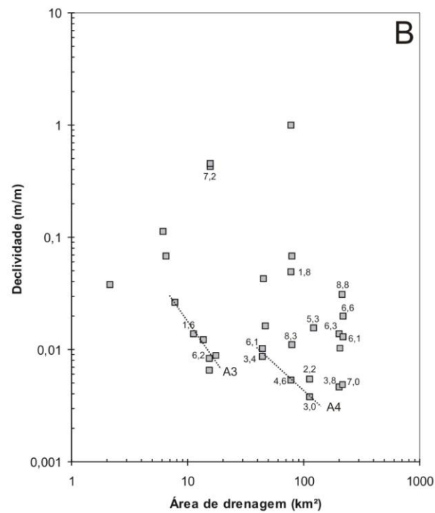
Figura 10.10. Relação declive-área para zonas de topo (A) e zonas de ruptura (B) do perfil longitudinal do Rio das Pedras, evidenciando a densidade de fraturas característica de cada trecho analisado em campo. Os alinhamentos A1, A2, A3 e A4 são os mesmos que aparecem na Figura 10.8.
