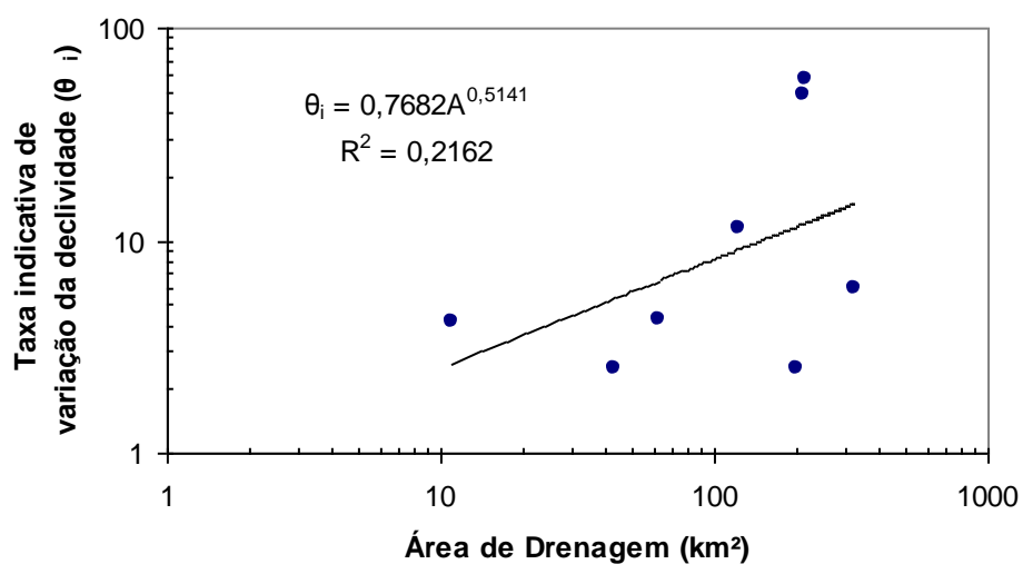
Figura 9.5. Relação entre a taxa indicativa da variação da declividade ( \theta_i ) e a área de drenagem.
