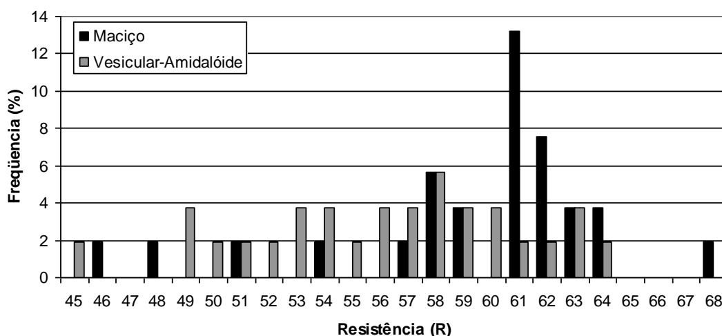
Figura 7.2. Distribuição de frequências da resistência da rocha intacta ( n = 53 ) conforme o subtipo de basalto da área de estudo. Como a amostragem foi efetuada por trechos do perfil, para evitar tendenciosidade foram excluídos os valores repetidos em um mesmo trecho.
