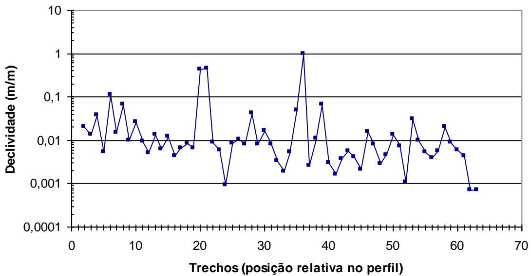
Figura 5.3. Relação entre declividade e posição relativa dos trechos do canal do Rio das Pedras. Os dados dos trechos foram plotados sequencialmente (posição relativa), sem escala, portanto não obedecendo o posicionamento absoluto, ou seja, a posição definida pela distância da nascente.
