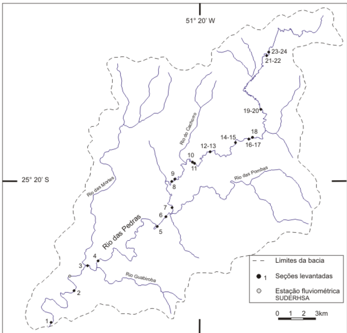
Figura 4.2. Localização das seções transversais levantadas ao longo do Rio das Pedras para cálculo da relação entre vazão de margens plenas e área de drenagem.
