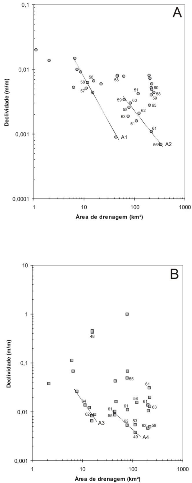
Figura 10.9. Relação declive-área para zonas de topo (A) e zonas de ruptura (B) do perfil longitudinal do Rio das Pedras, evidenciando a resistência da rocha intacta característica de cada trecho analisado em campo. Os alinhamentos A1, A2, A3 e A4 são os mesmos que aparecem na Figura 10.8.
