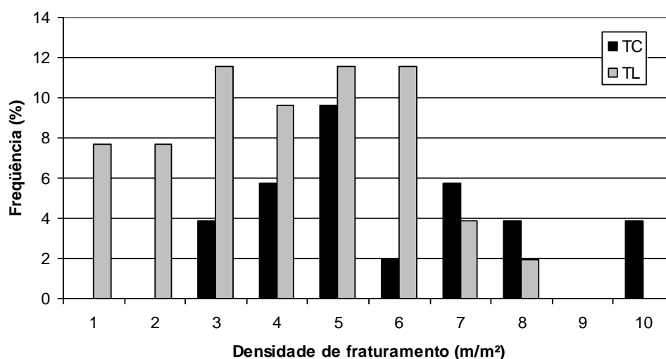
Figura 9.4. Distribuição de freqüência da densidade de fraturamento em trechos controlados direcionalmente por fraturas tectônicas (TC) e em trechos livres de controle (TL).
