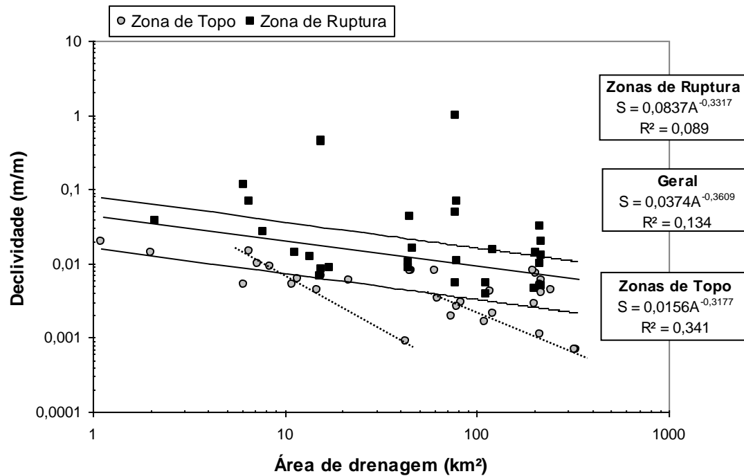
Figura 5.7. Relação entre declividade e área de drenagem no Rio das Pedras. As retas de regressão foram ajustadas separadamente para as zonas de ruptura (reta superior), zonas de topo (reta inferior) e para ambas as morfologias (reta intermediária). Alinhamentos aparentes de pontos estão identificados com linhas pontilhadas.
