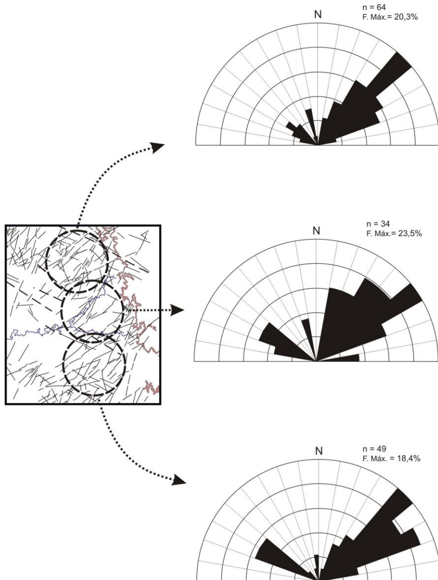
Figura 3.6. Orientações regionais de fraturamento. O mapa mostrado corresponde à Figura 3.5.
