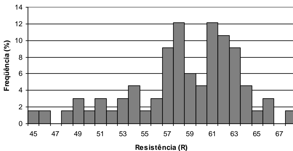
Figura 7.1. Distribuição de freqüência da resistência litológica medida com esclerômetro em 64 locais no leito do Rio das Pedras.
