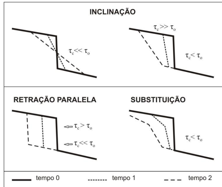
Figura 1.1. Modelos de evolução de rupturas de declive, segundo Gardner (1983).
