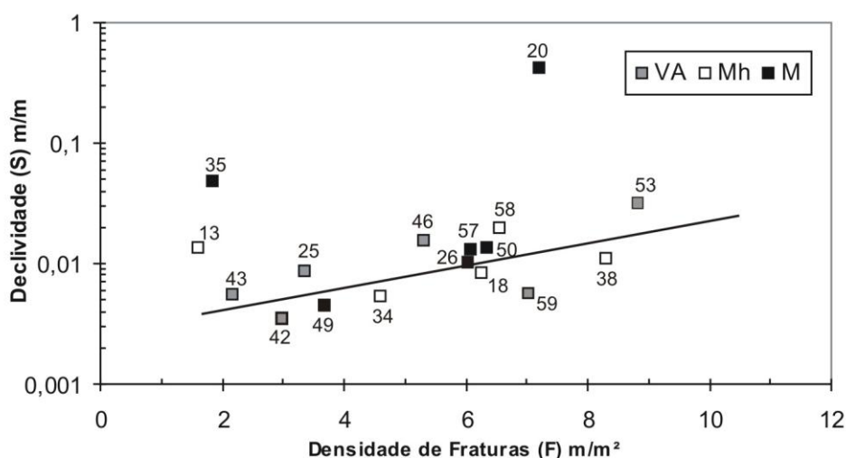
Figura 10.12. Relação entre declividade e densidade de fraturas em zonas de ruptura. Esta figura é a mesma apresentada no Capítulo 8 (Figura 8.5B), com exceção de que identifica os trechos, com números colocados junto aos símbolos, e apresenta para alguns trechos apenas a média de fraturamento. A linha de melhor ajuste é definida por S = 0,0036e^{0,17F} e não considera os valores extremos de declividade dos trechos 20 e 35. A dispersão vertical dos dados ocorre, sobretudo, em função do grau de controle tectônico sobre os declives: quanto maior o controle, maior é a declividade.
