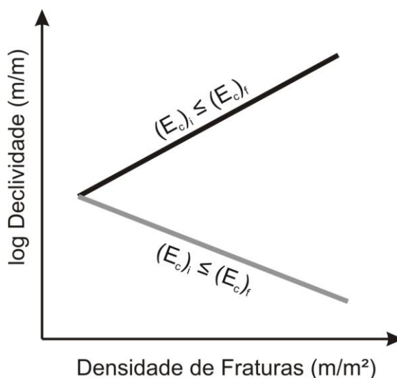
Figura 10.1. Representação esquemática da relação entre declividade do canal e densidade de fraturas. As retas que descrevem o comportamento de zonas de topo (linha cinza) e zonas de ruptura (linha preta) são baseadas nos resultados obtidos no capítulo 8. (E_c)_i é a capacidade erosiva no início de um determinado trecho e (E_c)_f é a capacidade erosiva no final desse trecho.
