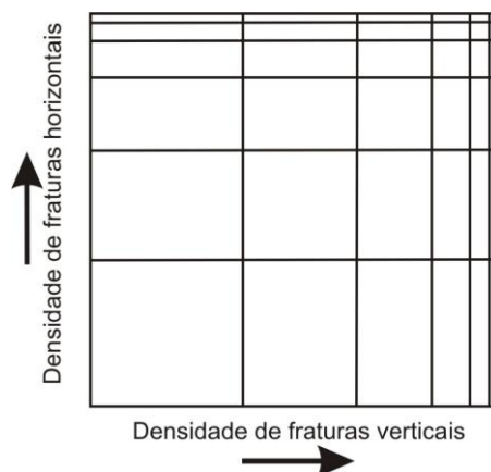
Figura 8.6. Representação esquemática da variação combinada de densidade de fraturas horizontais e verticais. A probabilidade de arranque aumenta de baixo para cima e da esquerda para direita.
