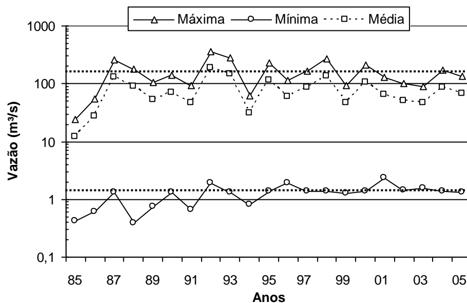
Figura 3.13. Vazões máxima, mínima e média do Rio das Pedras no período 1985-2005. As linhas pontilhadas horizontais indicam as médias máxima e mínima. Fonte: SUDERHSA/ANA.
