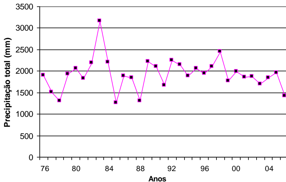
Figura 3.12. Precipitação total anual para o período 1976-2006 na área de estudo. Fonte: IAPAR.
