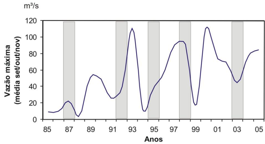
Figura 3.17. Médias das vazões máximas de primavera no período 1985-2005. As faixas cinza correspondem aos anos de El Niño mais acentuado. Fonte: dados hidrológicos – SUDERHSA/ANA; dados climáticos – www.cpc.ncep.noaa.gov .
