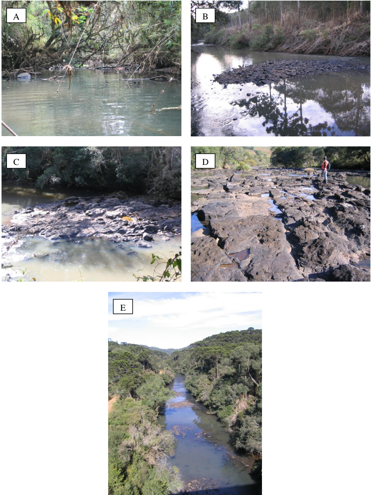
Figura 3.10. Características do leito do Rio das Pedras. Em A, leito aluvial em areia e cascalho fino (trecho 24); em B, seqüência de soleiras formadas por barras de cascalho muito grosso até blocos (trecho 49); em C, soleira rochosa (trecho 49); em D, leito rochoso extenso em zona de ruptura (trecho 57); em E, leito aluvial formando seqüência de soleiras e depressões (trecho 48).
