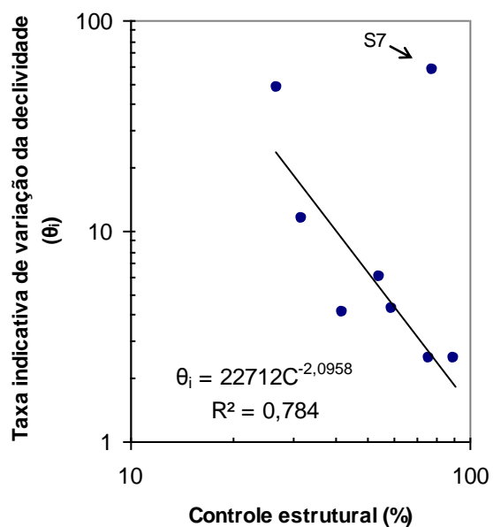
Figura 9.6. Relação entre a taxa indicativa de variação da declividade e o grau de controle estrutural sobre a direção do canal. A reta de melhor ajuste foi obtida desconsiderando o segmento 7 (S7). Ver discussão no texto.
