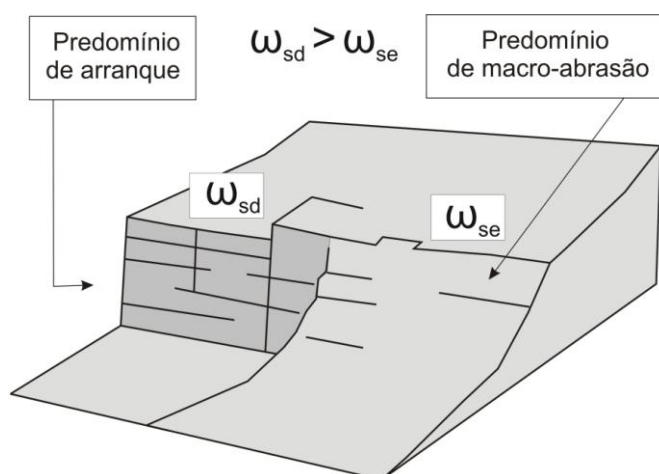
Figura 10.3. Morfologia dupla encontrada em rupturas de declive em basalto maciço e sua relação com a potência do escoamento e com os processos erosivos. No setor direito (sd) do canal a face da ruptura é íngreme e o arranque é mais eficiente devido à maior potência do escoamento ( \omega ). No setor esquerdo (se) a morfologia é de rampa, havendo predomínio de macro-abrasão, porque a potência do escoamento não é suficiente para deslocar os blocos.
