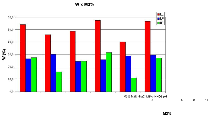
Figura 5.5: Variação de LL, LP e IP da amostra M3% com diferentes fluidos.
