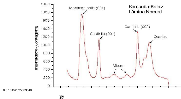
Figura 3.18: Difratoograma da bentonita (lâmina normal).
