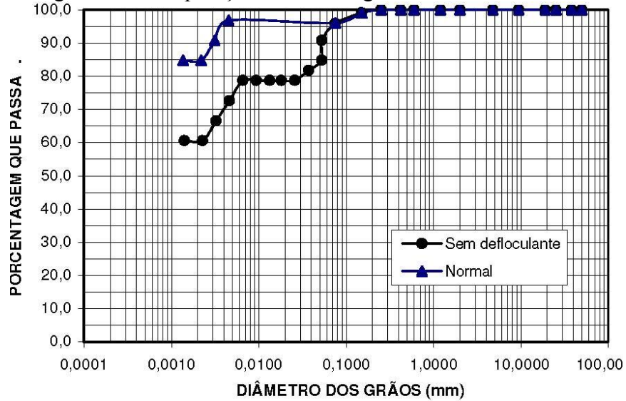
Figura 3.7: Comparação das curvas granulométricas de M6%.
