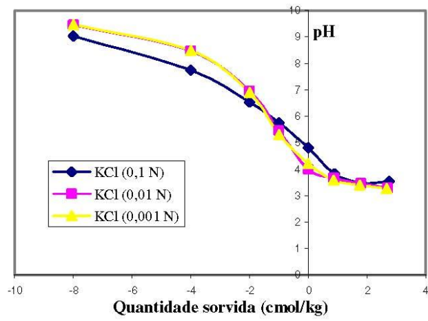
Figura 3.12: Diagrama da titulação potenciométrica para a amostra SN.
