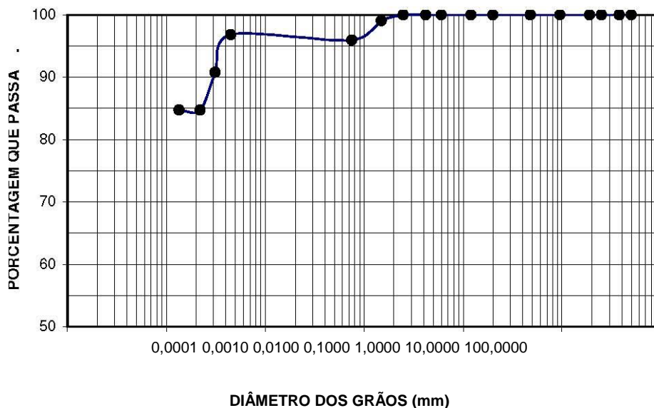
Figura 3.4: Curva granulométrica da bentonita.
