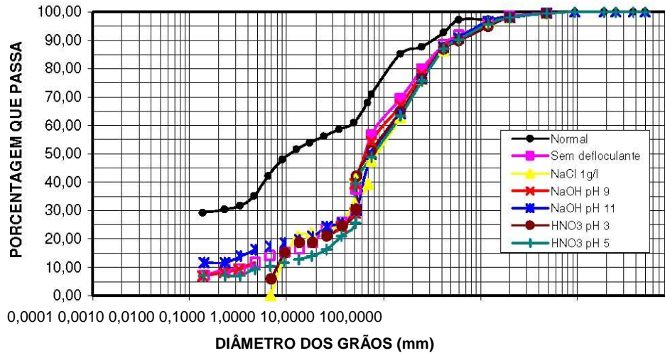
Figura 5.10: Curvas granulométricas da amostra M3% com diferentes soluções.
