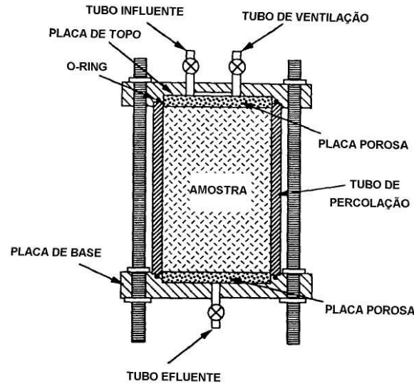
Figura 2.13: Esquema construtivo de um Permeâmetro de Parede Rígida segundo Daniel (1994).
