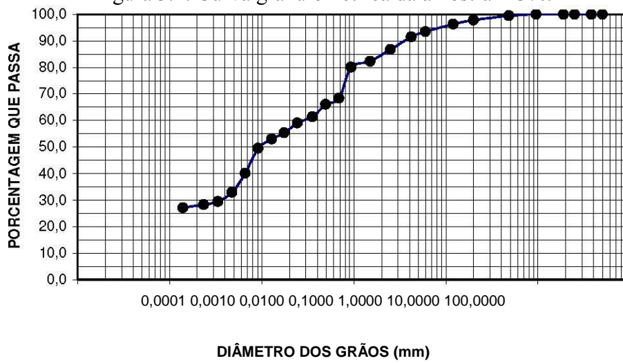
Figura 3.2: Curva granulométrica da amostra M3%.
