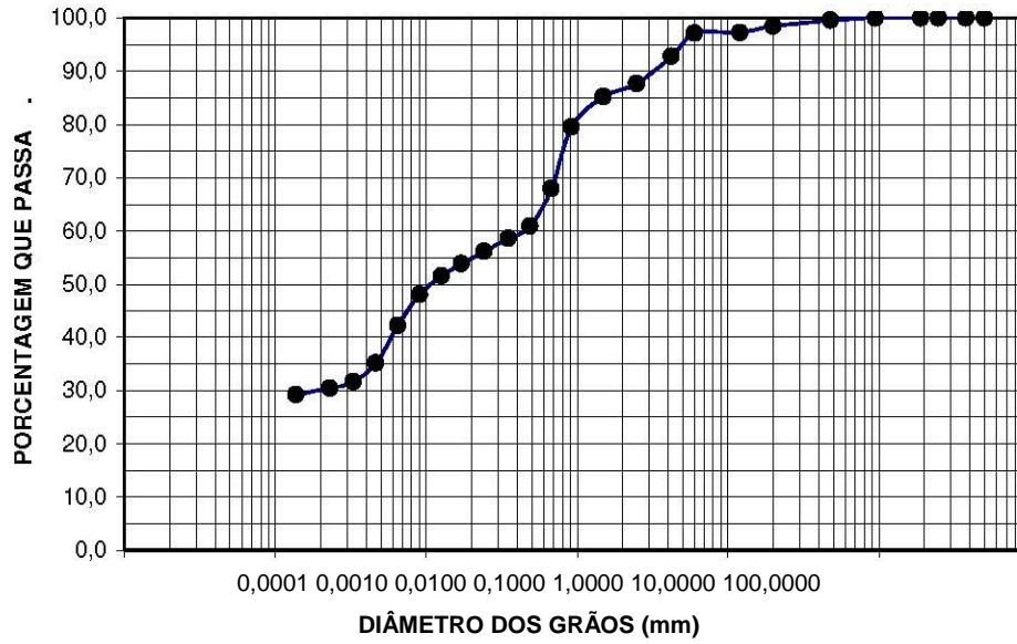
Figura 3.2: Curva granulométrica da amostra M3%.
