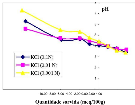
Figura 3.14: Diagrama da titulação potenciométrica para amostra M6%.
