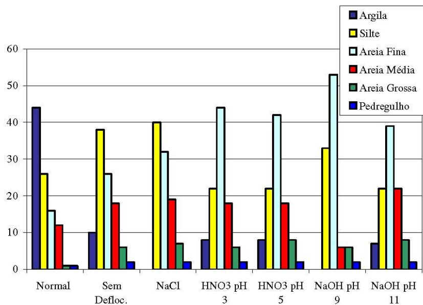
Figura 5.9: Frações granulométricas da amostra SN com diferentes soluções.
