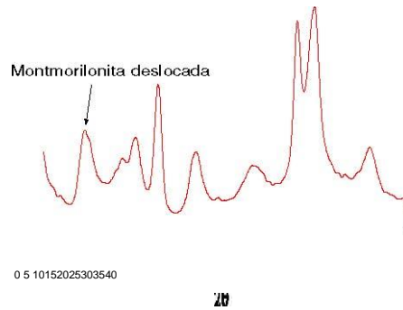
Figura 3.19: Difratoograma da bentonita (lâmina com etileno glicol).
