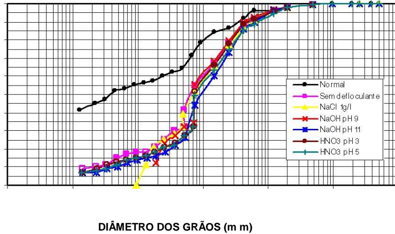
Figura 5.8: Curvas granulométricas da amostra SN com diferentes soluções.
