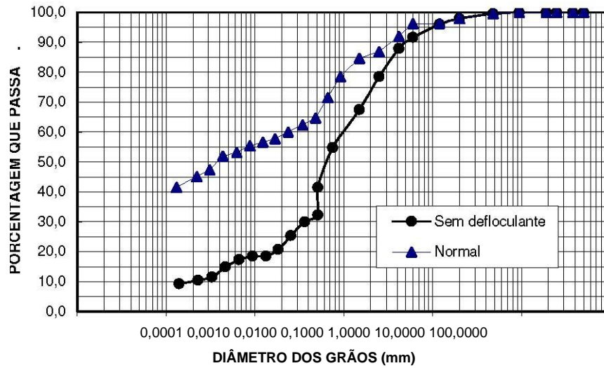
Figura 3.5: Comparação das curvas granulométricas de SN.
