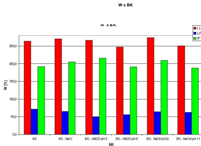
Figura 5.7: Variação de LL, LP e IP da amostra BK com diferentes fluidos.
