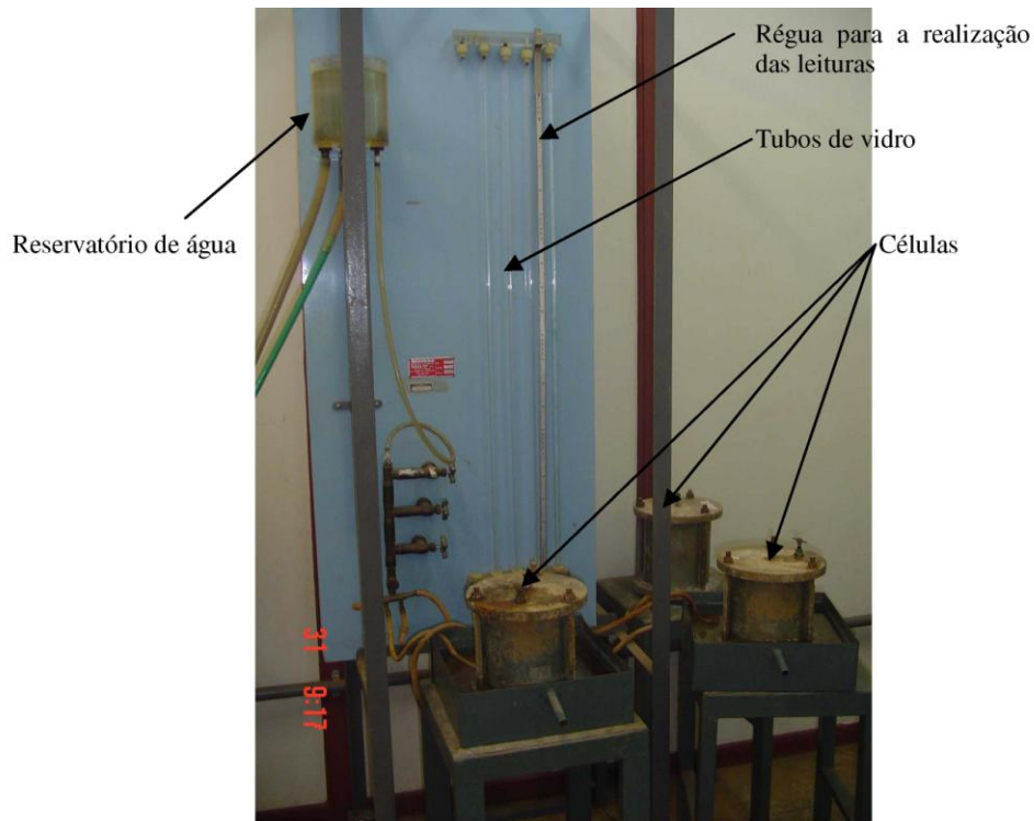
Figura 4.4: Aparato utilizado nas medidas da condutividade hidráulica das amostras.
