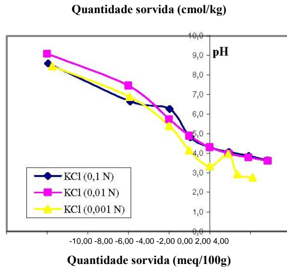
Figura 3.13: Diagrama da titulação potenciométrica para a amostra M3%.
