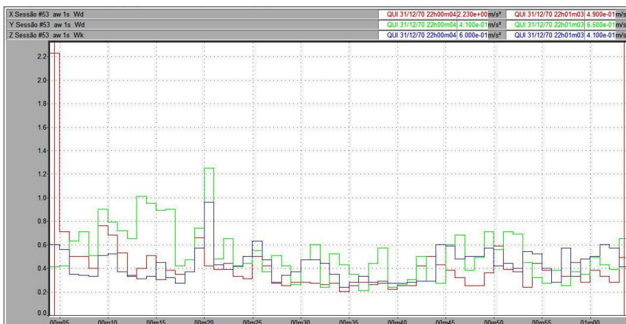
Figura 28 – Vibração no trator New Holland TL 75E no corpo inteiro, em pista de asfalto, com pressão de inflação dos pneus de 30 psi, na marcha II-2.
