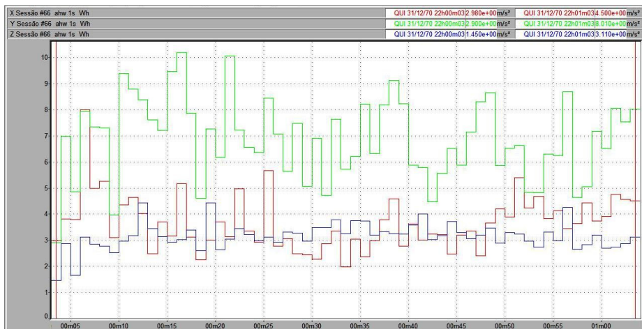
Figura 61 – Vibração no trator New Holland TL 75E no membro superior, em pista de asfalto, com pressão de inflação dos pneus de 25 psi, na marcha II-2.
