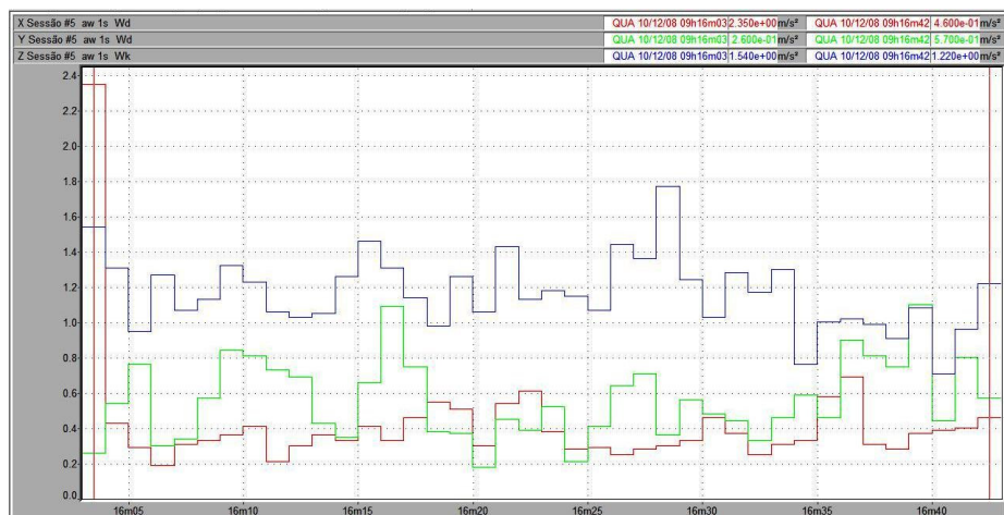
Figura 113 – Vibração no trator New Holland TS 110 no corpo inteiro, em pista de concreto, com pressão de inflação dos pneus de 30 psi, na marcha II-3.
