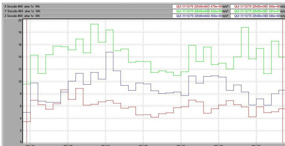
Figura 75 – Vibração no trator New Holland TL 75E no membro superior, em pista de concreto, com pressão de inflação dos pneus de 25 psi, na marcha II-4.
