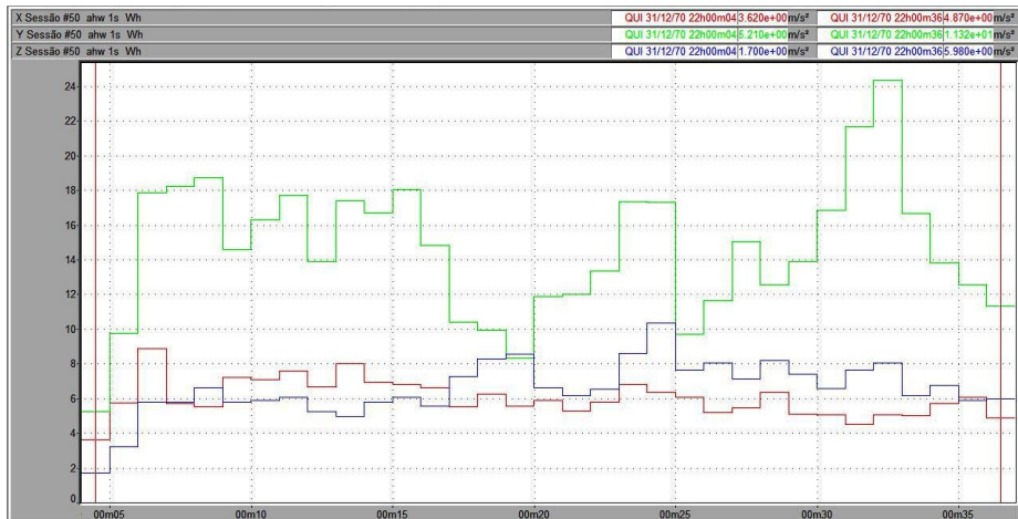
Figura 78 – Vibração no trator New Holland TL 75E no membro superior, em pista de concreto, com pressão de inflação dos pneus de 30 psi, na marcha II-4.
