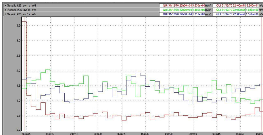
Figura 91 – Vibração no trator New Holland TS 110 no corpo inteiro, em pista de asfalto, com pressão de inflação dos pneus de 15 psi, na marcha II-2.
