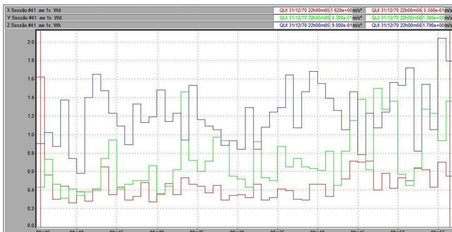
Figura 54 – Vibração no trator New Holland TL 75E no corpo inteiro, em pista de solo firme, com pressão de inflação dos pneus de 30 psi, na marcha II-4.
