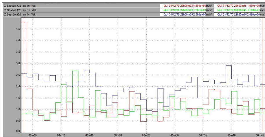
Figura 104 – Vibração no trator New Holland TS 110 no corpo inteiro, em pista de concreto, com pressão de inflação dos pneus de 15 psi, na marcha II-3.
