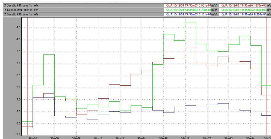
Figura 138 – Vibração no trator New Holland TS 110 no membro superior, em pista de asfalto, com pressão de inflação dos pneus de 30 psi, na marcha II-4.
