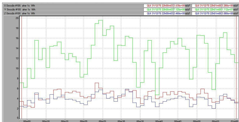
Figura 86 – Vibração no trator New Holland TL 75E no membro superior, em pista de solo firme, com pressão de inflação dos pneus de 25 psi, na marcha II-3.
