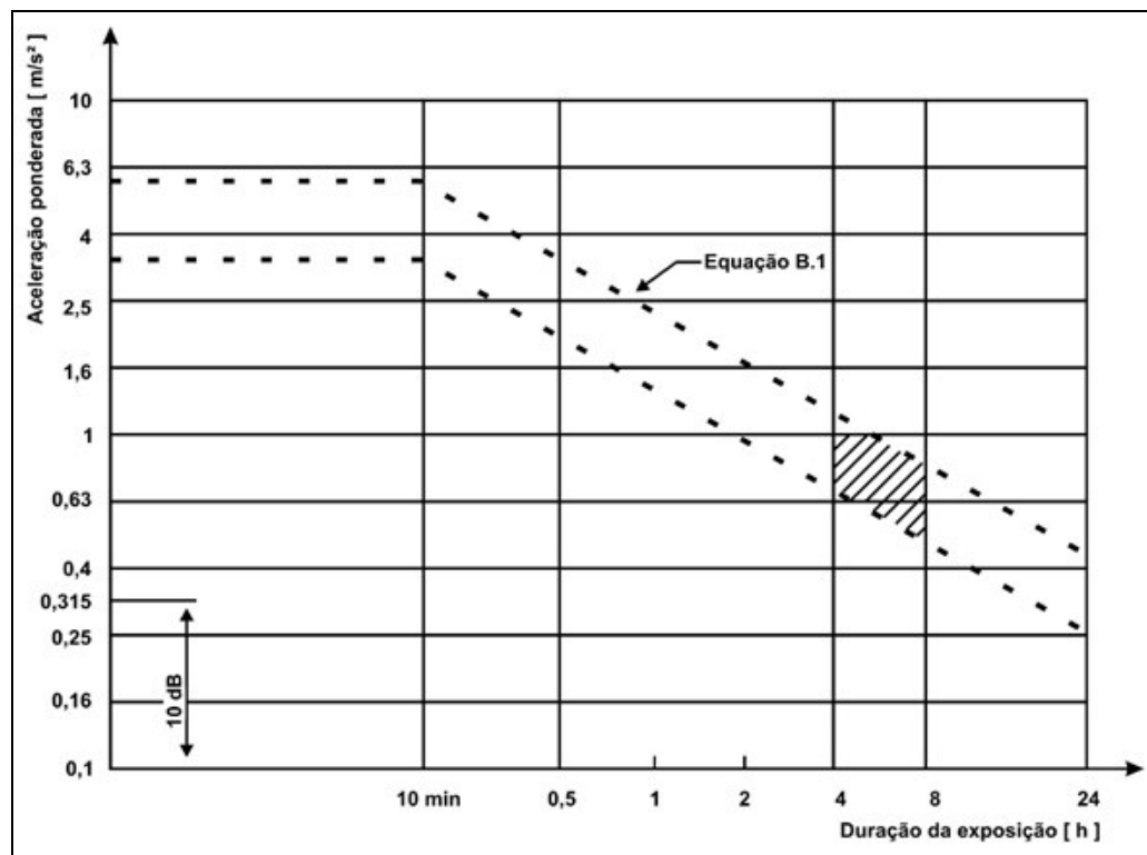
Figura 5 - Anexo B da ISO 2631/97 – guia à saúde – zonas de precaução.
