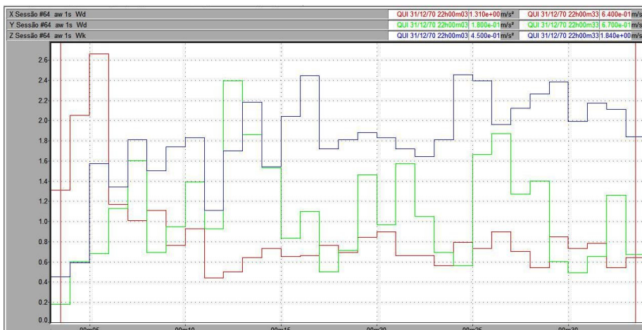
Figura 27 – Vibração no trator New Holland TL 75E no corpo inteiro, em pista de asfalto, com pressão de inflação dos pneus de 25 psi, na marcha II-4.
