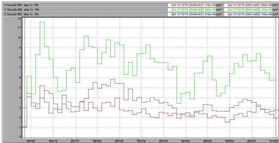
Figura 79 – Vibração no trator New Holland TL 75E no membro superior, em pista de solo firme, com pressão de inflação dos pneus de 15 psi, na marcha II-2.
