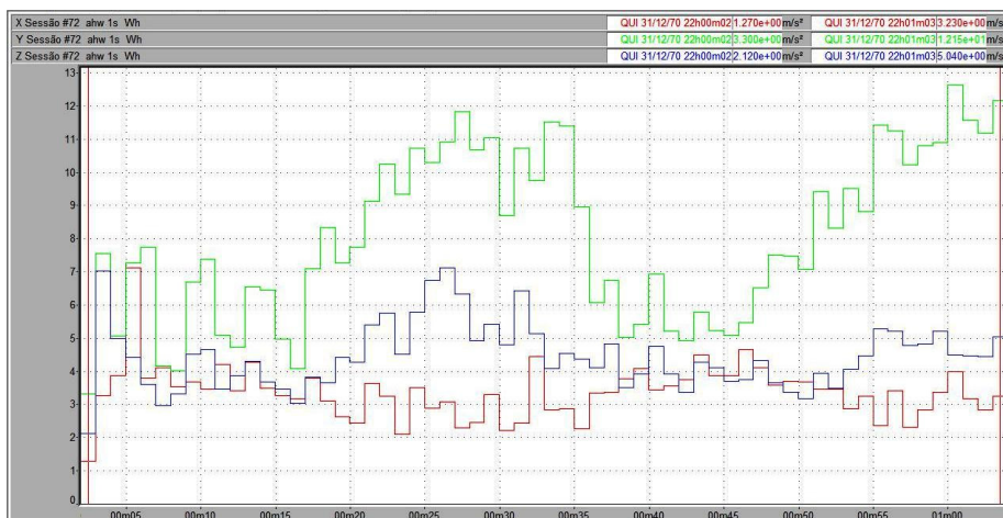
Figura 58 – Vibração no trator New Holland TL 75E no membro superior, em pista de asfalto, com pressão de inflação dos pneus de 20 psi, na marcha II-2.
