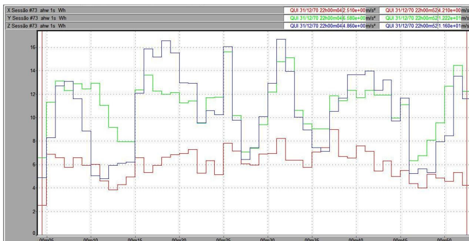
Figura 71 – Vibração no trator New Holland TL 75E no membro superior, em pista de concreto, com pressão de inflação dos pneus de 20 psi, na marcha II-3.
