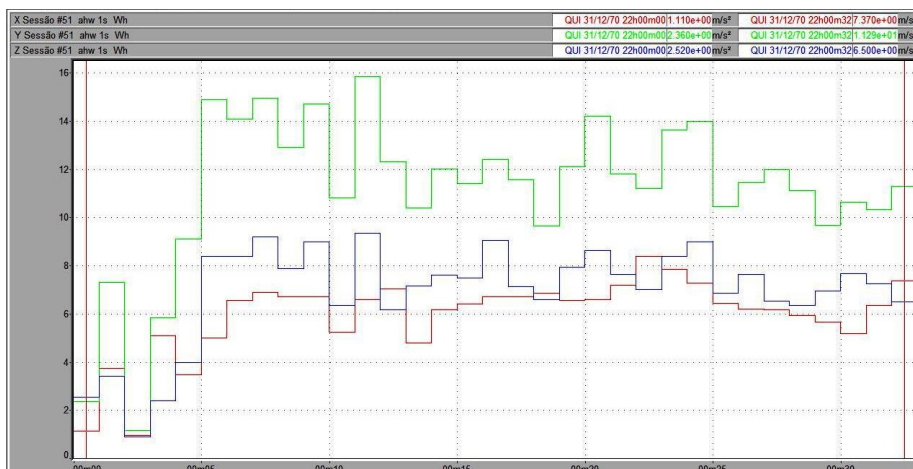
Figura 66 – Vibração no trator New Holland TL 75E no membro superior, em pista de asfalto, com pressão de inflação dos pneus de 30 psi, na marcha II-4.
