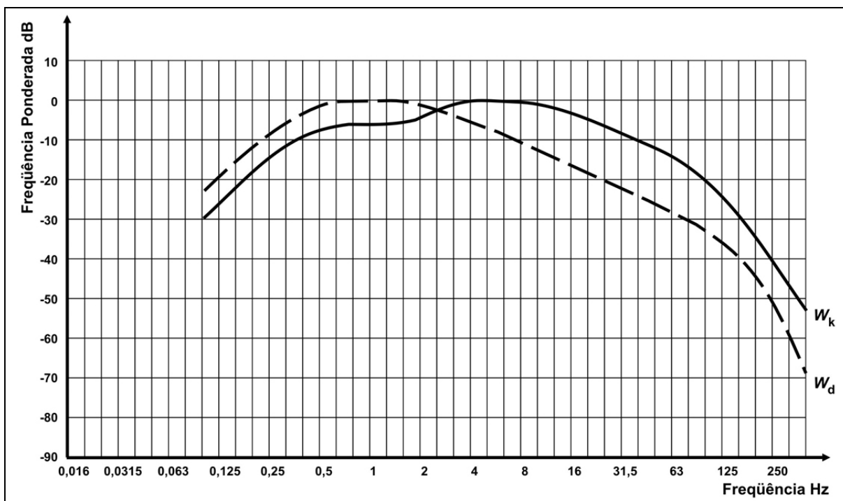
Figura 6 – Curva da frequência ponderada (dB) pela frequência (Hz), para os eixos x, y, e z.
