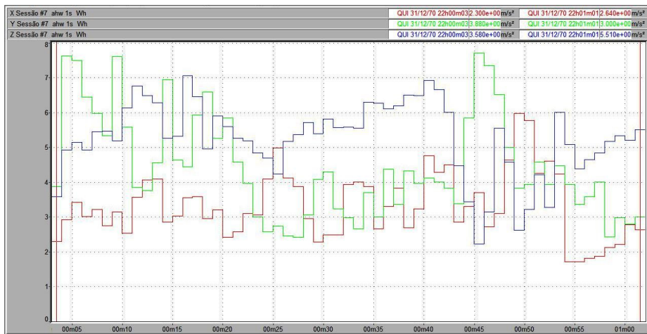
Figura 142 – Vibração no trator New Holland TS 110 no membro superior, em pista de concreto, com pressão de inflação dos pneus de 20 psi, na marcha II-2.
