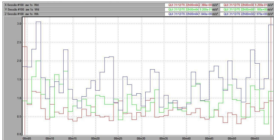
Figura 45 – Vibração no trator New Holland TL 75E no corpo inteiro, em pista de solo firme, com pressão de inflação dos pneus de 15 psi, na marcha II-4.
