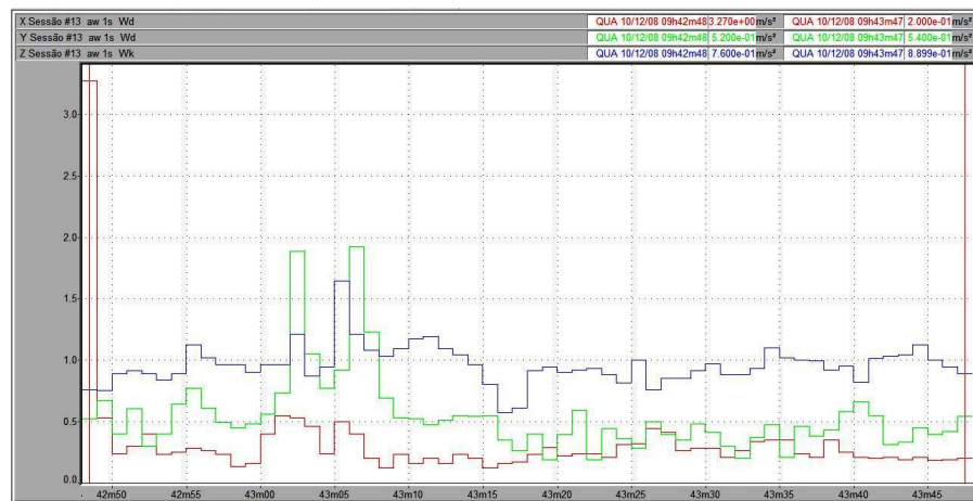
Figura 124 – Vibração no trator New Holland TS 110 no corpo inteiro, em pista de solo batido, com pressão de inflação dos pneus de 30 psi, na marcha II-2.
