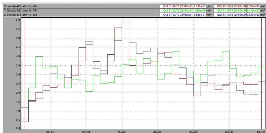
Figura 152 – Vibração no trator New Holland TS 110 no membro superior, em pista de solo firme, com pressão de inflação dos pneus de 15 psi, na marcha II-3.
