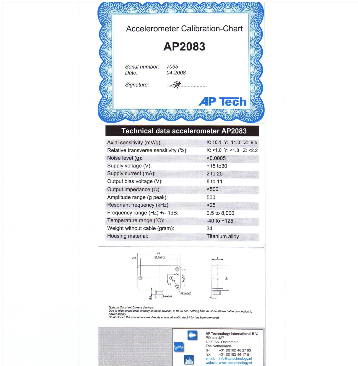
Figura 169 – Certificado de calibração do acelerômetro para corpo inteiro.
