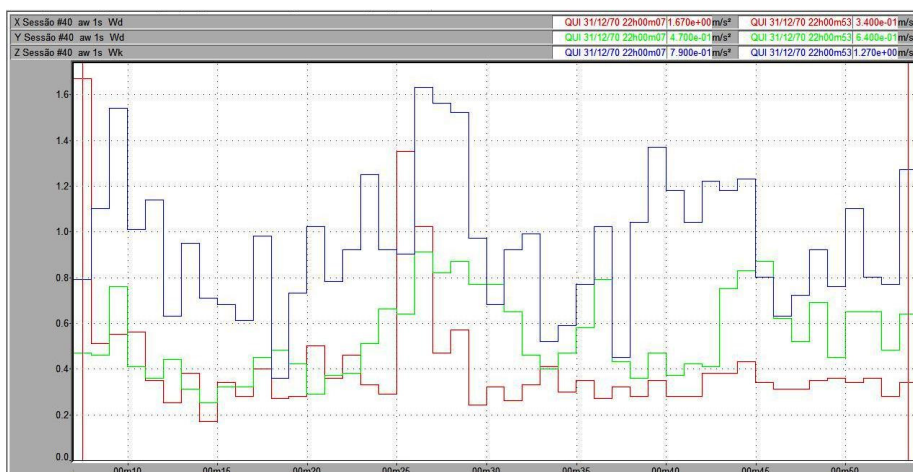
Figura 53 – Vibração no trator New Holland TL 75E no corpo inteiro, em pista de solo firme, com pressão de inflação dos pneus de 30 psi, na marcha II-3.
