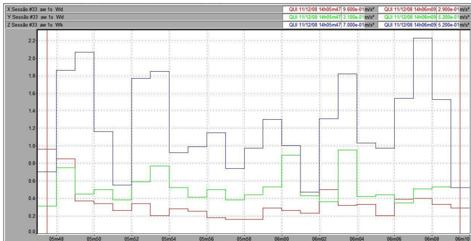
Figura 99 – Vibração no trator New Holland TS 110 no corpo inteiro, em pista de asfalto, com pressão de inflação dos pneus de 25 psi, na marcha II-4.
