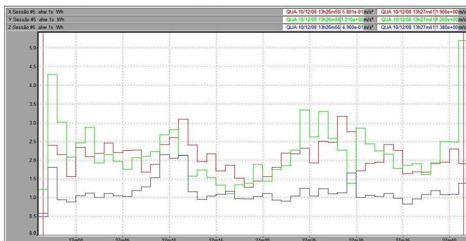
Figura 149 – Vibração no trator New Holland TS 110 no membro superior, em pista de concreto, com pressão de inflação dos pneus de 30 psi, na marcha II-3.
