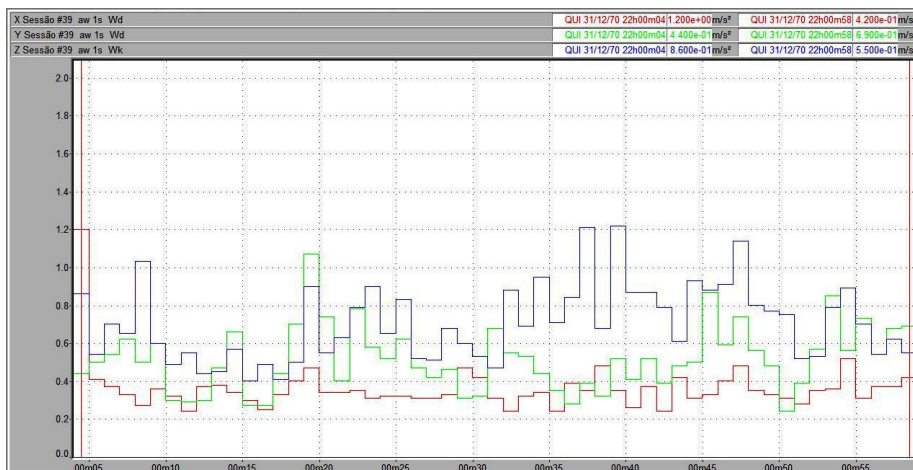
Figura 52 – Vibração no trator New Holland TL 75E no corpo inteiro, em pista de solo firme, com pressão de inflação dos pneus de 30 psi, na marcha II-2.
