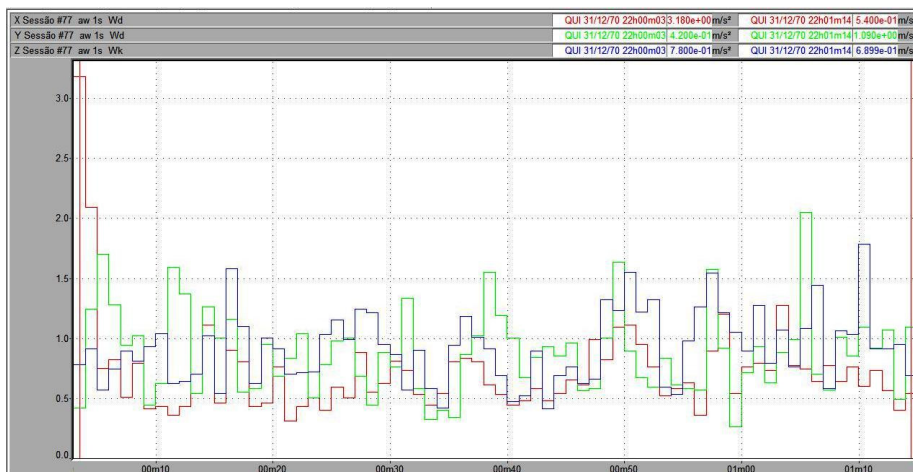
Figura 34 – Vibração no trator New Holland TL 75E no corpo inteiro, em pista de concreto, com pressão de inflação dos pneus de 20 psi, na marcha II-2.
