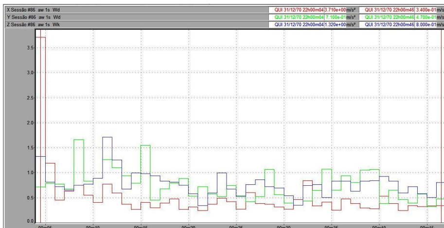
Figura 20 – Vibração no trator New Holland TL 75E no corpo inteiro, em pista de asfalto, com pressão de inflação dos pneus de 15 psi, na marcha II-3.
