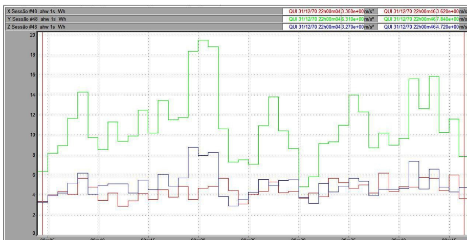
Figura 77 – Vibração no trator New Holland TL 75E no membro superior, em pista de concreto, com pressão de inflação dos pneus de 30 psi, na marcha II-3.
