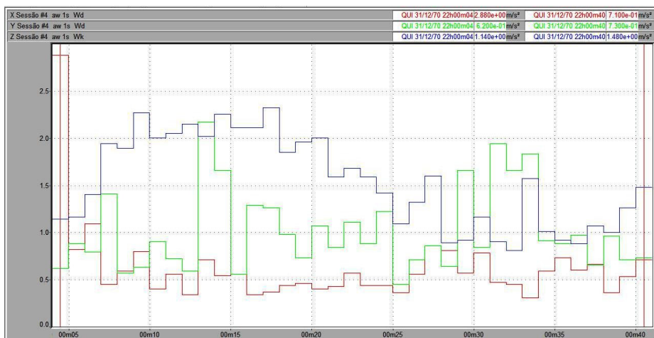
Figura 95 – Vibração no trator New Holland TS 110 no corpo inteiro, em pista de asfalto, com pressão de inflação dos pneus de 20 psi, na marcha II-3.
