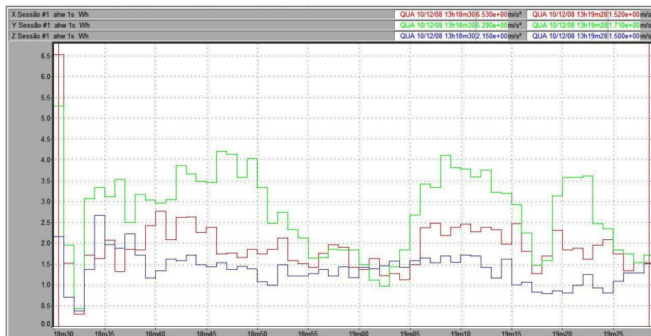
Figura 148 – Vibração no trator New Holland TS 110 no membro superior, em pista de concreto, com pressão de inflação dos pneus de 30 psi, na marcha II-2.
