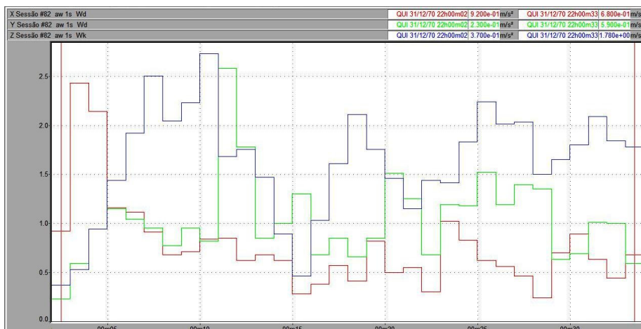
Figura 24 – Vibração no trator New Holland TL 75E no corpo inteiro, em pista de asfalto, com pressão de inflação dos pneus de 20 psi, na marcha II-4.
