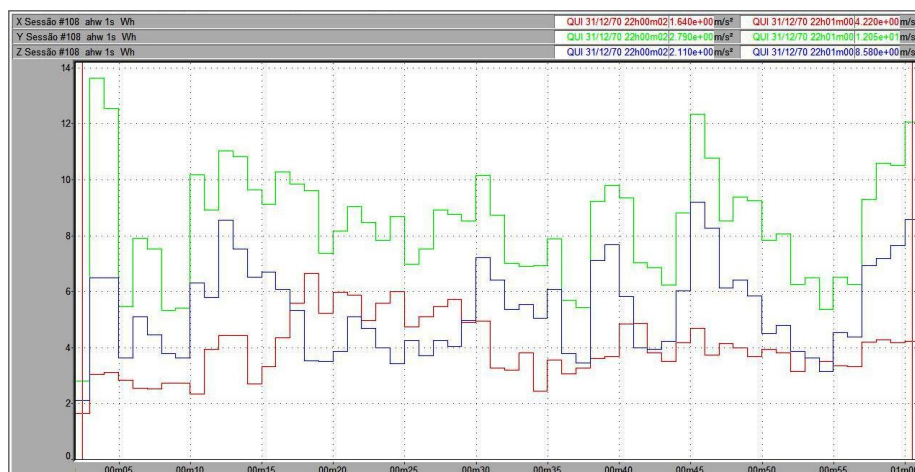
Figura 83 – Vibração no trator New Holland TL 75E no membro superior, em pista de solo firme, com pressão de inflação dos pneus de 20 psi, na marcha II-3.
