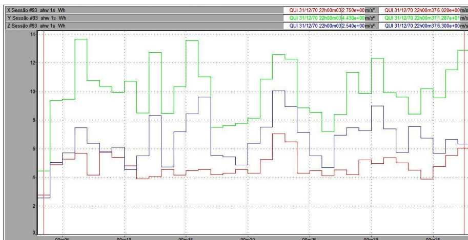
Figura 69 – Vibração no trator New Holland TL 75E no membro superior, em pista de concreto, com pressão de inflação dos pneus de 15 psi, na marcha II-4.
