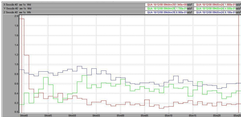
Figura 100 – Vibração no trator New Holland TS 110 no corpo inteiro, em pista de asfalto, com pressão de inflação dos pneus de 30 psi, na marcha II-2.
