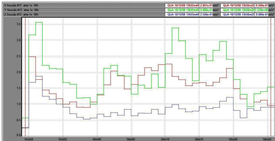
Figura 162 – Vibração no trator New Holland TS 110 no membro superior, em pista de solo firme, com pressão de inflação dos pneus de 30 psi, na marcha II-4.
