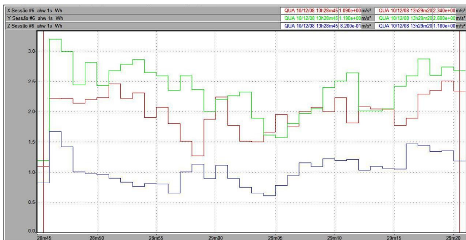
Figura 137 – Vibração no trator New Holland TS 110 no membro superior, em pista de asfalto, com pressão de inflação dos pneus de 30 psi, na marcha II-3.
