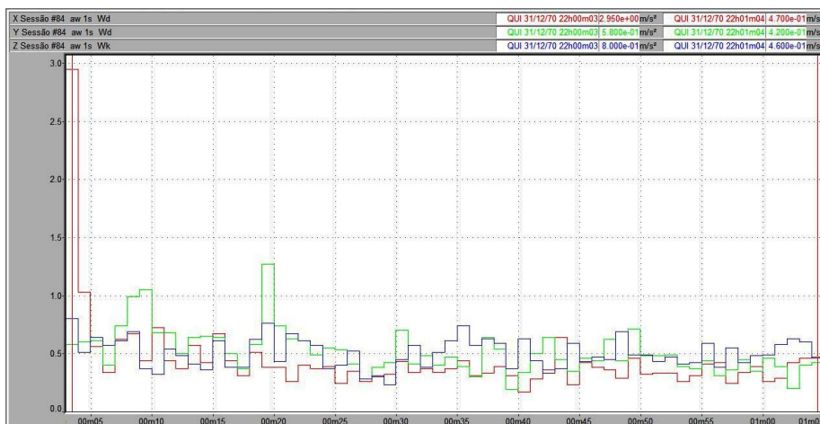
Figura 19 – Vibração no trator New Holland TL 75E no corpo inteiro, em pista de asfalto, com pressão de inflação dos pneus de 15 psi, na marcha II-2.
