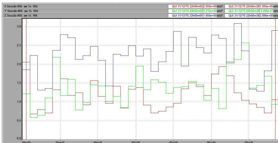
Figura 42 – Vibração no trator New Holland TL 75E no corpo inteiro, em pista de concreto, com pressão de inflação dos pneus de 30 psi, na marcha II-4.
