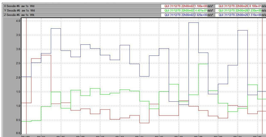
Figura 96 – Vibração no trator New Holland TS 110 no corpo inteiro, em pista de asfalto, com pressão de inflação dos pneus de 20 psi, na marcha II-4.
