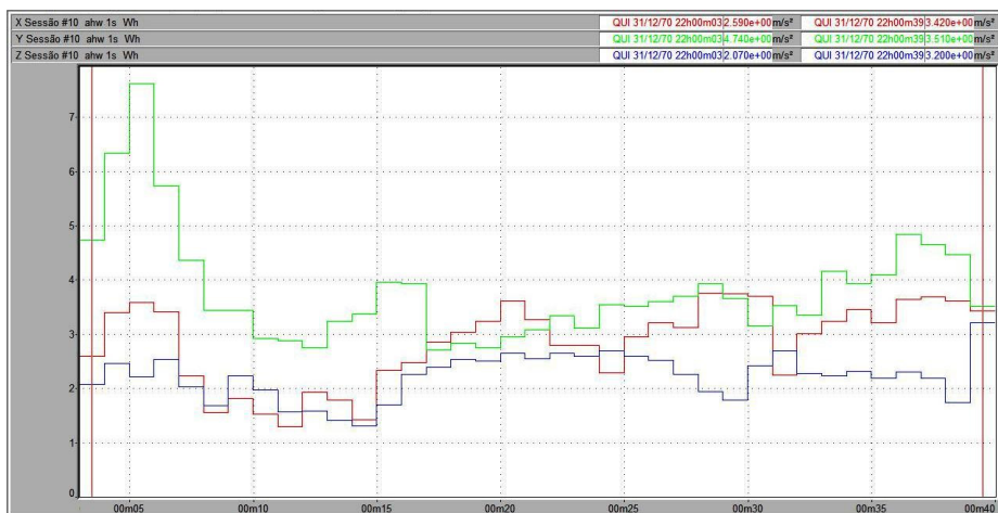
Figura 131 – Vibração no trator New Holland TS 110 no membro superior, em pista de asfalto, com pressão de inflação dos pneus de 20 psi, na marcha II-3.
