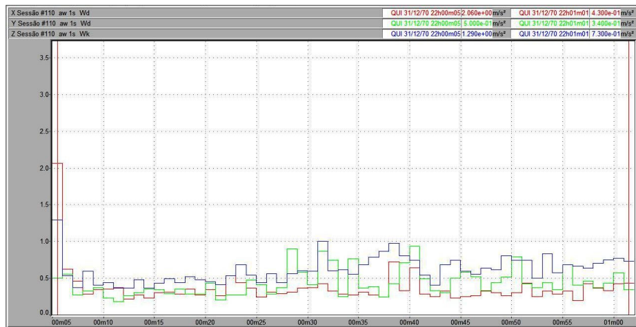
Figura 46 – Vibração no trator New Holland TL 75E no corpo inteiro, em pista de solo firme, com pressão de inflação dos pneus de 20 psi, na marcha II-2.
