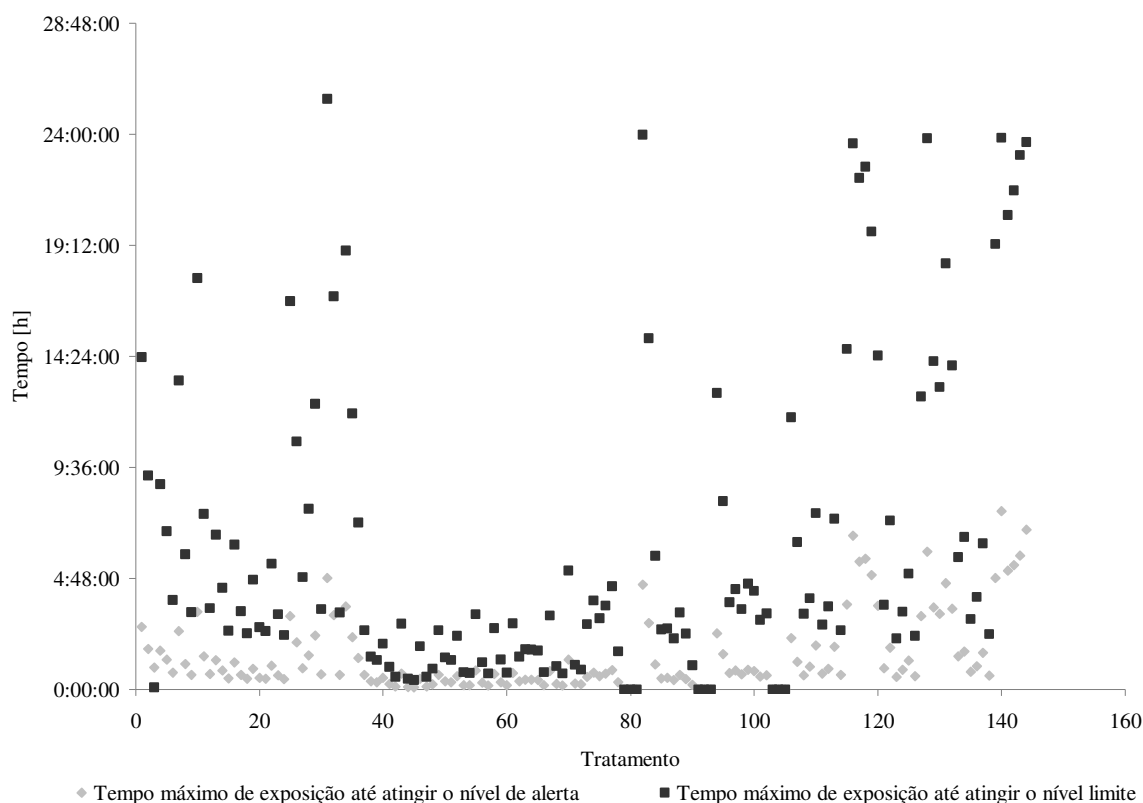
Figura 15 – Comparação entre os tempos de operação para se atingir os níveis de alerta e limite.
