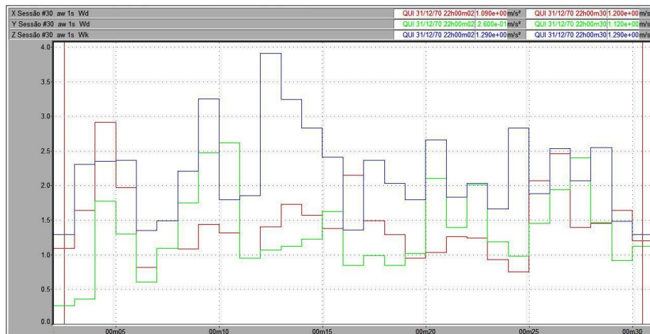
Figura 105 – Vibração no trator New Holland TS 110 no corpo inteiro, em pista de concreto, com pressão de inflação dos pneus de 15 psi, na marcha II-4.
