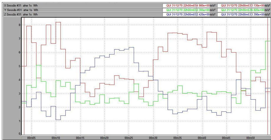
Figura 127 – Vibração no trator New Holland TS 110 no membro superior, em pista de asfalto, com pressão de inflação dos pneus de 15 psi, na marcha II-2.
