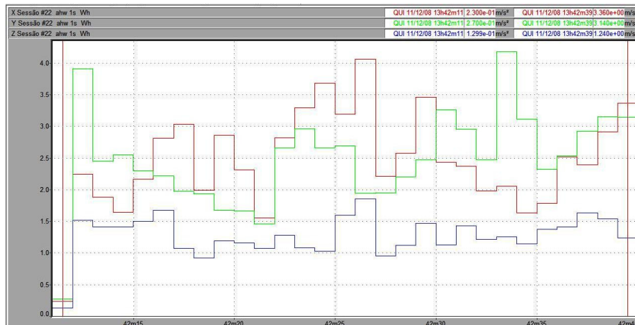
Figura 147 – Vibração no trator New Holland TS 110 no membro superior, em pista de concreto, com pressão de inflação dos pneus de 25 psi, na marcha II-4.
