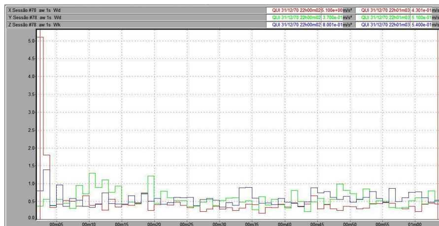
Figura 22 – Vibração no trator New Holland TL 75E no corpo inteiro, em pista de asfalto, com pressão de inflação dos pneus de 20 psi, na marcha II-2.
