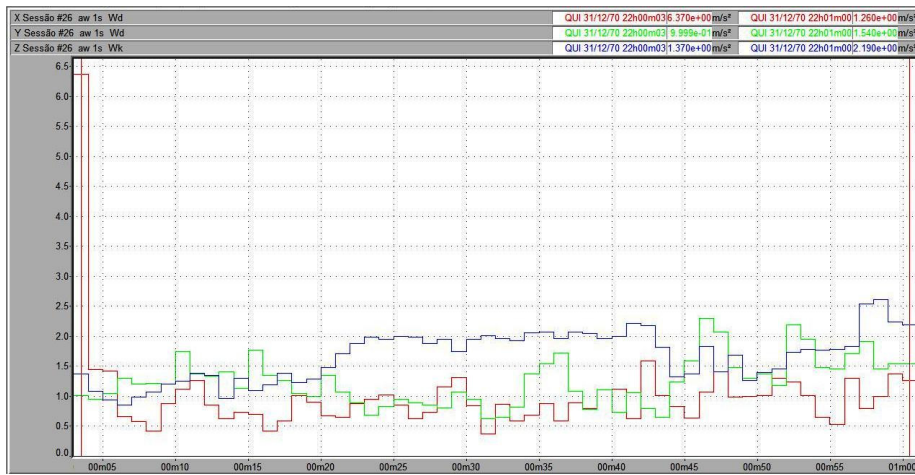
Figura 103 – Vibração no trator New Holland TS 110 no corpo inteiro, em pista de concreto, com pressão de inflação dos pneus de 15 psi, na marcha II-2.
