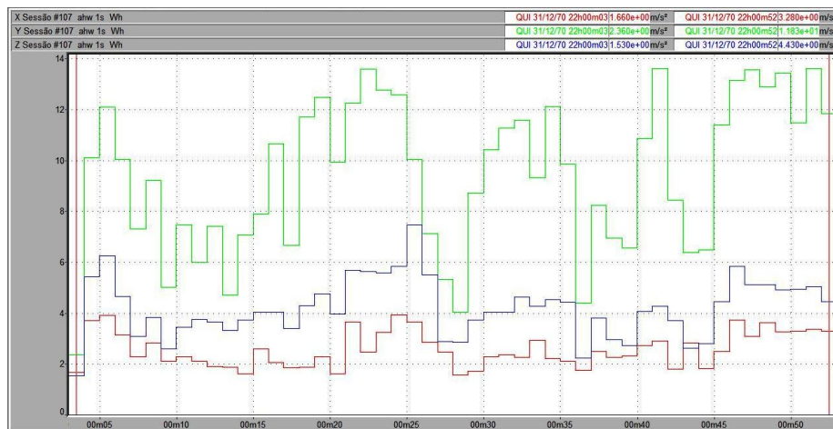
Figura 82 – Vibração no trator New Holland TL 75E no membro superior, em pista de solo firme, com pressão de inflação dos pneus de 20 psi, na marcha II-2.
