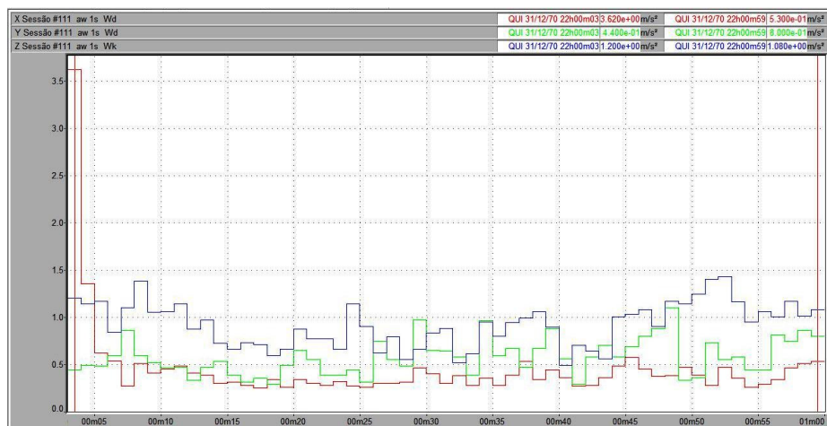
Figura 47 – Vibração no trator New Holland TL 75E no corpo inteiro, em pista de solo firme, com pressão de inflação dos pneus de 20 psi, na marcha II-3.
