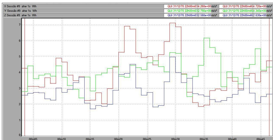
Figura 143 – Vibração no trator New Holland TS 110 no membro superior, em pista de concreto, com pressão de inflação dos pneus de 20 psi, na marcha II-3.
