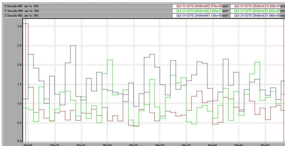
Figura 32 – Vibração no trator New Holland TL 75E no corpo inteiro, em pista de concreto, com pressão de inflação dos pneus de 15 psi, na marcha II-3.
