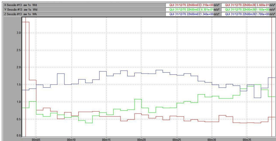
Figura 118 – Vibração no trator New Holland TS 110 no corpo inteiro, em pista de solo batido, com pressão de inflação dos pneus de 20 psi, na marcha II-2.
