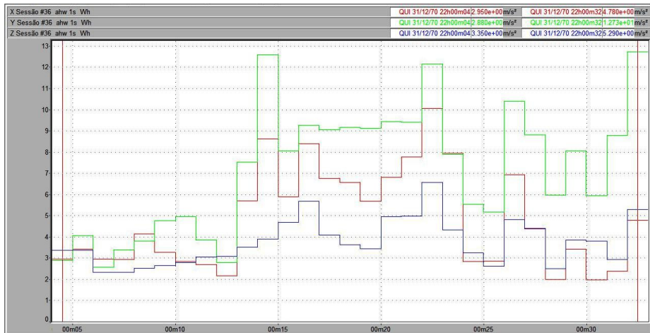
Figura 141 – Vibração no trator New Holland TS 110 no membro superior, em pista de concreto, com pressão de inflação dos pneus de 15 psi, na marcha II-4.
