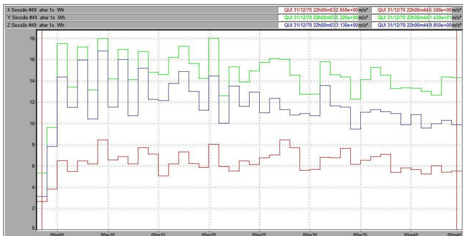
Figura 65 – Vibração no trator New Holland TL 75E no membro superior, em pista de asfalto, com pressão de inflação dos pneus de 30 psi, na marcha II-3.
