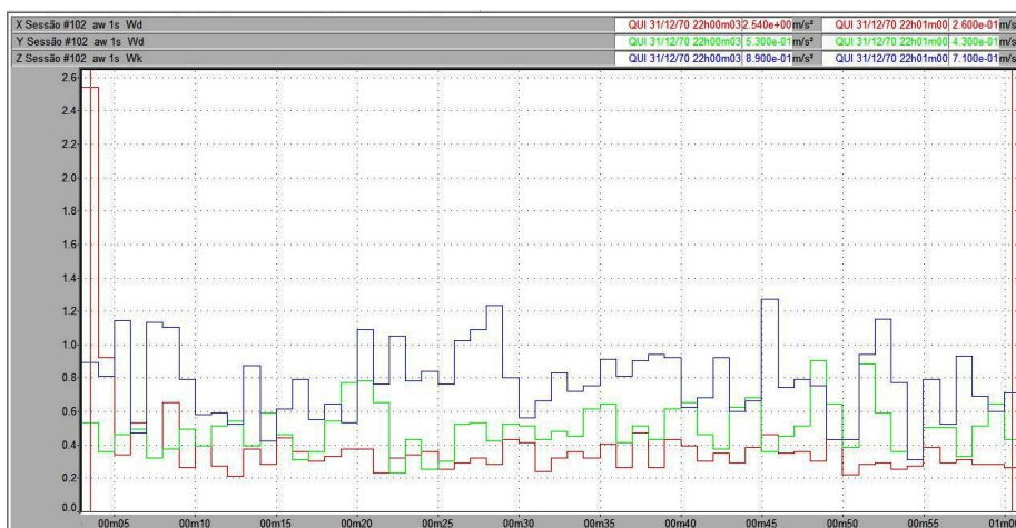
Figura 50 – Vibração no trator New Holland TL 75E no corpo inteiro, em pista de solo firme, com pressão de inflação dos pneus de 25 psi, na marcha II-3.
