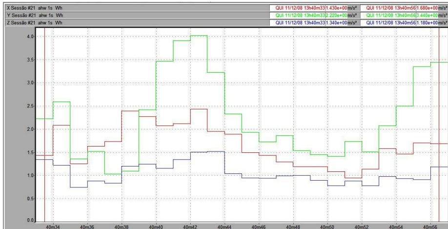
Figura 135 – Vibração no trator New Holland TS 110 no membro superior, em pista de asfalto, com pressão de inflação dos pneus de 25 psi, na marcha II-4.
