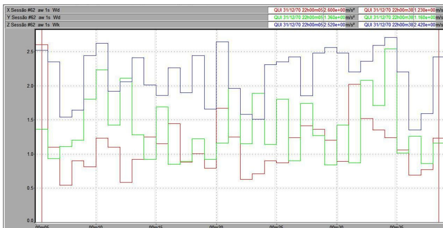
Figura 39 – Vibração no trator New Holland TL 75E no corpo inteiro, em pista de concreto, com pressão de inflação dos pneus de 25 psi, na marcha II-4.
