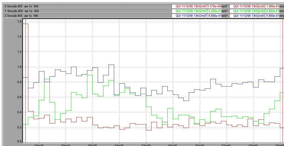
Figura 97 – Vibração no trator New Holland TS 110 no corpo inteiro, em pista de asfalto, com pressão de inflação dos pneus de 25 psi, na marcha II-2.
