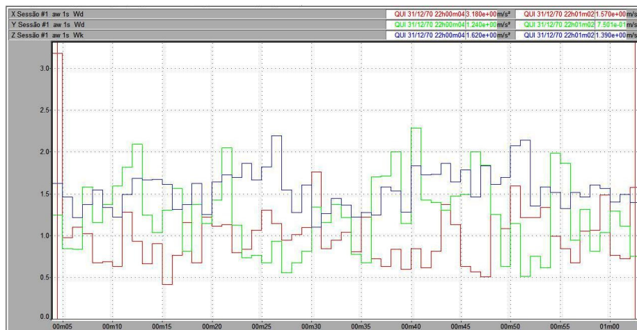
Figura 106 – Vibração no trator New Holland TS 110 no corpo inteiro, em pista de concreto, com pressão de inflação dos pneus de 20 psi, na marcha II-2.
