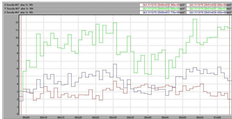
Figura 64 – Vibração no trator New Holland TL 75E no membro superior, em pista de asfalto, com pressão de inflação dos pneus de 30 psi, na marcha II-2.
