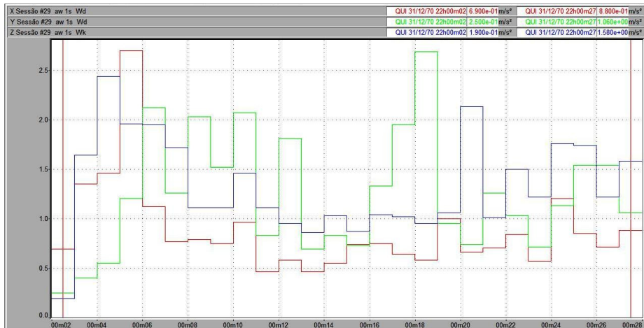
Figura 93 – Vibração no trator New Holland TS 110 no corpo inteiro, em pista de asfalto, com pressão de inflação dos pneus de 15 psi, na marcha II-4.
