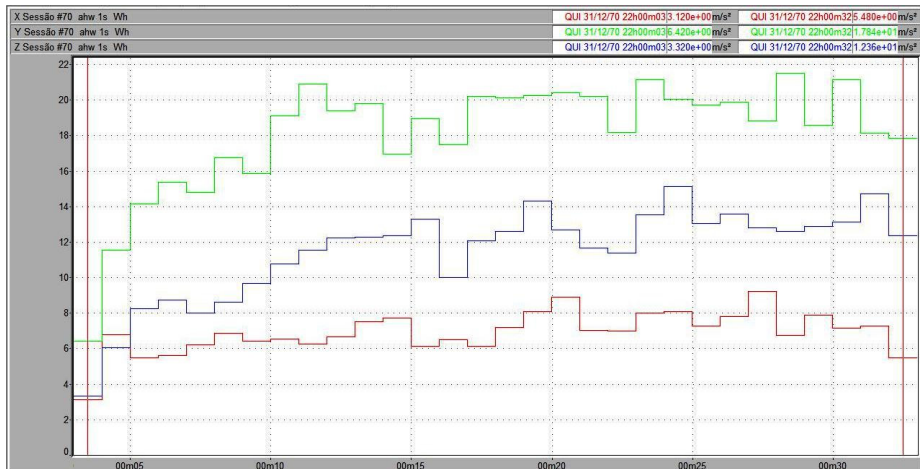
Figura 63 – Vibração no trator New Holland TL 75E no membro superior, em pista de asfalto, com pressão de inflação dos pneus de 25 psi, na marcha II-4.
