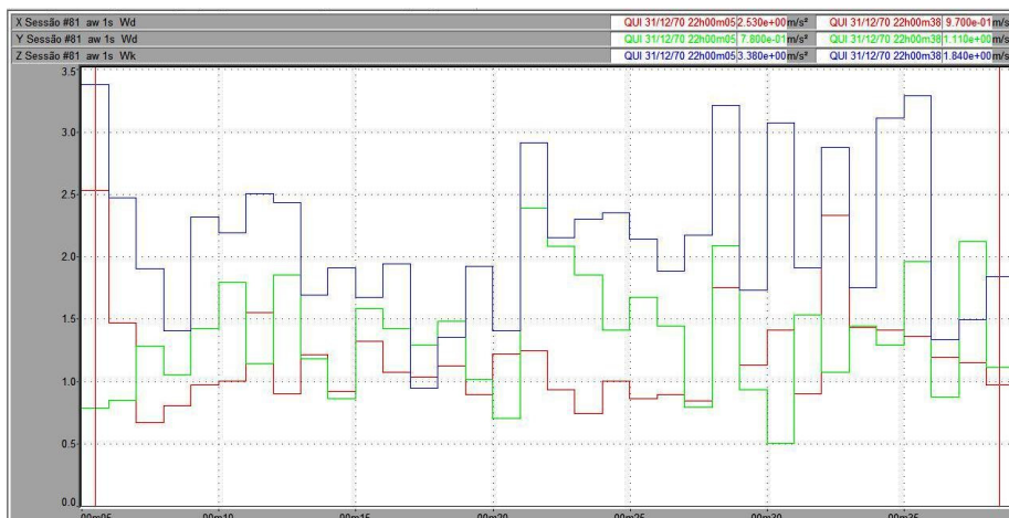
Figura 36 – Vibração no trator New Holland TL 75E no corpo inteiro, em pista de concreto, com pressão de inflação dos pneus de 20 psi, na marcha II-4.
