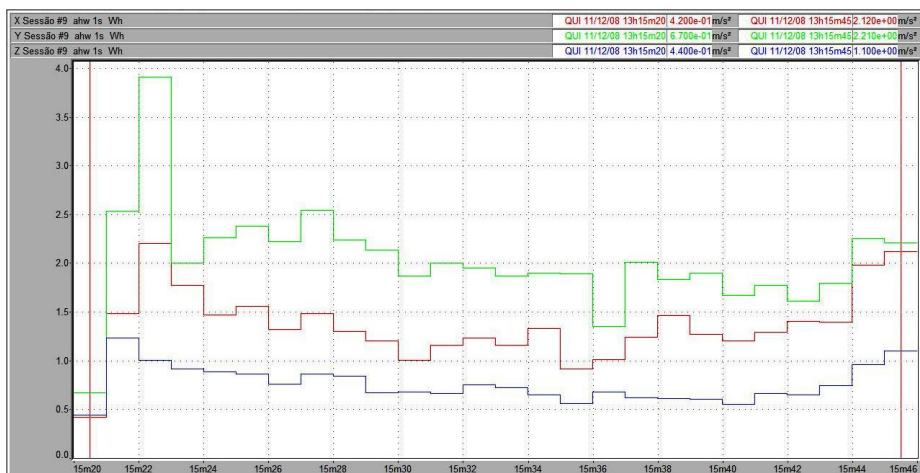
Figura 158 – Vibração no trator New Holland TS 110 no membro superior, em pista de solo firme, com pressão de inflação dos pneus de 125 psi, na marcha II-3.
