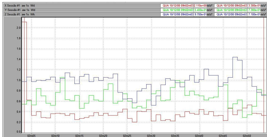
Figura 112 – Vibração no trator New Holland TS 110 no corpo inteiro, em pista de concreto, com pressão de inflação dos pneus de 30 psi, na marcha II-2.
