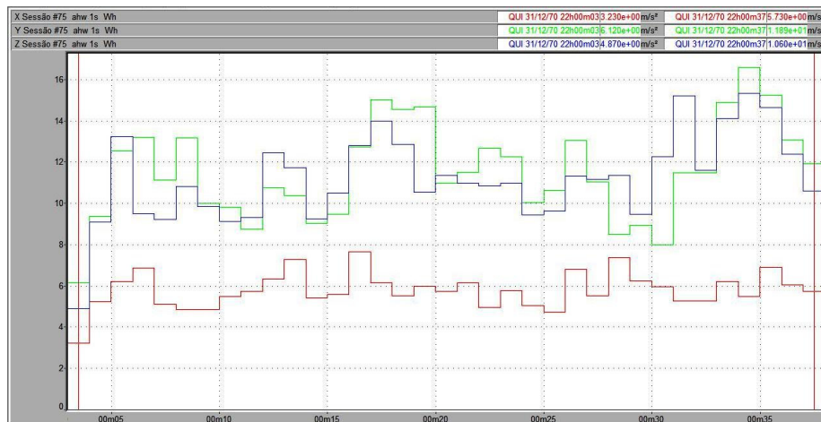
Figura 72 – Vibração no trator New Holland TL 75E no membro superior, em pista de concreto, com pressão de inflação dos pneus de 20 psi, na marcha II-4.
