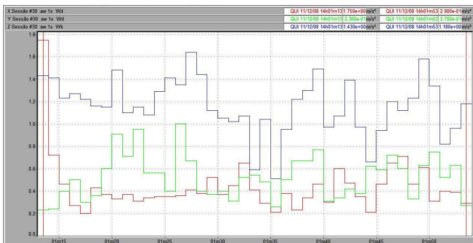
Figura 110 – Vibração no trator New Holland TS 110 no corpo inteiro, em pista de concreto, com pressão de inflação dos pneus de 25 psi, na marcha II-3.
