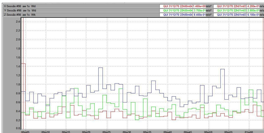
Figura 43 – Vibração no trator New Holland TL 75E no corpo inteiro, em pista de solo firme, com pressão de inflação dos pneus de 15 psi, na marcha II-2.
