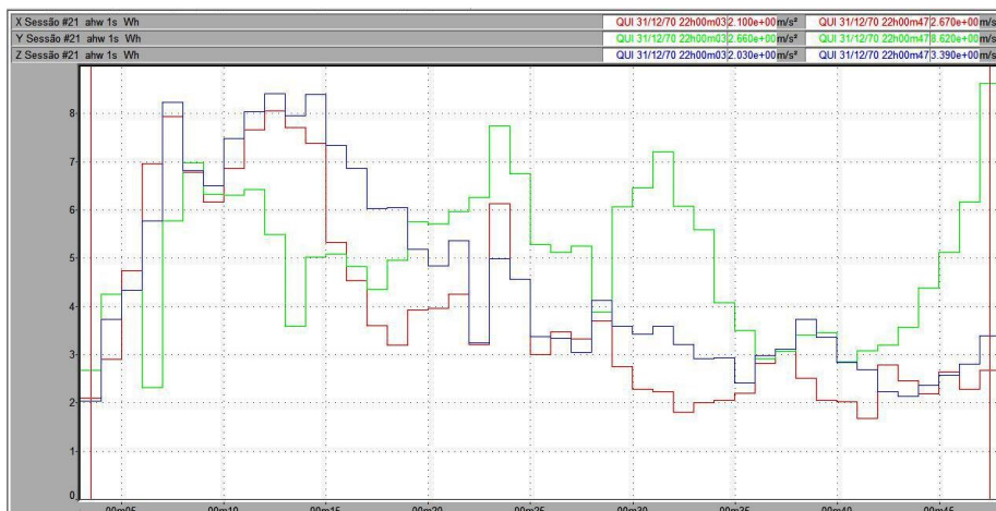
Figura 153 – Vibração no trator New Holland TS 110 no membro superior, em pista de solo firme, com pressão de inflação dos pneus de 15 psi, na marcha II-4.
