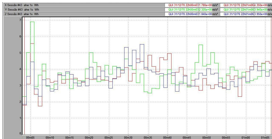
Figura 88 – Vibração no trator New Holland TL 75E no membro superior, em pista de solo firme, com pressão de inflação dos pneus de 30 psi, na marcha II-2.
