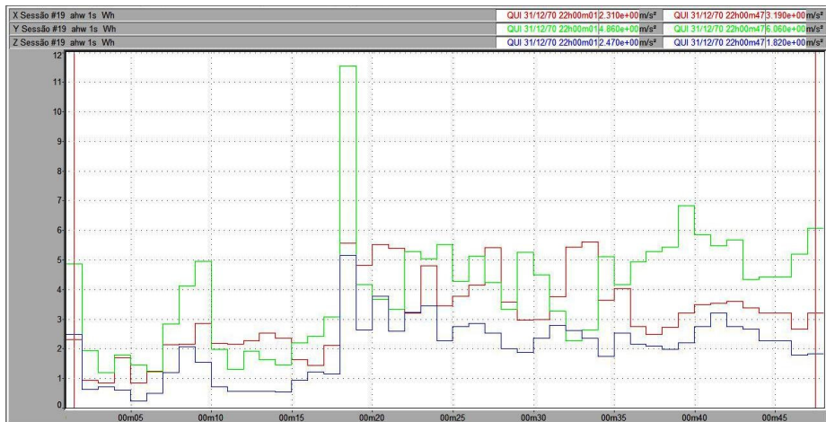
Figura 151 – Vibração no trator New Holland TS 110 no membro superior, em pista de solo firme, com pressão de inflação dos pneus de 15 psi, na marcha II-2.
