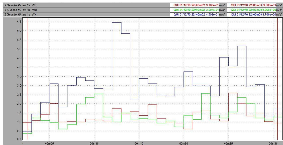
Figura 108 – Vibração no trator New Holland TS 110 no corpo inteiro, em pista de concreto, com pressão de inflação dos pneus de 20 psi, na marcha II-4.
