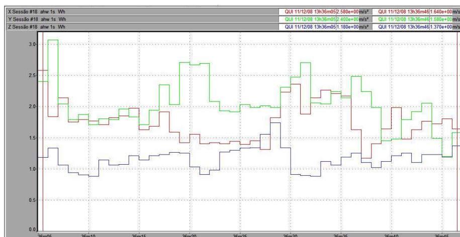
Figura 146 – Vibração no trator New Holland TS 110 no membro superior, em pista de concreto, com pressão de inflação dos pneus de 25 psi, na marcha II-3.
