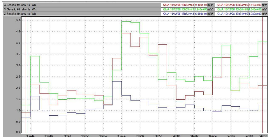
Figura 150 – Vibração no trator New Holland TS 110 no membro superior, em pista de concreto, com pressão de inflação dos pneus de 30 psi, na marcha II-4.
