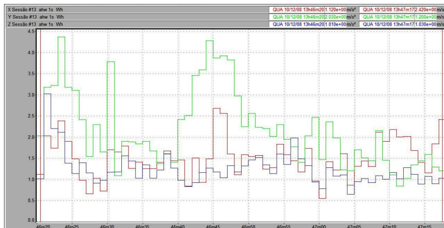
Figura 160 – Vibração no trator New Holland TS 110 no membro superior, em pista de solo firme, com pressão de inflação dos pneus de 30 psi, na marcha II-2.
