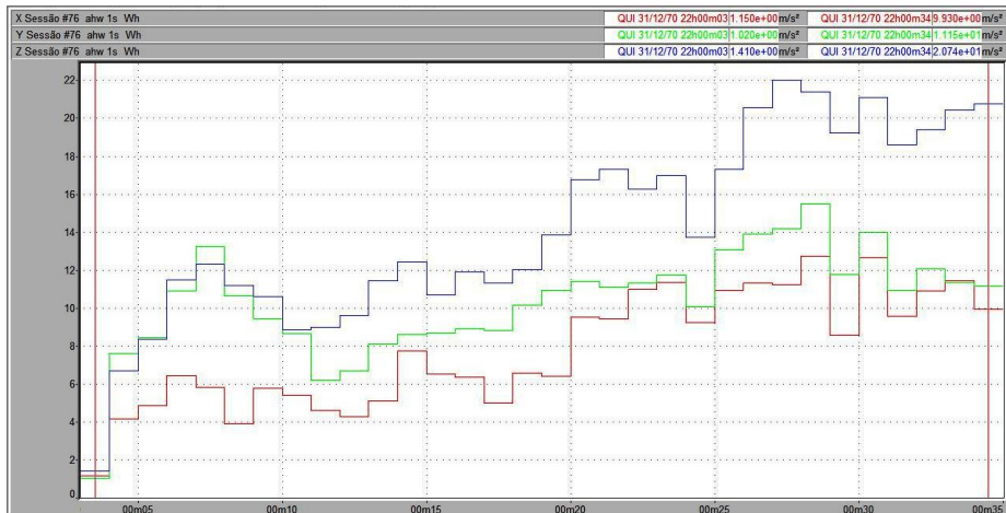
Figura 60 – Vibração no trator New Holland TL 75E no membro superior, em pista de asfalto, com pressão de inflação dos pneus de 20 psi, na marcha II-4.
