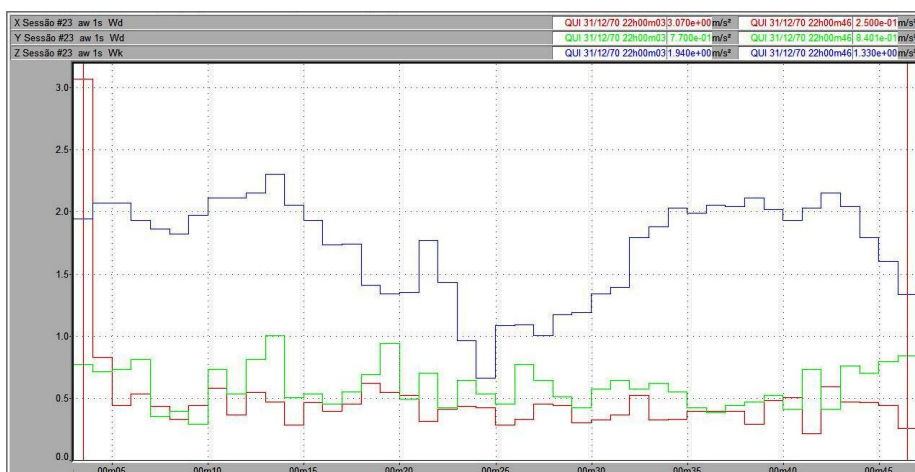
Figura 116 – Vibração no trator New Holland TS 110 no corpo inteiro, em pista de solo batido, com pressão de inflação dos pneus de 15 psi, na marcha II-3.
