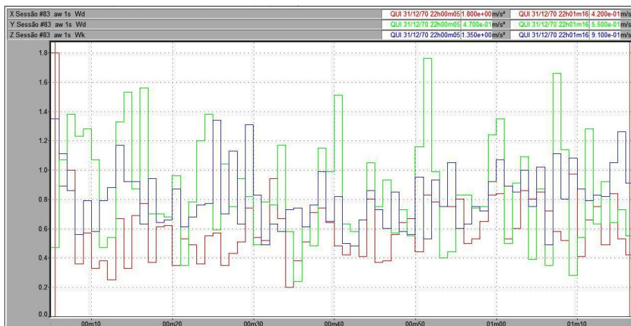
Figura 31 – Vibração no trator New Holland TL 75E no corpo inteiro, em pista de concreto, com pressão de inflação dos pneus de 15 psi, na marcha II-2.
