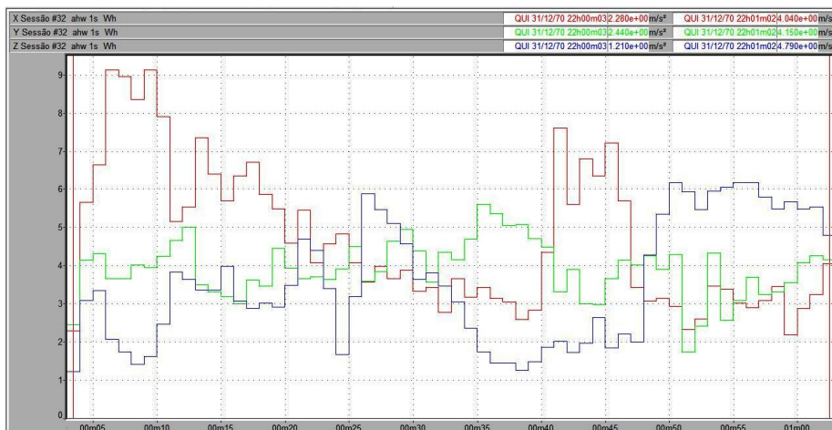
Figura 139 – Vibração no trator New Holland TS 110 no membro superior, em pista de concreto, com pressão de inflação dos pneus de 15 psi, na marcha II-2.
