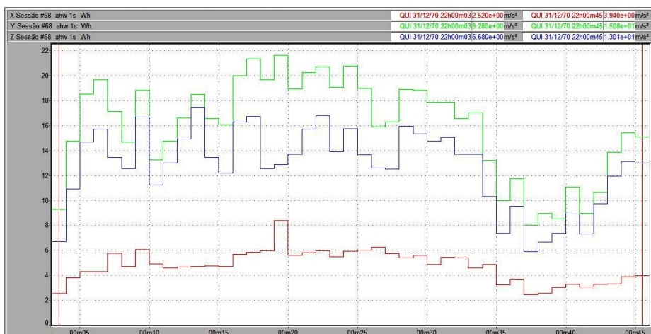
Figura 62 – Vibração no trator New Holland TL 75E no membro superior, em pista de asfalto, com pressão de inflação dos pneus de 25 psi, na marcha II-3.
