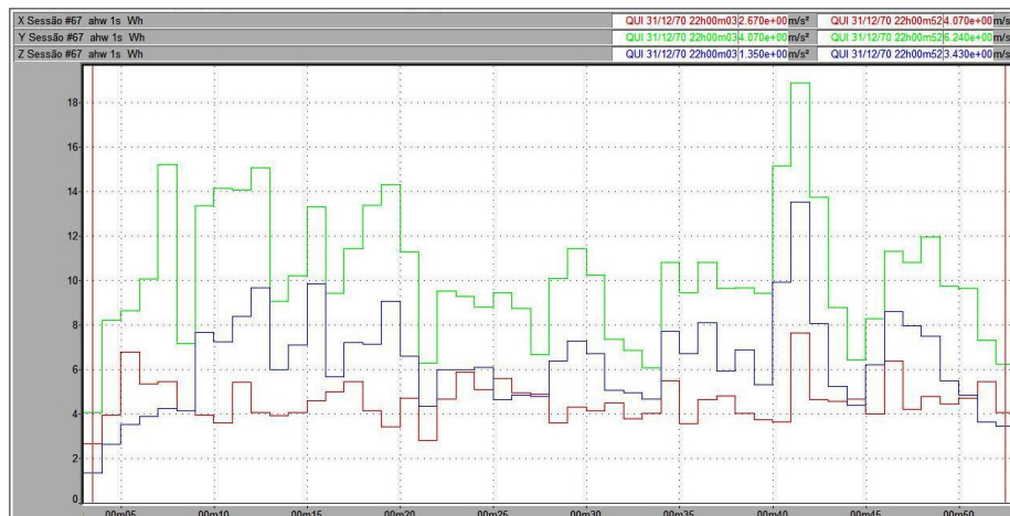
Figura 74 – Vibração no trator New Holland TL 75E no membro superior, em pista de concreto, com pressão de inflação dos pneus de 25 psi, na marcha II-3.
