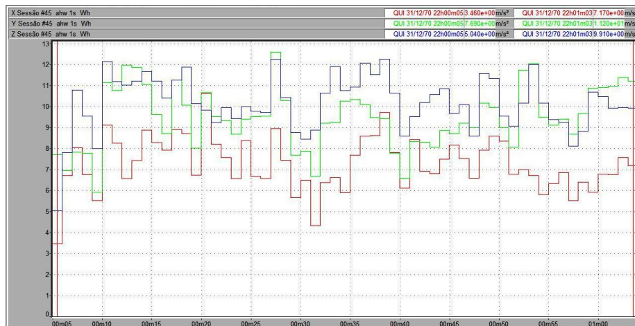
Figura 90 – Vibração no trator New Holland TL 75E no membro superior, em pista de solo firme, com pressão de inflação dos pneus de 30 psi, na marcha II-4.
