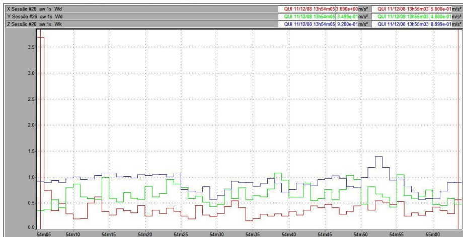
Figura 109 – Vibração no trator New Holland TS 110 no corpo inteiro, em pista de concreto, com pressão de inflação dos pneus de 25 psi, na marcha II-2.
