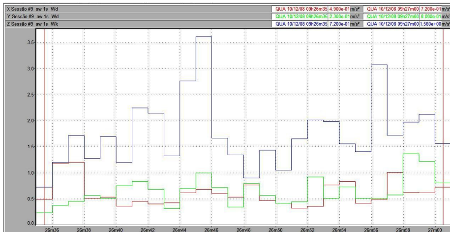
Figura 114 – Vibração no trator New Holland TS 110 no corpo inteiro, em pista de concreto, com pressão de inflação dos pneus de 30 psi, na marcha II-4.
