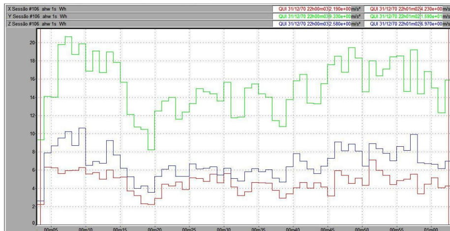
Figura 87 – Vibração no trator New Holland TL 75E no membro superior, em pista de solo firme, com pressão de inflação dos pneus de 25 psi, na marcha II-4.
