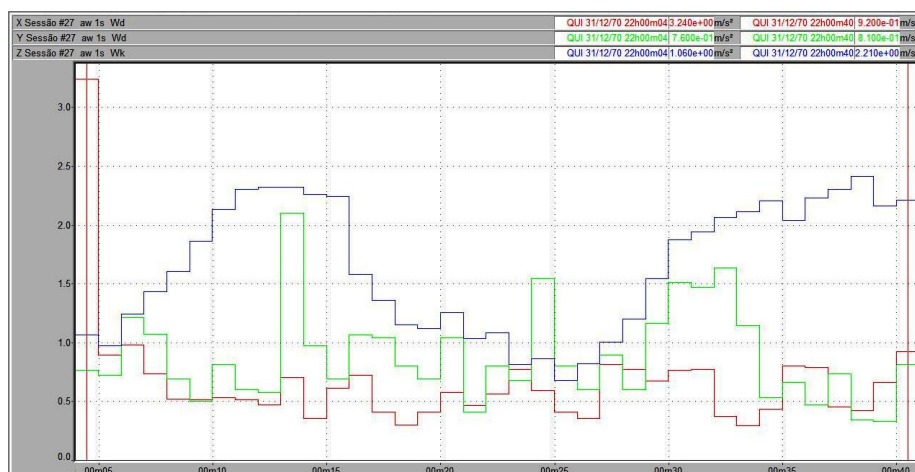
Figura 92 – Vibração no trator New Holland TS 110 no corpo inteiro, em pista de asfalto, com pressão de inflação dos pneus de 15 psi, na marcha II-3.
