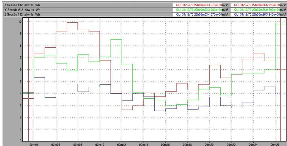
Figura 132 – Vibração no trator New Holland TS 110 no membro superior, em pista de asfalto, com pressão de inflação dos pneus de 20 psi, na marcha II-4.
