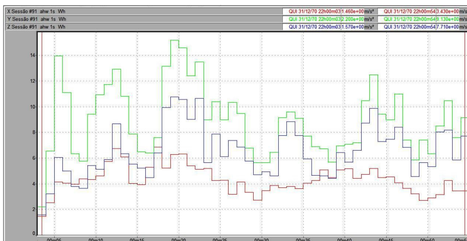
Figura 68 – Vibração no trator New Holland TL 75E no membro superior, em pista de concreto, com pressão de inflação dos pneus de 15 psi, na marcha II-3.
