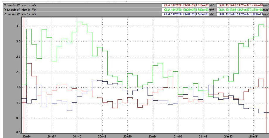
Figura 136 – Vibração no trator New Holland TS 110 no membro superior, em pista de asfalto, com pressão de inflação dos pneus de 30 psi, na marcha II-2.
