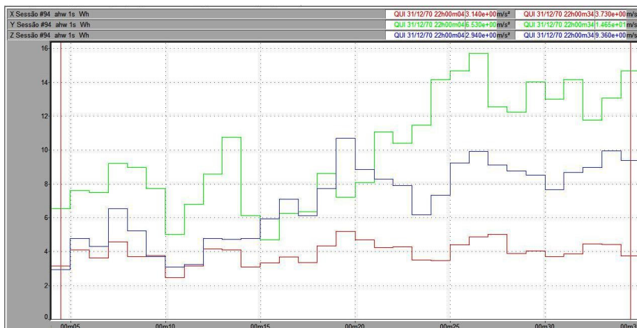
Figura 57 – Vibração no trator New Holland TL 75E no membro superior, em pista de asfalto, com pressão de inflação dos pneus de 15 psi, na marcha II-4.
