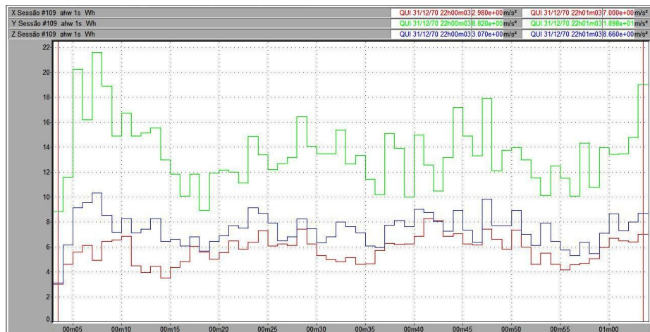
Figura 84 – Vibração no trator New Holland TL 75E no membro superior, em pista de solo firme, com pressão de inflação dos pneus de 20 psi, na marcha II-4.
