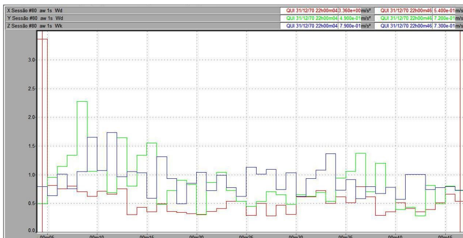
Figura 23 – Vibração no trator New Holland TL 75E no corpo inteiro, em pista de asfalto, com pressão de inflação dos pneus de 20 psi, na marcha II-3.
