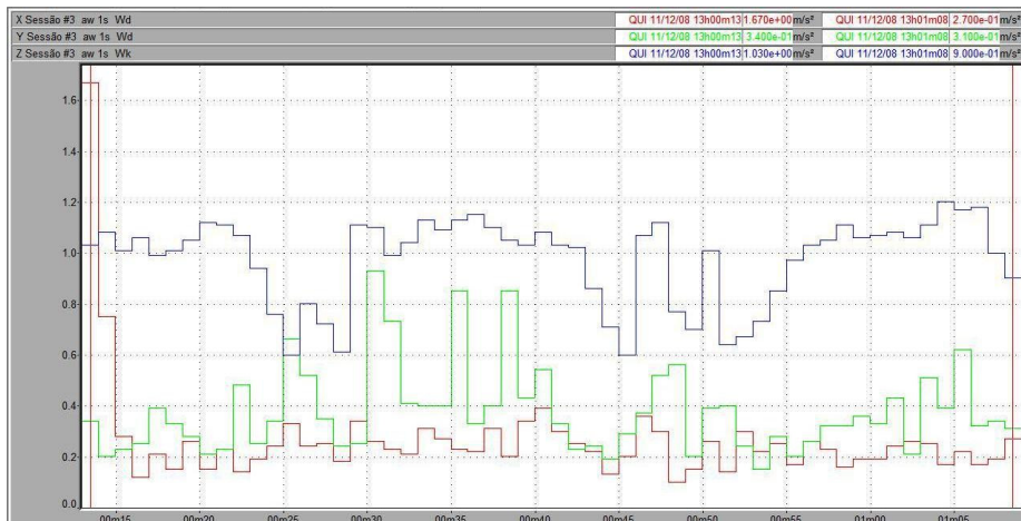
Figura 122 – Vibração no trator New Holland TS 110 no corpo inteiro, em pista de solo batido, com pressão de inflação dos pneus de 25 psi, na marcha II-3.
