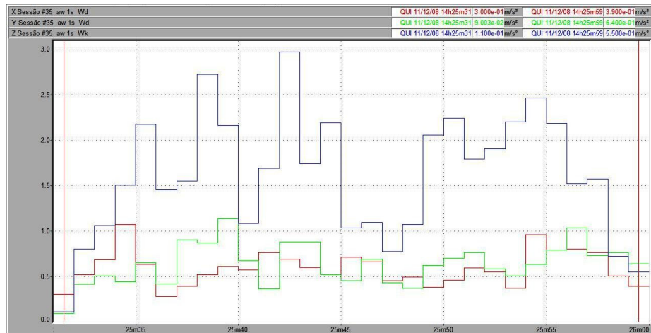
Figura 111 – Vibração no trator New Holland TS 110 no corpo inteiro, em pista de concreto, com pressão de inflação dos pneus de 25 psi, na marcha II-4.
