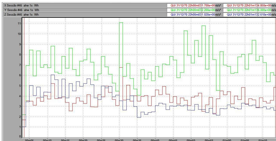
Figura 76 – Vibração no trator New Holland TL 75E no membro superior, em pista de concreto, com pressão de inflação dos pneus de 30 psi, na marcha II-2.
