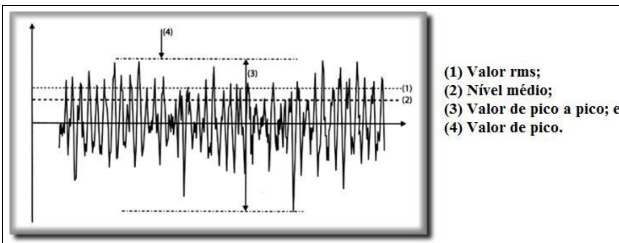
Figura 2 – Gráfico da aceleração em função do tempo, também apresentando o nível médio de vibração e os valores de rms, pico a pico e de pico.
