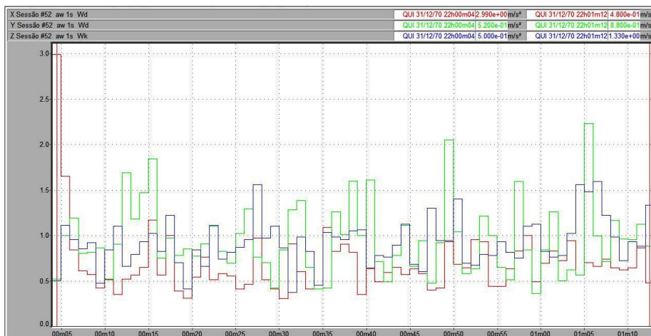
Figura 40 – Vibração no trator New Holland TL 75E no corpo inteiro, em pista de concreto, com pressão de inflação dos pneus de 30 psi, na marcha II-2.
