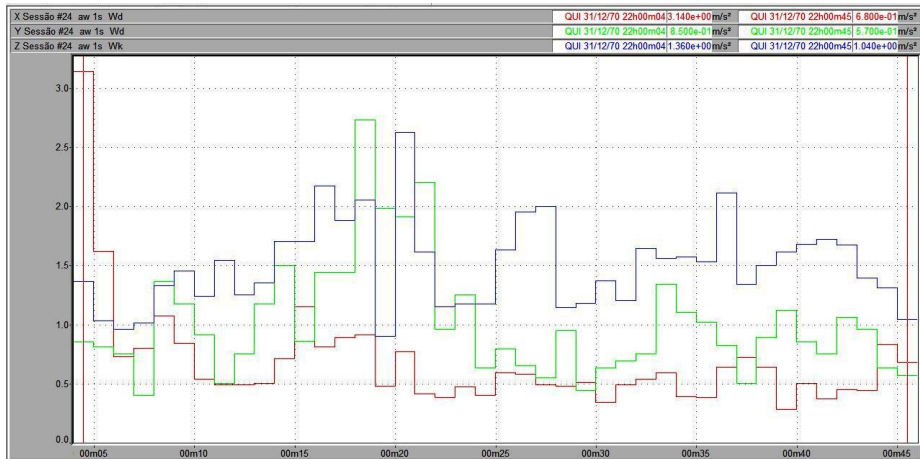
Figura 117 – Vibração no trator New Holland TS 110 no corpo inteiro, em pista de solo batido, com pressão de inflação dos pneus de 15 psi, na marcha II-4.
