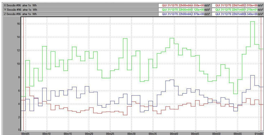
Figura 80 – Vibração no trator New Holland TL 75E no membro superior, em pista de solo firme, com pressão de inflação dos pneus de 15 psi, na marcha II-3.
