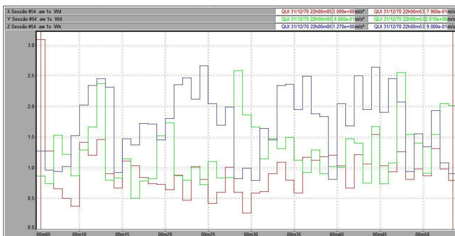
Figura 41 – Vibração no trator New Holland TL 75E no corpo inteiro, em pista de concreto, com pressão de inflação dos pneus de 30 psi, na marcha II-3.
