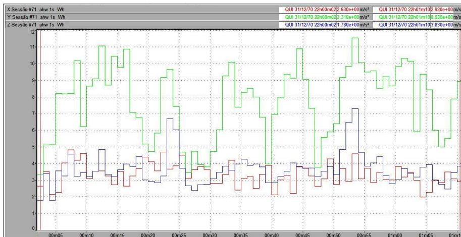
Figura 70 – Vibração no trator New Holland TL 75E no membro superior, em pista de concreto, com pressão de inflação dos pneus de 20 psi, na marcha II-2.
