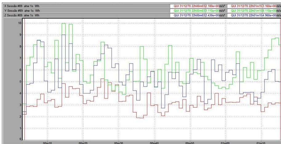
Figura 67 – Vibração no trator New Holland TL 75E no membro superior, em pista de concreto, com pressão de inflação dos pneus de 15 psi, na marcha II-2.
