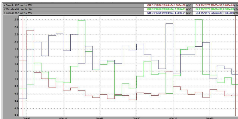
Figura 30 – Vibração no trator New Holland TL 75E no corpo inteiro, em pista de asfalto, com pressão de inflação dos pneus de 30 psi, na marcha II-4.
