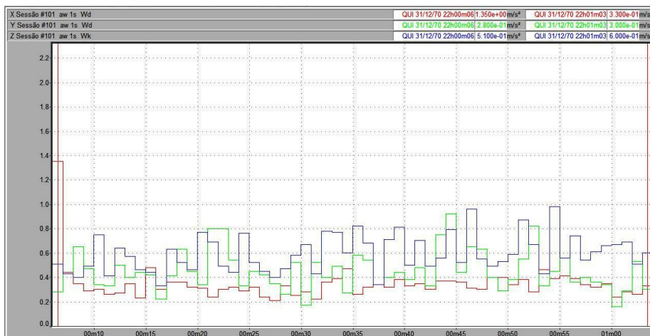
Figura 49 – Vibração no trator New Holland TL 75E no corpo inteiro, em pista de solo firme, com pressão de inflação dos pneus de 25 psi, na marcha II-2.
