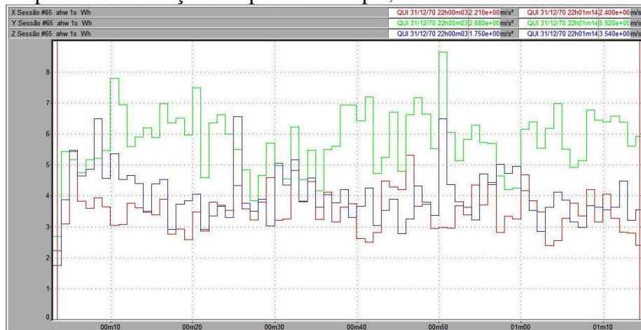
Figura 73 – Vibração no trator New Holland TL 75E no membro superior, em pista de concreto, com pressão de inflação dos pneus de 25 psi, na marcha II-2.
