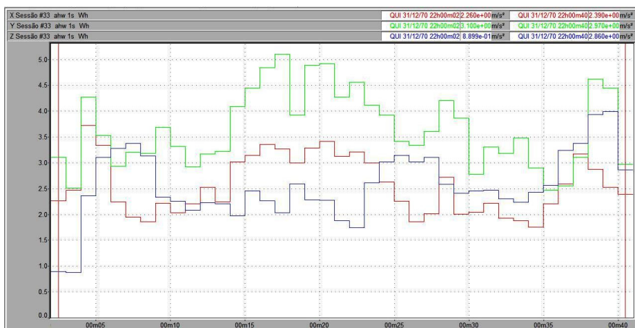
Figura 128 – Vibração no trator New Holland TS 110 no membro superior, em pista de asfalto, com pressão de inflação dos pneus de 15 psi, na marcha II-3.
