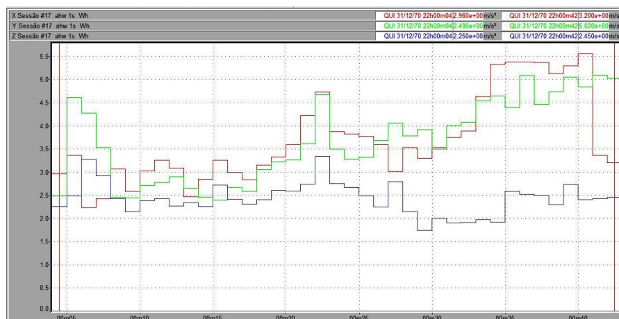
Figura 155 – Vibração no trator New Holland TS 110 no membro superior, em pista de solo firme, com pressão de inflação dos pneus de 20 psi, na marcha II-3.
