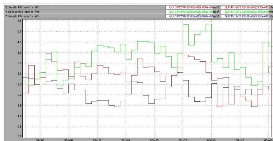
Figura 140 – Vibração no trator New Holland TS 110 no membro superior, em pista de concreto, com pressão de inflação dos pneus de 15 psi, na marcha II-3.
