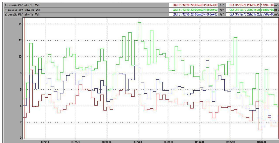
Figura 81 – Vibração no trator New Holland TL 75E no membro superior, em pista de solo firme, com pressão de inflação dos pneus de 15 psi, na marcha II-4.
