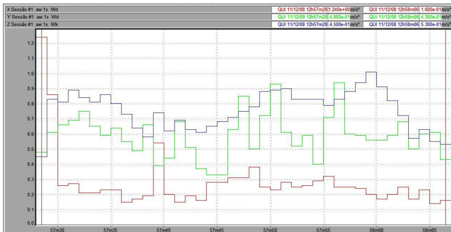
Figura 121 – Vibração no trator New Holland TS 110 no corpo inteiro, em pista de solo batido, com pressão de inflação dos pneus de 25 psi, na marcha II-2.
