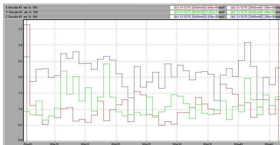
Figura 107 – Vibração no trator New Holland TS 110 no corpo inteiro, em pista de concreto, com pressão de inflação dos pneus de 20 psi, na marcha II-3.
