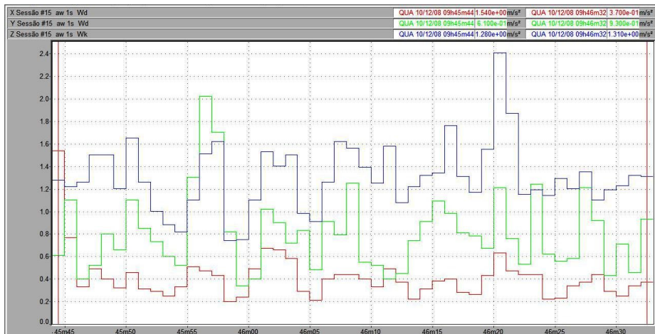
Figura 125 – Vibração no trator New Holland TS 110 no corpo inteiro, em pista de solo batido, com pressão de inflação dos pneus de 30 psi, na marcha II-3.
