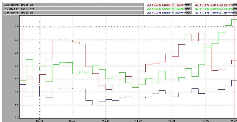
Figura 159 – Vibração no trator New Holland TS 110 no membro superior, em pista de solo firme, com pressão de inflação dos pneus de 25 psi, na marcha II-4.
