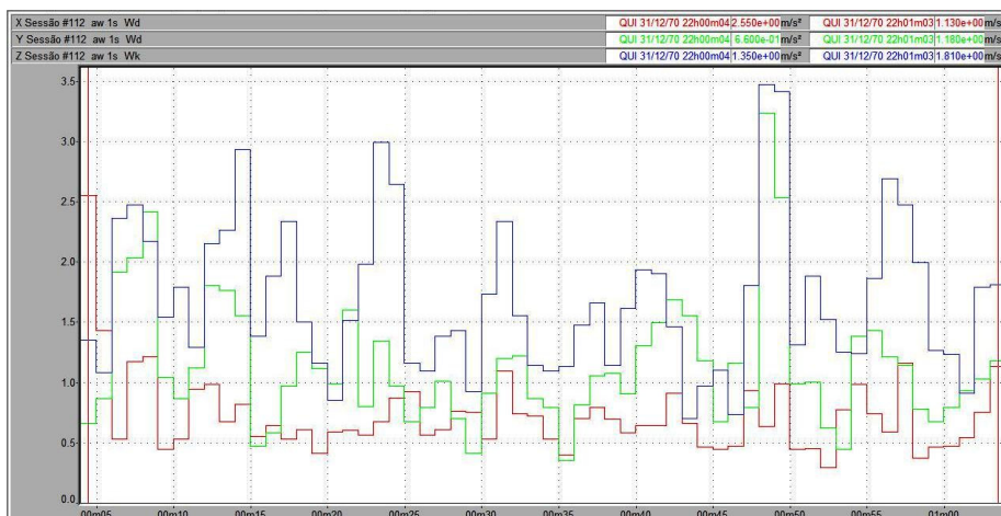
Figura 48- Vibração no trator New Holland TL 75E no corpo inteiro, em pista de solo firme, com pressão de inflação dos pneus de 20 psi, na marcha II-4.
