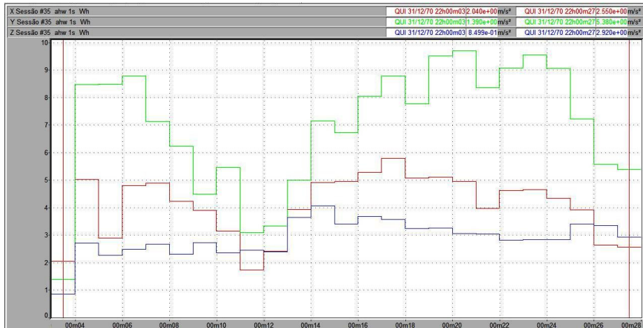
Figura 129 – Vibração no trator New Holland TS 110 no membro superior, em pista de asfalto, com pressão de inflação dos pneus de 15 psi, na marcha II-4.
