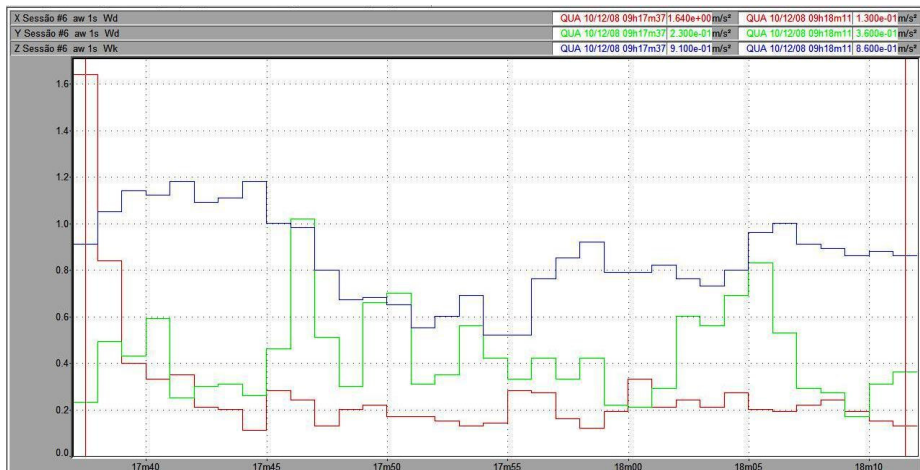
Figura 101 – Vibração no trator New Holland TS 110 no corpo inteiro, em pista de asfalto, com pressão de inflação dos pneus de 30 psi, na marcha II-3.
