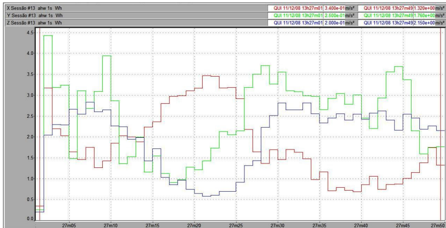
Figura 133 – Vibração no trator New Holland TS 110 no membro superior, em pista de asfalto, com pressão de inflação dos pneus de 25 psi, na marcha II-2.
