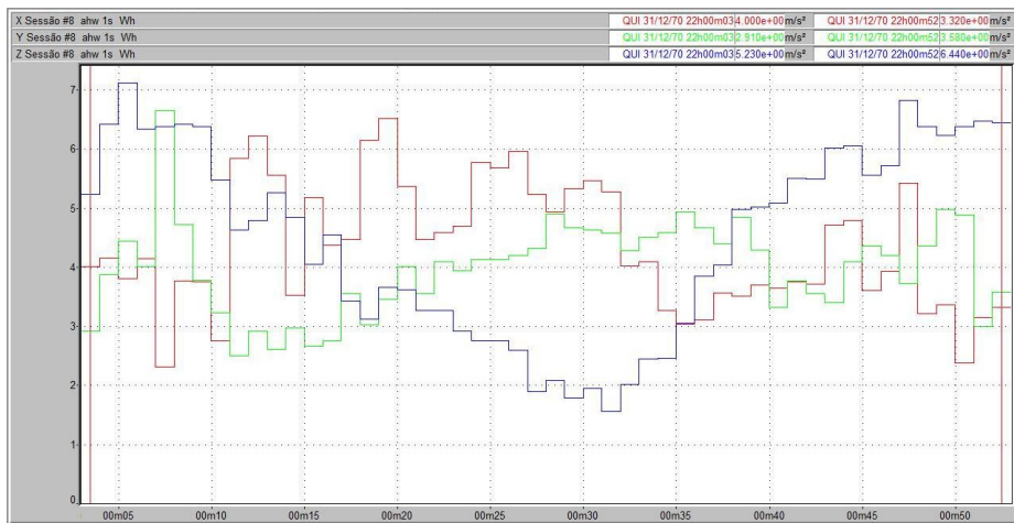
Figura 130 – Vibração no trator New Holland TS 110 no membro superior, em pista de asfalto, com pressão de inflação dos pneus de 20 psi, na marcha II-2.
