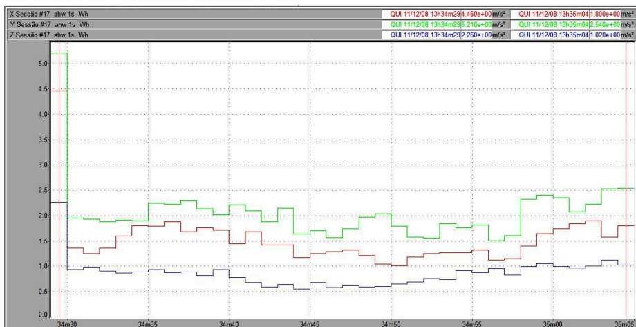
Figura 134 – Vibração no trator New Holland TS 110 no membro superior, em pista de asfalto, com pressão de inflação dos pneus de 25 psi, na marcha II-3.
