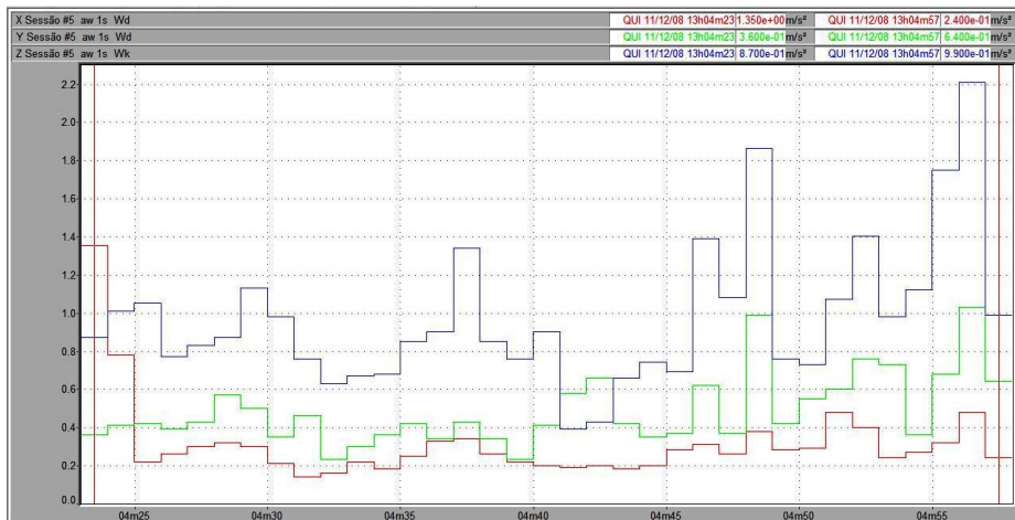
Figura 123 – Vibração no trator New Holland TS 110 no corpo inteiro, em pista de solo batido, com pressão de inflação dos pneus de 25 psi, na marcha II-4.
