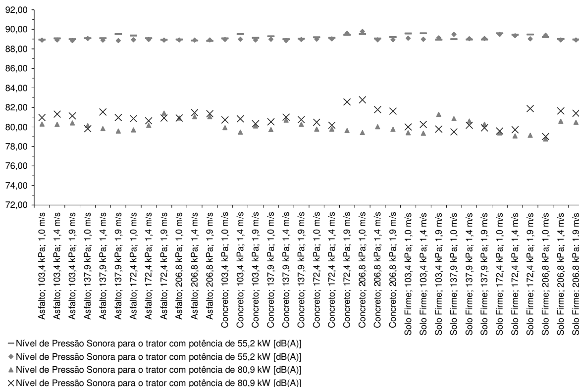
Figura 18 – Nível de pressão sonora para os tratores de 55,2 kW e 80,9 kW, em função dos tratamentos: tipo de pista, pressão de inflação dos pneus e velocidade média de deslocamento.
