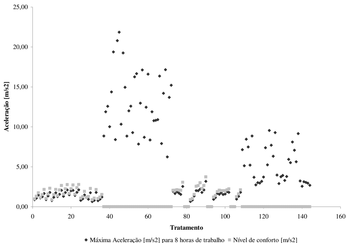
Figura 16 – Máximas acelerações para 8 horas de trabalho e nível de conforto em função da indexação da Tabela 7.
