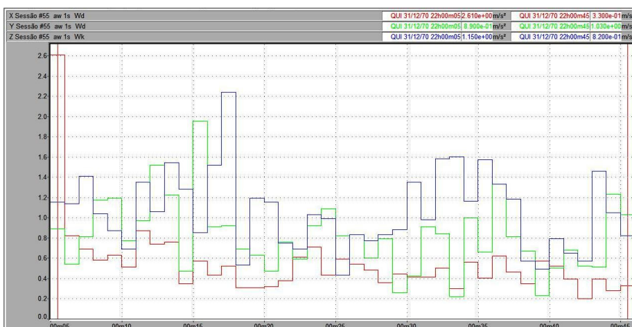
Figura 29 – Vibração no trator New Holland TL 75E no corpo inteiro, em pista de asfalto, com pressão de inflação dos pneus de 30 psi, na marcha II-3.
