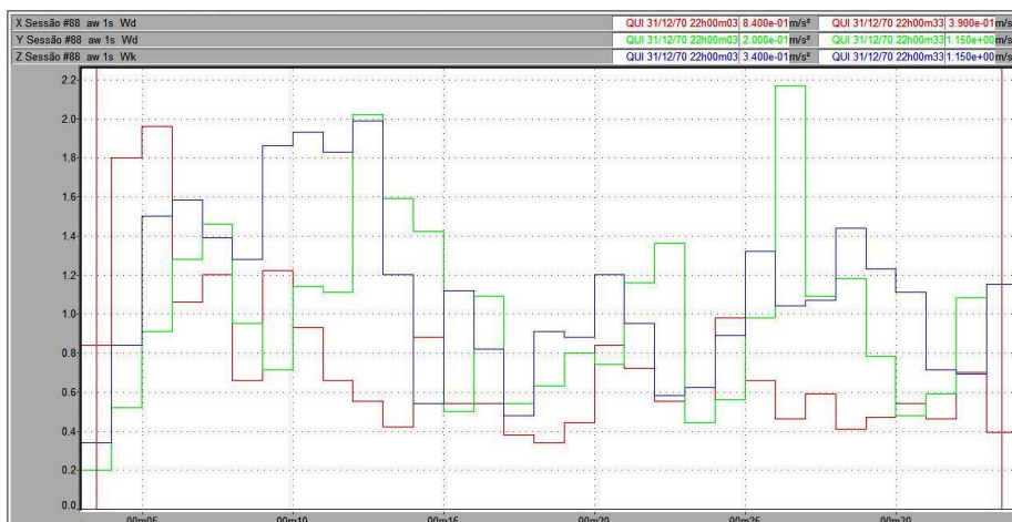
Figura 21 – Vibração no trator New Holland TL 75E no corpo inteiro, em pista de asfalto, com pressão de inflação dos pneus de 15 psi, na marcha II-4.
