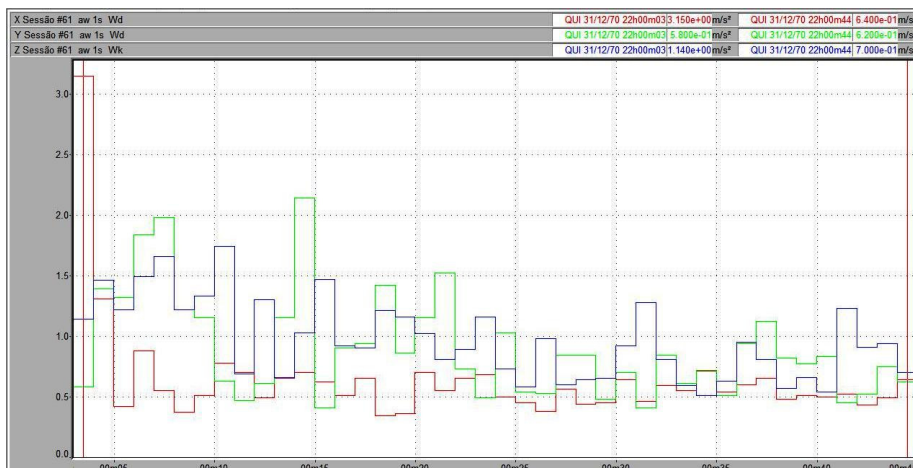
Figura 26 – Vibração no trator New Holland TL 75E no corpo inteiro, em pista de asfalto, com pressão de inflação dos pneus de 25 psi, na marcha II-3.
