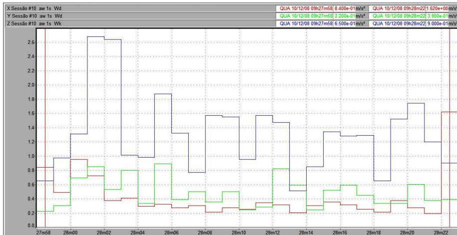
Figura 102 – Vibração no trator New Holland TS 110 no corpo inteiro, em pista de asfalto, com pressão de inflação dos pneus de 30 psi, na marcha II-4.
