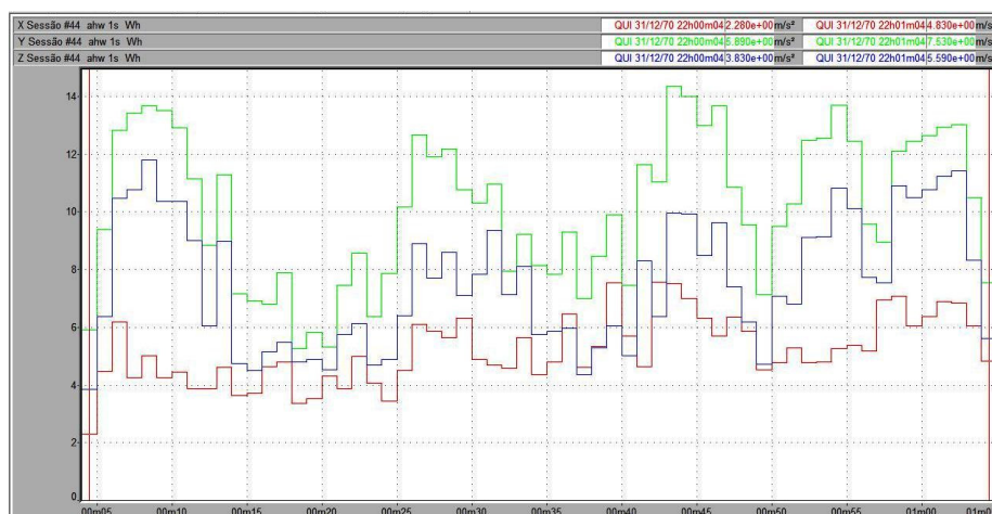
Figura 89 – Vibração no trator New Holland TL 75E no membro superior, em pista de solo firme, com pressão de inflação dos pneus de 30 psi, na marcha II-3.
