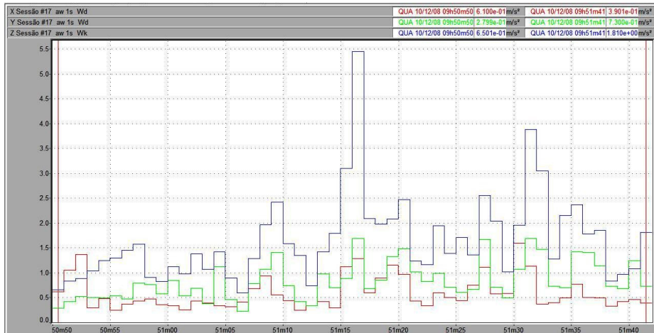
Figura 126 – Vibração no trator New Holland TS 110 no corpo inteiro, em pista de solo batido, com pressão de inflação dos pneus de 30 psi, na marcha II-4.
