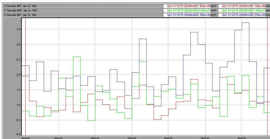
Figura 33 – Vibração no trator New Holland TL 75E no corpo inteiro, em pista de concreto, com pressão de inflação dos pneus de 15 psi, na marcha II-4.
