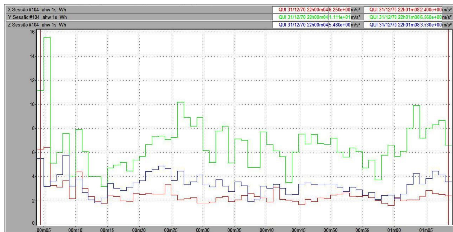
Figura 85 – Vibração no trator New Holland TL 75E no membro superior, em pista de solo firme, com pressão de inflação dos pneus de 25 psi, na marcha II-2.
