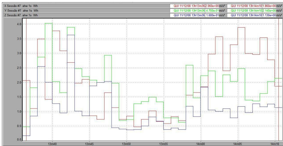
Figura 157 – Vibração no trator New Holland TS 110 no membro superior, em pista de solo firme, com pressão de inflação dos pneus de 25 psi, na marcha II-2.
