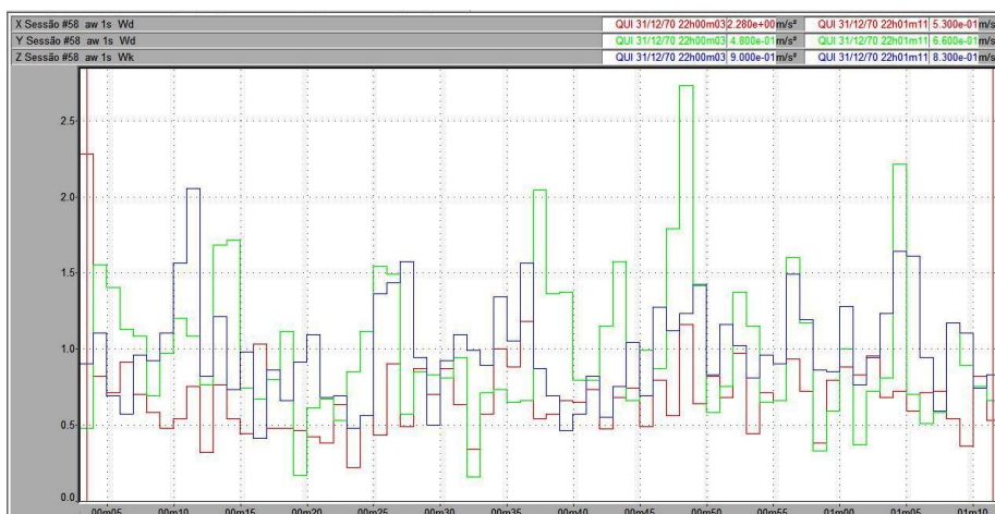
Figura 37 – Vibração no trator New Holland TL 75E no corpo inteiro, em pista de concreto, com pressão de inflação dos pneus de 25 psi, na marcha II-2.
