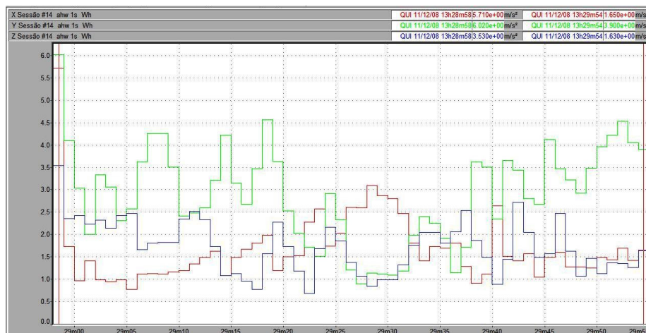
Figura 145 – Vibração no trator New Holland TS 110 no membro superior, em pista de concreto, com pressão de inflação dos pneus de 25 psi, na marcha II-2.
