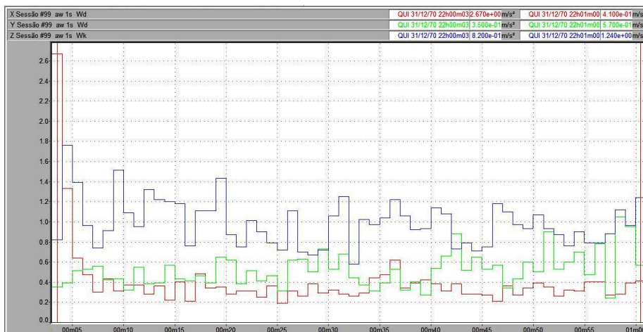
Figura 44 – Vibração no trator New Holland TL 75E no corpo inteiro, em pista de solo firme, com pressão de inflação dos pneus de 15 psi, na marcha II-3.
