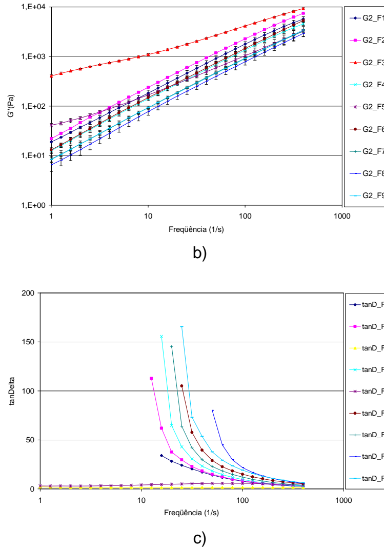
Figura 4.4. Módulo elástico (a), módulo viscoso (b) e \tan\delta (c) medidos a 150°C para as formulações F1 a F9
