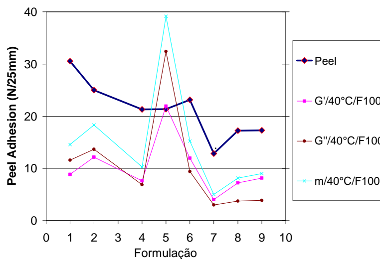
Figura 4.18. Correlação entre Peel e propriedades reológicas
