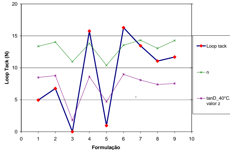
Figura 4.21. Correlação entre Loop Tack e propriedades reológicas
