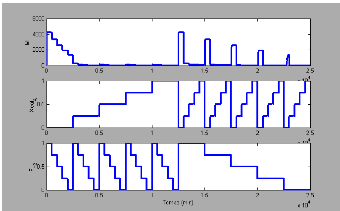
Figure 5.6: Perturbações realizadas para realizar a conversão do modelo fenomenológico em simplificado (sentido reverso)
