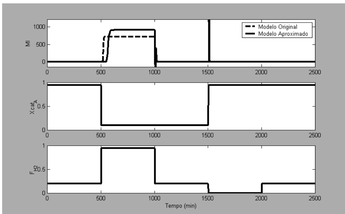
Figure 5.13: Comparação da resposta dos modelos original e aproximado para uma identificação baseada em momentos. Perturbações diferentes das utilizadas na identificação.
