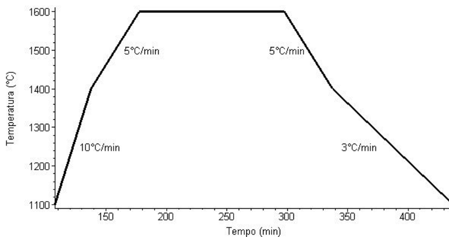
Figura 3.2: Curva de aquecimento/resfriamento
