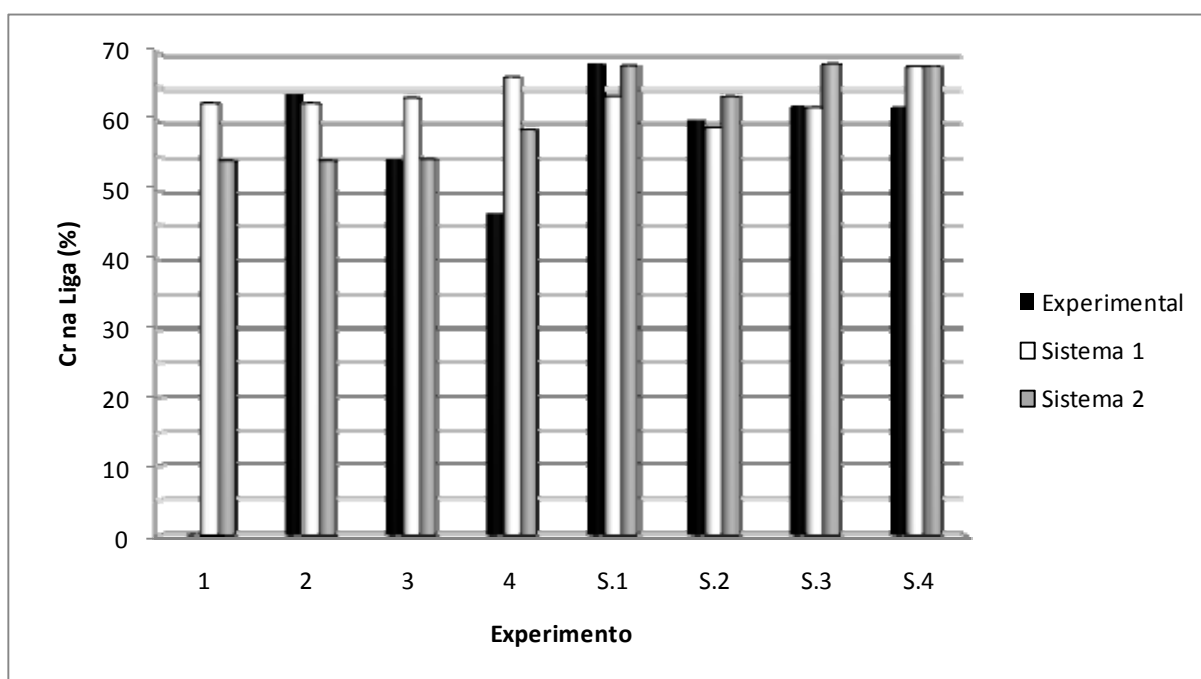
Figura 4.5: Comparação do resultado experimental com as simulações considerando dois diferentes sistemas para predição do teor de cromo na fase metálica
