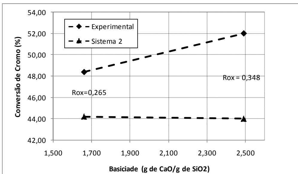
Figura 4.11: Conversão de cromo em função do parâmetro B para R_R = -39,54\% e R_{OX} variável
