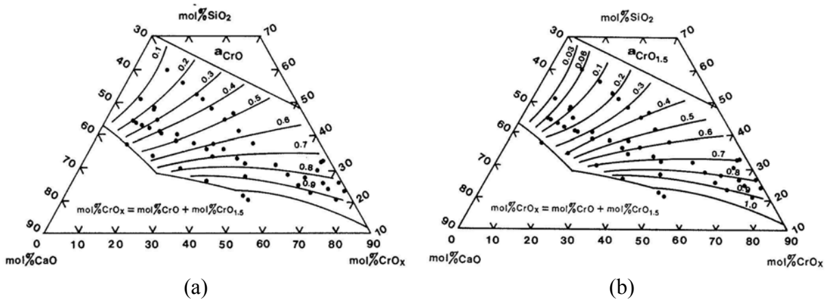
Figura 2.16: Diagrama de isoatividade do CrO (a) e \text{CrO}_{1,5} (b) na região líquida do sistema quasi-ternário CaO- \text{SiO}_2 - \text{CrO}_x à 1600^\circ\text{C} . Fonte: Xiao e Holappa (1993)
