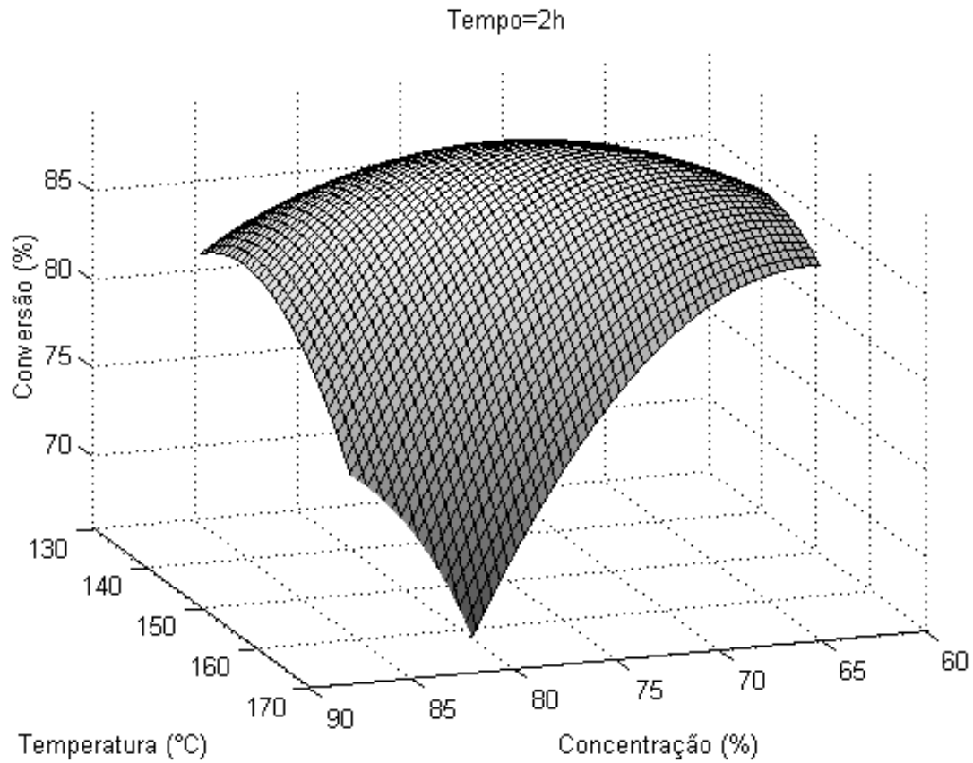
Figura 4.14: Superfície de resposta da conversão de cromo: (a) em função de t e C , com T=150^{\circ}\text{C} ; (b) em função de t e T com C=75\% ; (c) em função de T e C , com t=2\text{h}
