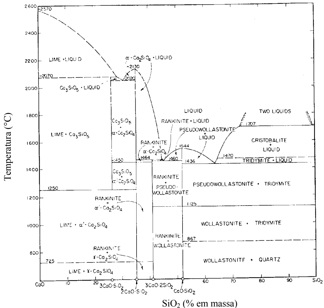
Figura 2.9: Diagrama de fases do sistema CaO-SiO 2 . Fonte: Muan e Osborn (1965) apud Villiers e Muan (1992)
