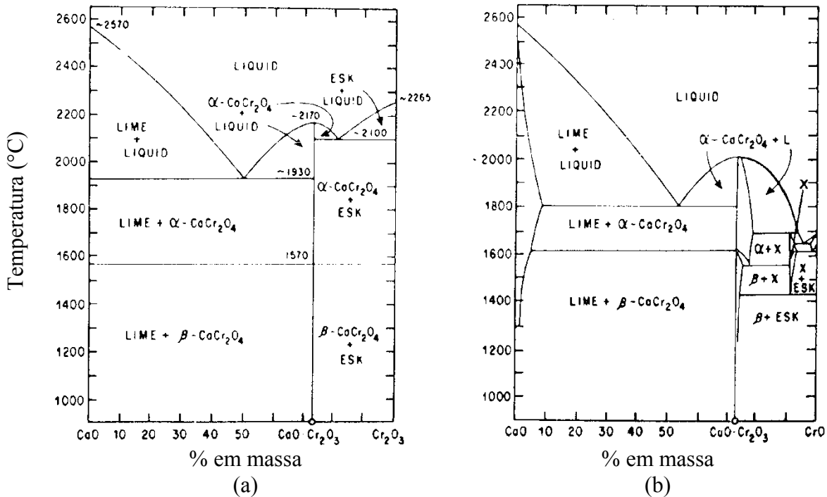
Figura 2.10: Diagrama de fases do sistema CaO-óxido de cromo; (a) condição redutora intermediária, e (b) em contato com cromo metálico. Fonte: Villiers e Muan (1992) citando, em (a), Ol'shanskii et al. (1955) e, em (b), Muan (1983)
