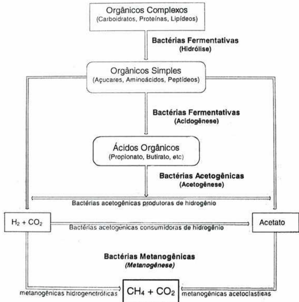
Figura 3.5 – Sequências metabólicas e grupos microbianos envolvidos na digestão anaeróbia
