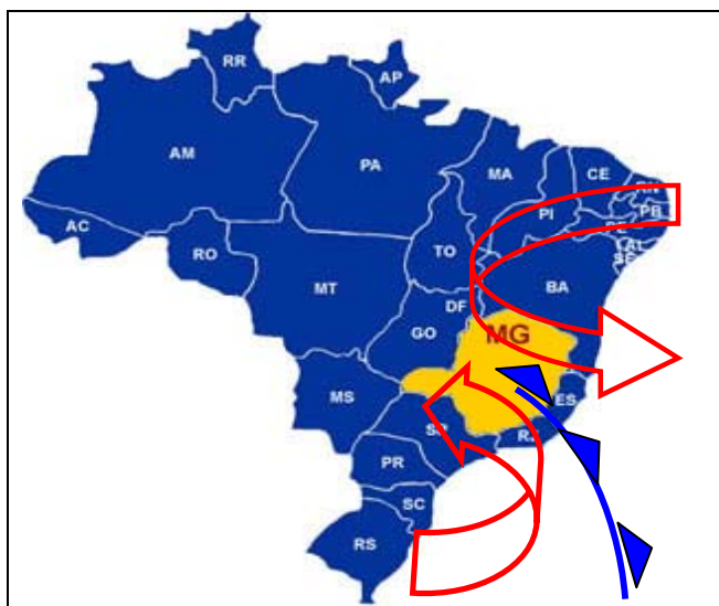
FIGURA 2 – Esquema da atuação dos sistemas frontais no qual são acompanhados por anticiclones de origem polar em escala sinótica em Belo Horizonte.
