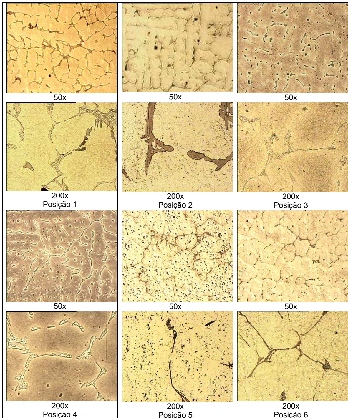
Figura 5.9. Microestruturas das seções transversais. Ataque: HF 0,5%. Condição 1.
