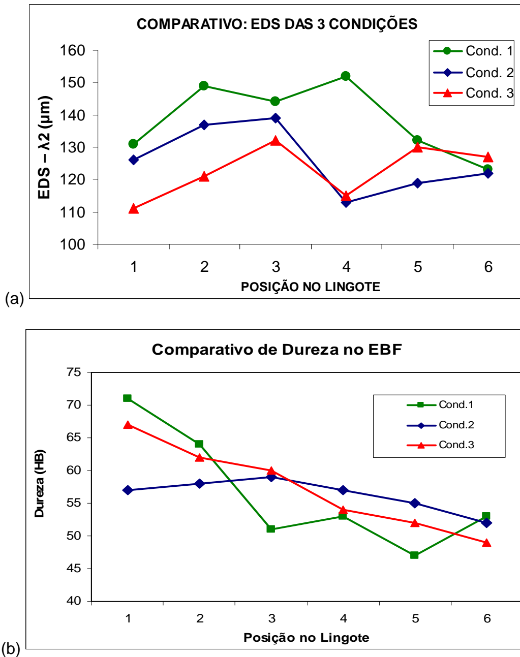
Figura 5.27.(a) e (b) Comportamento dos espaçamentos dendríticos secundários e das durezas no lingote fundido para as condições analisadas.
