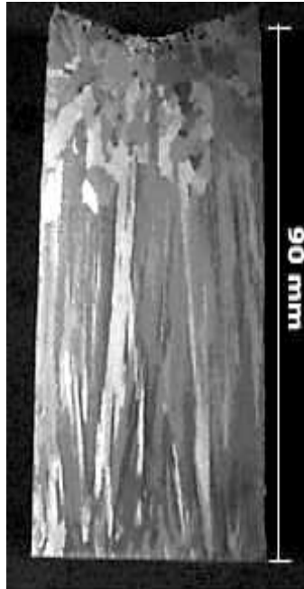
Figura 3.7. Macroestrutura de uma liga Al-Cu fundida vista a olho nu (FINARDI, 1988).
