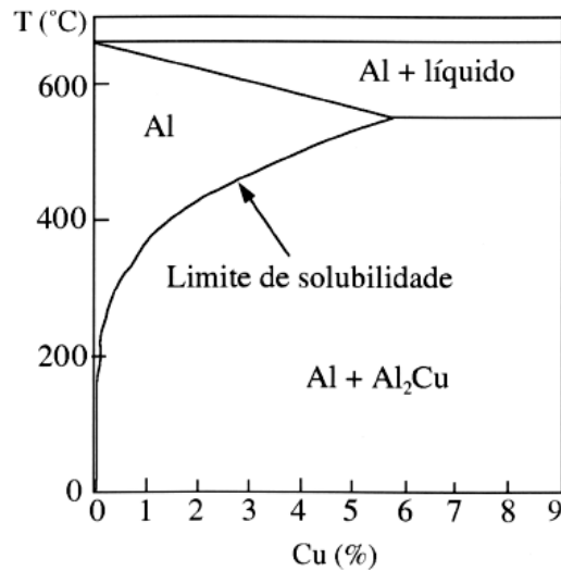
Figura 3.17. Detalhe do diagrama de equilíbrio Al-Cu (BRADASCHIA, 2002).
