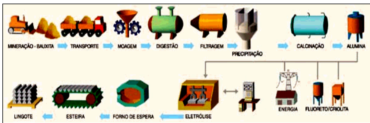
Figura 3.1. Fluxograma da produção do alumínio a partir da bauxita.
