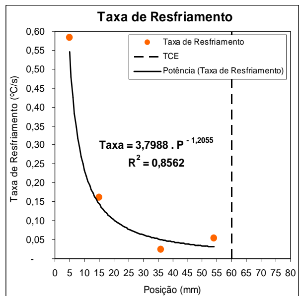
Taxa de Resfriamento x Posição
