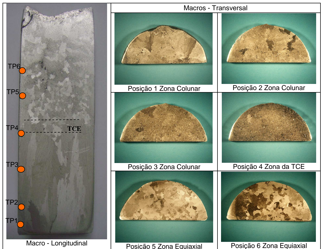
Figura 5.15. Macroestruturas do lingote – secção longitudinal e transversal - Condição 2.
