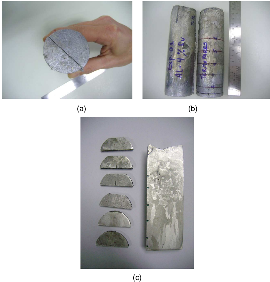
Figura 4.13. (a), (b) e (c) preparação das amostras.
