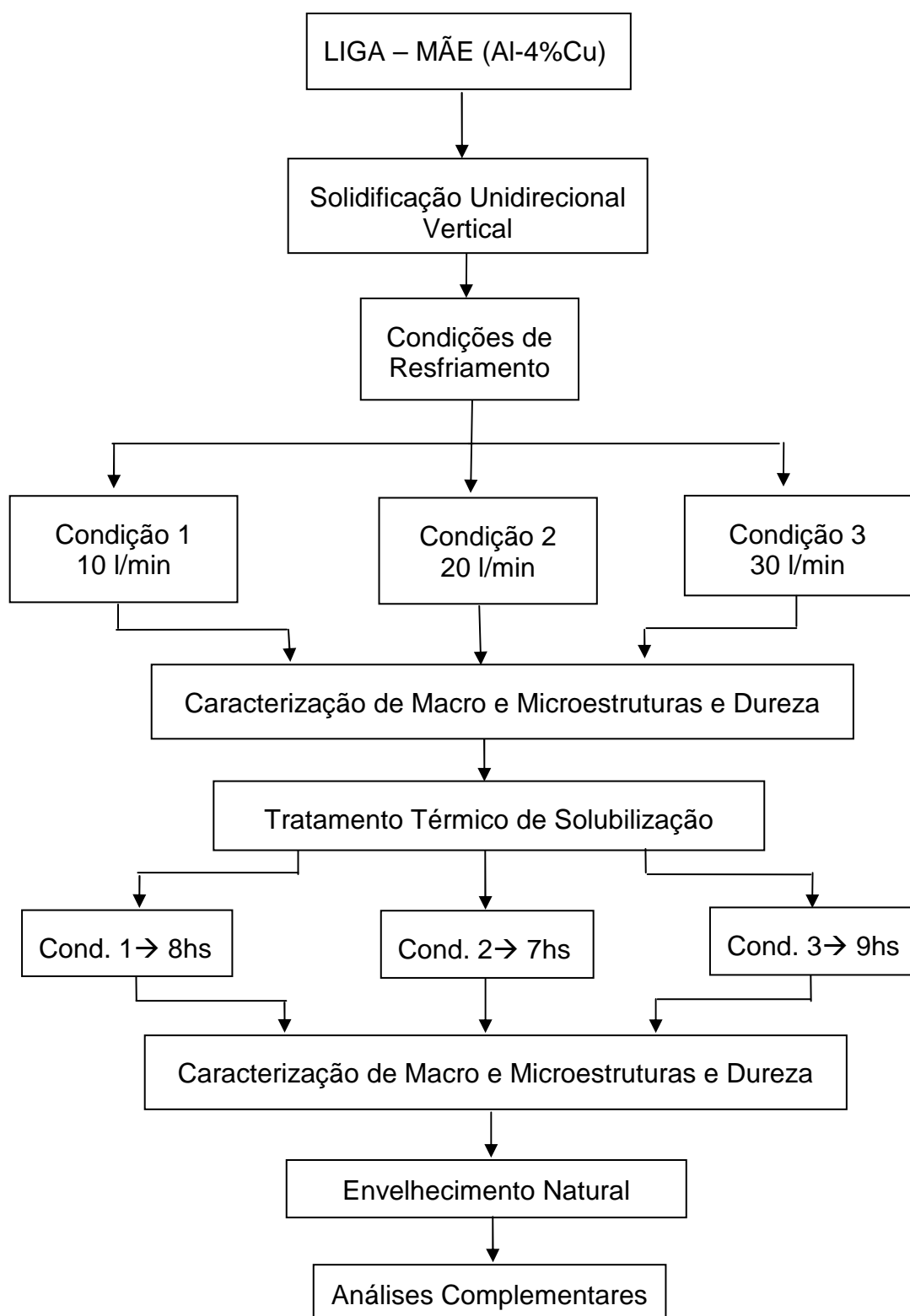
Figura 4.12. Fluxograma do modelo experimental.
