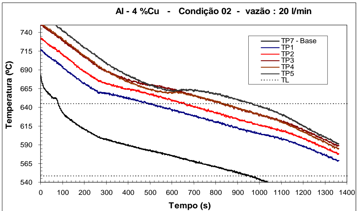
Figura 5.13. Curvas de resfriamento - Vazão 20 l/min - Condição 2.
