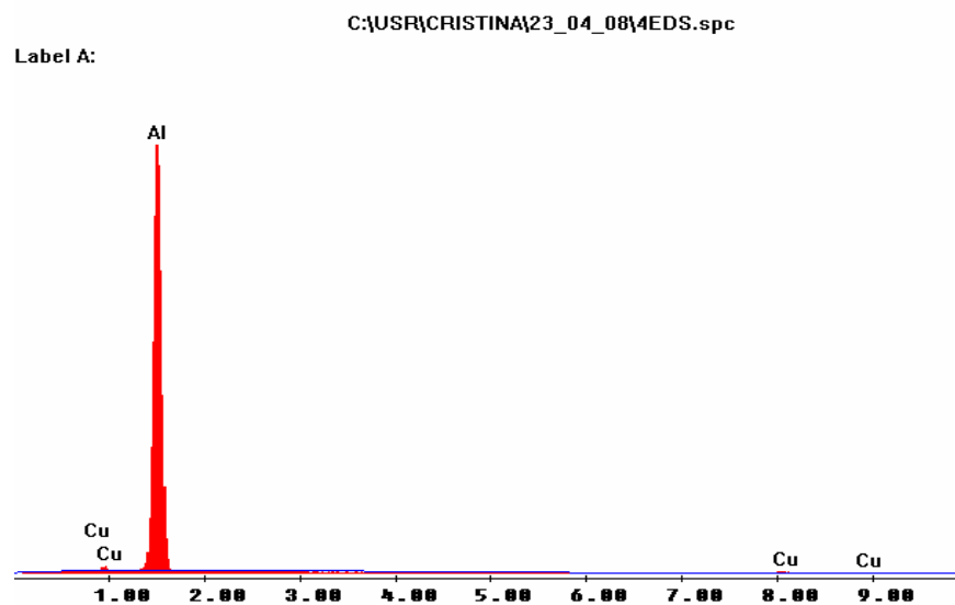
Figura 5.2. Espectro de EDS – MEV do Lote 01.
