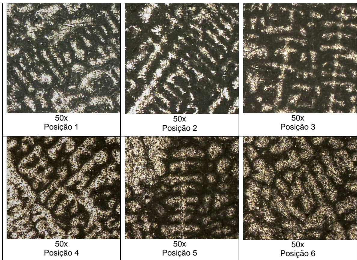
Figura 5.23. Microestruturas das seções transversais. Ataque: HF 0,5% - Condição 3.
