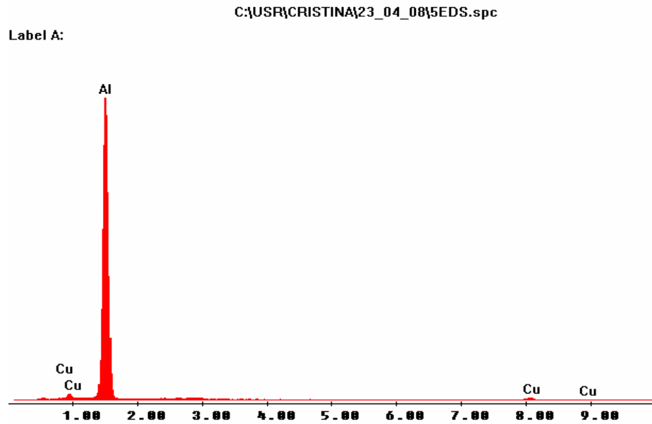
Figura 5.4. Espectro de EDS - MEV do Lote 02.
