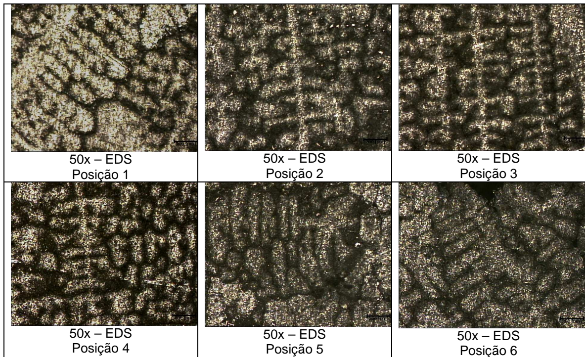
Figura 5.17. Estruturas dendríticas das seções transversais. Ataque Água Régia Fluorada-Condição 2.
