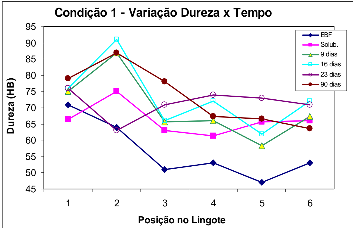
Figura 5.12. Variação da dureza Brinell em função do tempo e posição – Condição 1.
