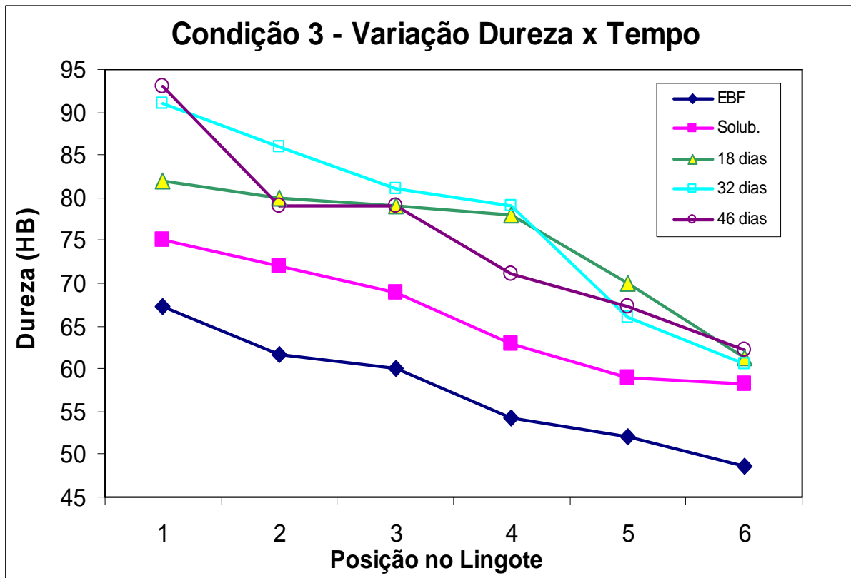
Figura 5.25. Variação da dureza Brinell em função do tempo e posição – Condição 03.
