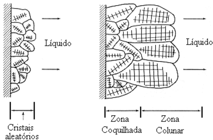
Figura 3.9. Representação esquemática do crescimento de grãos na zona coquilhada e surgimento da zona colunar (GARCIA, 2001).
