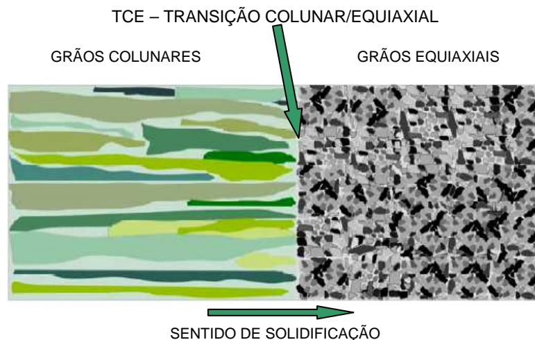
Figura 3.8. Ilustração esquemática da transição colunar/equiaxial (Adaptada de GARCIA, 2001).
