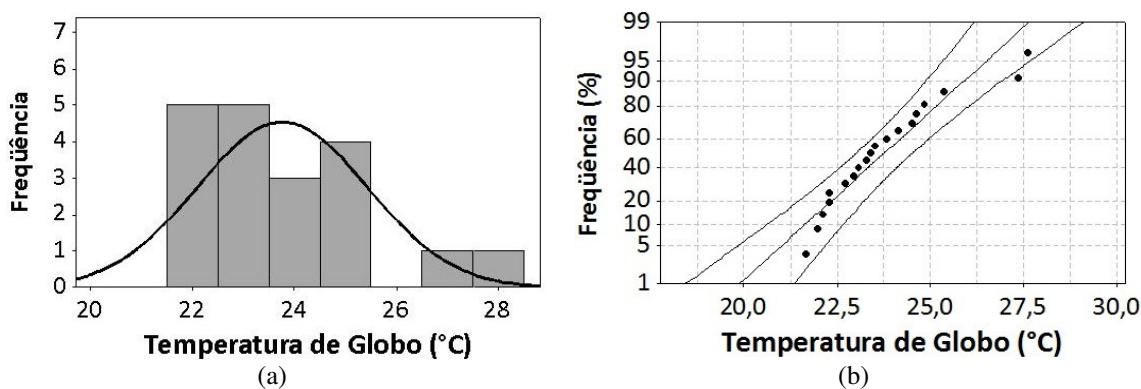
Figura 4.3 – Histograma de frequência com curva normal (a) e gráfico da probabilidade (b) da Temperatura de Globo.
