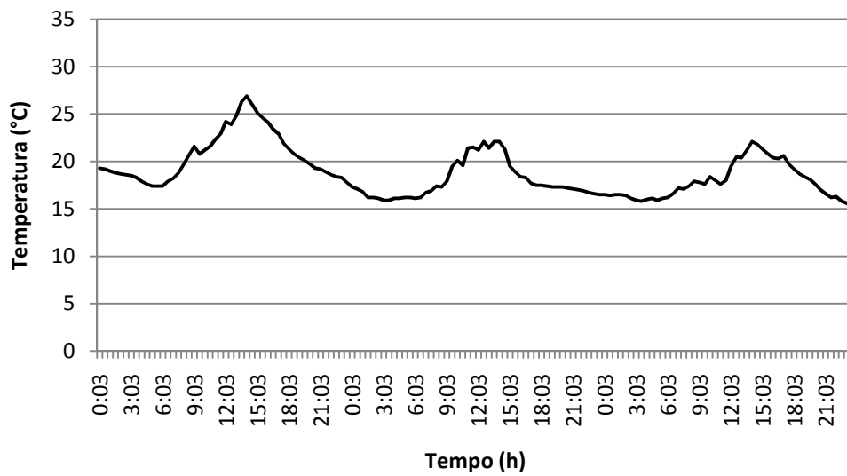
Figura B.5 – Temperatura externa do ar nos dias 17, 18 e 19 de novembro de 2008.
