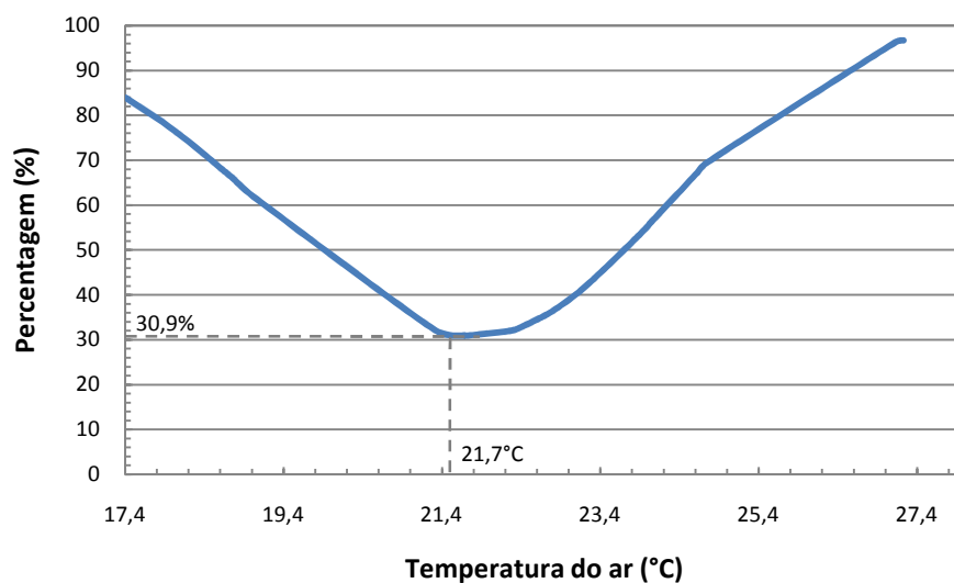
Figura 4.43 – Porcentagem de pessoas insatisfeitas estimada por regressão probit em função da temperatura do ar.
