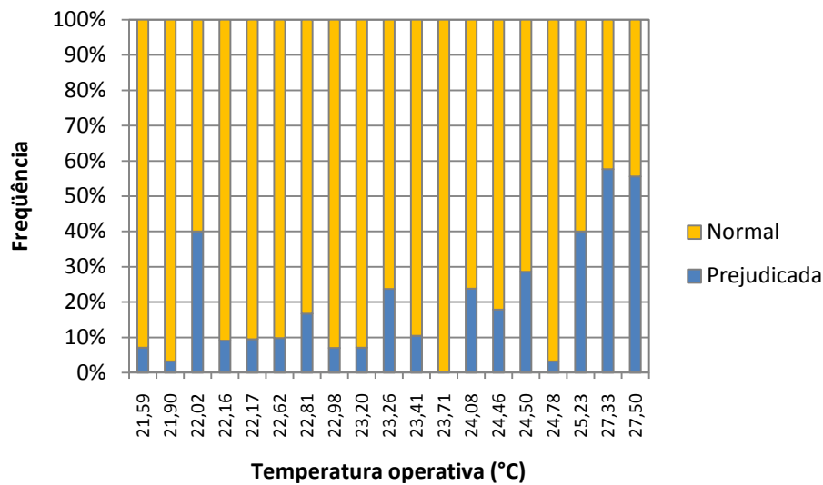
Figura 4.38 – Cruzamento da temperatura operativa com a capacidade de estudar no ambiente.
