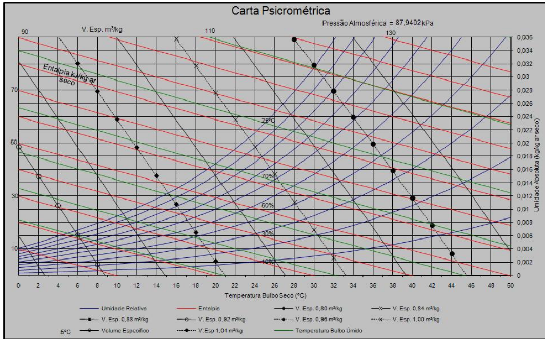
Figura B.7 – Carta psicrométrica para a cidade de Ouro Preto. Fonte: DIAS; MACHADO; KOURY, 2005.
