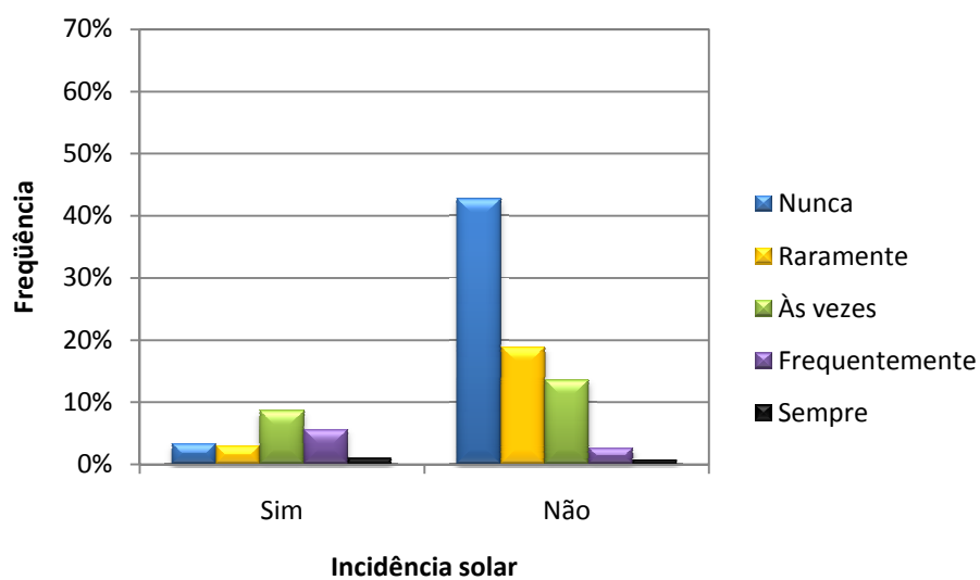
Figura 4.23– Incidência solar e necessidade de controle através de cortinas/persianas (E.M.).
