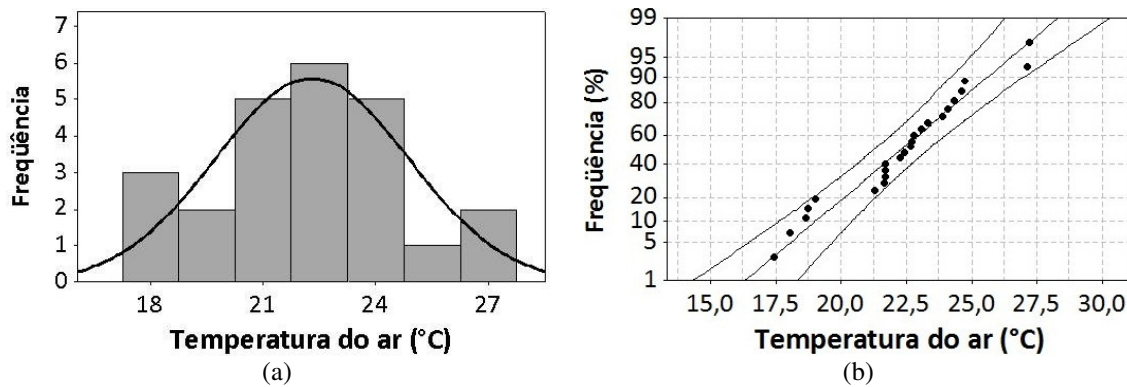
Figura 4.1 – Histograma de frequência com curva normal (a) e gráfico da probabilidade (b) da Temperatura do ar.
