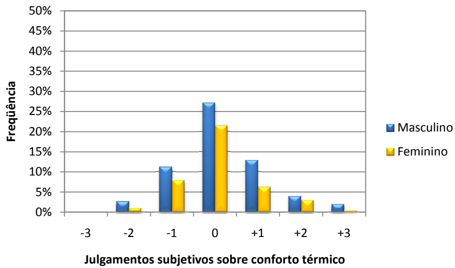
Figura 4.11– Julgamentos subjetivos sobre conforto térmico de acordo com o sexo dos usuários (E.M.).
