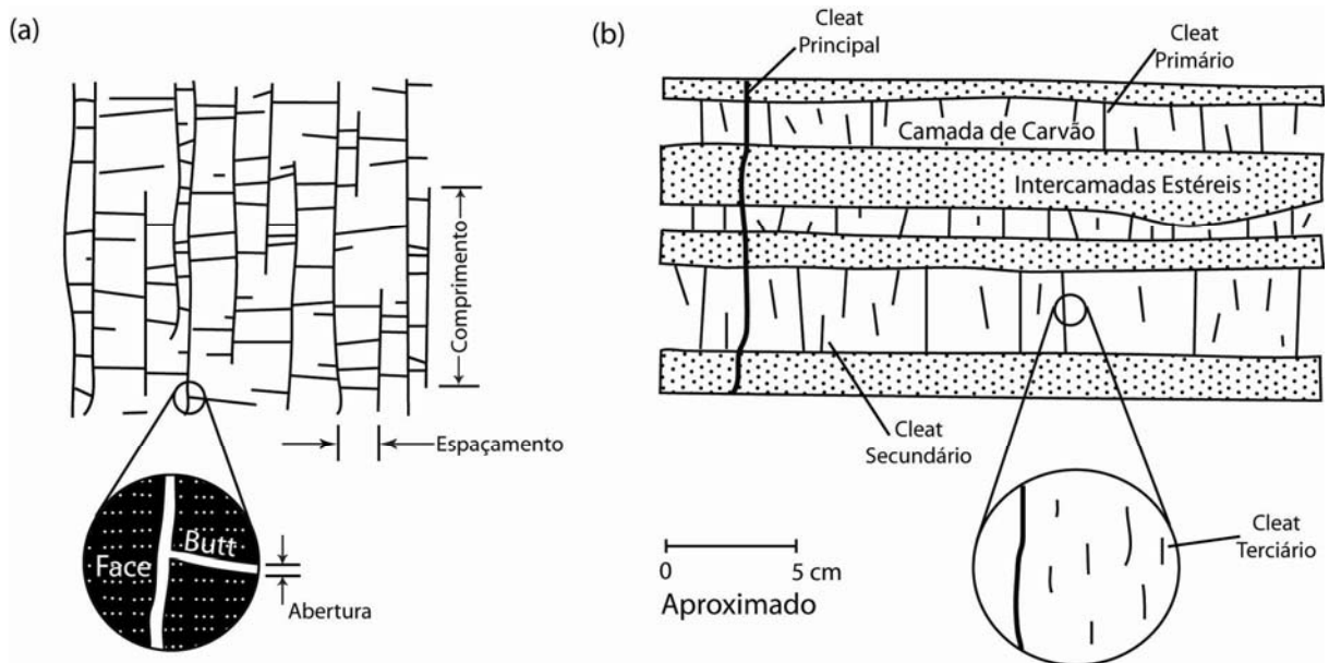
Figura 3.6. Estrutura esquemática do carvão. Adaptado de Laubach et al. (1998).
