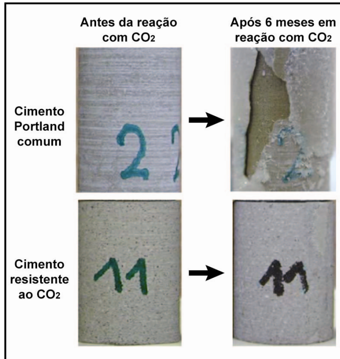
Figura 3.15. Comparação entre cimento Portland comum e cimento resistente ao \text{CO}_2 produzido pela empresa Schlumberger após 6 meses de reação. Adaptado de Barlet-Goédard et al. (2006).
