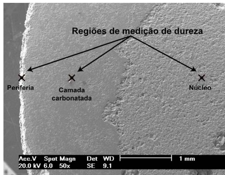
Figura 5.18. Indicação das regiões onde foram realizados os ensaios de microdureza Vickers em cada corpo-de-prova.
