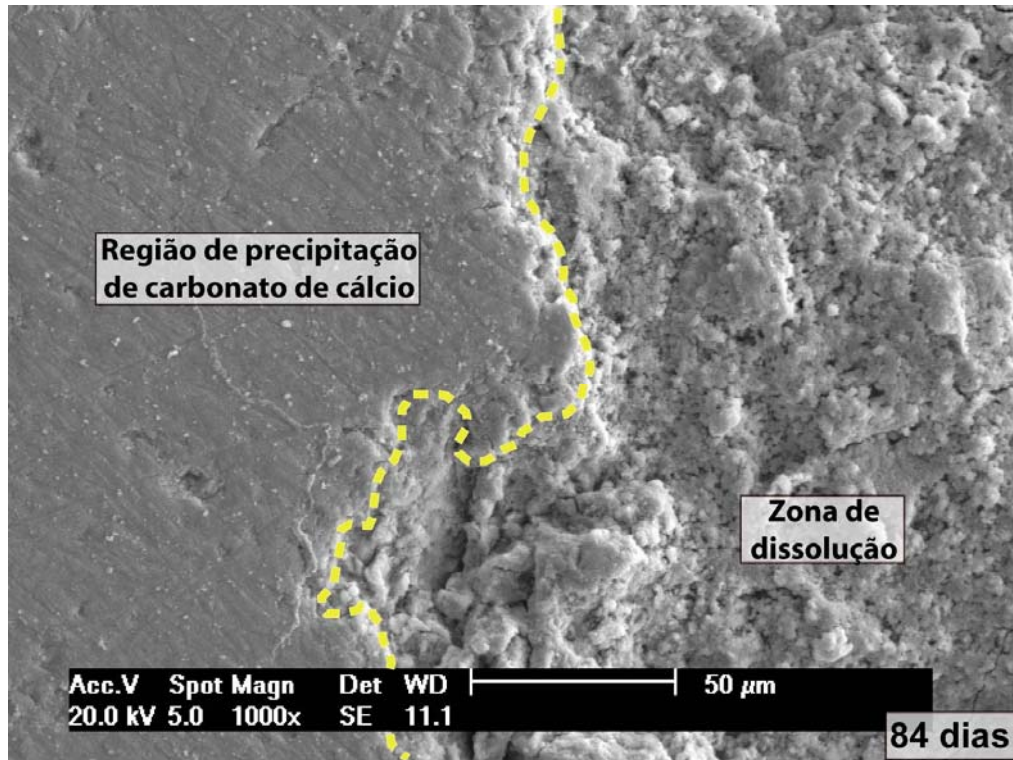
Figura 5.5. Interface entre a camada carbonatada e zona de dissolução de um corpo-de-prova com 84 dias de reação em \text{CO}_2 supercrítico úmido
