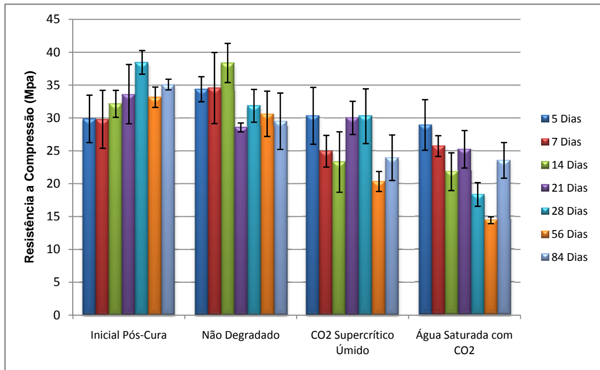
Figura 5.22. Resultado dos ensaios de resistência à compressão ao longo do tempo com corpos-de-prova de pasta de cimento nos dois meios de degradação.
