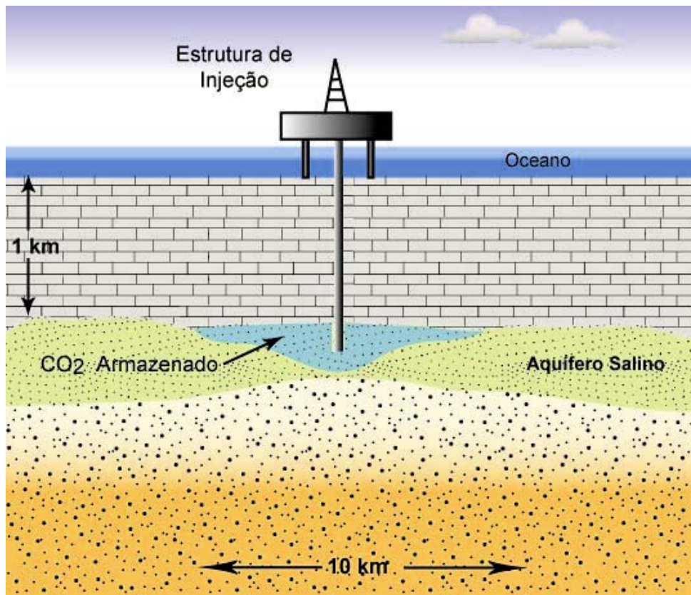
Figura 3.5. Exemplo de armazenamento de CO 2 em aquífero salino. Adaptado de Bentham et al. (2005).
