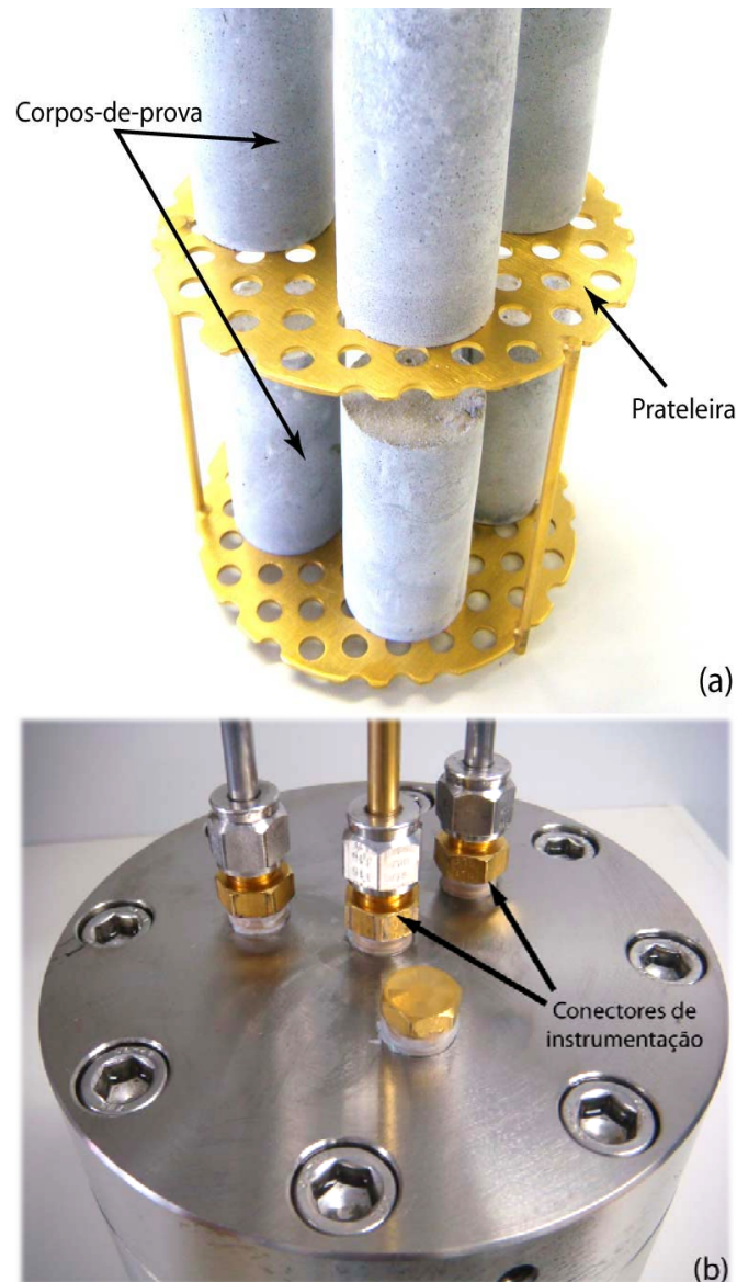
Figura 4.5. Prateleira utilizada para acomodar os corpos-de-prova em dois meios diferentes de degradação no interior do vaso de pressão (a) e conectores de instrumentação com tratamento superficial de nitreto de titânio (b).
