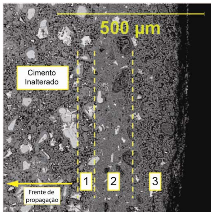
Figura 3.12. Alteração microestrutural da pasta de cimento classe H após reação em meio com \text{CO}_2 supercrítico e sua dinâmica de reações. Fonte: Kutchko et al. (2007).
