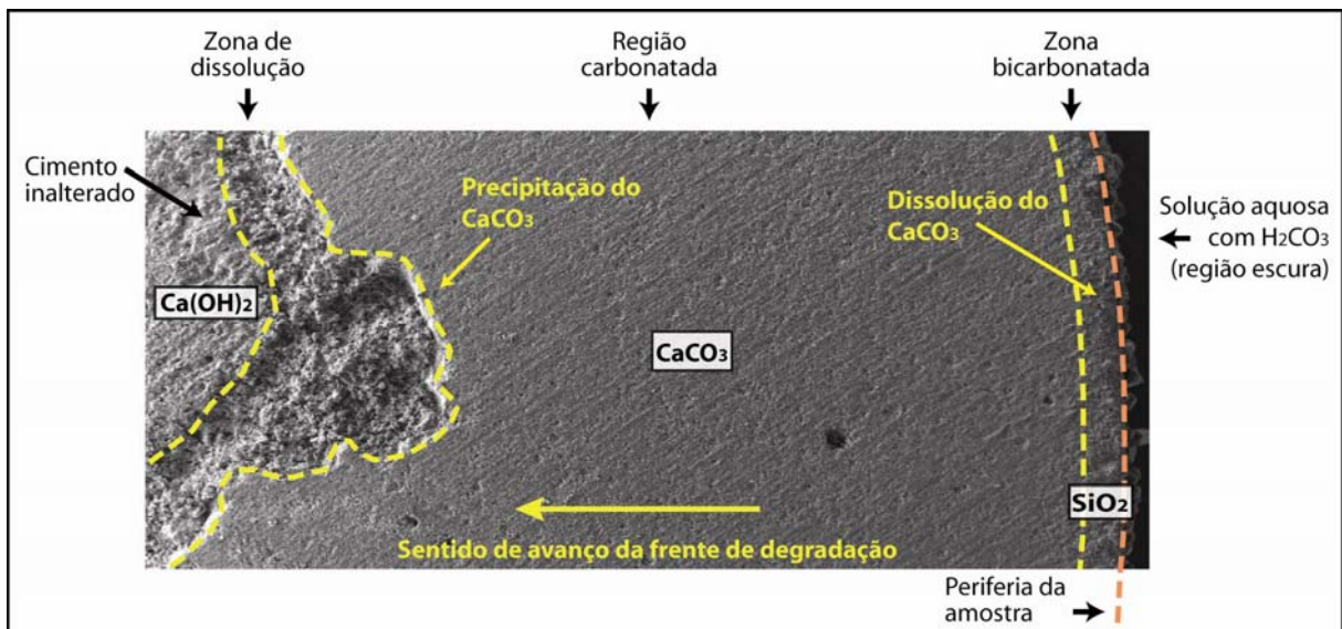
Figura 5.16. Exemplo do mecanismo de avanço da frente de degradação em pastas de cimento quando expostas a meios ricos \text{CO}_2 supercrítico
