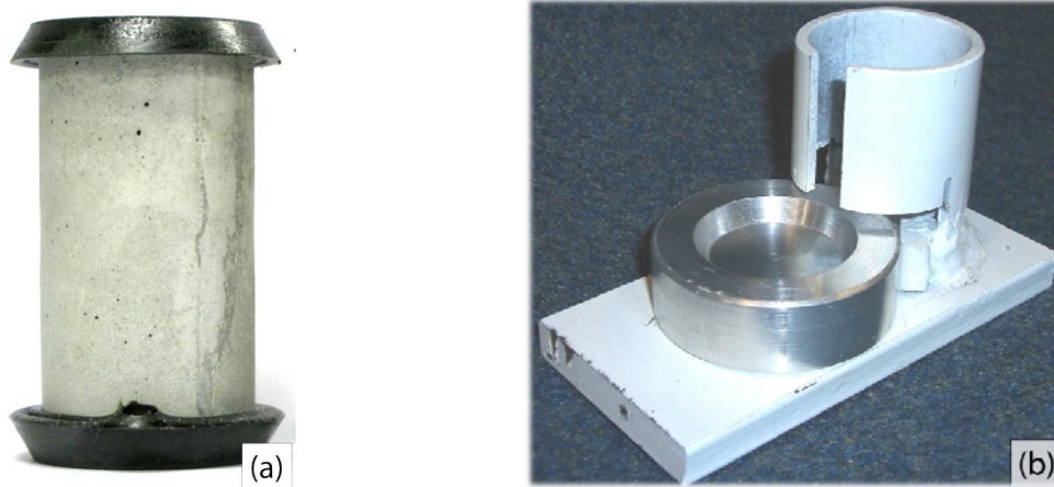
Figura 4.11. Fotografia do corpo-de-prova pronto para ensaio de compressão após o capeamento (a) e fotografia do dispositivo para fazer o capeamento dos corpos-de-prova (b).
