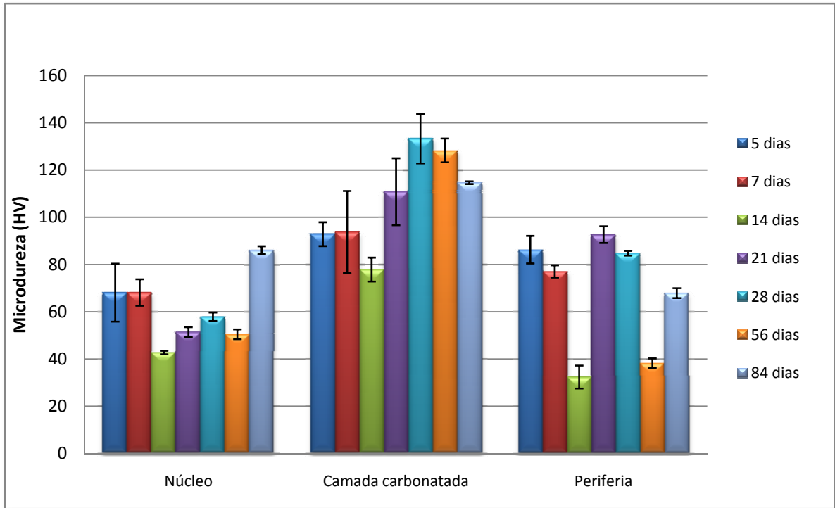
Figura 5.19. Resultados dos ensaios de microdureza Vickers dos experimentos em \text{CO}_2 supercrítico úmido.
