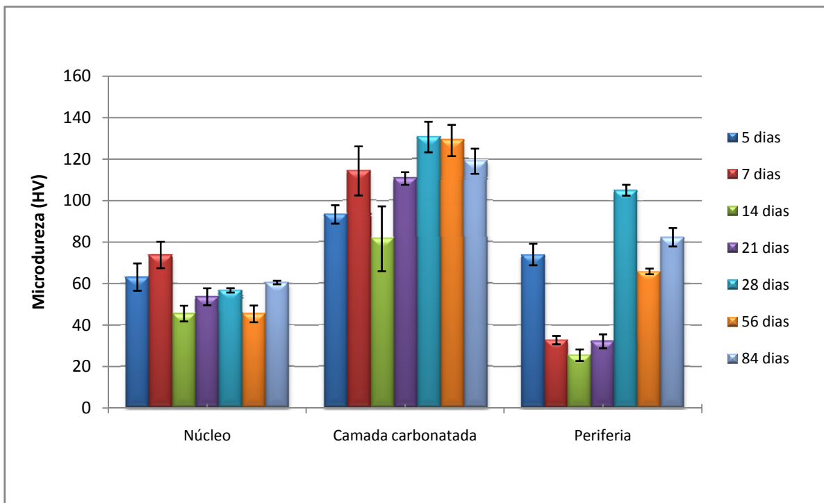
Figura 5.20. Resultados dos ensaios de microdureza Vickers dos experimentos em água saturada com \text{CO}_2 .
