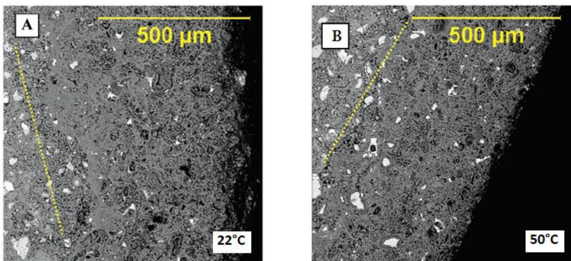
Figura 3.17. Efeito da temperatura de cura no avanço da frente de carbonatação. Fonte: Kutchko et al. (2007).
