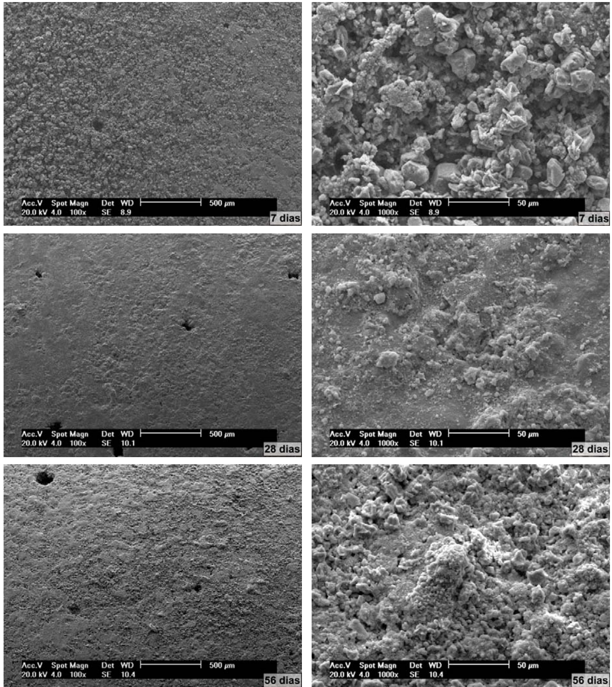
Figura 5.14. Microestrutura da superfície da pasta de cimento em alguns tempos de reação em CO 2 supercrítico úmido.
