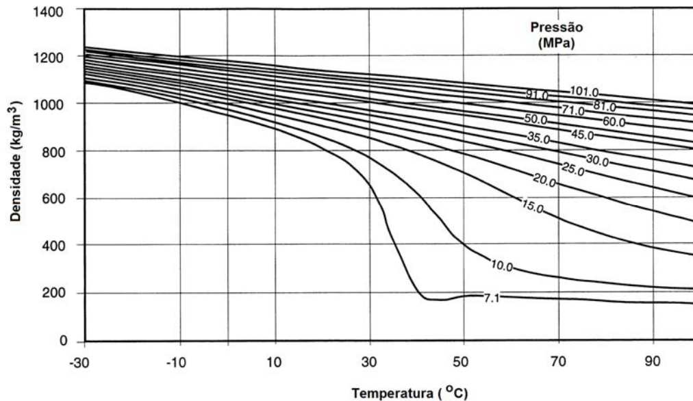
Figura 3.2. Variação na densidade do CO 2 líquido em função da temperatura e pressão (Bachu, 2000).
