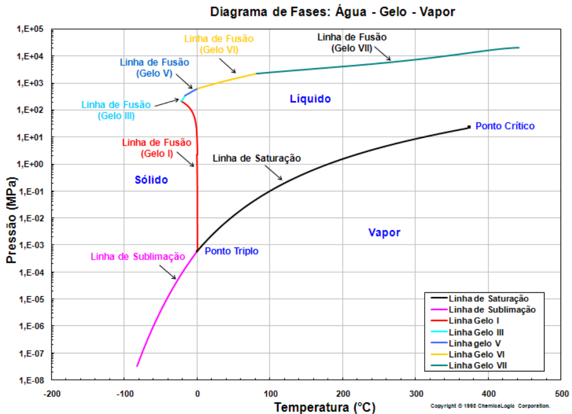
Figura 3.3. Diagrama de fases da água. Adaptado de http://www.chemicallogic.com/download/phase_diagram.pdf .
