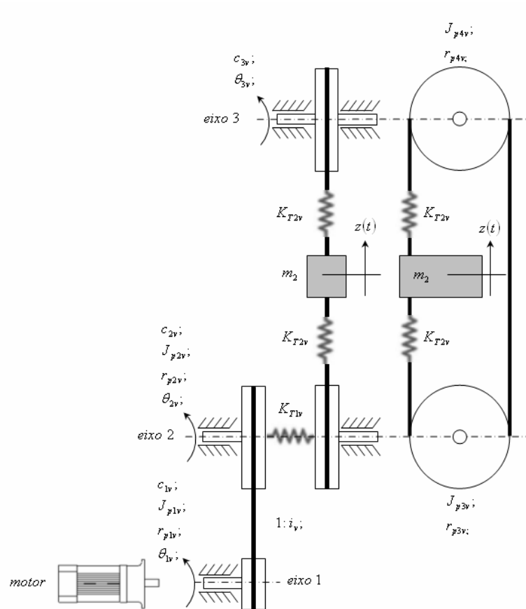
Figura 20 - Modelo da transmissão do posicionamento do elo vertical
