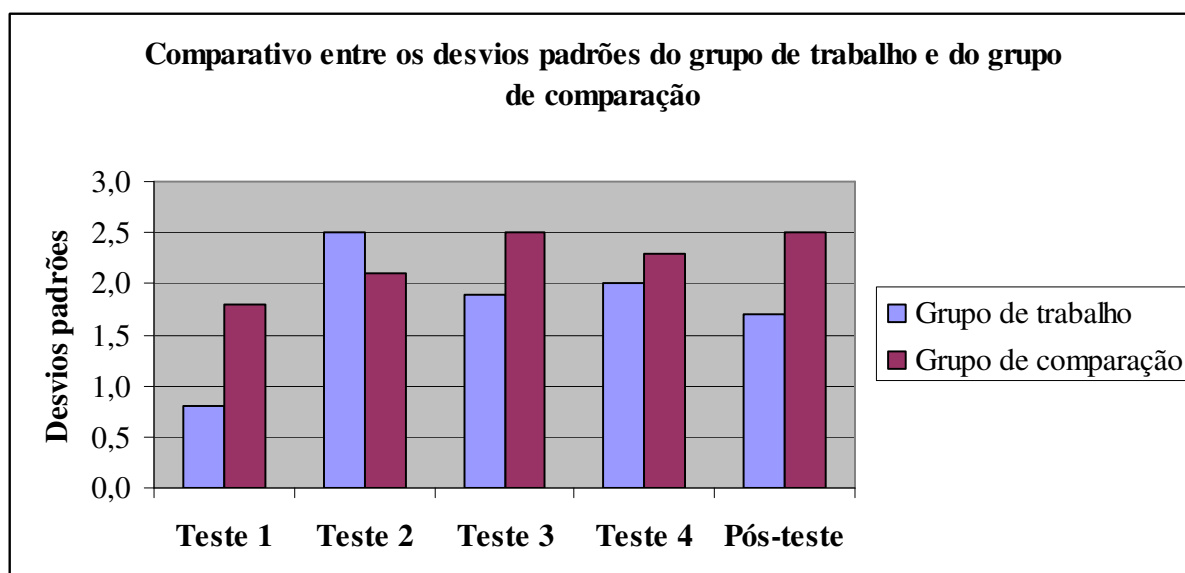
Figura 17 – Gráfico comparativo entre os desvios padrões das notas dos testes.
