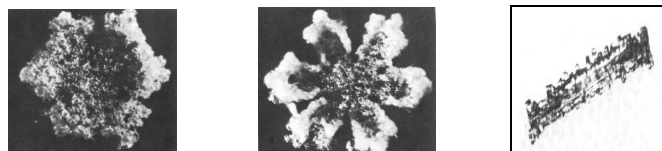
Figura 3.5 – Placa (esquerda), dendrito (centro) e coluna (direita) em processo de riming.
