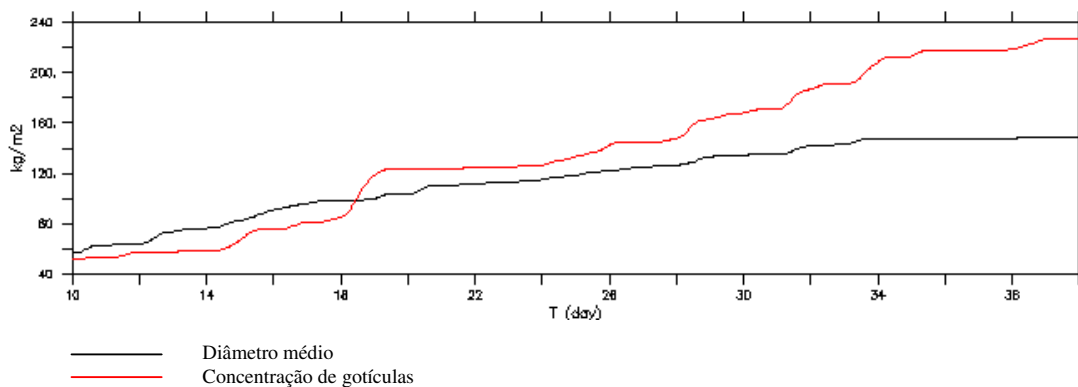
Figura 5.23 – Chuva média acumulada em \text{kg}\cdot\text{m}^{-2} (ou \text{mm}\cdot\text{m}^{-2} ) durante o período de 40 dias (vermelho, simulação com a concentração de partículas e preto, simulação com o diâmetro médio)
