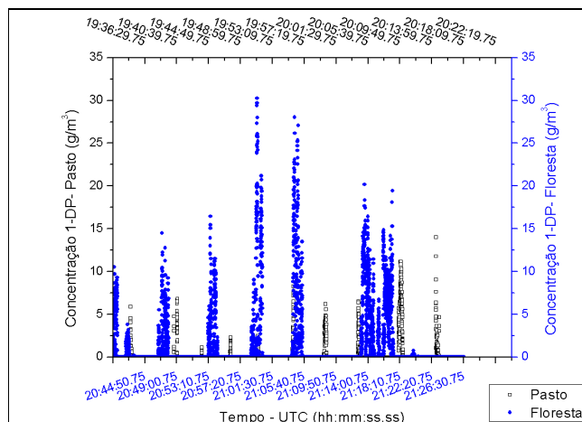
Figura 5.5 - Concentração da 1-DP em quadrados abertos para o pasto e em círculos sólidos para floresta
