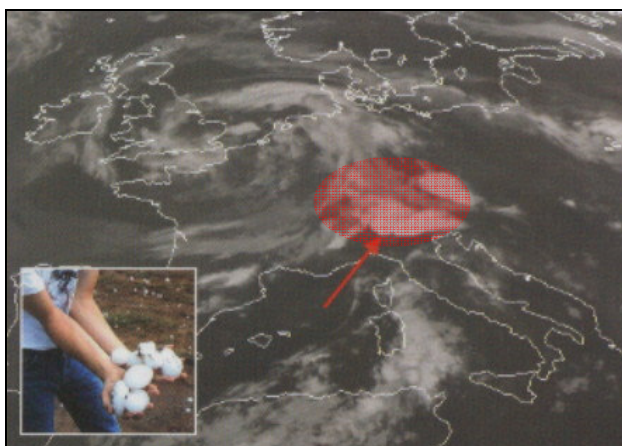
Figura 3.7 – Pedras de granizo coletadas após uma severa chuva de granizo no Norte da Itália em 4 de agosto de 2002. As maiores têm dimensões de vários centímetros e pesavam acima de 700 g. As rajadas de vento atingiram até 36,7 m/s e se registrou precipitação acumulada em 20 minutos de 37,8 mm. A elipse ao fundo indica o sistema de nuvens responsável (canal infravermelho do satélite METEOSAT 00:00h UTC) Adaptada da revista IMAGE, n. 17, novembro de 2002, EUMETSAT.
