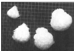
Figura 3.6 – Partículas de graupel coletadas na Suíça. À distância entre as linhas é de 0,2 mm (Aufdermauer, 1963).
