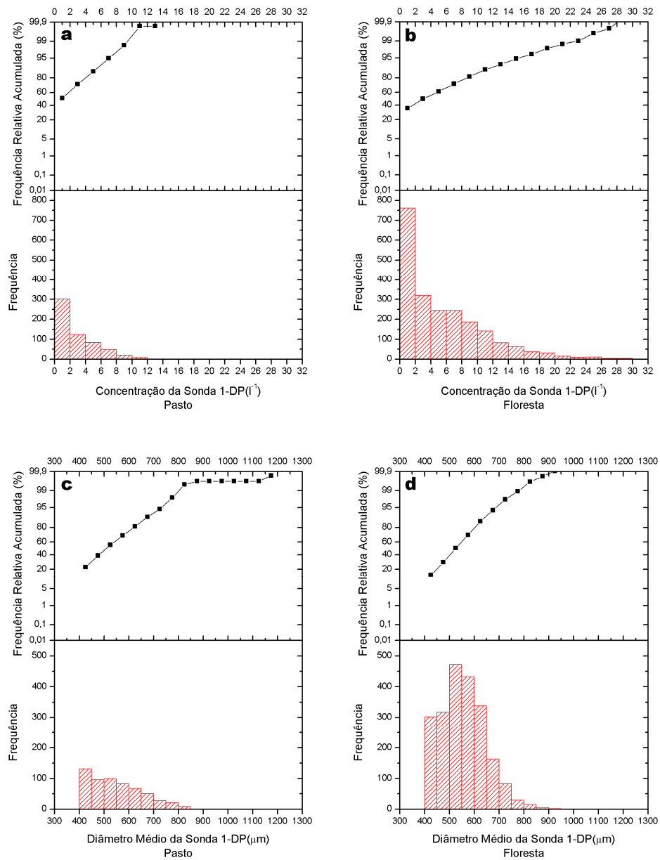
Figura 5.17 – Distribuição de freqüências e freqüência relativa acumulada para a concentração (a e b) e o diâmetro médio (c e d) da sonda 1-DP no pasto e na floresta.
