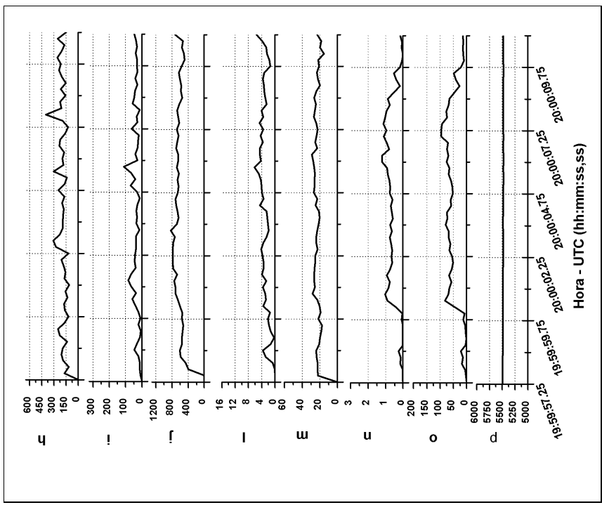
Figura 4.21 - e - Diâmetro Médio 2-DC ( \mu\text{m} ), i - Concentração 2-DC ( \text{l}^{-1} ), j - Diâmetro Médio 1-DP ( \mu\text{m} ), l - Concentração 1- DP ( \text{l}^{-1} ), m - Diâmetro Médio FSSP ( \mu\text{m} ), n - Água Líquida da FSSP ( \text{g}/\text{m}^3 ), o - Concentração FSSP ( \text{cm}^{-3} ), p - Altitude - GPS (m) entre 19:59:57h e 20:00:09h UTC.
