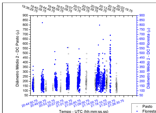
Figura 5.9- Diâmetro médio 2-DC em quadrados abertos para o pasto e em círculos sólidos para floresta
