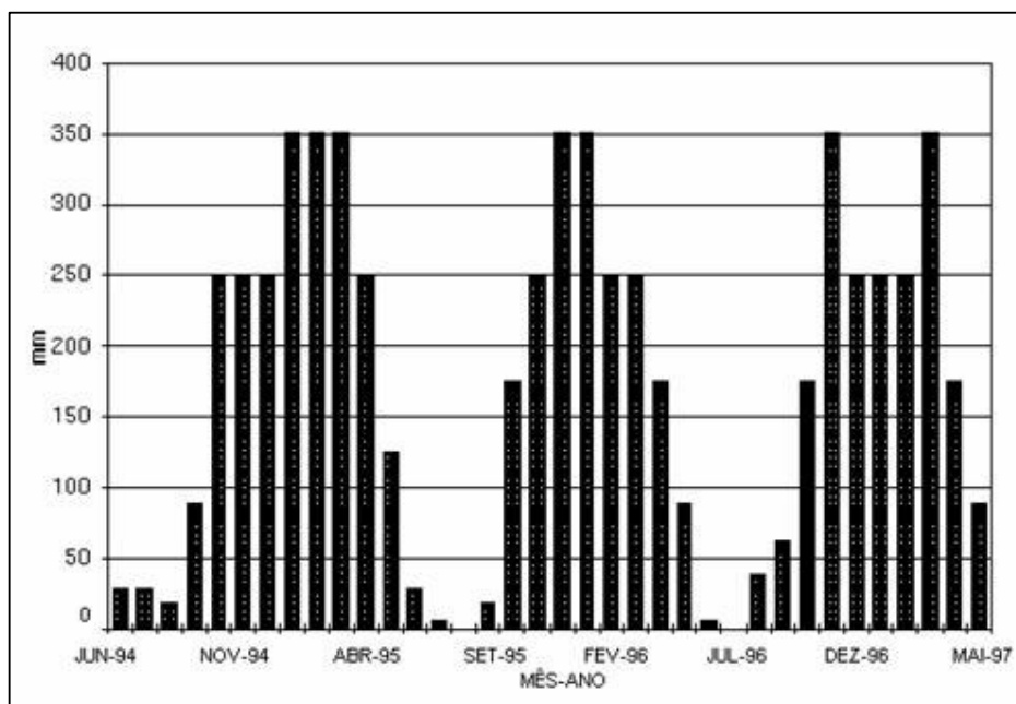
Figura 2.3 - Índices de precipitação de junho de 1994 a maio de 1997 no estado de Rondônia, segundo dados obtidos no experimento ABRACOS.
