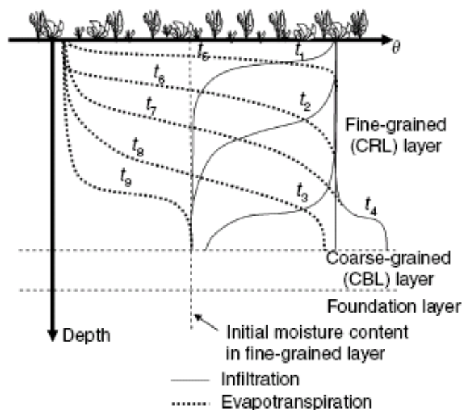
Figura 3.8- flutuação do teor de umidade (ZORNBERG, 2007)
