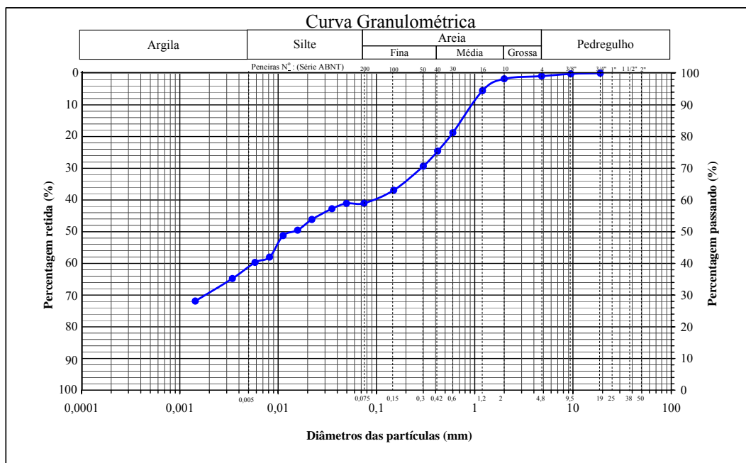
Figura 4.10 – Curva granulométrica – Rio das Ostras (PIRES, 2007)
