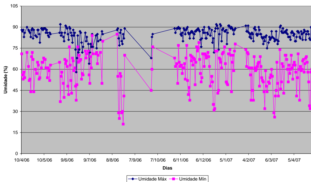
Figura 4.2 – Gráfico Umidade (%) x Dia (Niterói)
