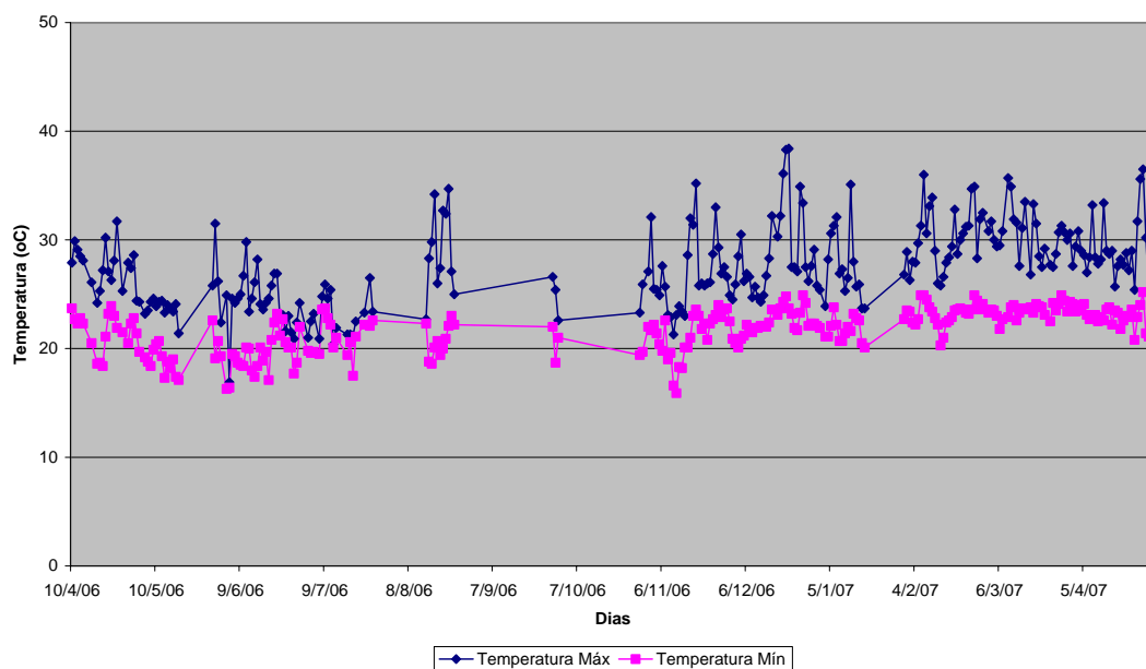
Figura 4.3 – Gráfico Temperatura (°C) x Dia (Niterói)
