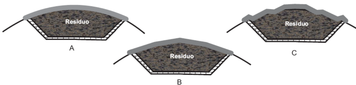
Figura 3.5 – Tipos de configurações de cobertura final (KOERNER e DANIEL, 1997)
