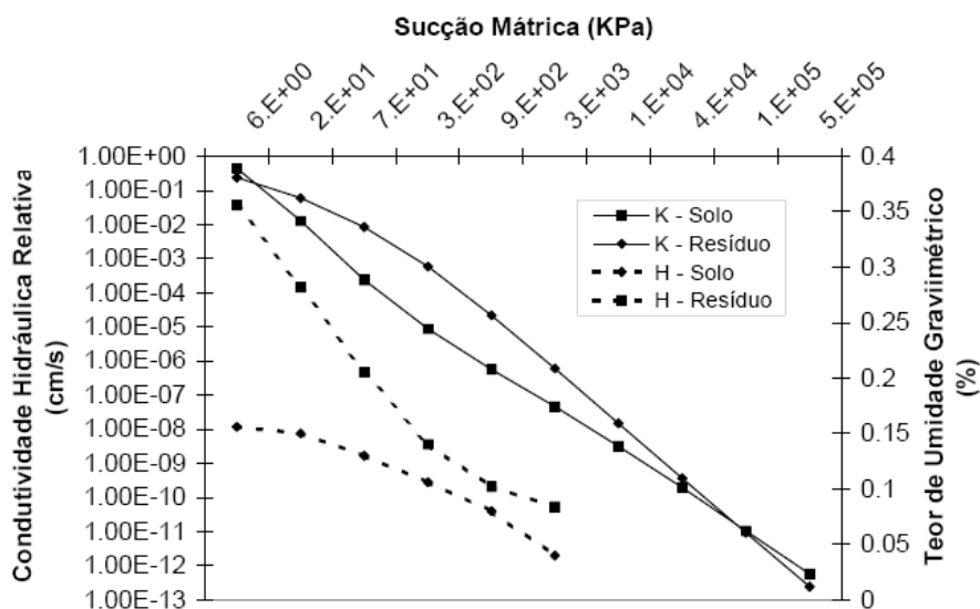
Figura 3.13 – Curva característica dos materiais e condutividade hidráulica, ambas fornecidas ao programa SoilCover (MENDONÇA ET AL., 2003)
