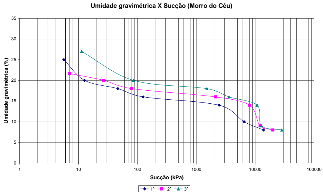
Figura 4.18 – Curva característica Morro do Céu
