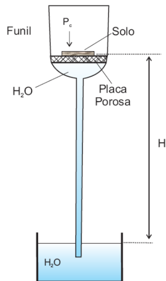
Figura 2.6 – Funil de Placa Porosa (REICHARDT, 1985)
