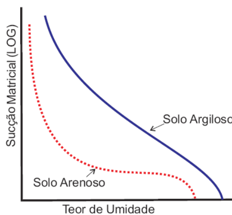
Figura 2.9 – Curvas características de solos argilosos e arenosos (HILLEL, 1971).
