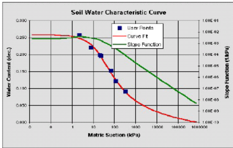
Figura 3.9 – Curva sucção x umidade – Aterro de Palmas (VIDAL E BORMA, 2006)
