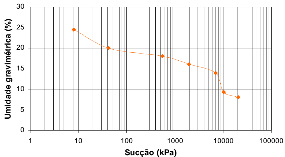
Figura 4.19 – Curva característica média Morro do Céu
