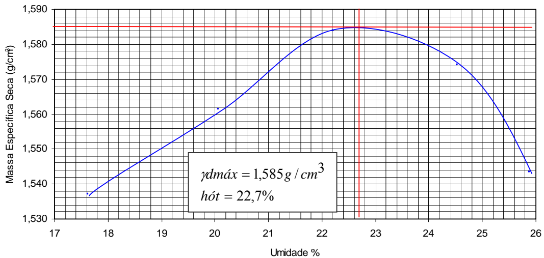
Figura 4.12 – Curva de Compacção – Rio das Ostras
