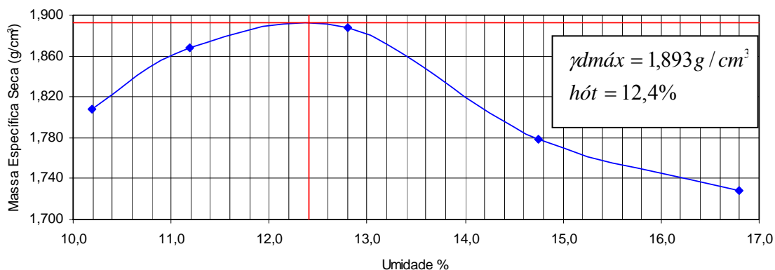
Figura 4.11 – Curva de Compactação – amostra nº 2 Morro do Céu
