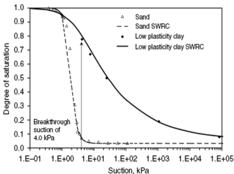
Figura 3.6 – efeito “quebra” de capilaridade (ZORNBERG, 2007)
