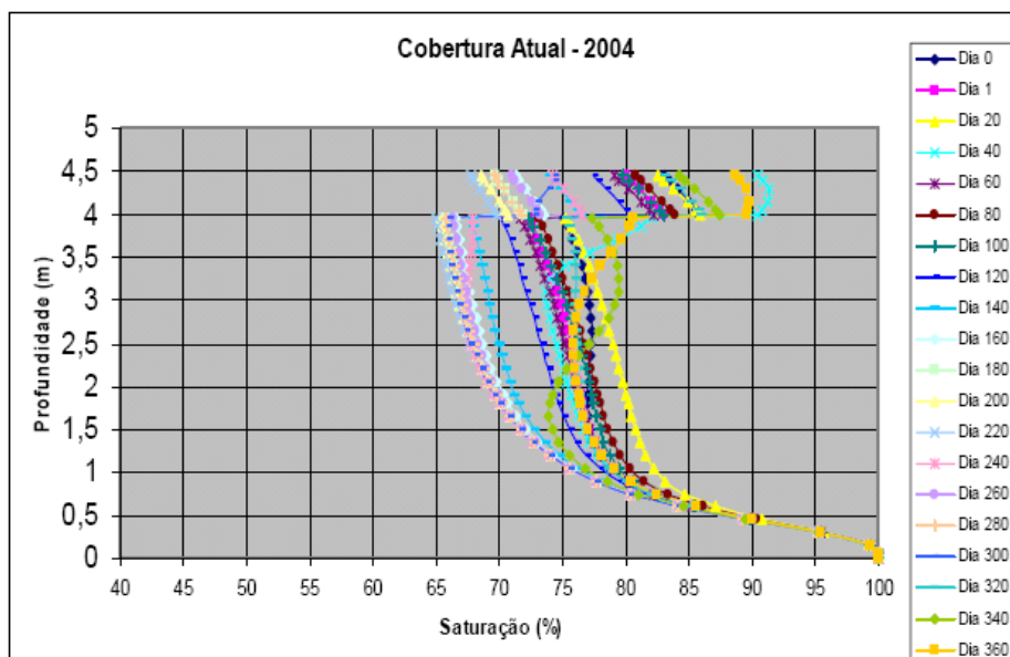
Figura 3.12 - Perfil de saturação ano de 2004 (VIDAL E BORMA, 2006)
