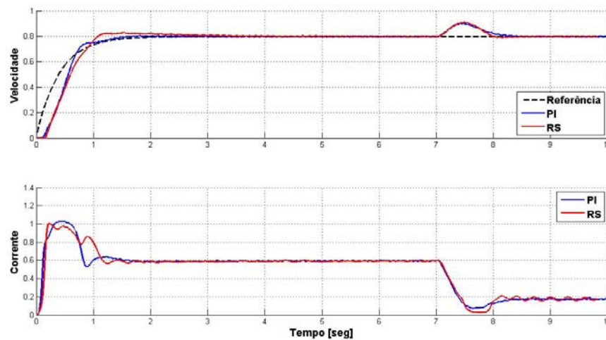
Figura 5.14 – Respostas reais com partida a carga plena e referência 0,8 [pu].
