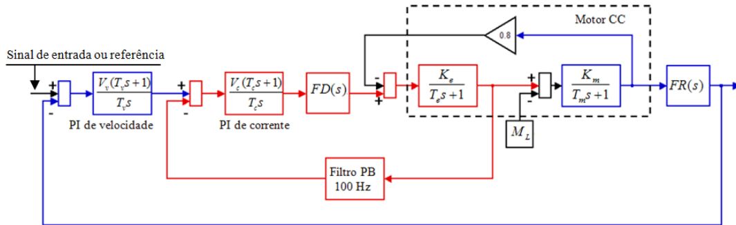
Figura 3.16 – Diagrama em blocos das malhas de controle resultantes.
