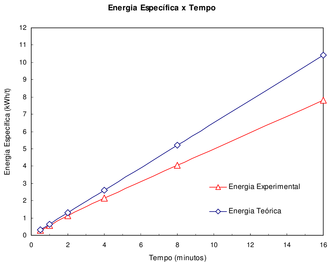
Figura 5.7 - Energia específica experimental e teórica do teste em moinho de laboratório na condição otimizada prevista pela simulação do moinho industrial.
