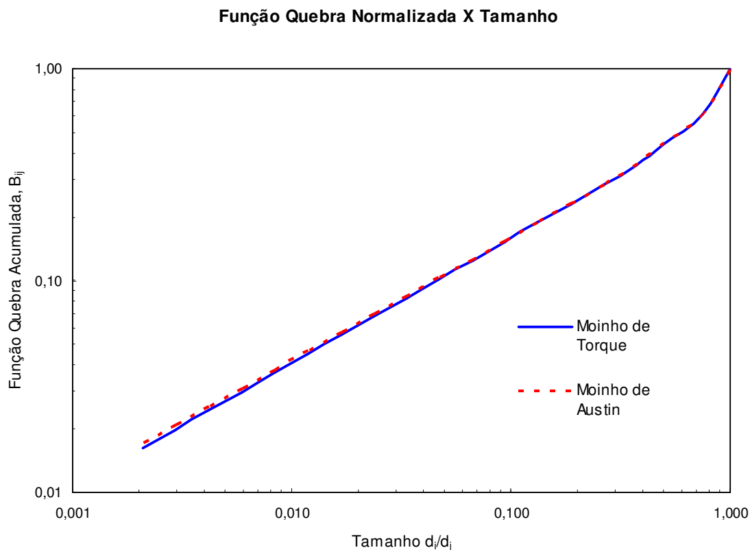
Figura 5.11 - Função quebra normalizada.
