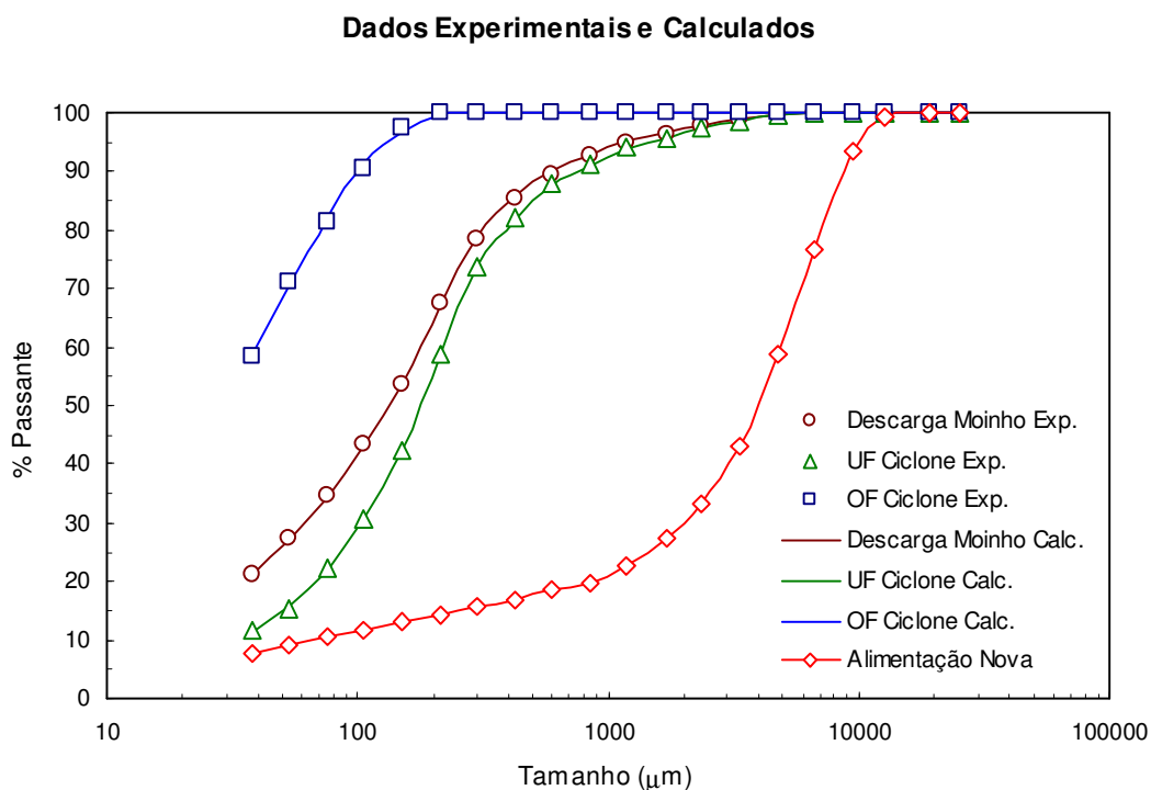
Figura 5.3 - Dados experimentais e calculados do circuito.
