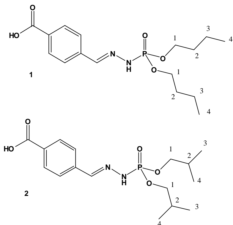
Figura 4.7. Estruturas das fosforilidrazonas 1 e 2 sintetizadas e testadas como inibidores de germinação por nosso grupo (NOGUEIRA et al. , 2007). Os átomos de hidrogênio foram omitidos.
