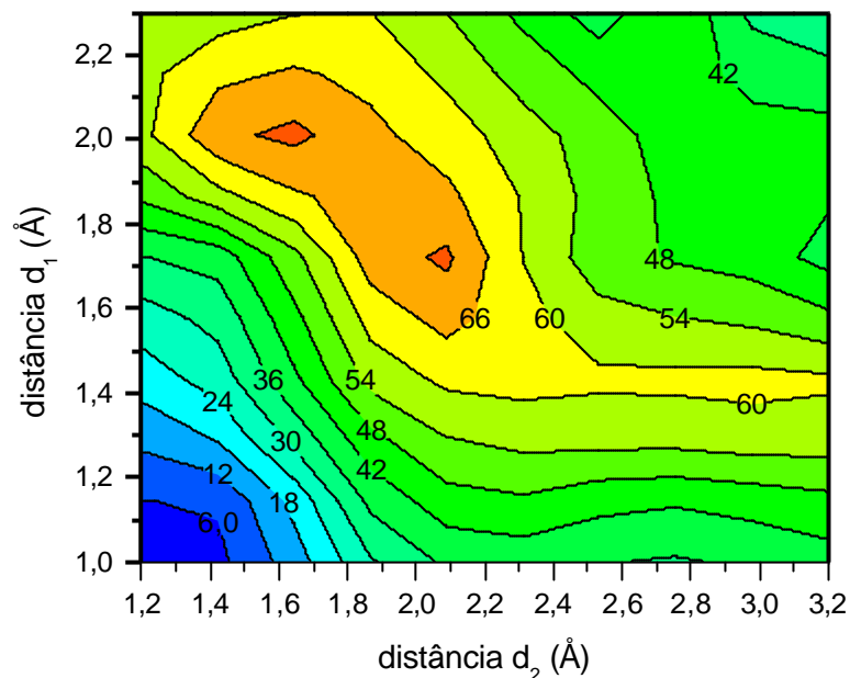
Figura 5.7 Superfície com os contornos de entalpia da reação, com Glu362 atuando como um catalisador básico na etapa de eliminação para a formação do produto EPSP.
