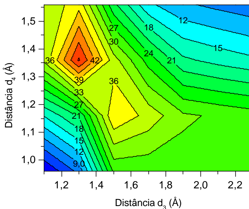
Figura 5.43. Contornos de entalpia da segunda parte do mecanismo, com Lys432 atuando como catalisador ácido e Asp334 atuando como catalisador básico indireto, em função das distâncias d_3 e d_4 .
