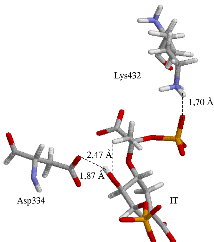
Figura 5.37. Representação do IT e dos resíduos Asp334 e Lys432 no modelo da EPSPS de O. sativa . Os demais resíduos e moléculas de água foram omitidos para maior clareza. As cores branca, vermelha, azul, cinza e amarela mostram, respectivamente, os átomos de hidrogênio, oxigênio, nitrogênio, carbono e fósforo.
