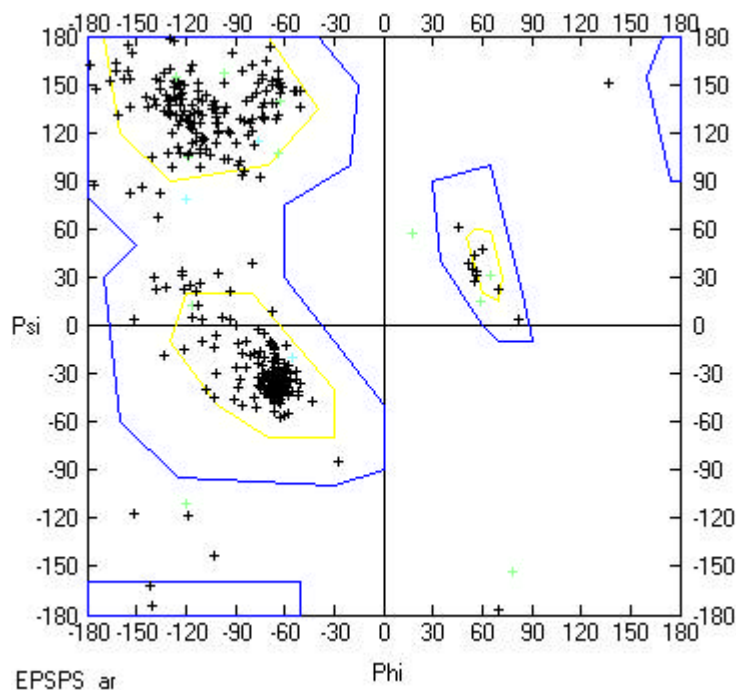
Figura 5.3 Gráfico de Ramachandran do modelo homólogo da O. sativa . As cruzes em ciano e verde representam resíduos localizados nas sequências de inserção.
