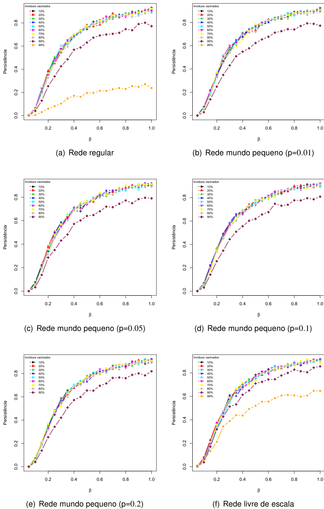
Figura 3.12: Persistência nos três tipos de rede com vacinação por conglomerados \sigma = 1 .
