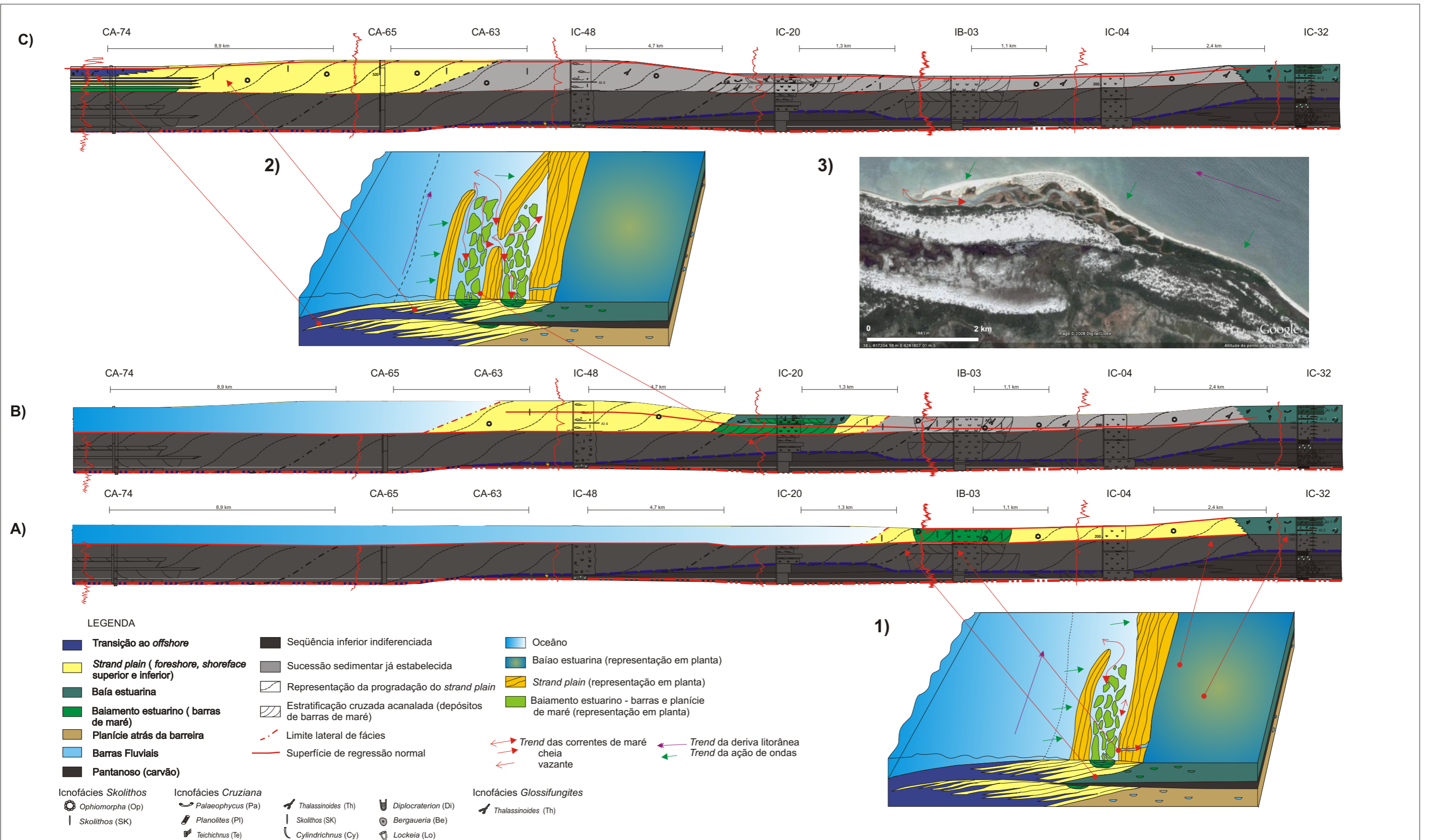
Figura 5.13 - Modelo sedimentológico e estratigráfico para a construção do strand plain que caracteriza o topo da Sequência D: A, B e C) desenvolvimento da linha de costa no espaço e tempo no intermediário de maior frequência (Seção 4). Observar a relação entre as fácies de shoreface e de baiamentos estuarinos evoluindo em sentido ao oceano, juntamente com o estabelecimento das icnofácies sin-depositivas ( Skolithos e Cruziana ) e pós-depositivas ( Glossifungites ); 1 e 2) modelo esquemático de desenvolvimento da linha de praia, associando os ambientes com os descritos na seção; 3) análogo atual localizado na costa oeste da ilha de Madagascar, África, com a área interna aos cordões litorâneos.
