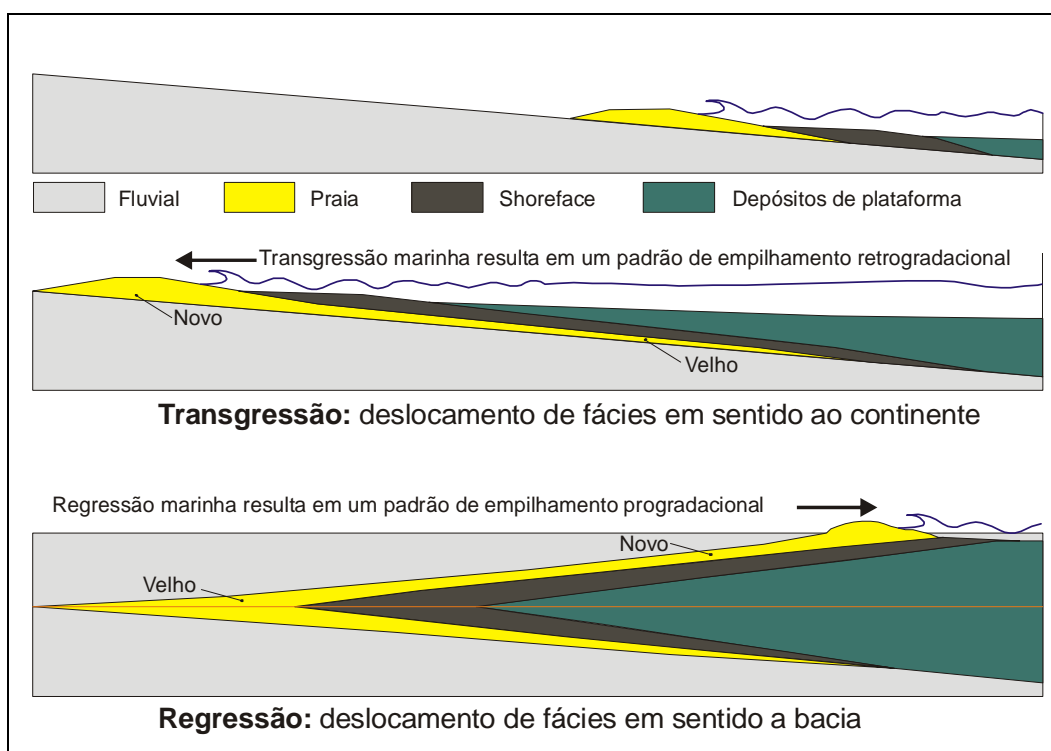
Figura 3.3 – Representação simplificada de depósitos transgressivos e regressivos, expondo as variações laterais de fácies, bem como a superfície que separa os depósitos retrogradacionais sobrepostos por geometrias progradacionais. Essa superfície é definida como superfície de máxima inundação ( maximum flooding surface – MFS) (Catuneanu 2002).
