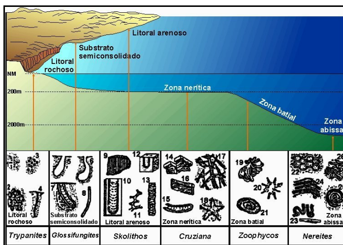
Figura 4.14 – Distribuição das icnofácies conforme Frey & Pemberton (1985). Icnogêneros: 1 Caulostrepsis ; 2 Entobia ; 3 perfurações de equinóides; 4 Trypanites ; 5 Teredolites ; 6 Thalassinoides ; 7-8 Gastrochaenolites ; 9 Diplocraterion ; 10 Skolithos ; 11-12 Psilonichnus ; 13 Macanopsis ; 14 Skolithos ; 15 Diplocraterion ; 16 Arenicolites ; 17 Ophiomorpha ; 18 Phycodes ; 19 Rhizocorallium ; 20 Teichichnus ; 21 Planolites ; 22 Asteriacites ; 23 Zoophycos ; 24 Lorenzina ; 25 Zoophycos ; 26 Paleodictyon ; 27 Taphrhelminthopsis ; 28 Helminthoidea; 29 Cosmorhaphie ; 30 Spirorhaphie .
