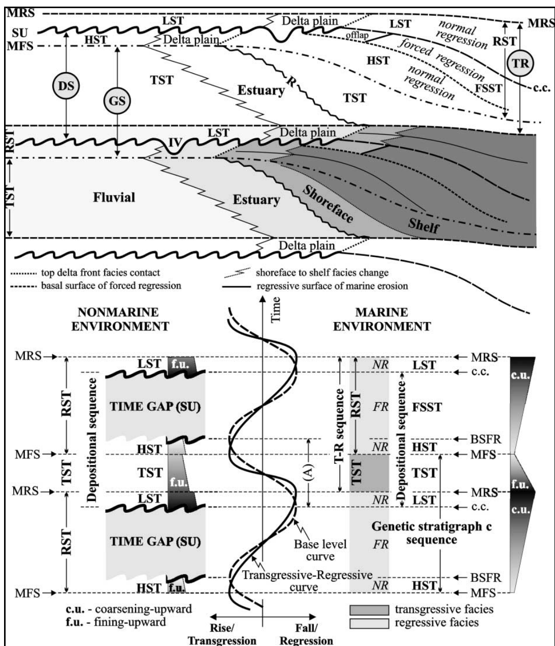
Figura 3.7 - Sequências, tratos de sistemas e superfícies estratigráficas definidas em relação à curva de variação do nível de base e curva T-R (Catuneanu 2006). Abreviações: SU— subaerial unconformity ; c.c.— correlative conformity ; BSFR— basal surface of forced regression ; MRS— maximum regressive surface ; MFS— maximum flooding surface ; R— ravinement surface ; IV— incised valley ; (A)— espaço de acomodação positivo (subida do nível de base) ; NR— normal regression ; FR— forced regression ; LST— lowstand systems tract ; TST— transgressive systems tract ; HST— highstand systems tract ; FSST— falling stage systems tract ; RST— regressive systems tract ; DS— depositional sequence ; GS— genetic stratigraphic sequence ; e TR— transgressive-regressive sequence .
