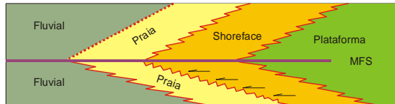
Figura 3.10 – Arquitetura das fácies e superfícies estratigráficas no ponto de máxima transgressão da linha de praia. A posição da WNRS varia com o tipo de configuração da linha de praia, que pode ser de mar aberto ou de desembocaduras de rios (deltas). Neste contexto, a superfície de ravinamento geralmente se assenta na base de fácies de shoreface transgressivas. A superfície de máxima inundaçã (MFS) separa os depósitos retrogradacionais (sotopostos) dos depósitos progradacionais (sobrepostos). Nos tratos transgressivos dentro do padrão de fácies, o contato de fácies arenosas de shoreface com as argilas de plataforma é definido pela WFS ( within-trend flooding surface ) (Catuneanu 2002).
