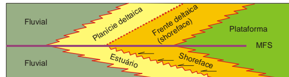
Figura 3.10 – Arquitetura das fácies e superfícies estratigráficas no ponto de máxima transgressão da linha de praia. A posição da WNRS varia com o tipo de configuração da linha de praia, que pode ser de mar aberto ou de desembocaduras de rios (deltas). Neste contexto, a superfície de ravinamento geralmente se assenta na base de fácies de shoreface transgressivas. A superfície de máxima inundaçã (MFS) separa os depósitos retrogradacionais (sotopostos) dos depósitos progradacionais (sobrepostos). Nos tratos transgressivos dentro do padrão de fácies, o contato de fácies arenosas de shoreface com as argilas de plataforma é definido pela WFS ( within-trend flooding surface ) (Catuneanu 2002).
