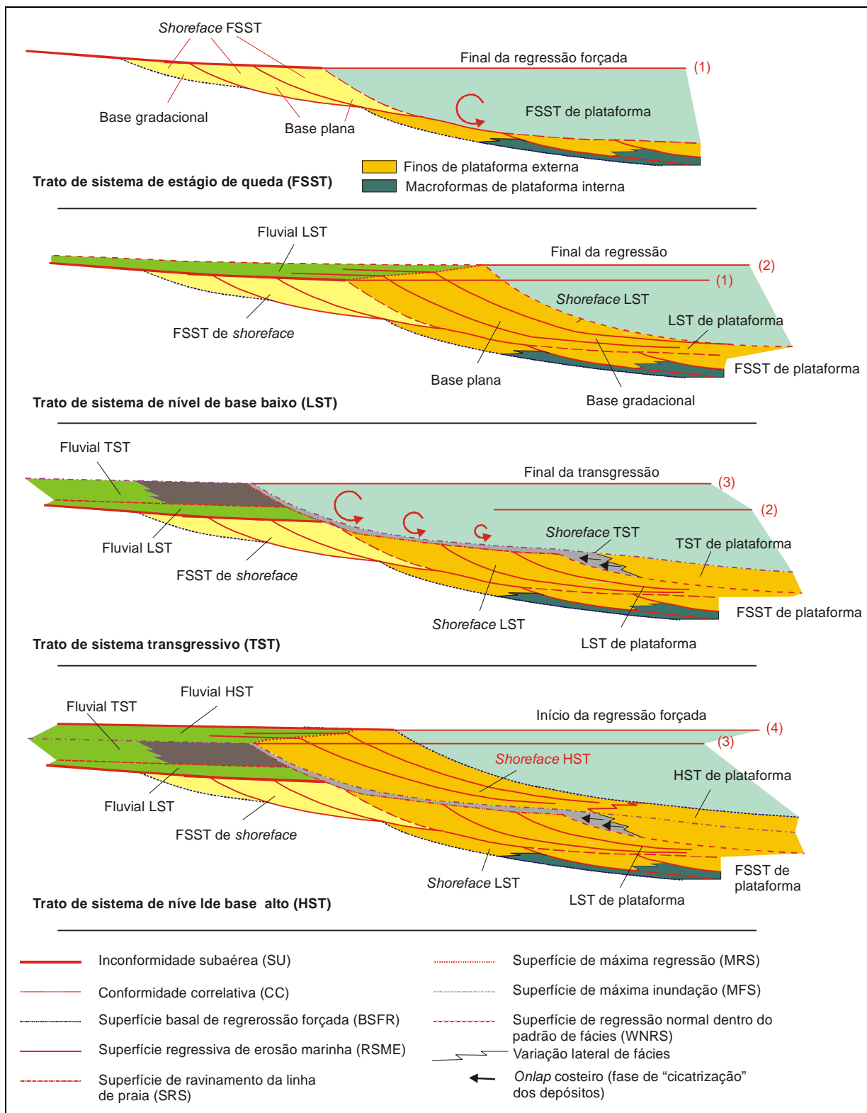
Figura 3.13 – Arquitetura detalhada das fácies e superfícies estratigráficas em uma zona transicional entre os ambientes fluviais e marinhos rasos (Catuneanu 2002).
