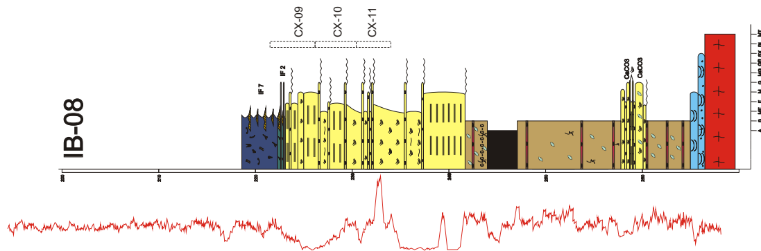
Figura 4.7 - Detalhe do poço IB-08, apresentando associação de fácies praias relacionadas a interdigitação de depósitos de shoreface (Qa2) com depósitos de foreshore (Qa1). Acima, observam-se depósitos de baía estuarina rasa (Ht / IF 1) sobrepostos por depósitos de costa a fora (Ht / IF 7).
