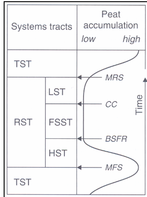
Figura 3.15 – Tendências de acumulação de turfeiras durante os vários estágios dos ciclos de variação do nível de base em resposta às mudanças do espaço de acomodação. Abreviações: TST – trato de sistemas transgressivos; RST – trato de sistemas regressivos; HST – trato de sistemas de mar alto; FSST – trato de sistemas de início de queda; LST – trato de sistema de nível de base baixo; MFS – superfície de máxima inundação, BSFR – superfície basal de regressão forçada; CC - conformidade correlativa e; MRS – superfície de máxima regressão (Catuneanu 2006).
