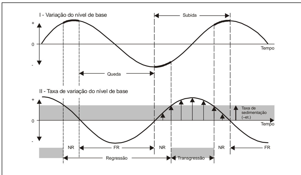
Figura 3.2 - Conceito de transgressão, regressão normal e regressão forçada definido através da interação entre sedimentação e variação do nível de base (Catuneanu 2002). A curva em sino superior expõe a magnitude da variação do nível de base através do tempo. As porções mais espessas da curva indicam o estágio inicial e o final da subida do nível de base, quando o estágio de subida (crescente e decrescente a partir de zero, respectivamente) é ultrapassado pela taxa de sedimentação. A curva em sino inferior representa as taxas de variação do nível de base. Note que as taxas de variação do nível de base são zero no início do estágio de subida e de queda. As taxas de variação do nível de base são maiores nos pontos de inflexão do topo da curva. Para simplificar, a taxa de sedimentação foi mantida constante para representar as flutuações do nível de base. Abreviações: FR = regressão forçada; NR = regressão normal.
