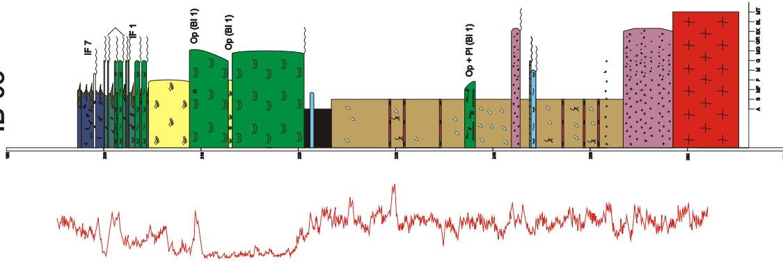
Figura 4.10 - Detalhe do poço IB-03, apresentando fácies de shoreface superior (litofácies Qa2) sobreposta por dedepósitos relacionados a ambientes de baía estuarina (Ht) contendo a icnofábrica IF1 (litofácies Ht) cortada por delgadas camadas arenosas (Aq4). Topo da seqüência já apresenta uma condição marinha mais equilibrada, com maior icnodiversidade (IF7) e ocorrência esporádica da litofácies Qa4.
