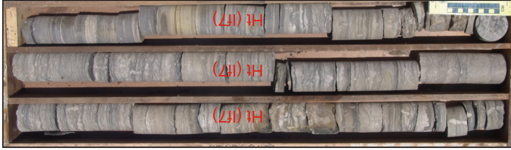
Figura 4.10 - Detalhe do poço IB-03, apresentando fácies de shoreface superior (litofácies Qa2) sobreposta por dedepósitos relacionados a ambientes de baía estuarina (Ht) contendo a icnofábrica IF1 (litofácies Ht) cortada por delgadas camadas arenosas (Aq4). Topo da seqüência já apresenta uma condição marinha mais equilibrada, com maior icnodiversidade (IF7) e ocorrência esporádica da litofácies Qa4.
