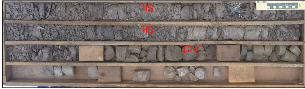
Figura 4.3 - Detalhe do poço IB-74, apresentando associação de fácies lagunares pantanosas (Slt e SltC) cortadas por depósitos arenosos de origem fluvial (litofácies Ac1e Ac2).
