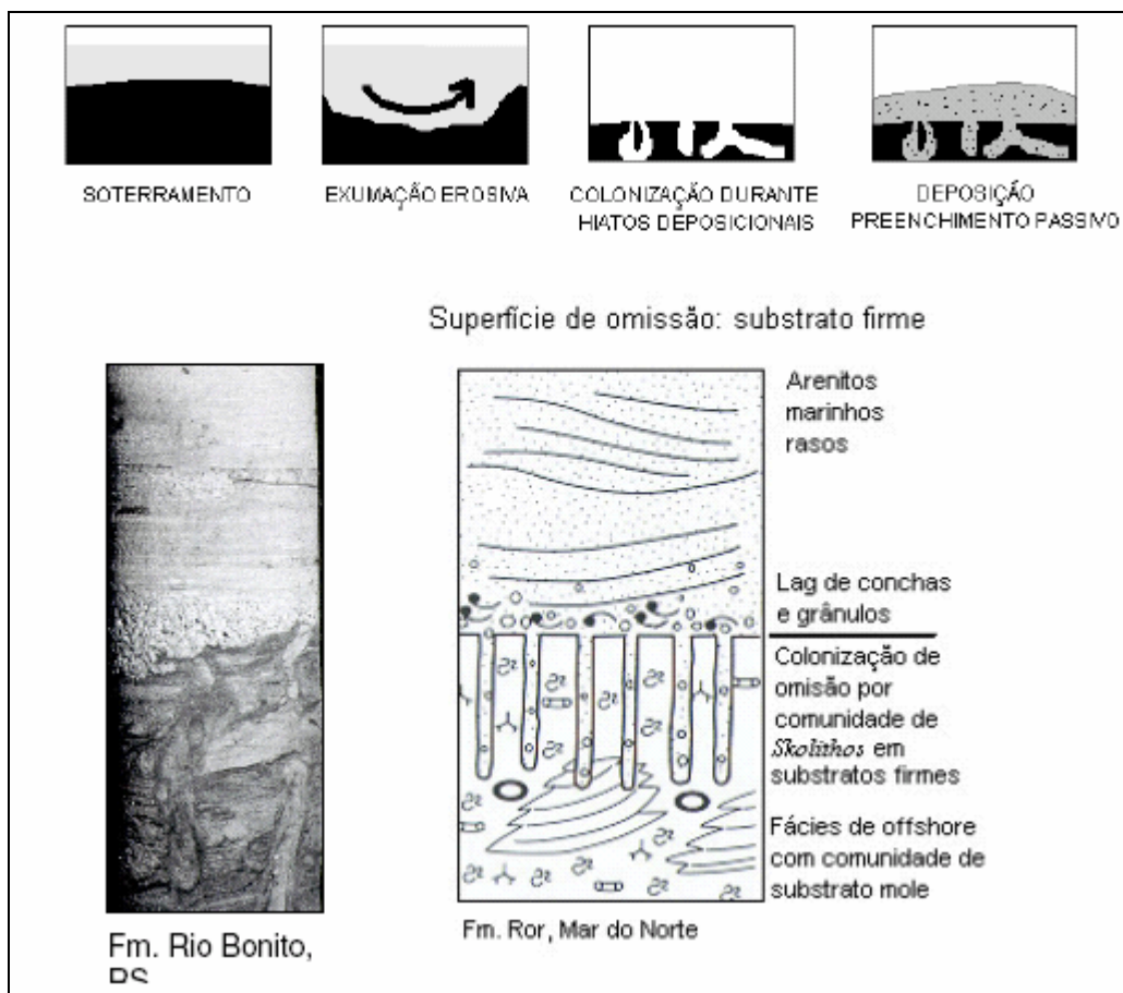
Figura 3.12. - Estágios de desenvolvimento da Icnofácies Glossifungites e seu papel na diagnose de superfícies de omissão (Netto 2001).
