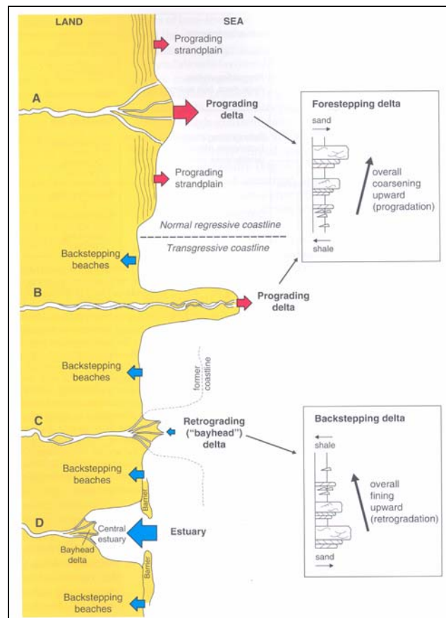
Figura 3.14 – Representação gráfica simplificada do desenvolvimento da linha de praia durante a subida do nível de base. O caráter progradacional ou retrogradacional da linha de praia em cenários dominados por rios ou de mar aberto são controlados pelo balanço entre a taxa de suprimento sedimentar e taxa de elevação do nível de base. Linhas de costas controladas por regressão normal (mar alto e mar baixo) são caracterizadas pela progradação de sistemas fluviais em sentido a porção marinha da bacia. As linhas de costa transgressivas são caracterizadas pelo padrão retrogradacional em costas de mar aberto, enquanto que em cenários dominados pela ação de rios, o caráter pode ser progradacional (delatas) ou retrogradacional (estuários e bayhead deltas). A -sistemas deltaicos progradacionais associados à regressão normal; B -sistemas deltaicos progradacionais associados a cenários transgressivos; C -sistemas deltaicos retrogradacionais ( bayhead ) em cenários transgressivos; e D -sistemas estuarinos bem desenvolvidos (Catuneanu 2006).
