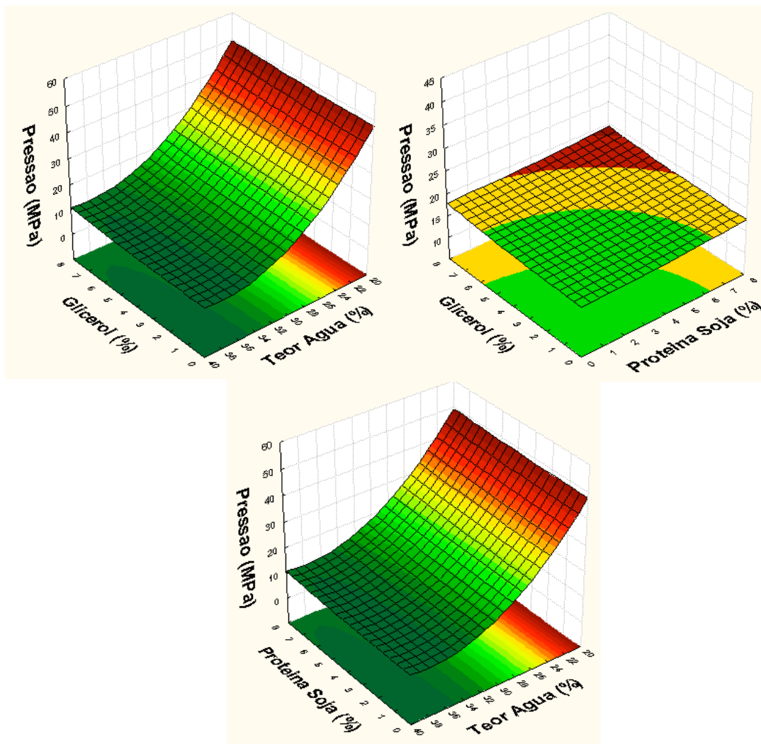
Figura 14. Efeito das variáveis quantitativas Glicerol (%), Proteína de Soja (%) e Teor de água (%), na Pressão de saída (MPa) dos filmes biodegradáveis extrusados de farinha de mandioca.
