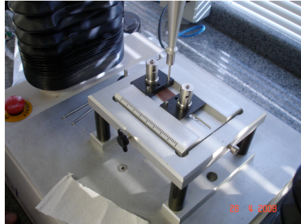
Figura 8. Análise de perfuração com o Texturômetro TA.TX2 Stable Micro Systems.
