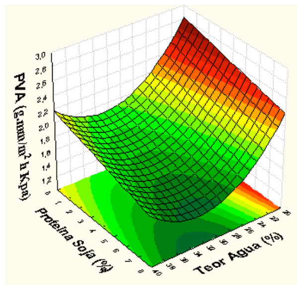
Figura 13. Efeito das variáveis quantitativa Proteína de Soja (%) e Teor de água (%), na Permeabilidade ao vapor da água (g.mm/m 2 h KPa), dos filmes biodegradáveis extrusados de farinha de mandioca.
