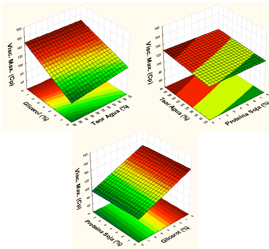
Figura 26. Efeito das variáveis quantitativas Glicerol (%), Proteína de Soja (%) e Teor de água (%), na Viscosidade Máxima (cP) dos filmes biodegradáveis extrusados de farinha de mandioca.
