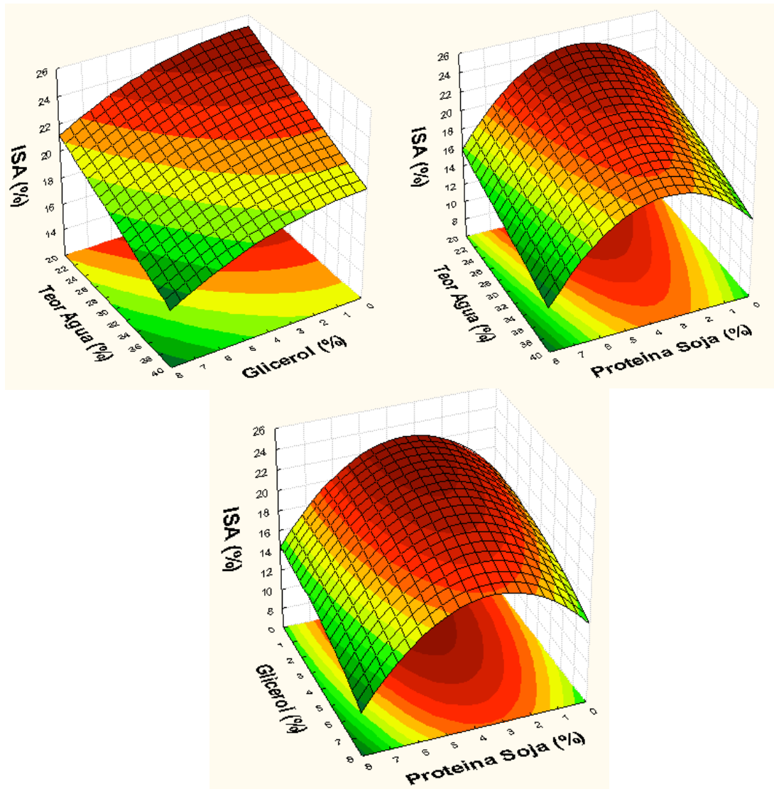
Figura 21. Efeito das variáveis quantitativas Glicerol (%), Proteína de Soja (%) e Teor de água (%), no ISA (%) dos filmes biodegradáveis extrusados de farinha de mandioca.
