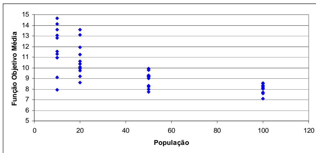
Figura B.6 – Valor médio de função objetivo em função do tamanho da população para a aptidão calculada através de classificação.
