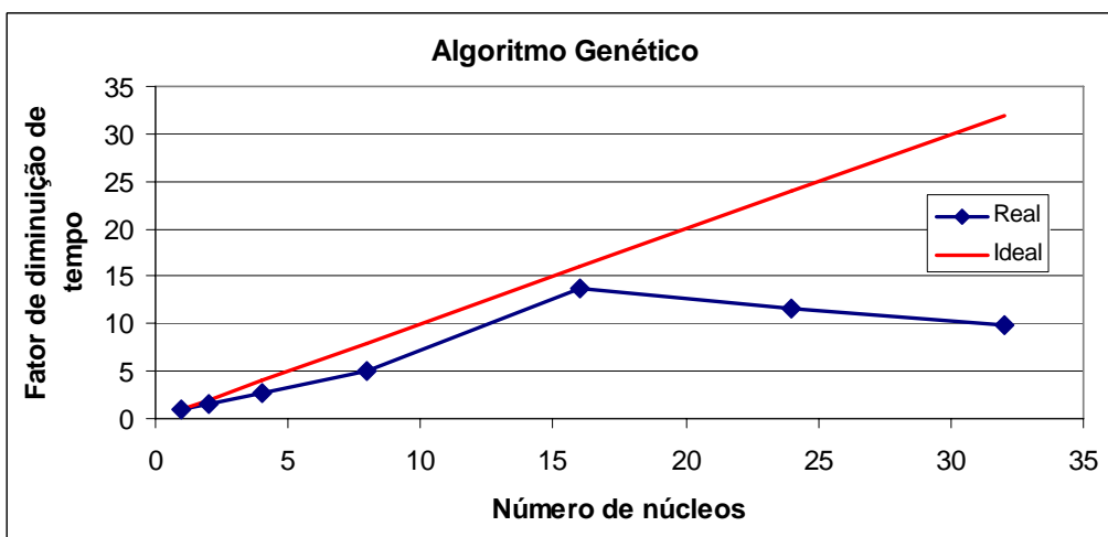
Figura 7.10 – Ganho de desempenho com a paralelização para o Algoritmo Genético.
