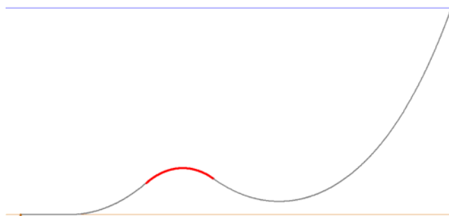
Figura 7.7 – Linha Elástica da configuração ótima para o caso com correntezas fora do plano.
