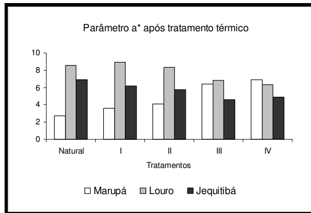
Figura 4.3: Parâmetro colorimétrico a* das madeiras de Simarouba amara , Sextonia rubra e Cariniana micrantha em condição natural e após aplicação de quatro tratamentos térmicos (I: 150°C/1h; II: 150°C/2h; III: 200°C/1h; IV: 200°C/2h).
