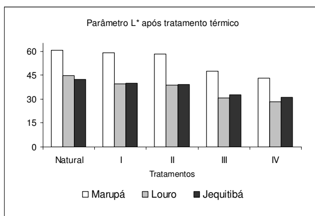
Figura 4.2: Parâmetro colorimétrico L^* das madeiras de Simarouba amara , Sextonia rubra e Cariniana micrantha em condição natural e após aplicação de quatro tratamentos térmicos (I: 150°C/1h; II: 150°C/2h; III: 200°C/1h; IV: 200°C/2h).
