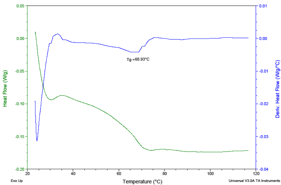
FIGURA 18 - Resina acrílica modificada 1,5%.
