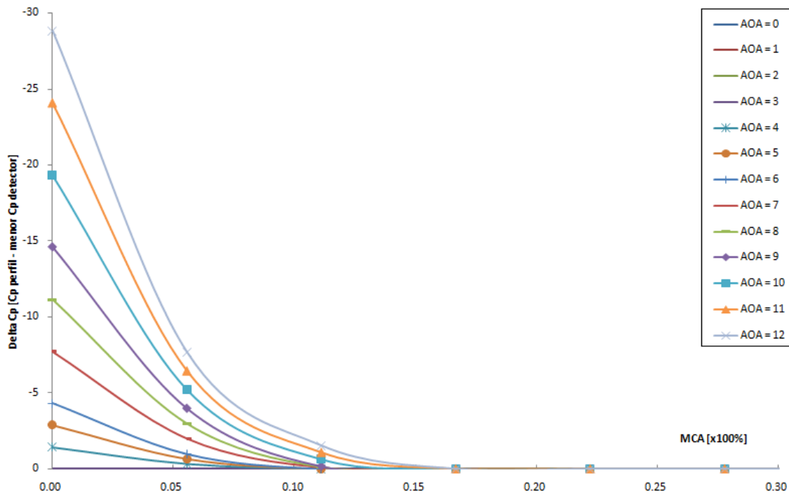
Figura 7.1 – Avaliação da susceptibilidade a formação de gelo não-detectável, perfil NACA0004.
