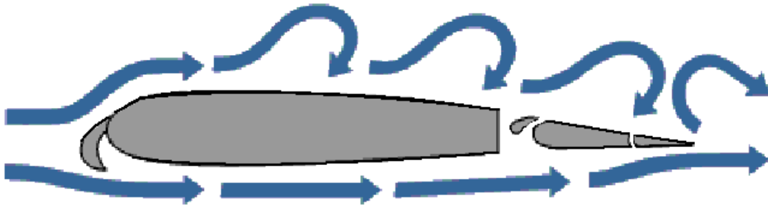
Figura 2.5 - Efeito da camada de 'clear ice' ou 'mixed ice' no escoamento junto a superfície de uma asa.
