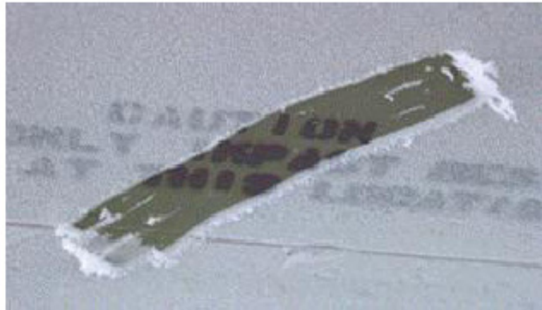
Figura 2.1 - Formação de Gelo Branco 'rime ice' .
