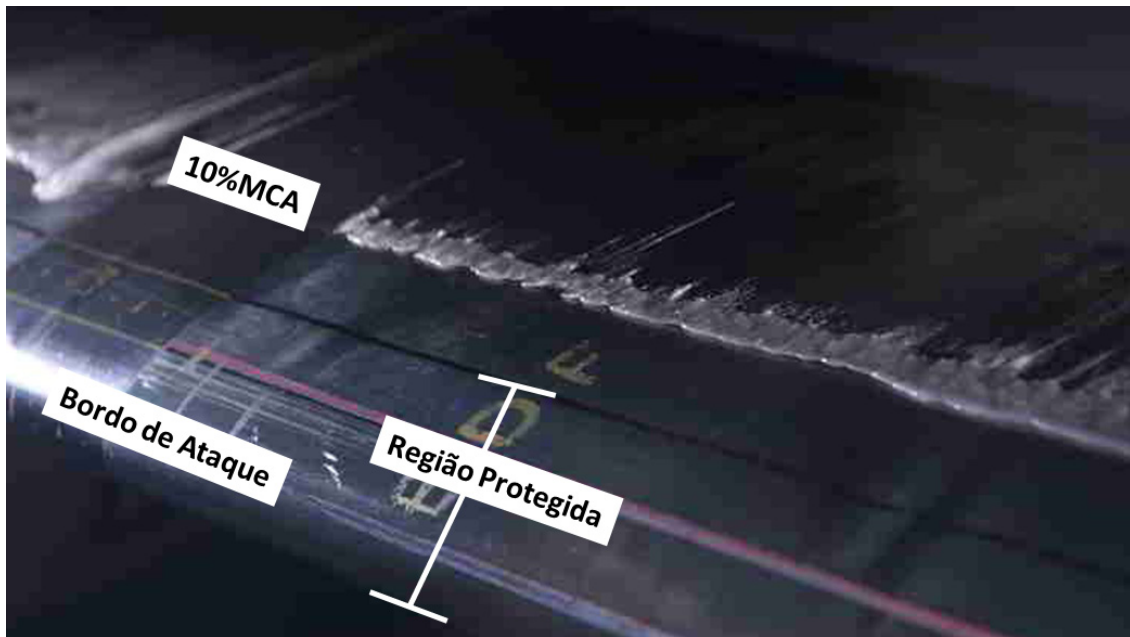
Figura 8.8 – Fotografia com a formação do gelo tipo ‘clear ice’ com a posição de ocorrência deste gelo (FAA/AC 25.1419-A1).
