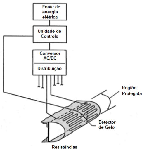
Figura 3.3 - Hélice com sistema de proteção contra gelo por aquecimento elétrico.
