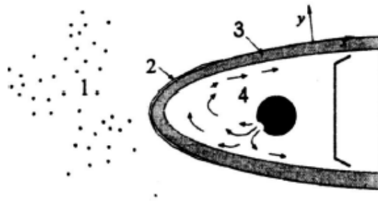
Figura 2.18 - Modelo matemático da formação de gelo: diferentes regiões de estudo.
