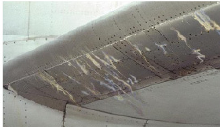
Figura 2.2 - Formação de Gelo Claro 'clear ice' .
