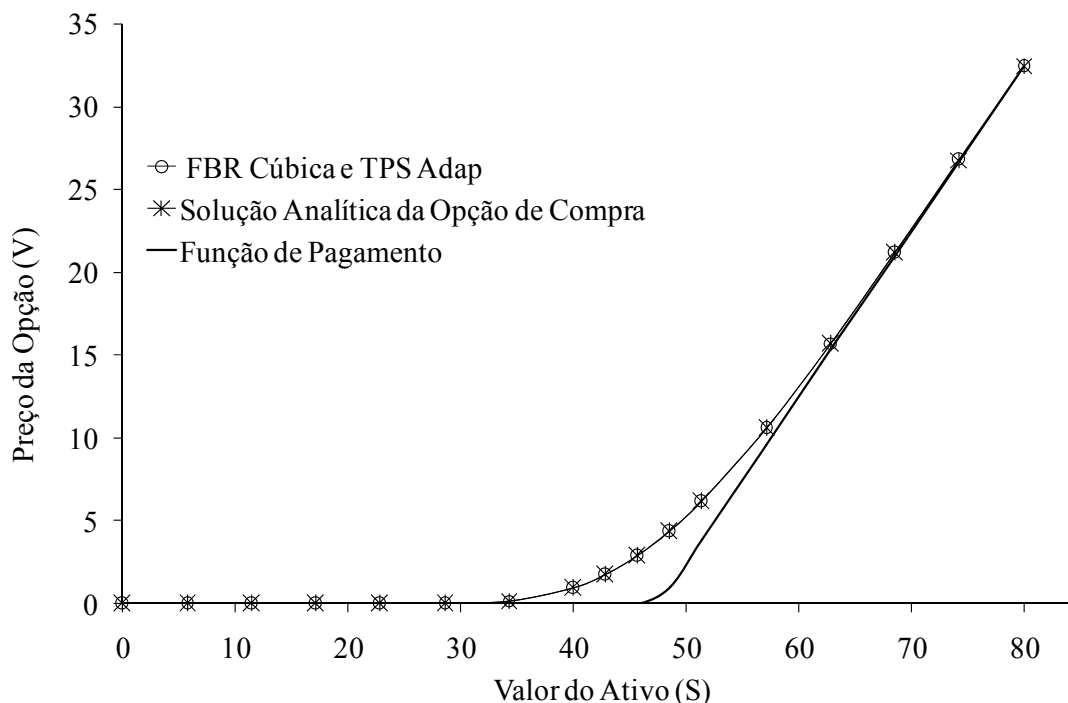
Figura 3.3. Valores simulados da FBR Cúbica e TPS adaptativa de uma opção de compra comparados aos valores da solução analítica e da função de pagamento; E = 50 , T = 1 , \sigma = 20\% , r = 5\% .
