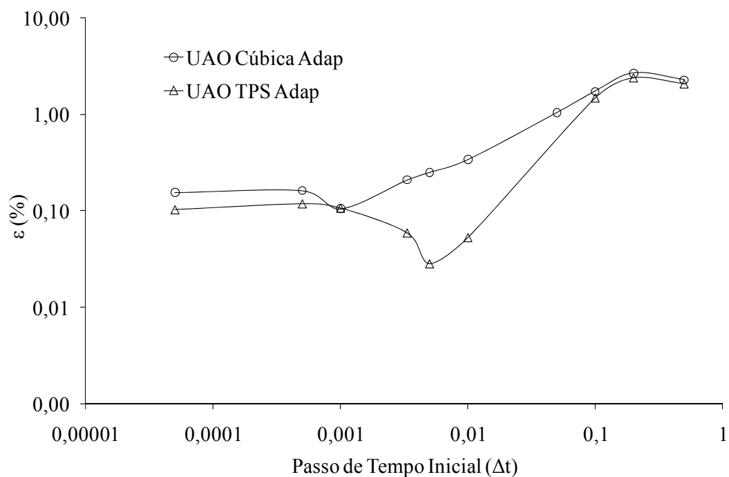
Figura 3.13. Erro relativo de preços preditos de opção de barreira Up-and-Out FBR em função do passo de tempo inicial; E = 50 , T = 1 , \sigma = 20\% , r = 5\% , N = 100 , S_{max} = 250 , \theta = 1 , \varepsilon = 1 \times 10^{-4} para FBR Cúbica adaptativa e FBR TPS adaptativa.
