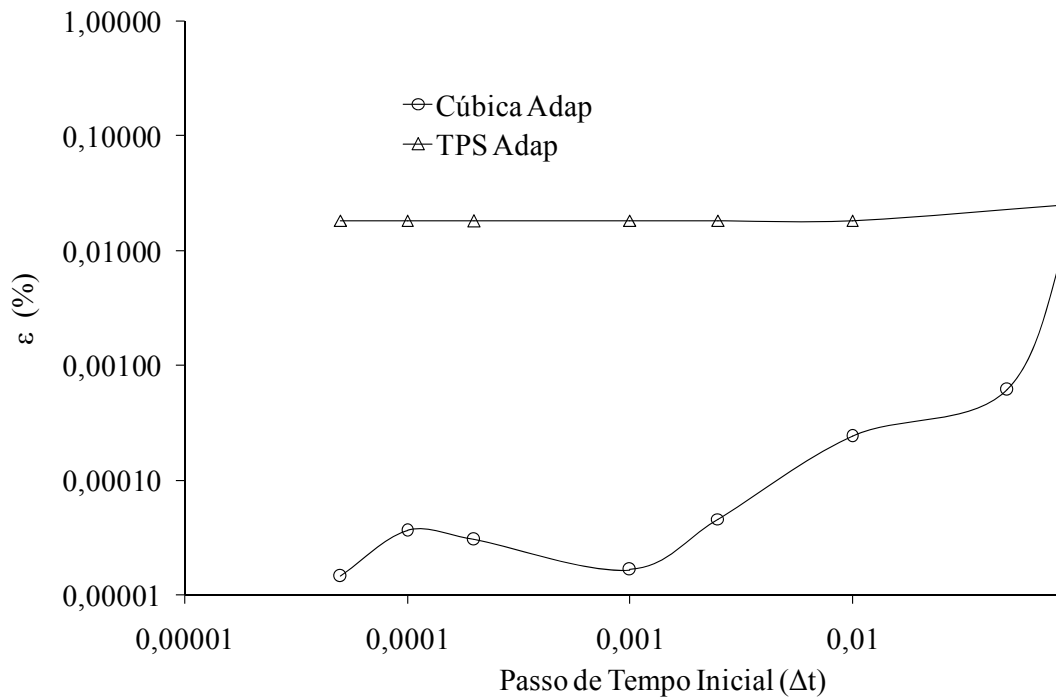
Figura 3.8. Erro relativo de valores preditos de opção de compra FBR em função do passo de tempo inicial; E = 50 , T = 1 , \sigma = 20\% , r = 5\% , N = 112 , S_{max} = 80 , \theta = 0,5 , \epsilon\epsilon = 1 \times 10^{-7} para FBR Cúbica adaptativa e FBR TPS adaptativa.
