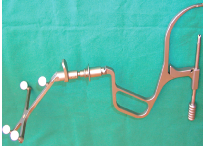
Figura 10: Guia tibial acoplado ao corpo passivo móvel.
