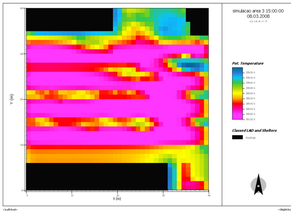
Figura 63 – Simulação da área 3 – 15 h
