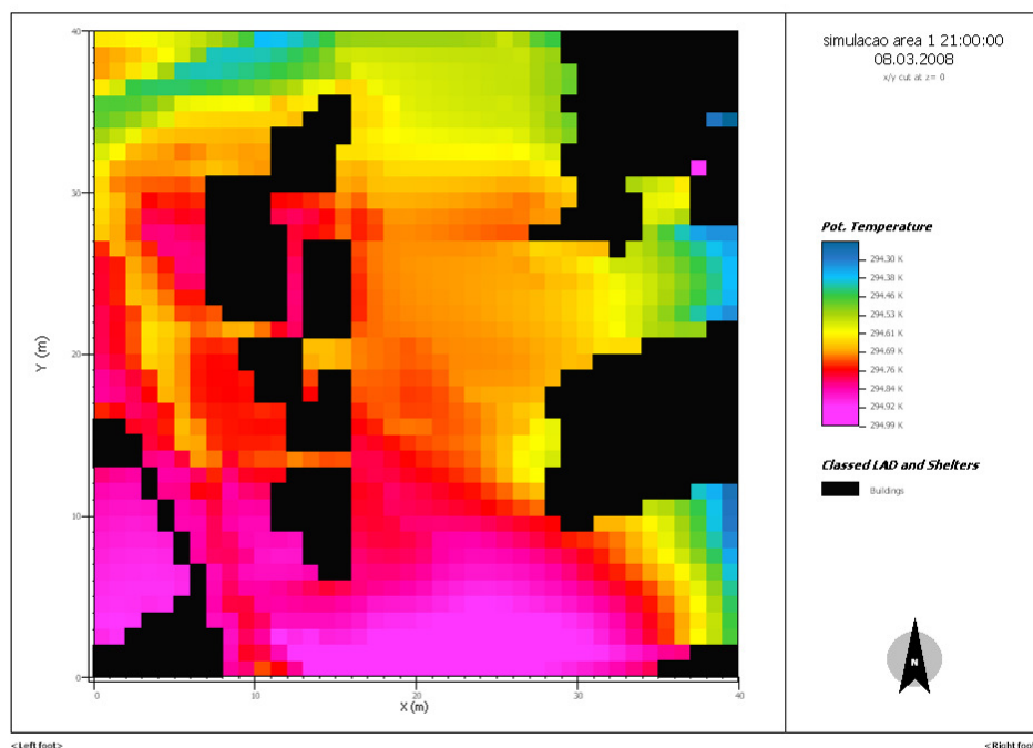
Figura 65 – Simulação da área 1 – 21 h
