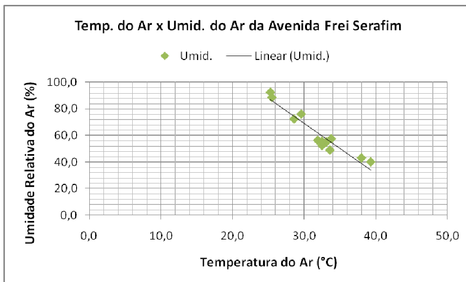
Gráfico 31 – Relação de proporção inversa entre temperatura do ar e umidade do ar na área 2
