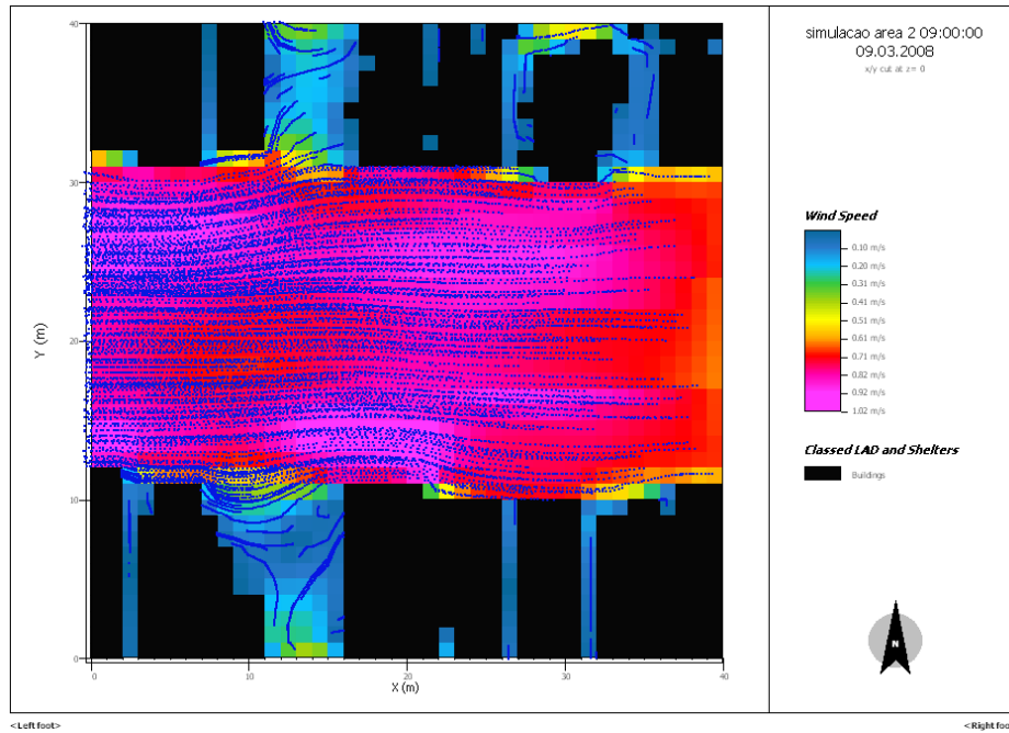
Figura 70 – Simulação de ventilação na área 2 – 9 h
