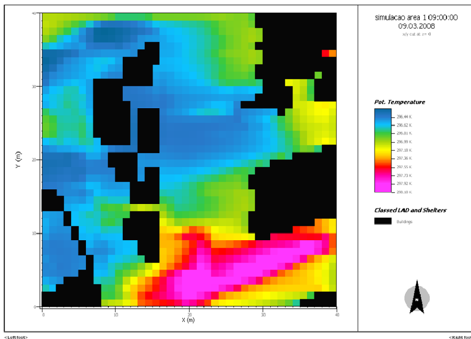
Figura 57 – Simulação da Área 1 – 9h
