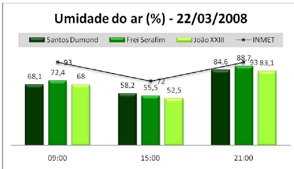
Gráfico 16 – Umidade do ar (%) em 22/03/2008
