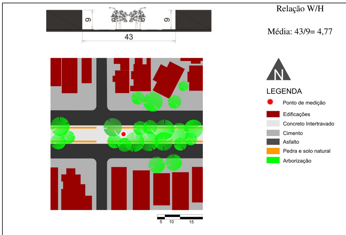
Figura 30 - Ponto 2 – Avenida Frei Serafim – Corte e Planta esquemáticos
