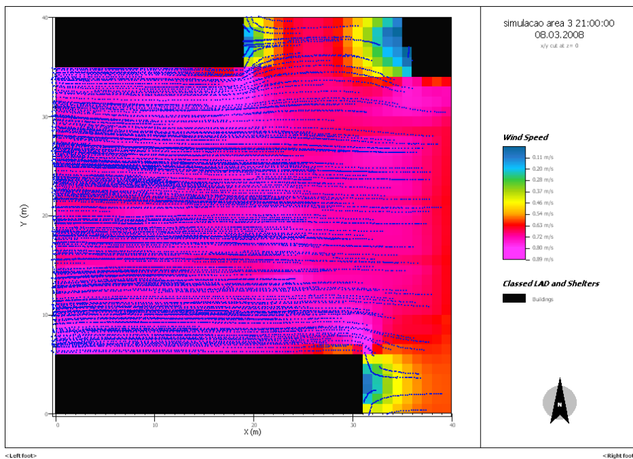
Figura 79 – Simulação da ventilação na área 3 – 21 h
