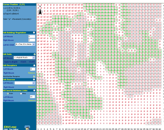
Figura 44 – Entrada de dados no ENVI-met da área 1 – Revestimento do Solo
