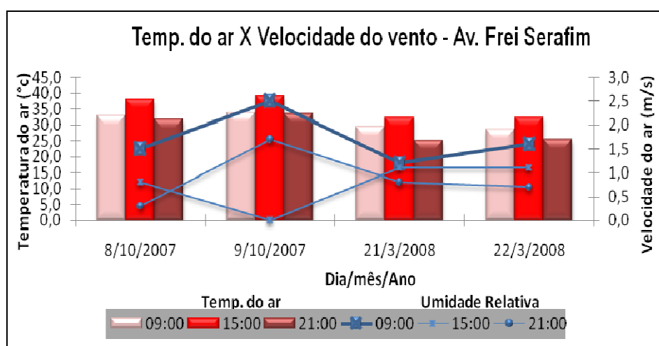
Gráfico 34 – Inter-relação entre temperatura do ar e velocidade do vento na área 2
