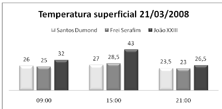
Gráfico 23 – Temperatura superficial (°C) em 21/03/2008
