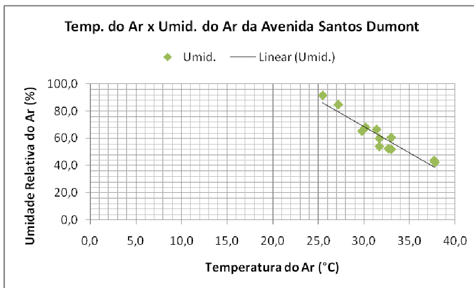
Gráfico 25 – Relação de proporção inversa entre temperatura do ar e umidade do ar na área 1
