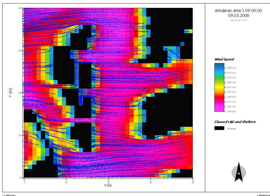
Figura 69 – Simulação de ventilação na área 1 – 9 h
