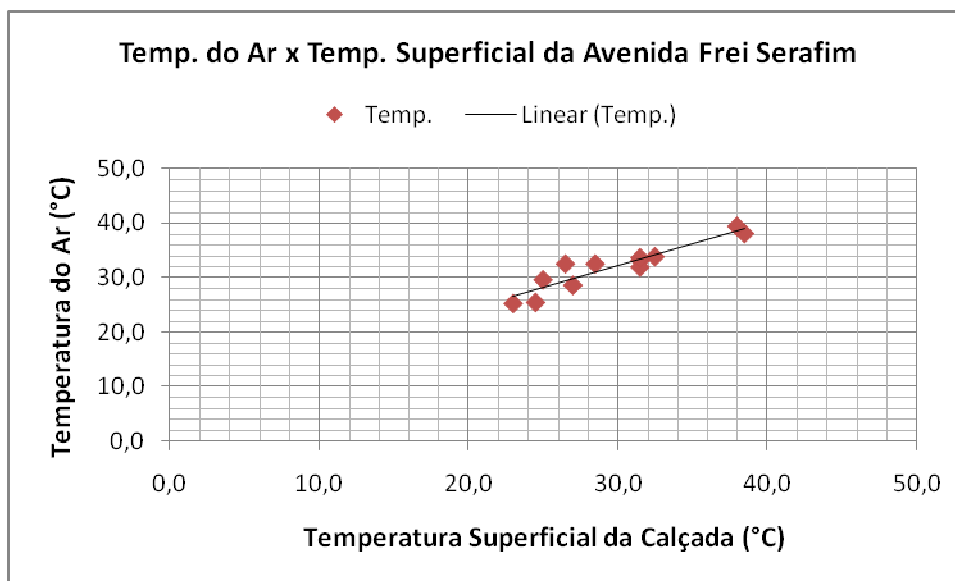
Gráfico 35 – Relação de proporção direta entre temperatura do ar e temperatura superficial na área 2
