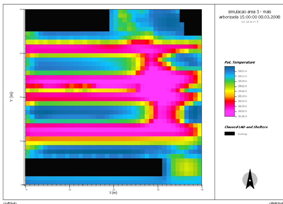
Figura 64 - Simulação da área 3 – hipotética – 15 h
