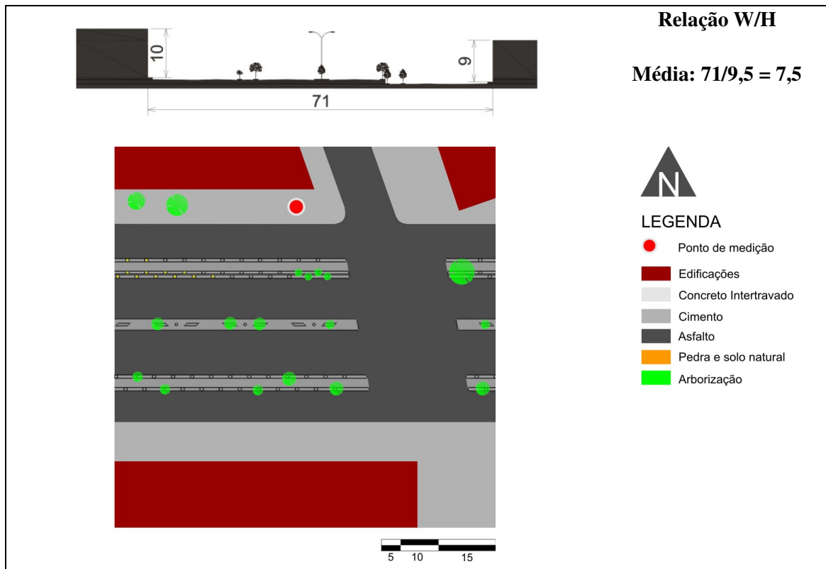
Figura 34 - Ponto 3 – Avenida João XXIII – Corte e Planta esquemáticos
