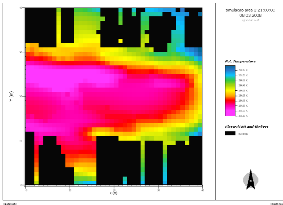
Figura 66 – Simulação da área 2 – 21 h
