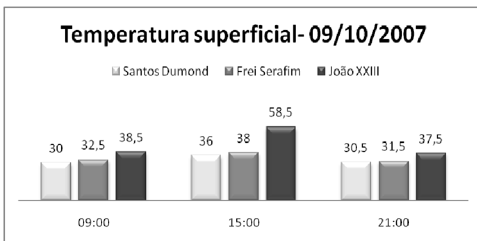
Gráfico 22 – Temperatura superficial (°C) em 09/10/2007
