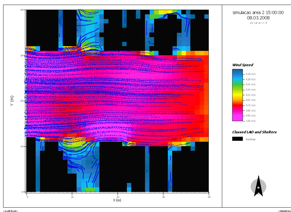
Figura 74 – Simulação da ventilação na área 2 – 15 h
