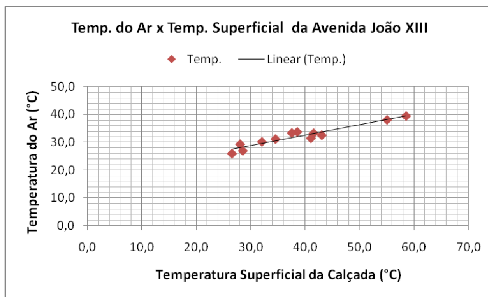
Gráfico 41 – Relação de proporção direta entre temperatura do ar e temperatura superficial na área 3
