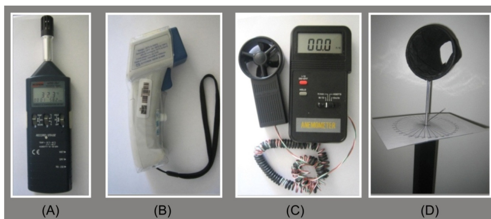
Figura 37: Aparelhos portáteis utilizados nas medições in loco . a: termohigrômetro; b: termômetro infravermelho; c: anemômetro; d: biruta.
