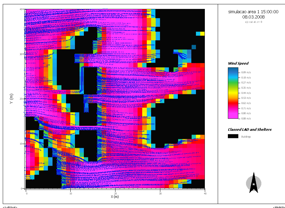
Figura 73 – Simulação da ventilação na área 1 – 15 h
