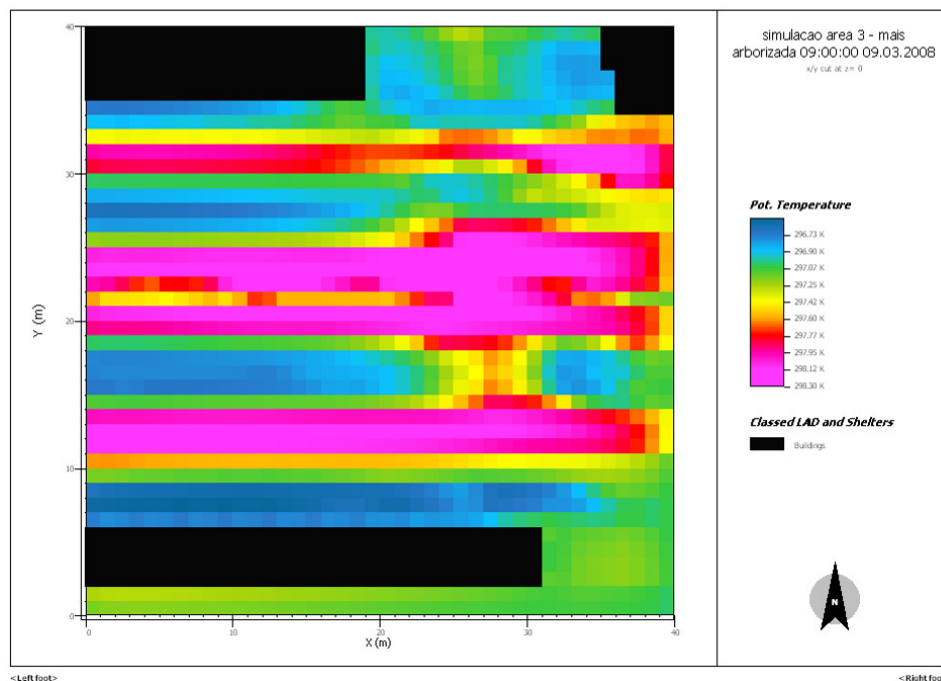
Figura 60 – Simulação da Área 3 (hipotética) – 9 h
