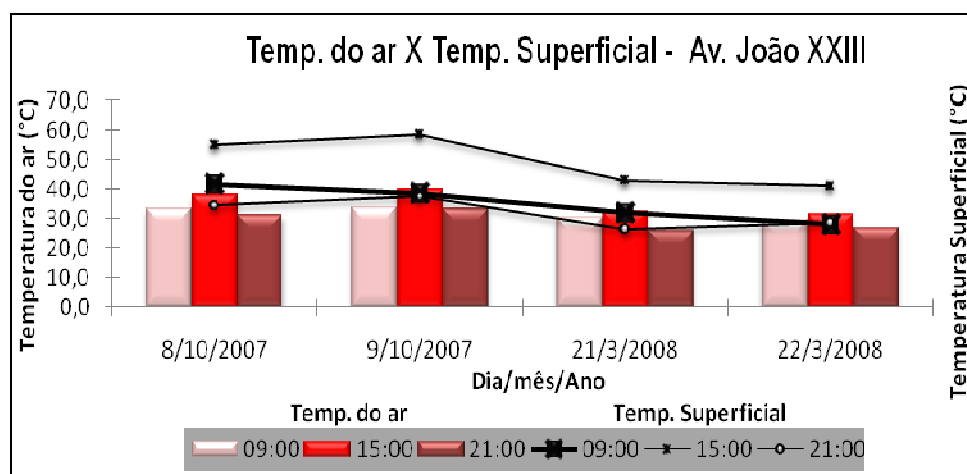
Gráfico 42 – Inter-relação entre temperatura do ar e temperatura superficial na área 3
