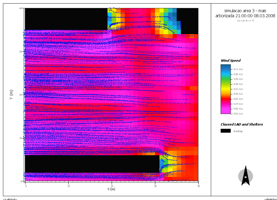
Figura 80 – Simulação da ventilação na área 3 - hipotética – 21 h
