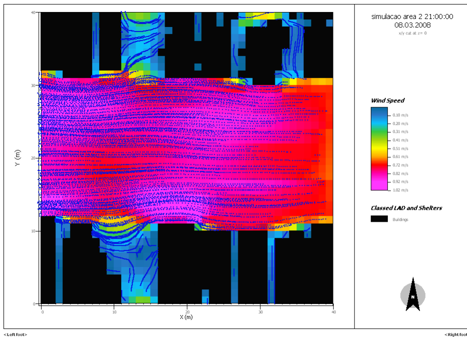
Figura 78 – Simulação da ventilação na área 2 – 21 h
