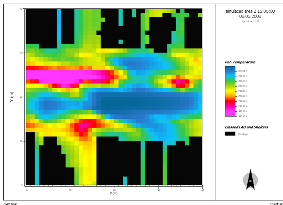
Figura 62 – Simulação da área 2 – 15h
