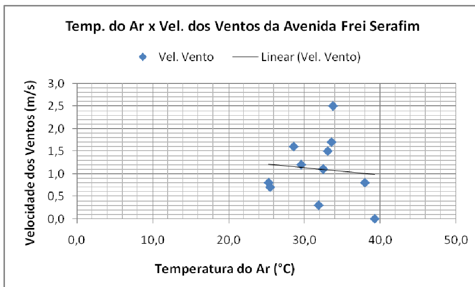
Gráfico 33 – Inter-relação entre temperatura do ar e velocidade do vento na área 2
