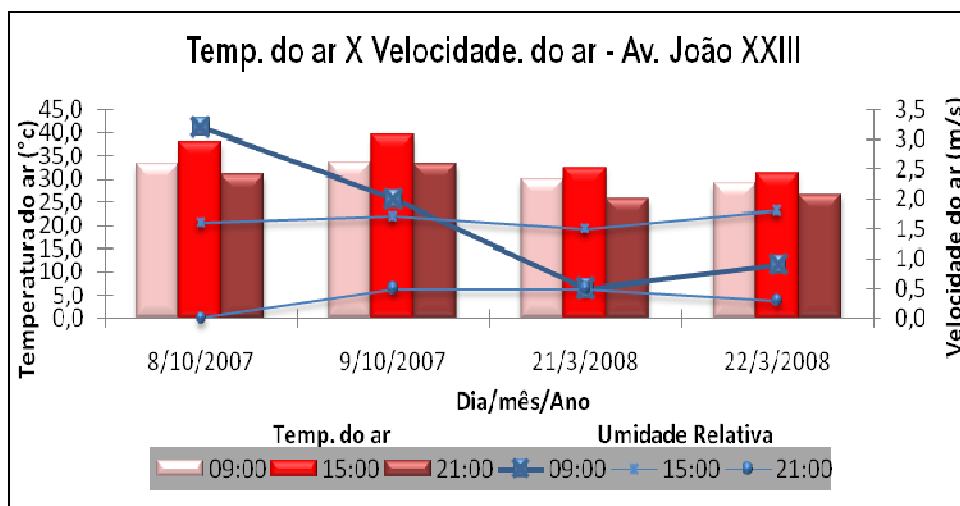
Gráfico 40 – Inter-relação entre temperatura do ar e velocidade do vento na área 3
