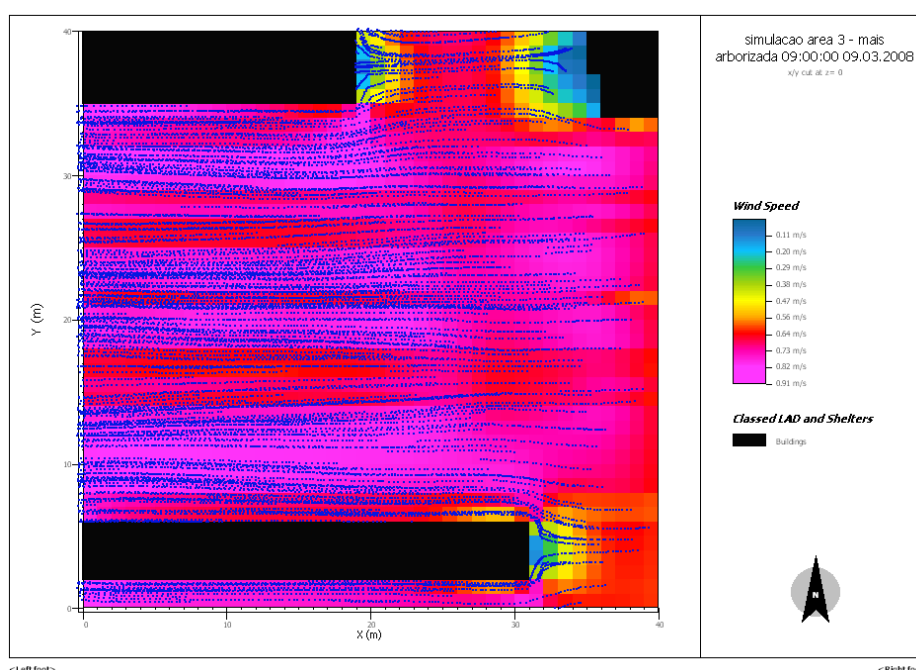
Figura 72 – Simulação da ventilação na área 3 – hipotética – 9 h
