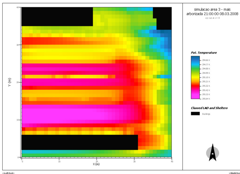
Figura 68 – Simulação da área 3 - hipotética – 21 h
