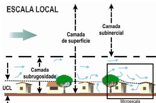
Figura 4 – Escala Local. Adaptado de Oke (2004, p.3) apud Kallas (2008)
