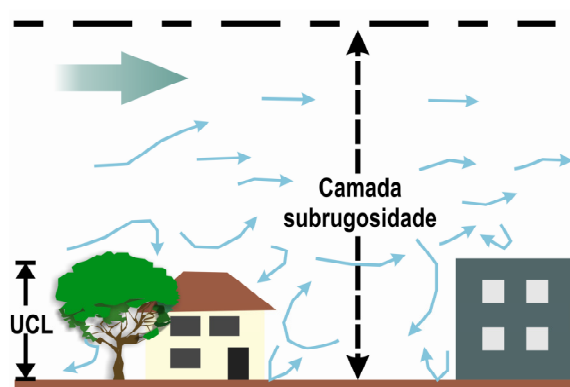
Figura 5 – Microescala. Adaptado de Oke (2004, p.3) apud Kallas (2008)
