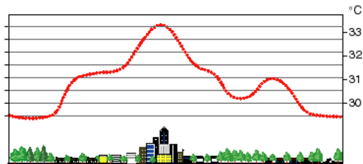
Figura 3 – Mesoescala, a camada limite urbana. Adaptado de Oke (2004) apud Kallas (2008)
