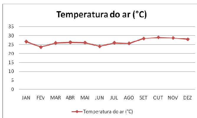
Gráfico 1 – Temperatura média do ar em Teresina (PI) período de 1961-1990
