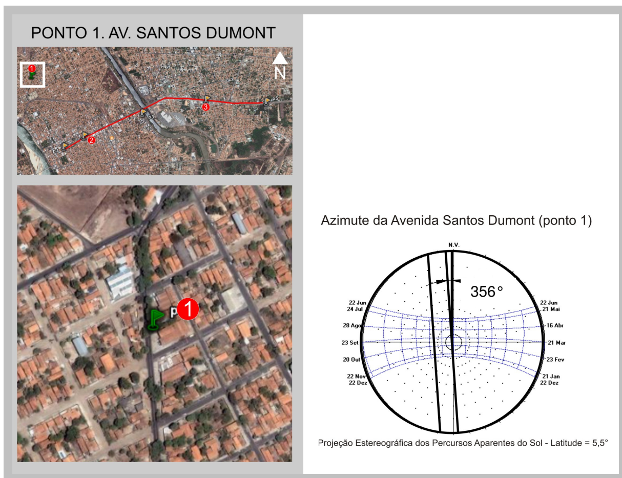
Figura 18 – Localização e Azimute da Área 1
