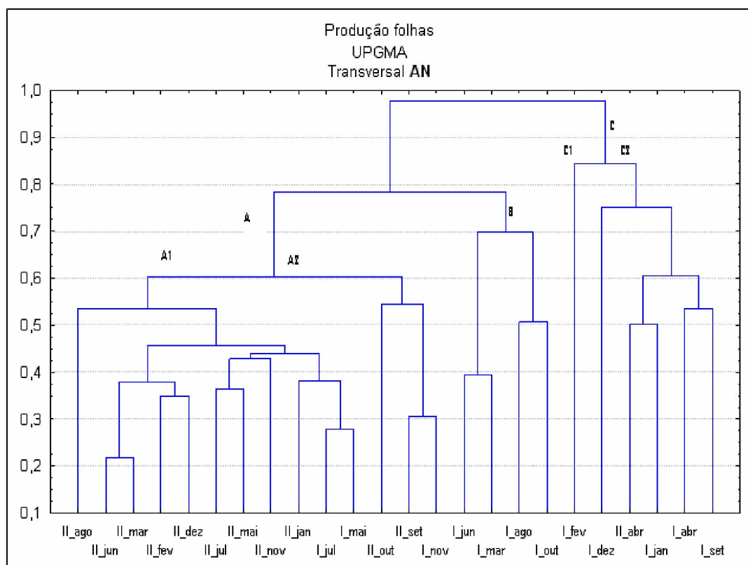
Figura 22: Análise de agrupamento para a produção de folhas na transversal AN. (I) – Estação de franja (AN1) e (II) Estação de bacia (AN3).
