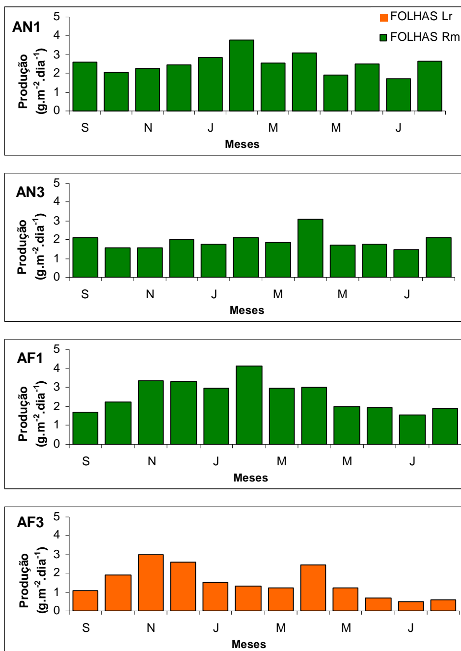
Figura 11: Produção de folhas nas quatro estações de estudo. Onde Lr – L. racemosa e Rm – R. mangle .
