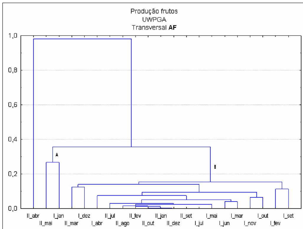
Figura 26: Análise de agrupamento para a produção de frutos na transversal AF. (I) – Estação de franja (AF1) e (II) Estação de bacia (AF3).
