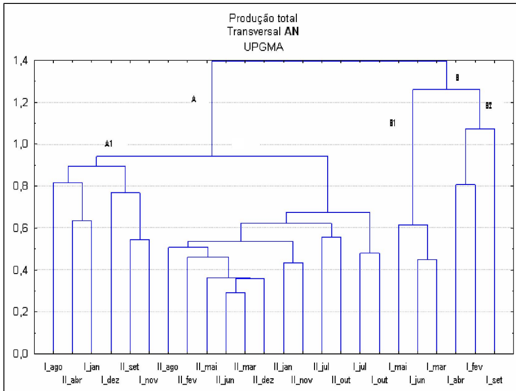
Figura 21: Análise de agrupamento para a produção total de serapilheira na transversal AN. (I) – Estação de franja (AN1) e (II) Estação de bacia (AN3).
