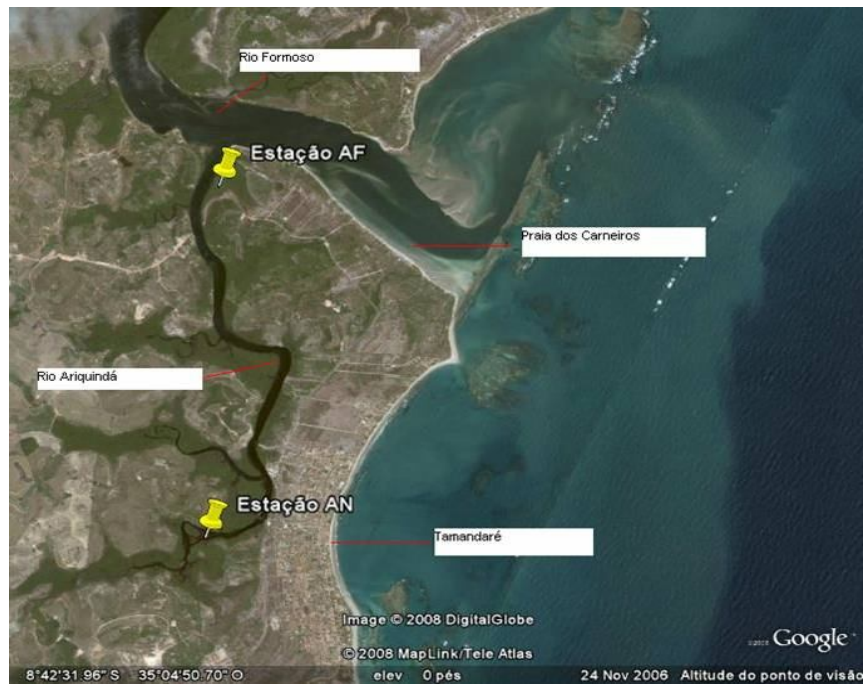
Figura 03: Figura esquemática da localização das estações de estudo (Fonte: Google Earth).
