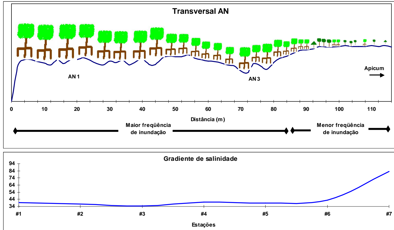
Figura 07: Desenho esquemático do perfil topográfico e da zonação do bosque de mangue da estação AN, mostrando as estações e os pontos de coleta de salinidade (Modificado de Nascimento-Filho, 2007).
