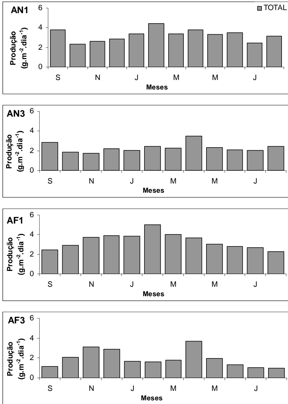
Figura 10: Produção total de serapilheira nas quatro estações de estudo.
