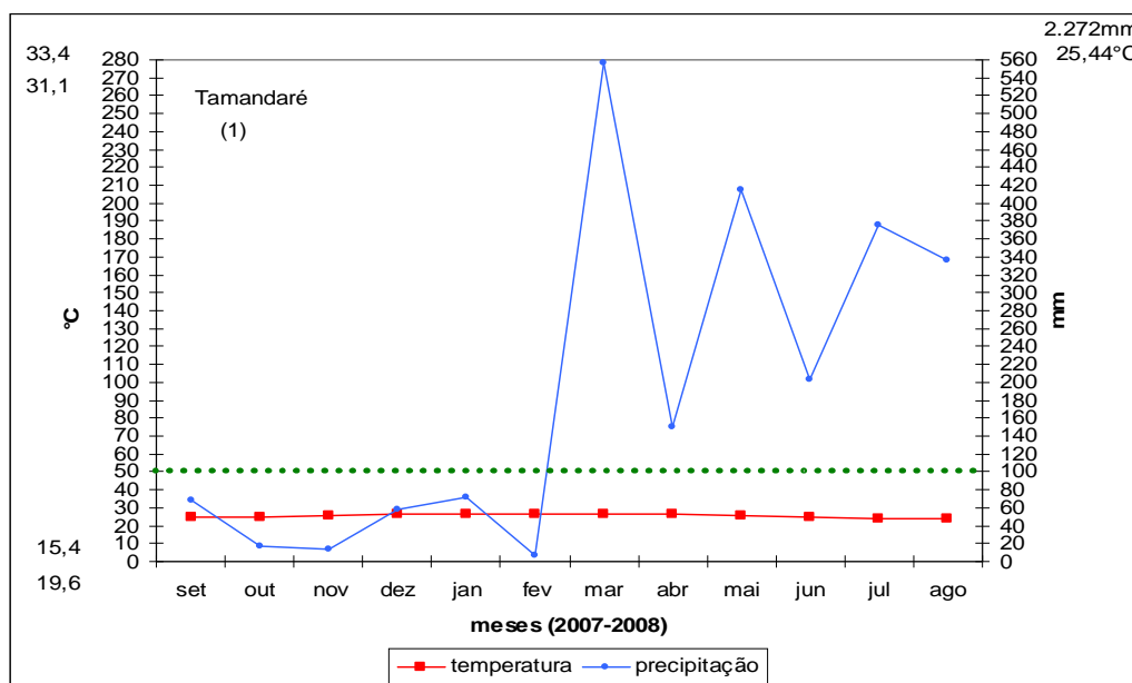
Figura 20: Diagrama climático da região de Tamandaré-PE no período de setembro de 2007 a agosto de 2008. Dados obtidos na estação meteorológica de Barreiros (Fonte: ITEP/LAMEPE).
