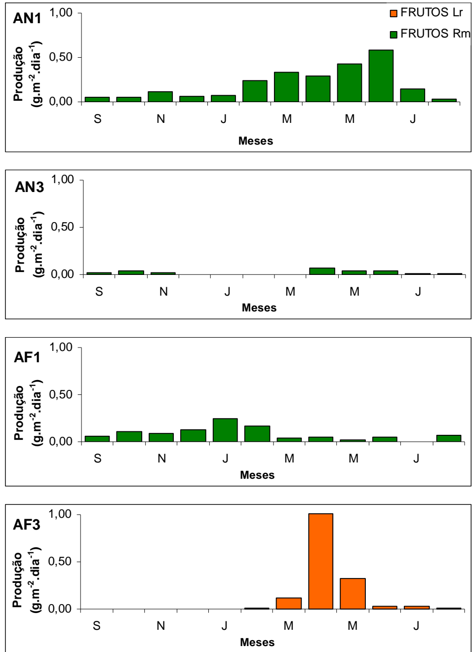
Figura 13: Produção de frutos nas quatro estações de estudo. Onde Lr – L. racemosa e Rm – R. mangle .
