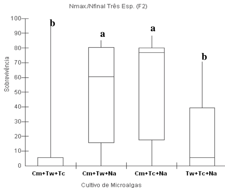
Figura 40: Taxa de sobrevivência dos indivíduos cultivados de Pseudodiaptomus acutus , alimentados com uma mistura de três espécies de microalga Cm ( Chaetoceros muelleri ) + Tw ( Thalassiosira weissflogii ) + Tc ( Tetraselmis chuii ), Cm ( Chaetoceros muelleri ) + Tw ( Thalassiosira weissflogii ) + Nanno ( Nannochloropsis sp. chloropsis sp. ), Cm ( Chaetoceros muelleri ) + Tc ( Tetraselmis chuii ) + Nanno. ( Nannochloropsis sp. ) e Tw ( Thalassiosira weissflogii ) + Tc ( Tetraselmis chuii ) + Nanno ( Nannochloropsis sp. ) cultivada em meio F2. As letras iguais mostraram similaridade estatística com os testes utilizados.
