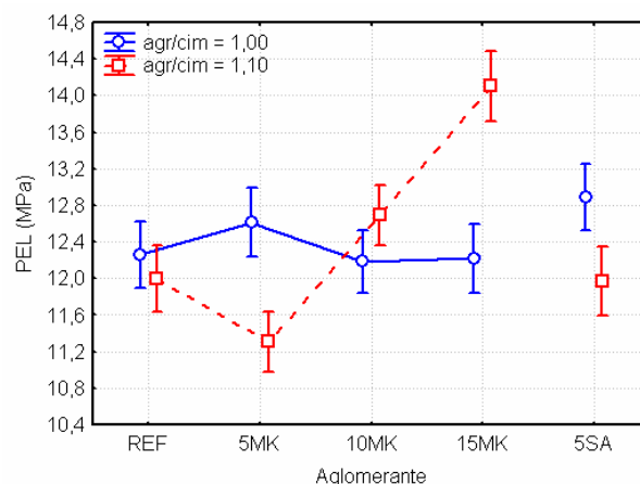
Figura 5.11: efeito da interação entre agregado/cimento e tipo de aglomerante sobre o PEL
