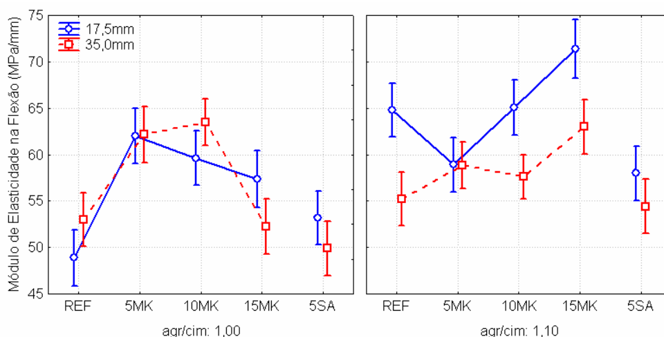
Figura 5.41: efeito conjunto do tamanho das fibras, aglomerante e relação agregado/cimento sobre o MEF
