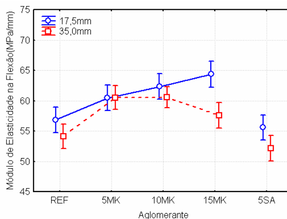
Figura 5.39: efeito conjunto do tamanho das fibras e tipo de aglomerante sobre o MEF
