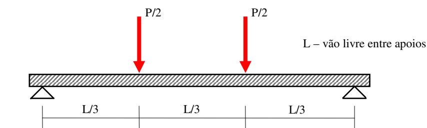
Figura 4.8: representação esquemática do ensaio de flexão
