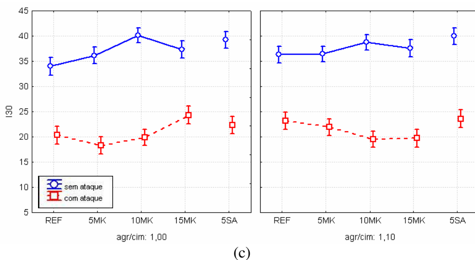
Figura 5.29: efeito da interação entre relação agregado/cimento, aglomerante e ataque sobre os índices de tenacidade. (a) I5, (b) I10 e (c) I30
