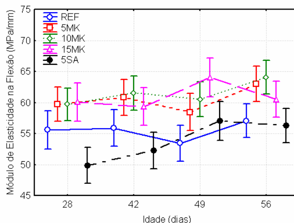
Figura 5.34: efeito da interação entre aglomerante e idade sobre o MEF
