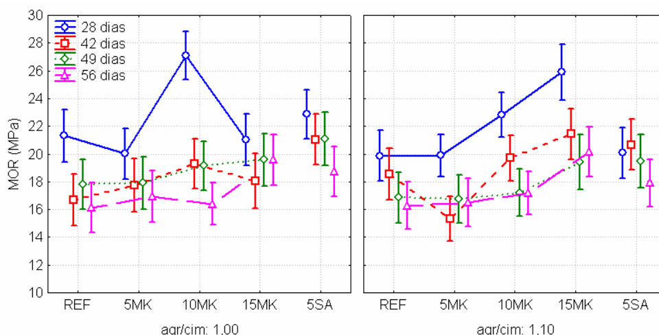
Figura 5.20: efeito da interação entre aglomerante, agregado/cimento e idade sobre o MOR
