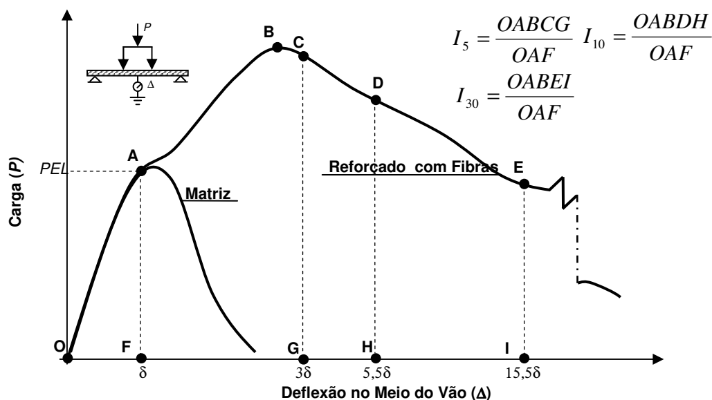
Figura 4.13: determinação dos índices de tenacidade da ASTM C1018 (ACI COMMITTEE 544, 1999)
