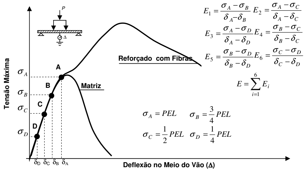
Figura 4.14: determinação do módulo de elasticidade na flexão
