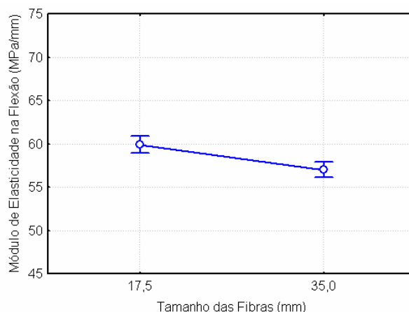
Figura 5.38: efeito isolado do tamanho das fibras sobre o MEF
