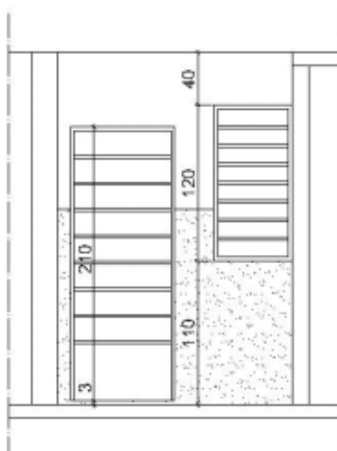
FIGURA 5.3 – Corte BB, projeto original.
