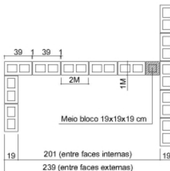
FIGURA: Modulação M=20. Medidas reais
