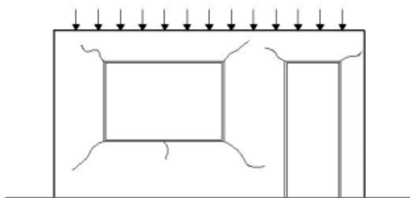
FIGURA 5.9 – Fissuração típica em parede com presença de aberturas, devido à atuação de carga uniformemente distribuída (ABCI, 1990).
