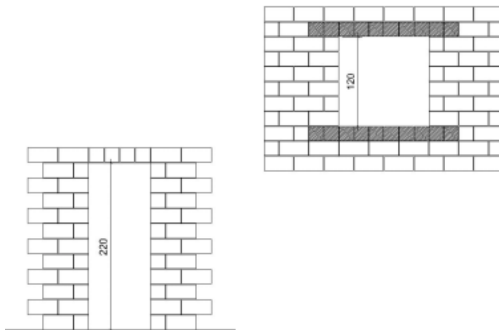
FIGURA: Aberturas de portas e janelas com módulo M=20.
