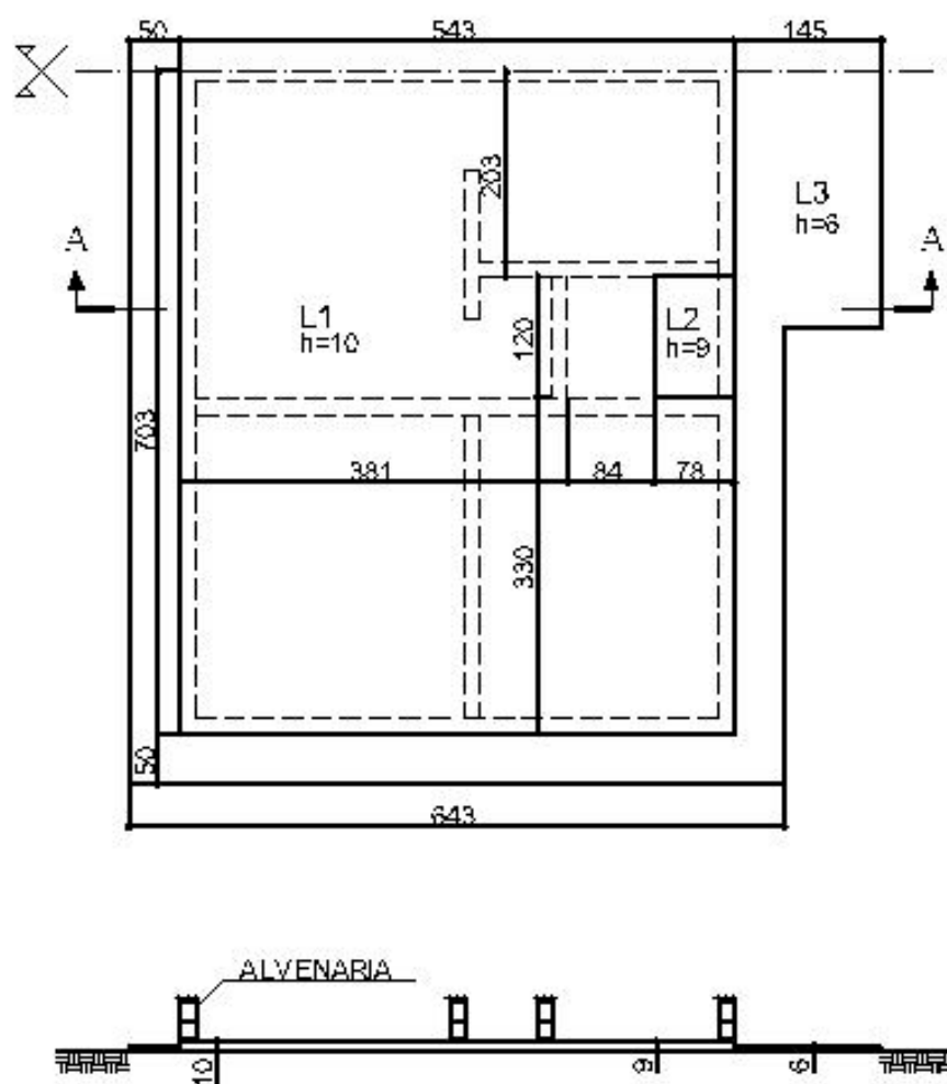
FIGURA 5.13 – Forma da laje de fundação e corte AA
