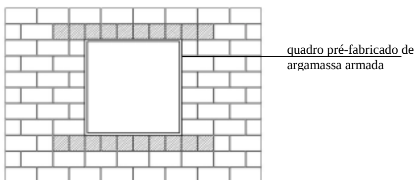
FIGURA 5.18 – Detalhe de abertura da janela empregando-se quadro pré-moldado e blocos canaletas de 9x19x19cm (PRUDÊNCIO JR et al.,2002).
