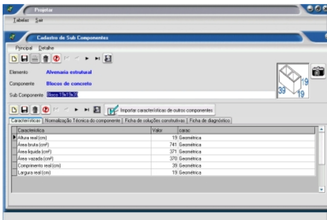
FIGURA 6.10 – Tela de cadastro de sub-componentes – características
