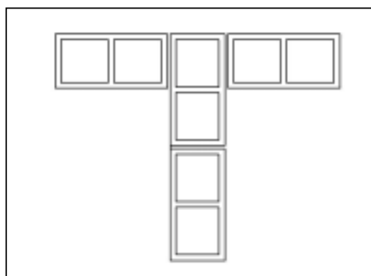
Planta 1º e 3º fiadas
