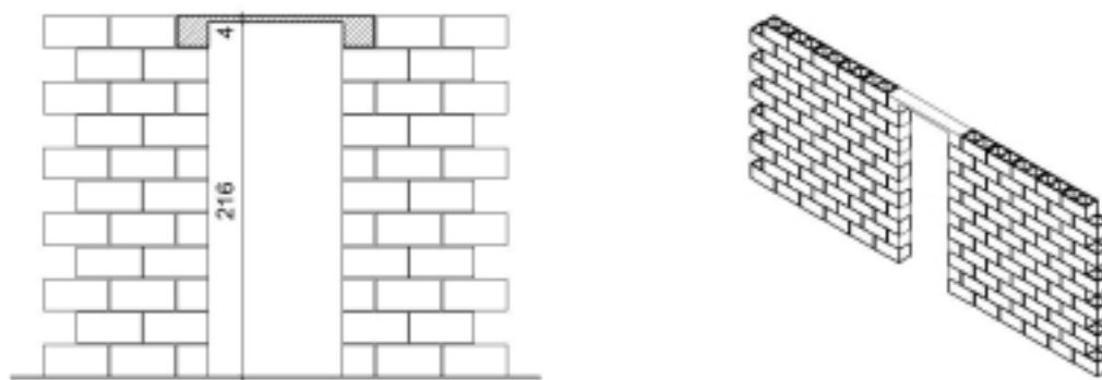
FIGURA 5.17 – Detalhe de verga pré-moldada de concreto sobre a abertura da porta (PRUDÊNCIO et al.,2002).
