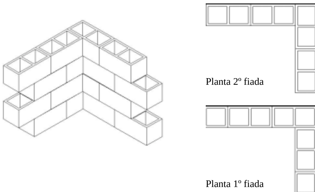
FIGURA: Detalhe típico de canto de paredes empregando-se blocos de 19x19x39cm
