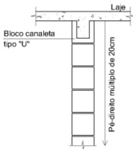
FIGURA: Detalhe das paredes externas
