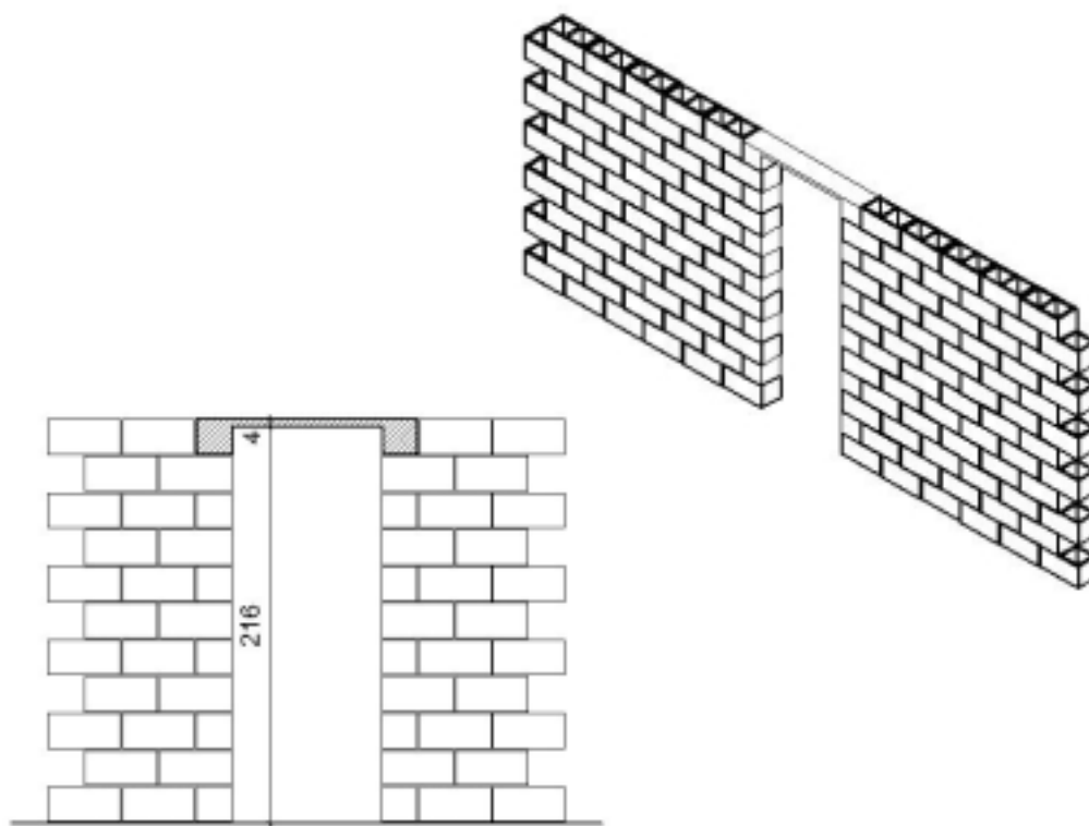
FIGURA: Detalhe de verga pré-moldada de concreto sobre a abertura da porta.
