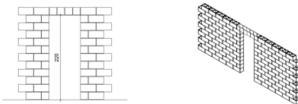
FIGURA 5.16 – Detalhe de verga com blocos canaleta de 9x19x19cm (PRUDÊNCIO et al., 2002).
