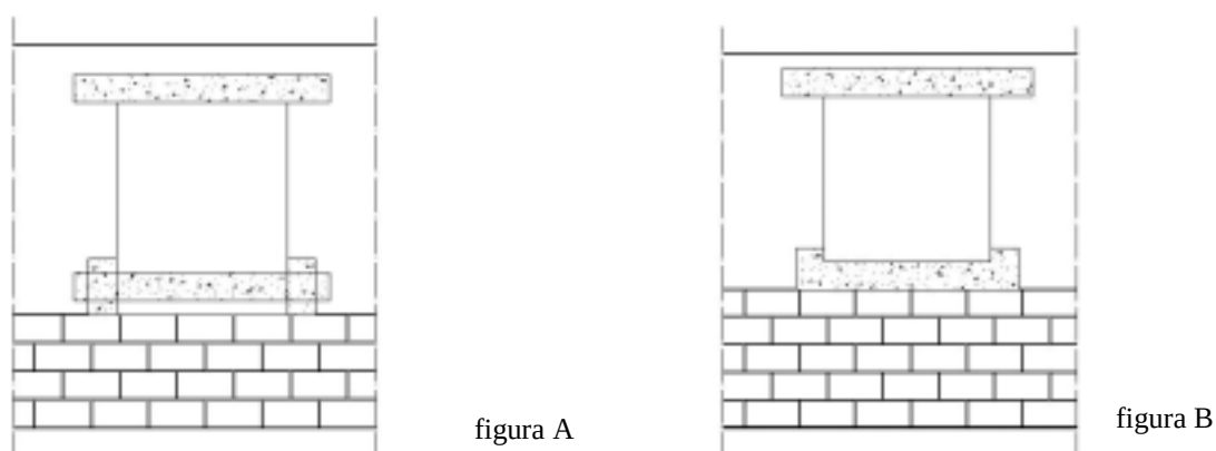
FIGURA 5.11 – A figura A mostra como a verga e contraverga foram projetadas, e a figura B mostra como foram executadas.
