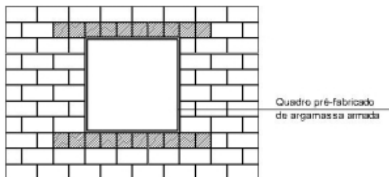
FIGURA: Detalhe de verga e contraverga empregando-se blocos canaletas
