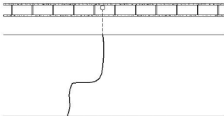
FIGURA 5.2 – Fissura provocada pela retração da alvenaria, em seção enfraquecida pela presença de tubulação
