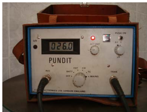
Figura 31: realização da aferição do ultra-som a) aferição do equipamento; b) leitura do tempo
