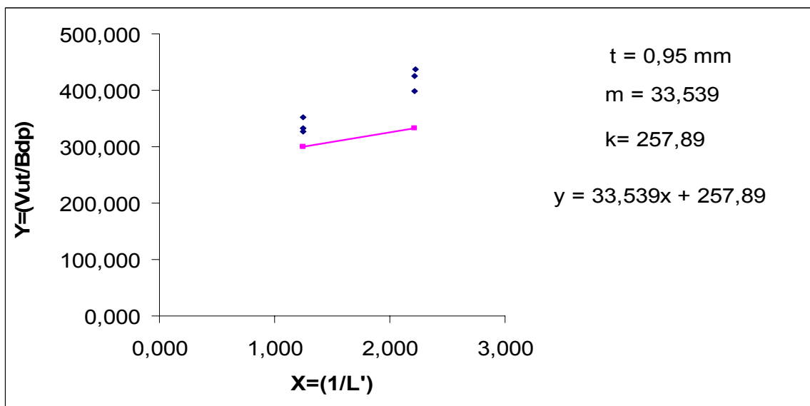
FIGURA 4.2 - Resistência nominal característica ao cisalhamento longitudinal (modelos com t = 0,95 \text{ mm} )
