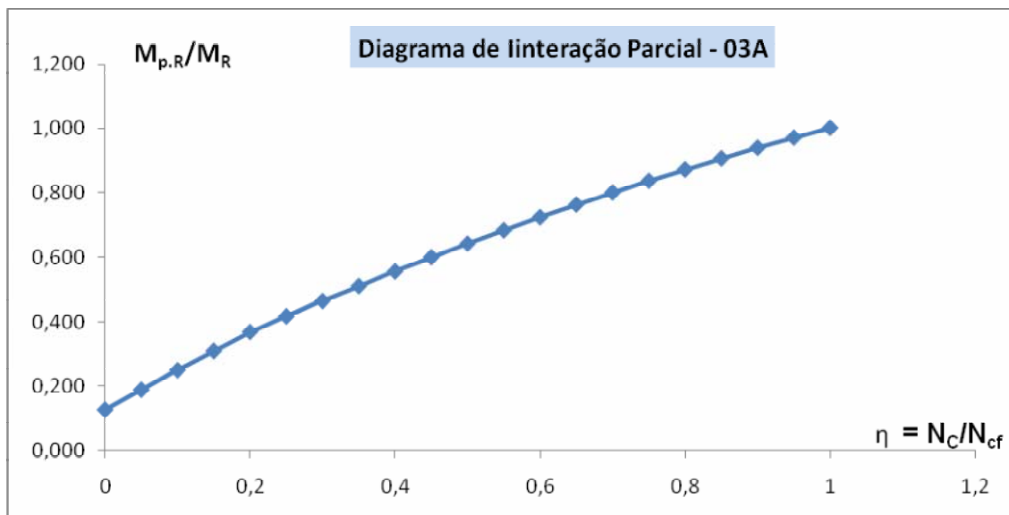
FIGURA 5.8-Diagrama de resistência para a determinação do grau de interação do modelo 03A
