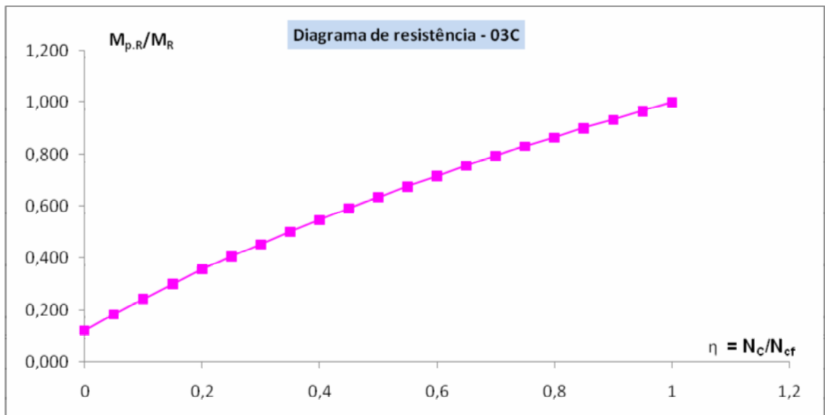
FIGURA B.9 - Diagrama de resistência-modelo 03C
