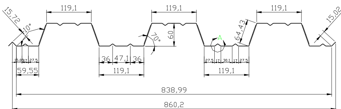
FIGURA 2.1 - Seção transversal típica do perfil do DECK 60
