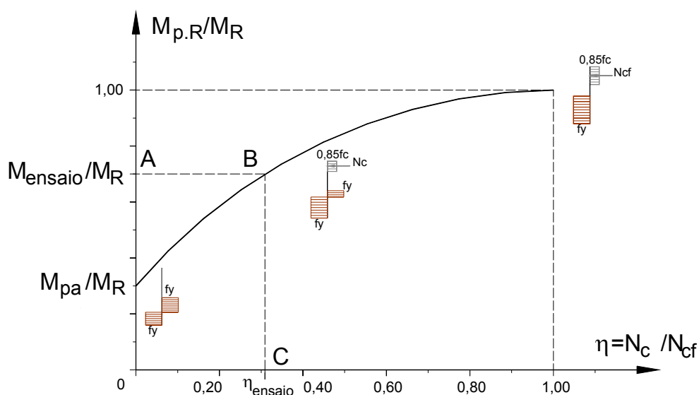
FIGURA 5.6 - Diagrama de resistência para a determinação do grau de interação – adaptado de SOUZA NETO (2001)
