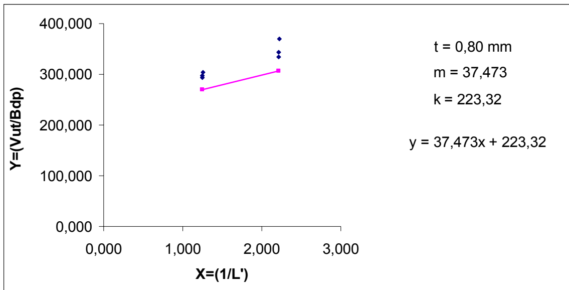
FIGURA 4.1 - Resistência nominal característica ao cisalhamento longitudinal (modelos com t = 0,80\text{mm} )
