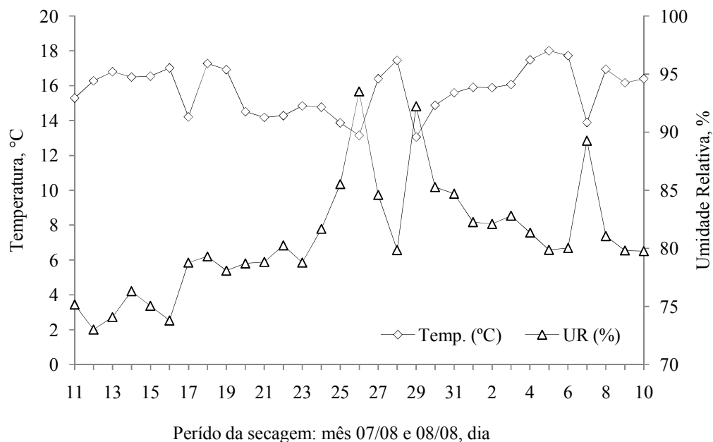
Figura 7 – Valores médios de temperatura e umidade relativa ocorridos na segunda e primeira quinzena dos meses de julho e agosto de 2008, durante o processo de secagem do café em coco.
