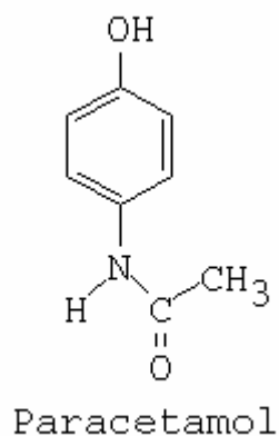
Figura 07. Estrutura molecular do paracetamol
