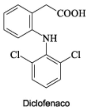
Figura 06. Estrutura molecular do diclofenaco
