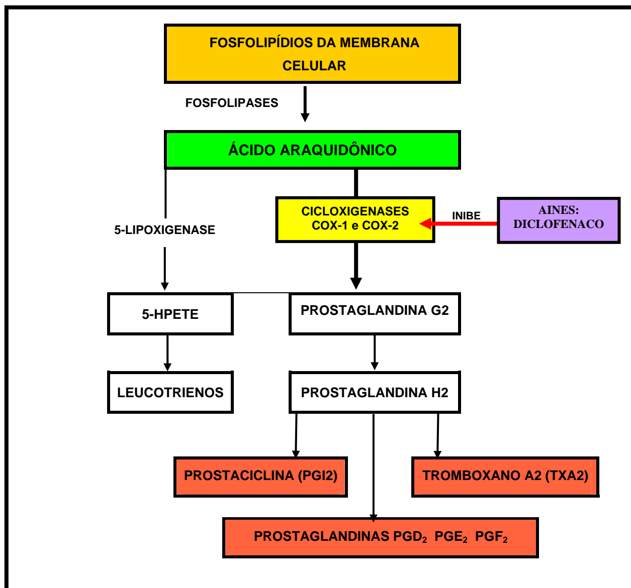
Figura 05. Cascata do ácido araquidônico. O Diclofenaco é um potente inibidor não seletivo da atividade da cicloxigenase, inibindo COX-1 e COX-2, causando redução da formação de prostaglandina, prostaciclina e tromboxano, todos mediadores da resposta inflamatória.
