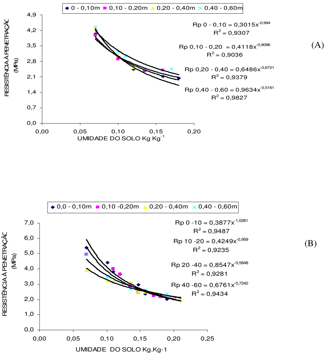
Figura 2 - Resistência à penetração (MPa) de um Latossolo Amarelo Coeso cultivado com lima ácida 'tahiti' em sistema convencional (A) linha, (B) entrelinha. Cruz das Almas, BA.
