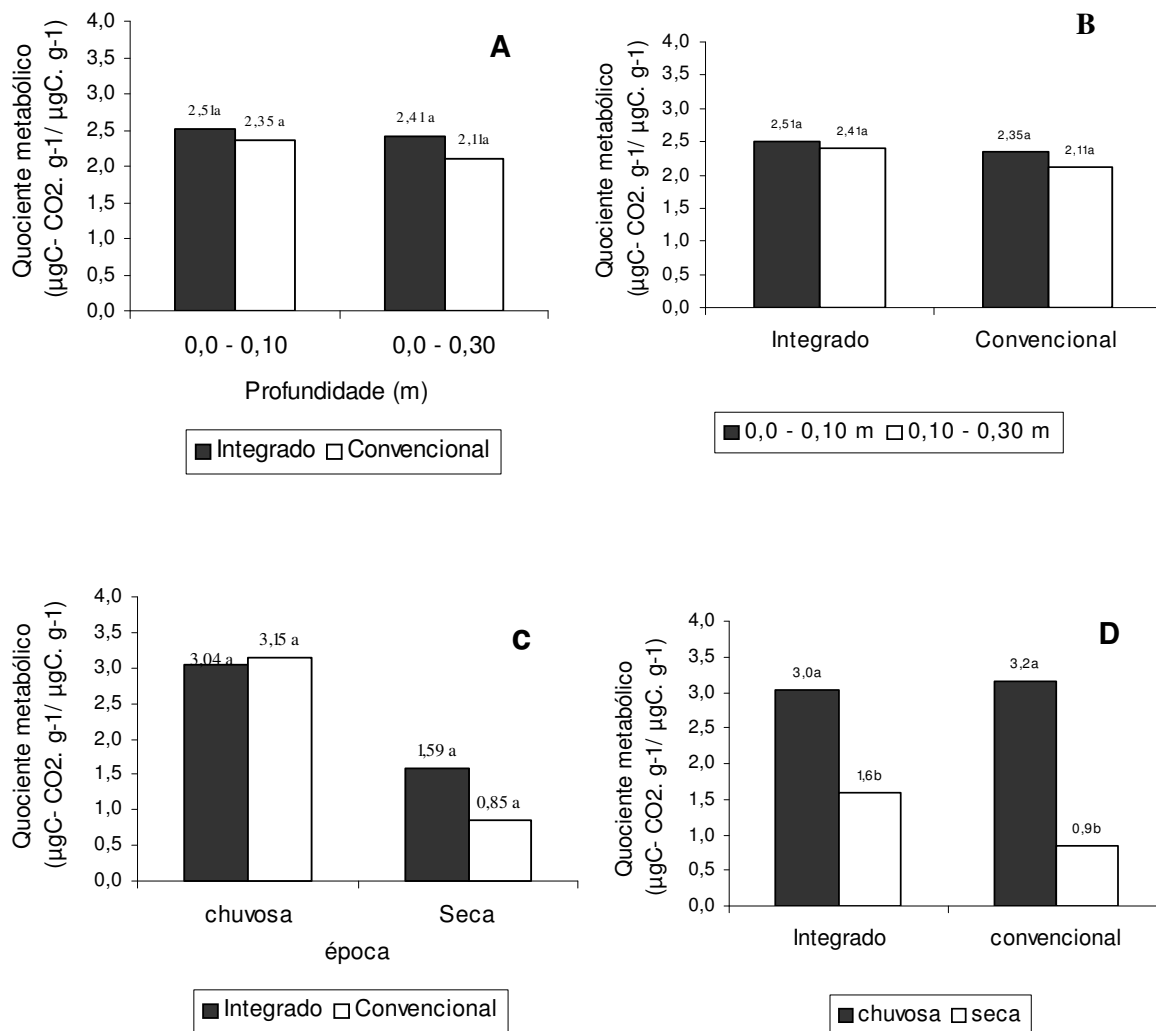
Figura 5 - Quociente metabólico ( \mu\text{g C g}^{-1}\text{h}^{-1} ) na linha de plantio de um Latossolo amarelo coeso cultivado com lima ácida “Tahiti”, submetido a dois sistemas de manejo T1e T2. em duas épocas do ano (chuvosa e seca) e duas profundidades (0-0,10 m e 0,10-0,30 m). Cruz das Almas - BA.
