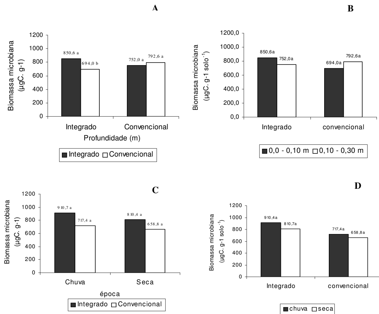
Figura 2 – Carbono da biomassa microbiana ( \mu\text{g C g}^{-1} solo seco -1 ) nas entrelinhas de plantio de um Latossolo Amarelo coeso cultivado com lima ácida “Tahiti”, submetido a dois sistemas de manejo (T1e T2) em duas épocas do ano (chuvosa e seca) e duas profundidades (0-0,10 m e 0,10-0,30 m) Cruz das Almas - BA.
