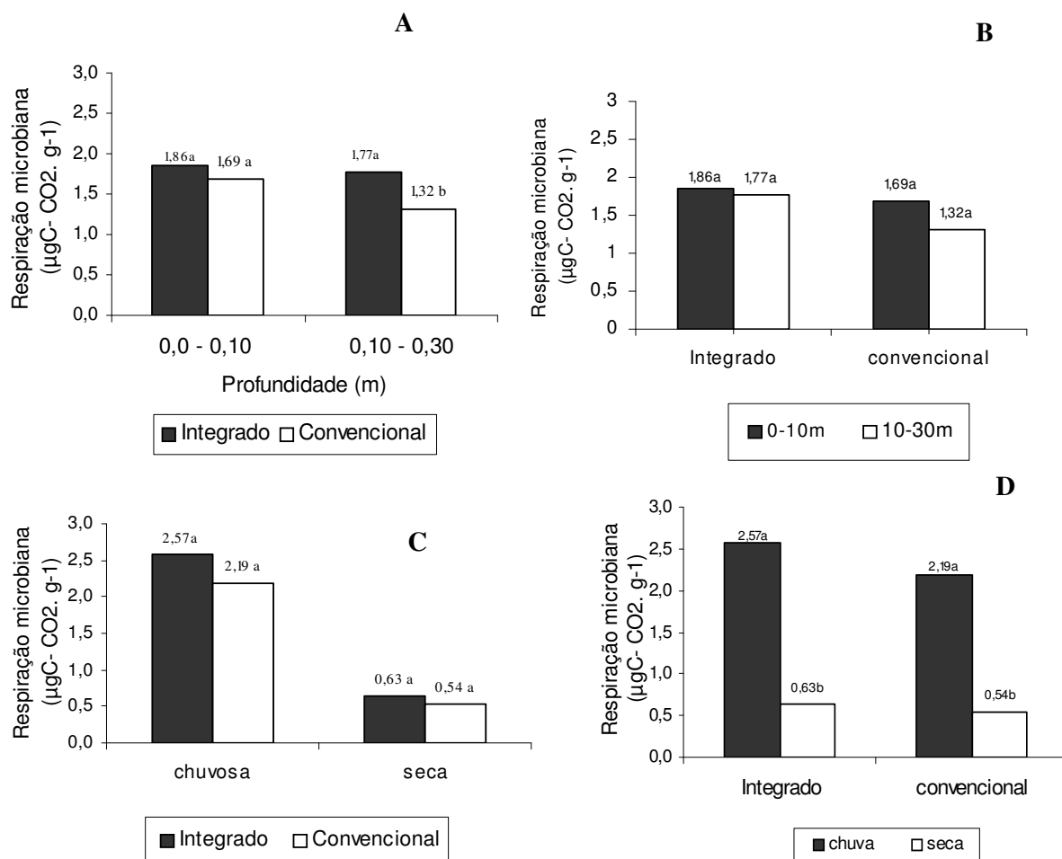
Figura 4 - Respiração microbiana ( \mu\text{g C g}^{-1} \text{ h}^{-1} ) nas entrelinhas de plantio de um latossolo amarelo coeso cultivado com lima ácida “Tahiti”, submetido a dois sistemas de manejos T1 e T2, em duas épocas do ano (chuvosa e seca) e duas profundidades (0-0,10 m e 0,10-0,30 m)), Cruz das Almas – BA.
