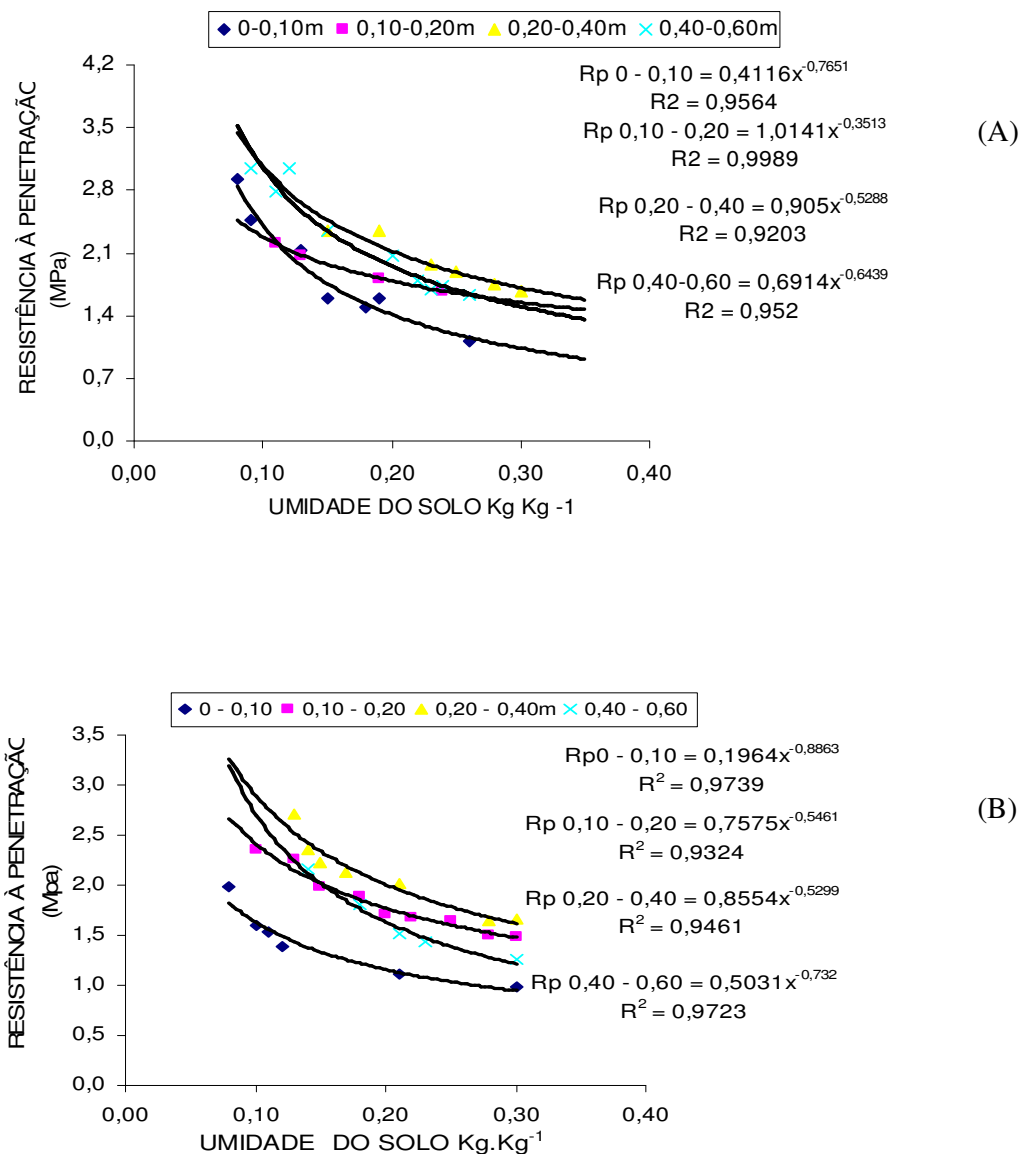
Figura 1 - Resistência à penetração (MPa) de um Latossolo Amarelo Coeso cultivado com lima ácida 'tahiti' em sistema integrado (A) linha, (B) entrelinha. Cruz das Almas, BA.
