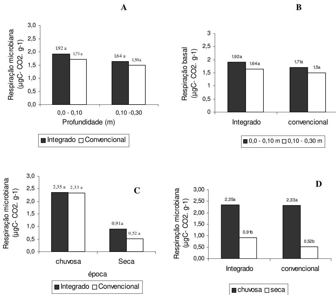
Figura 3 – Respiração microbiana ( \mu\text{g C g}^{-1} \text{ h}^{-1} ) nas linhas de plantio de um Latossolo amarelo coeso cultivado com lima ácida “Tahiti”, submetido a dois sistemas de manejo T1 e T2 em duas épocas do ano (chuvosa e seca) e duas profundidades (0-0,10 m e 0,10-0,30 m). Cruz das Almas – BA.
