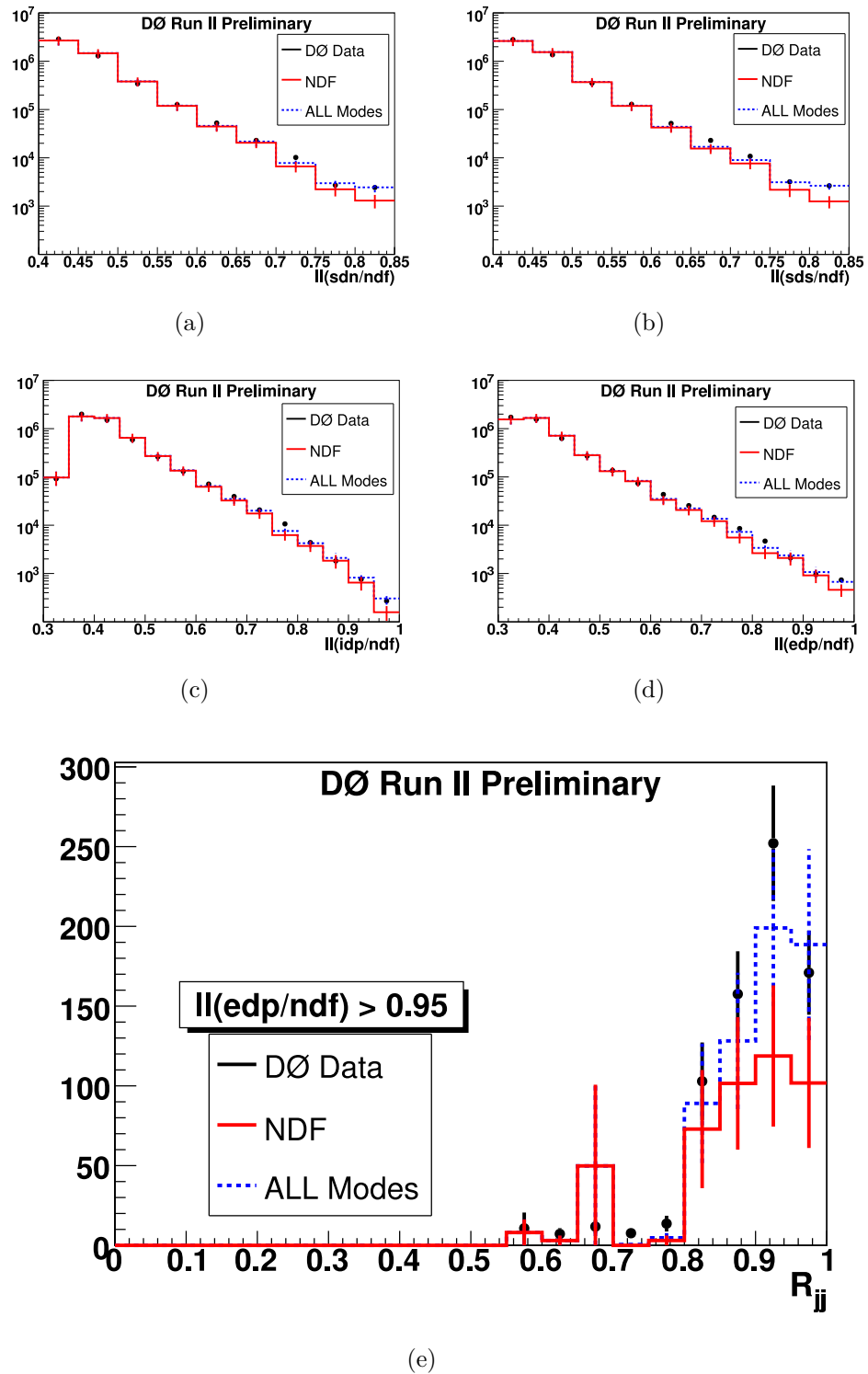
Figura 6.19: Distribuições do discriminante construído pelo método multivariável de verossimilhança para as quatro produções difrativas e a distribuição R_{ij} depois do corte ll(\text{edp}/\text{ndf}) > 0,95 .
