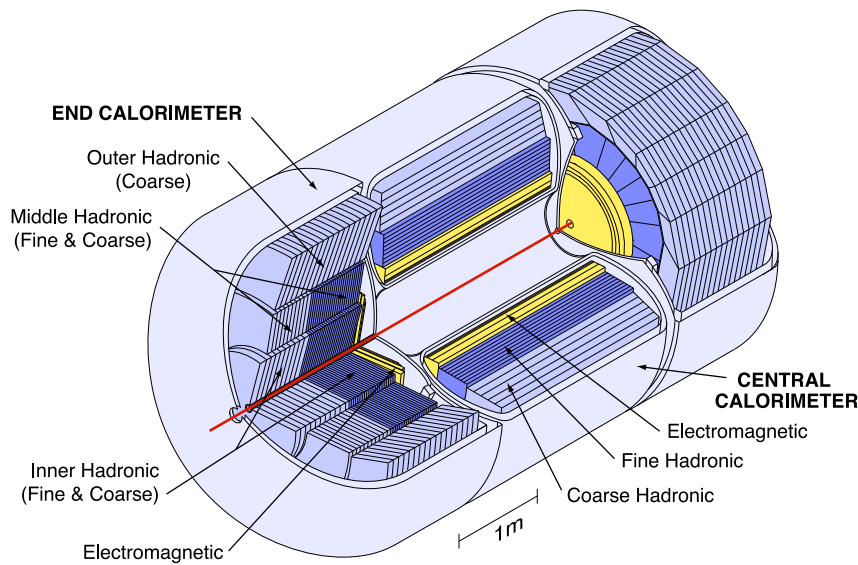
Figura 3.7: Calorímetro central e frontal ilustrados.
