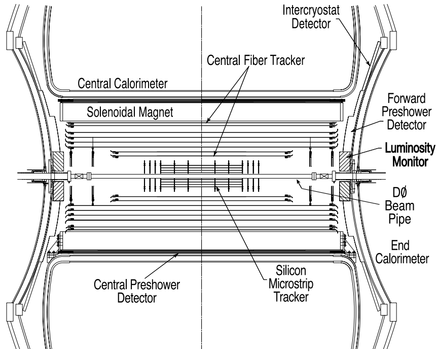
(b) Seção transversal da parte central do detector.
