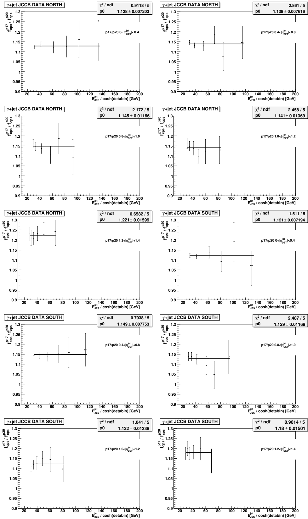
Figura A.19: Comparação da função f_{CPS} para eventos reais de dijato entre as amostras p17 e p20 com jatos reconstruídos com cone \Delta R = 0,5 .
