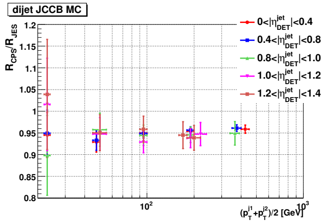
Figura A.16: Melhoria da resolução da energia do jato para eventos simulados de dijetto com jatos reconstruídos com cone \Delta R = 0,7 .
