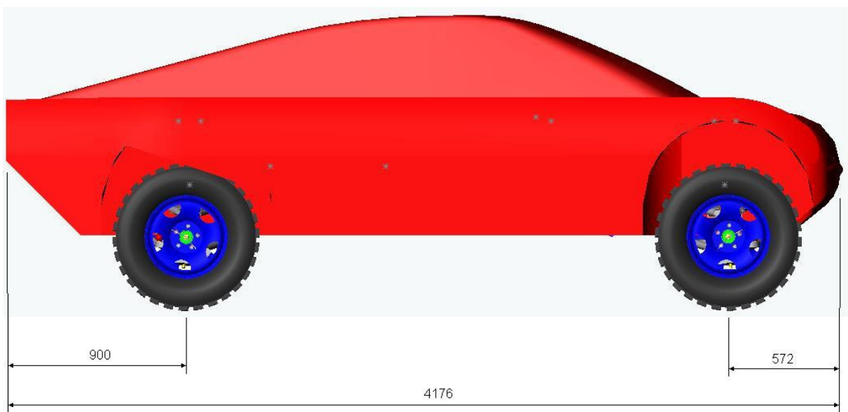
Figura 4.59: Dimensões longitudinais do veículo no seu desenho final.
