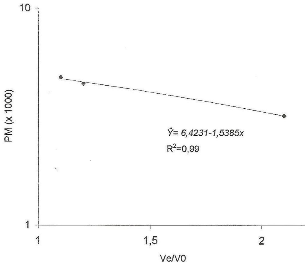
Figura 1. Curva padrão para a determinação de massa molecular em coluna de filtração em gel (1,0 cm x 58,0 cm) de Sephacryl S-100-HR. Padrões moleculares: albumina de soro bovino (66 KDa); anidrase carbônica (29 KDa) e bacitracina (1,45 KDa). O volume vazio da coluna (V0) foi determinado com azul de dextrana, na concentração de 2 mg mL -1 . Amostras de 1 mL eluídas em Tris-HCl 10 mM, pH 8,0. Frações coletadas de 2 mL, a fluxo de 1 mL min -1 .
