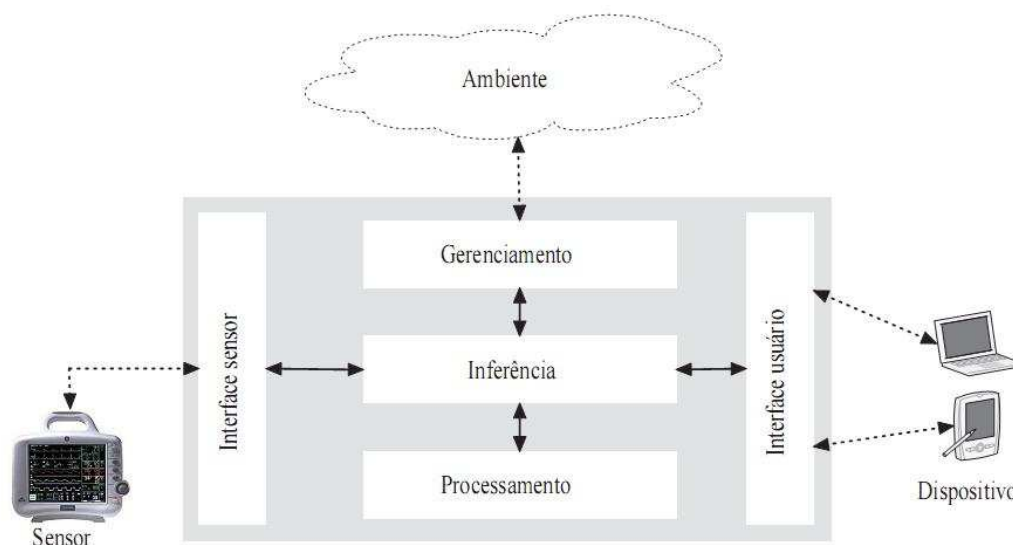
Figura 3.2: Componentes da arquitetura do Grid-M (ROLIM, 2007)
