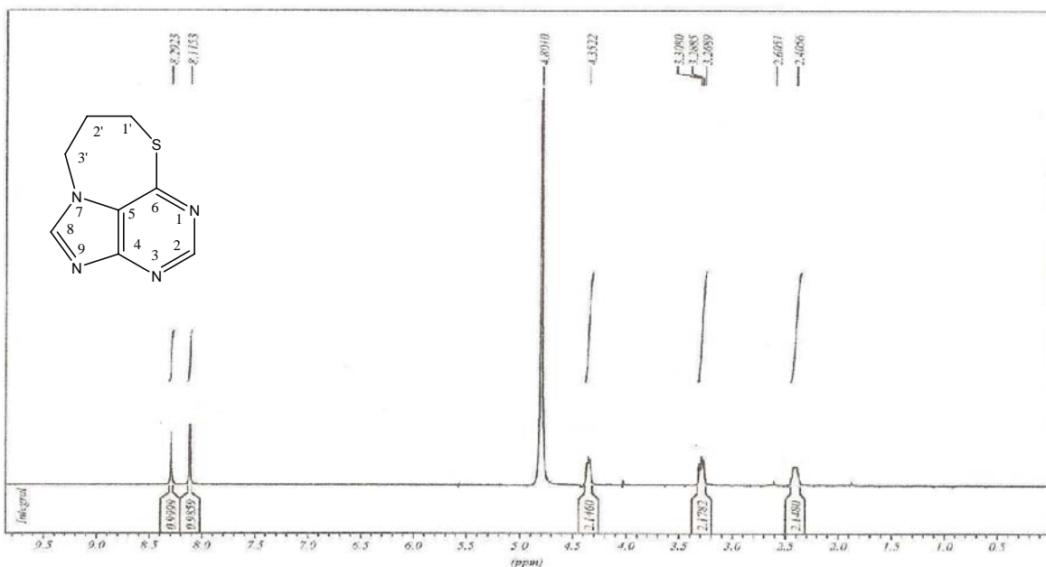
Figura 25. Espectro de RMN de ^1\text{H} do composto 2 ( \text{D}_2\text{O} , 300MHz)
