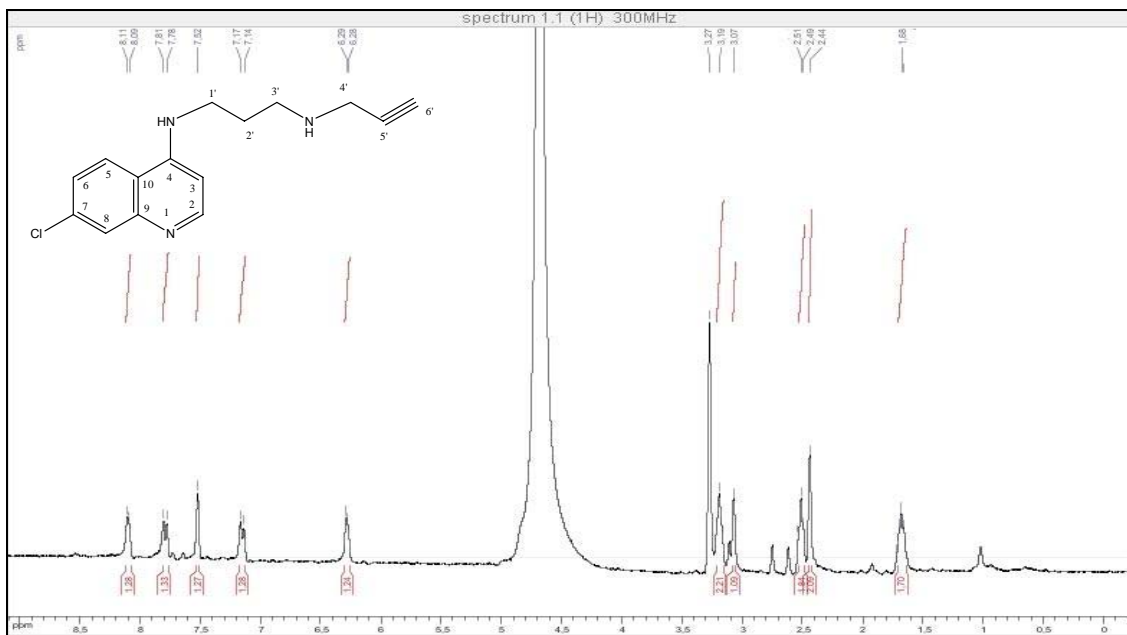
Figura 39. Espectro de RMN de 1 H do composto 7 (CD 3 OD, 300MHz).
