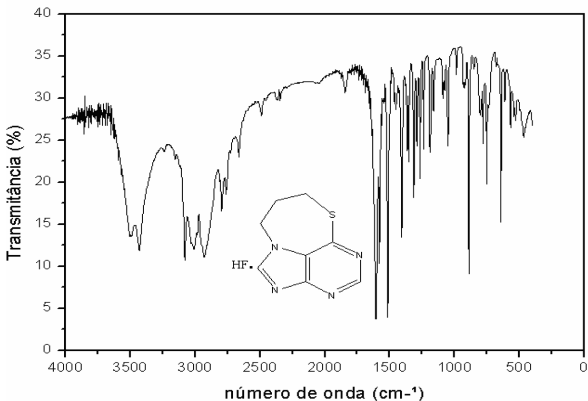
Figura 34. Espectro de IV do composto 4a .
