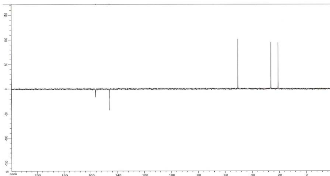
Figura 38. Espectro DEPT 135^\circ\text{C} de ^{13}\text{C} do composto 4a
