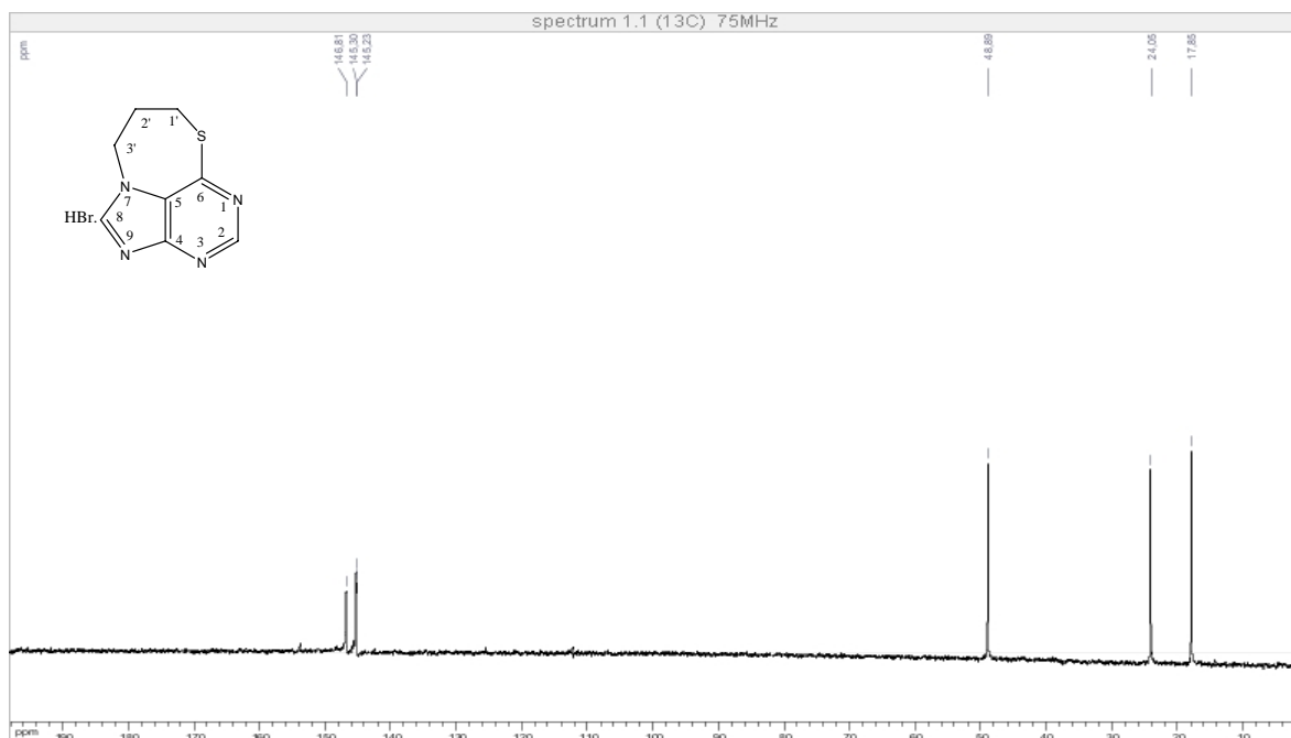
Figura 48. Espectro de RMN de 13 C do composto 4c (D 2 O, 75MHz)
