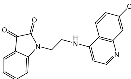
Figura 7. Estrutura química do conjugado 2,3-dioxoindol/ derivado quinolínico.
