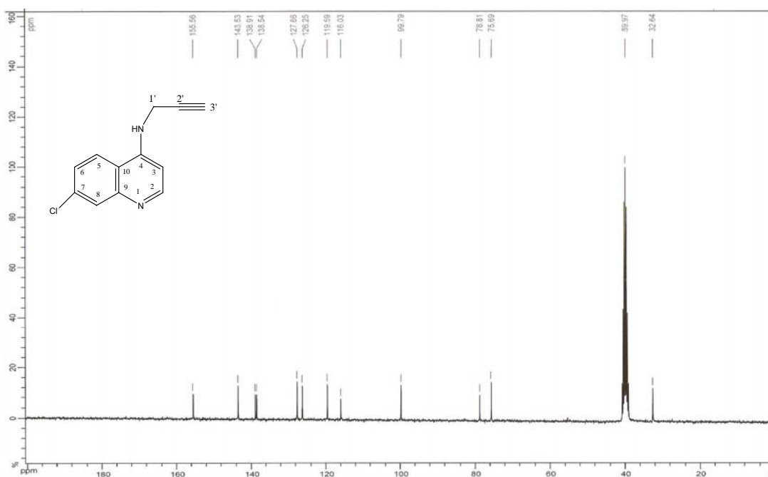
Figura 31. Espectro de RMN de ^{13}\text{C} do composto 5 (DMSO, 75MHz)
