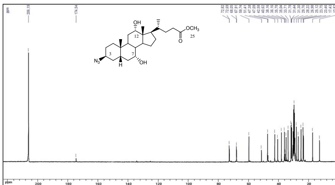
Figura 54. Espectro de RMN de ^{13}\text{C} do composto 11 (acetona deuterada, 75MHz).
