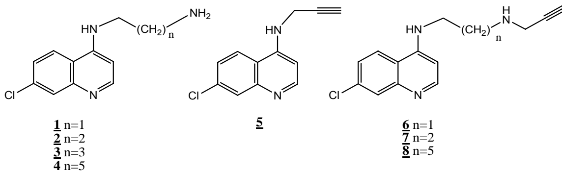
Figura 12. Derivados quinolínicos.
