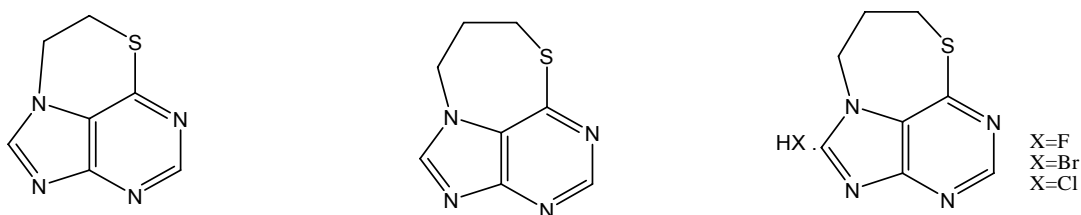
Figura 14. Compostos tricíclicos derivados de 6-MP propostos.
