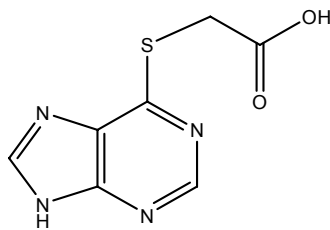
Figura 15. Estrutura do 6-CMMP (composto 5 ).
