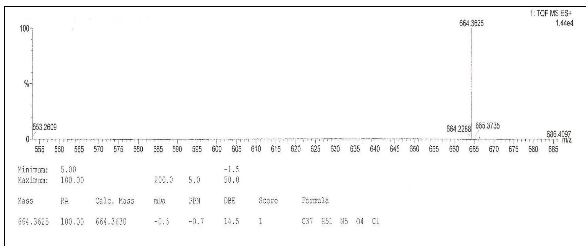
Figura 59. Espectro de massas (HMRS) do composto 12 .
