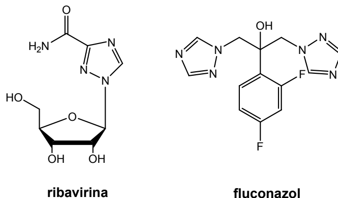
Figura 8. Exemplos de derivados triazólicos farmacologicamente ativos.
