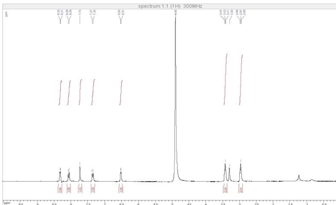
Figura 16. Espectro de RMN de 1 H do composto 1 (CD 3 OD, 300MHz)
