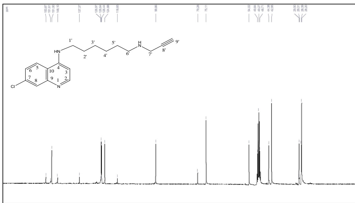
Figura 43. Espectro de RMN de 13 C do composto 8 (CD 3 OD, 75MHz).
