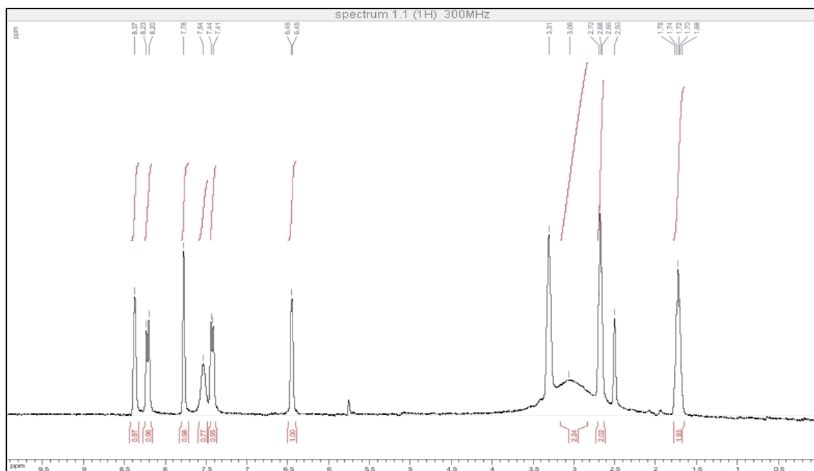
Figura 19. Espectro de RMN de 1 H do composto 2 (DMSO, 300MHz).
