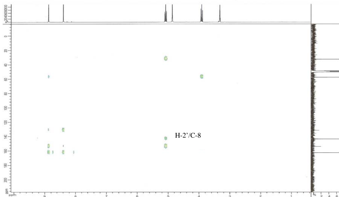
Figura 21. Mapa de contornos HMBC do composto 1 .
