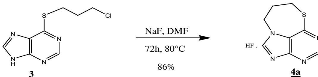
Figura 33. Esquema de reação para obtenção do composto 4a .
