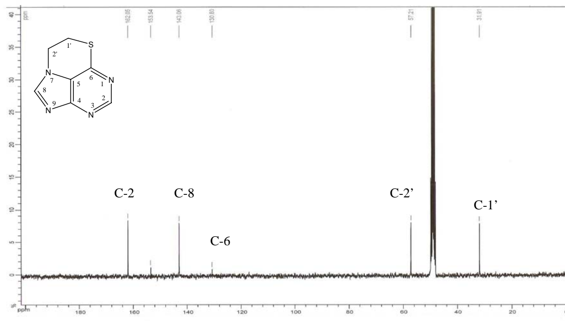
Figura 20. Espectro de RMN de ^{13}\text{C} do composto 1 ( \text{CD}_3\text{OD} , 75MHz)
