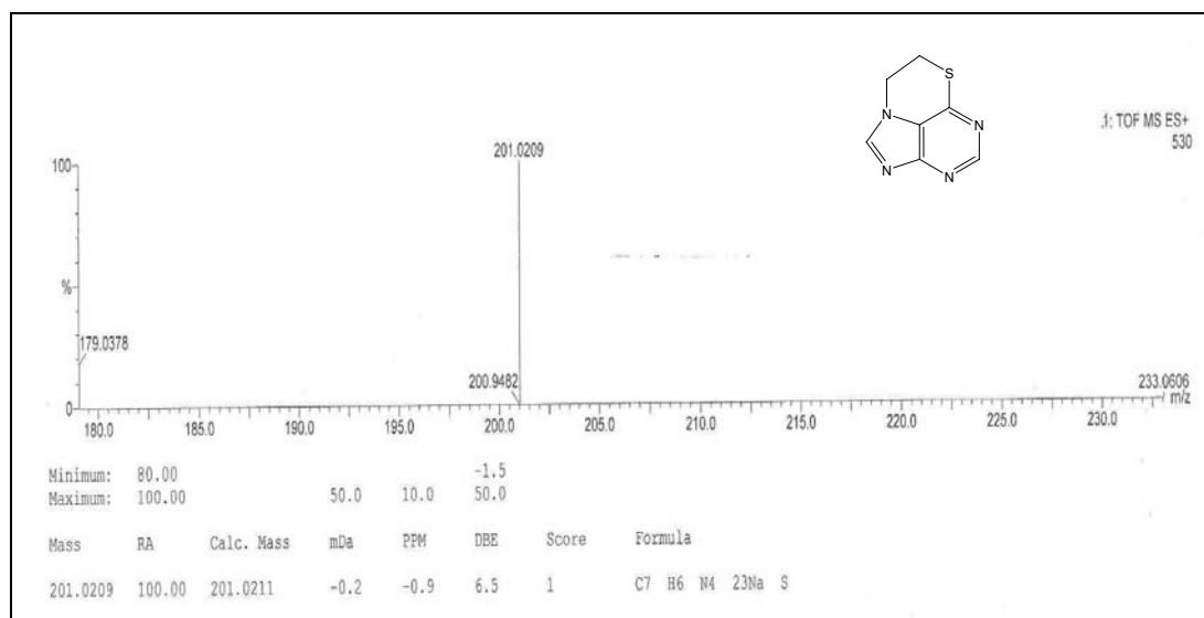
Figura 22. Espectro de massas HMRS do composto 1 .
