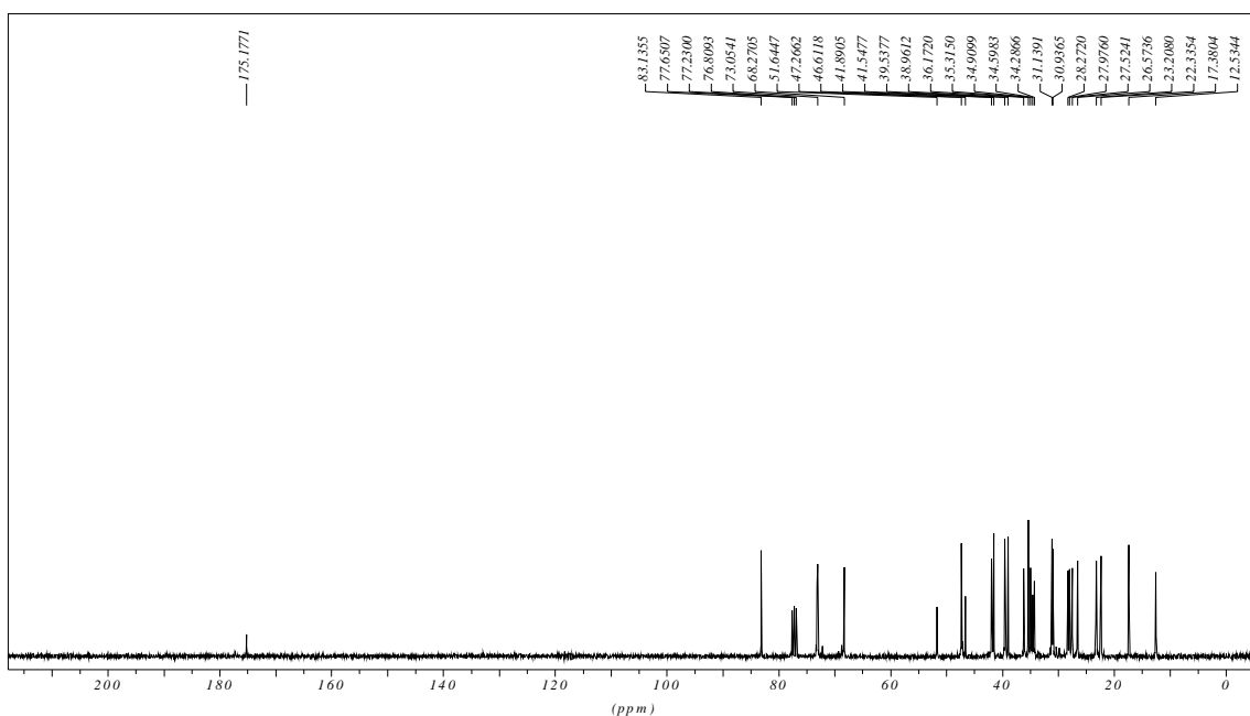
Figura 50. Espectro de RMN de 13 C do composto 10 (CDCl 3 , 75MHz).
