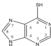
Figura 13. Estrutura da 6-MP.
