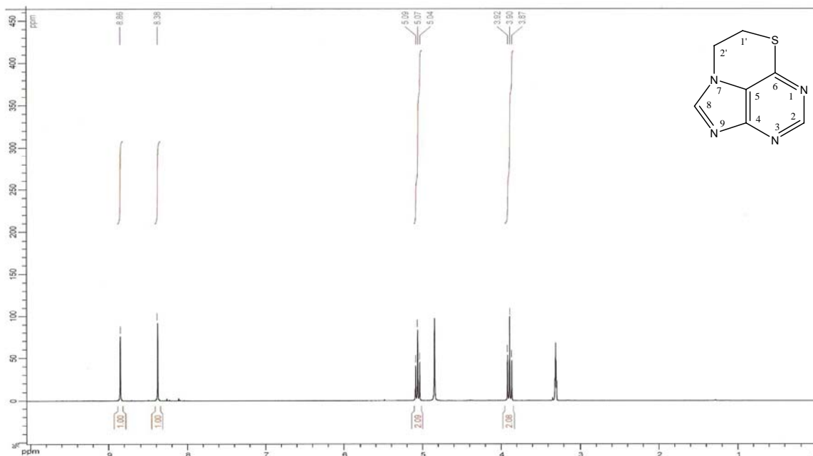
Figura 19. Espectro de RMN de ^1\text{H} do composto 1 ( \text{CD}_3\text{OD} , 300MHz)
