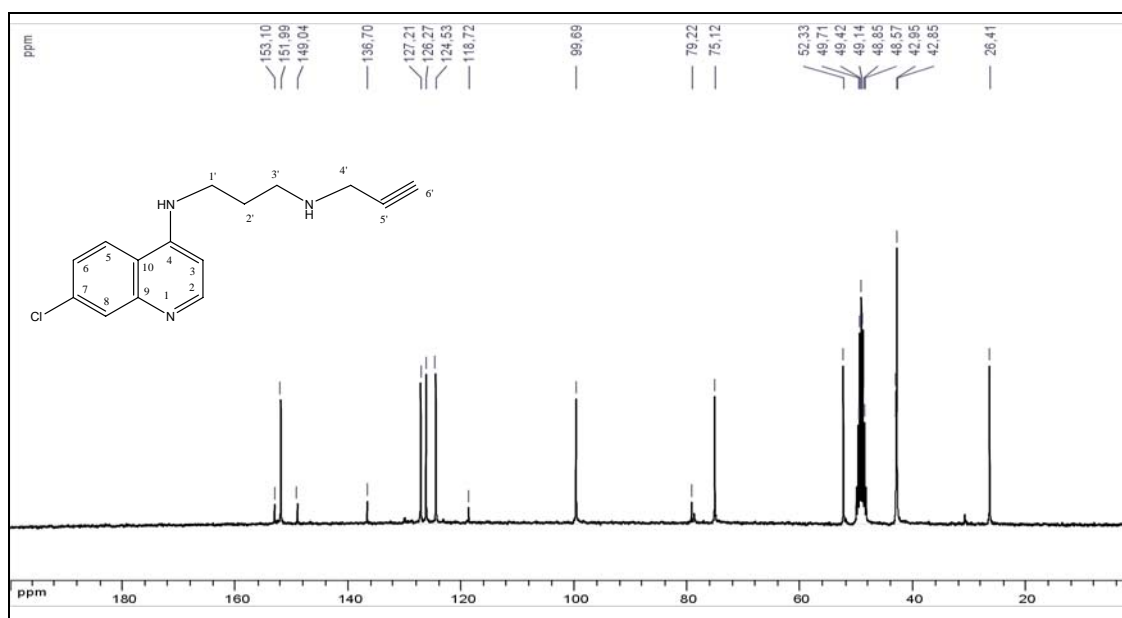
Figura 40. Espectro de RMN de 13 C do composto 7 (CD 3 OD, 75MHz).
