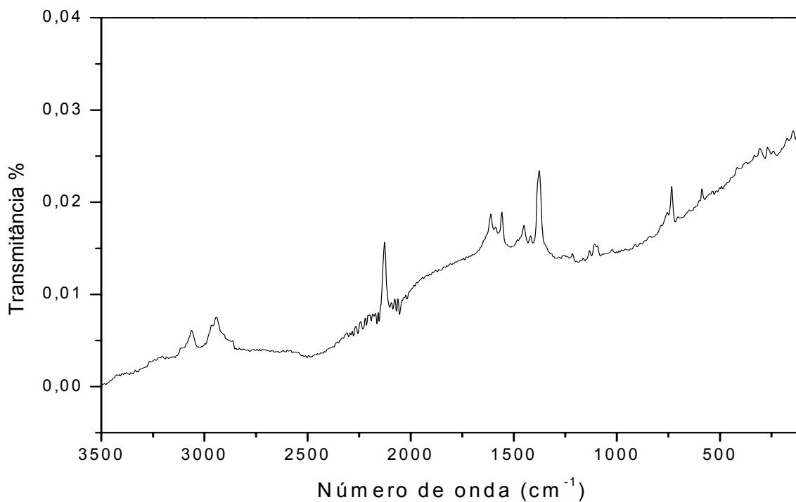
Figura 38. Espectro Raman do composto 7 .
