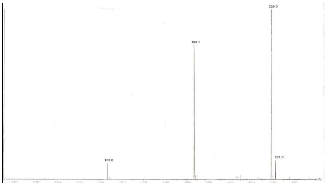
Figura 32. Espectro de massa (ES) do composto 3 .
