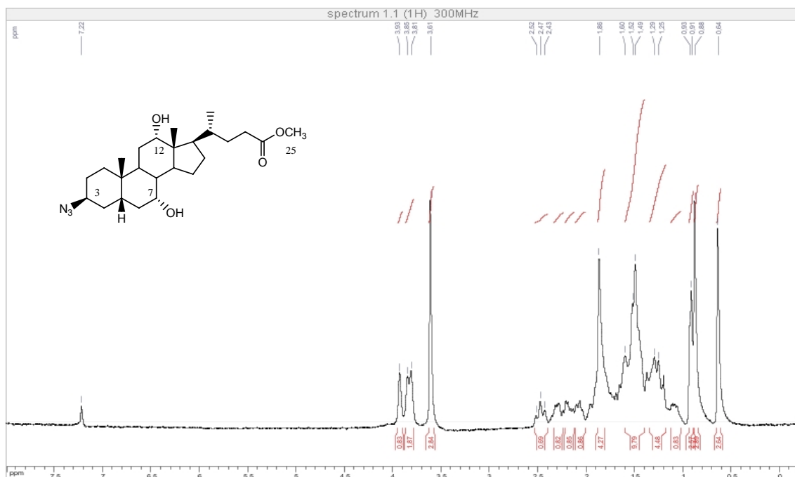
Figura 52. Espectro de RMN de ^1\text{H} do composto 11 ( \text{CDCl}_3 , 300MHz).
