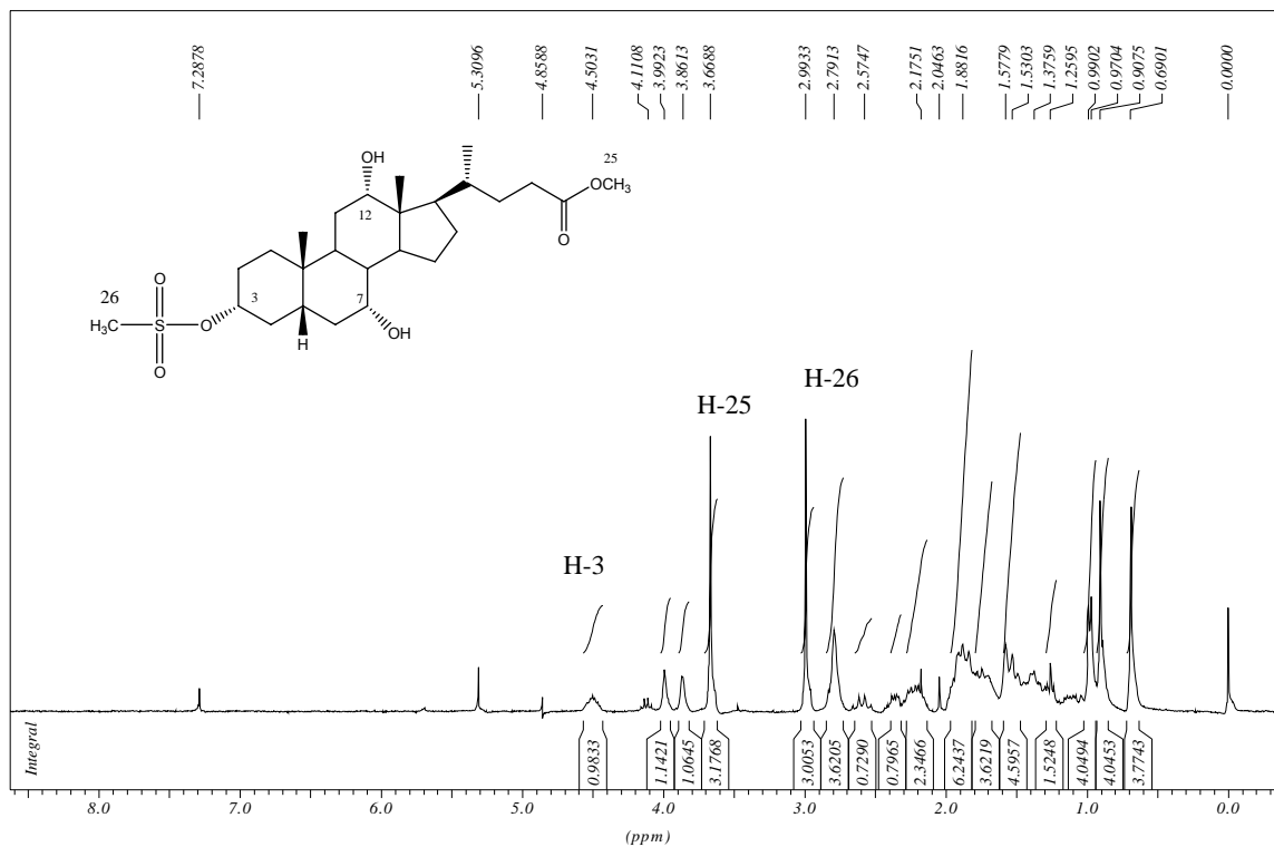
Figura 49. Espectro de RMN de 1 H do composto 10 (CDCl 3 , 300MHz).
