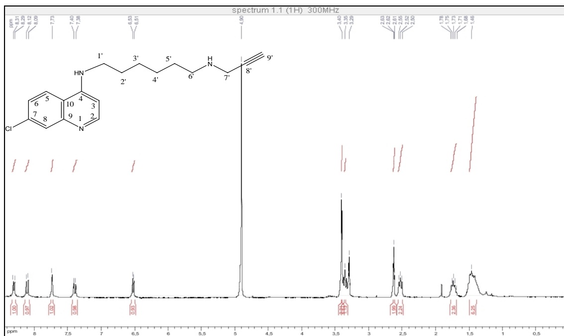
Figura 42. Espectro de RMN de 1 H do composto 8 (CD 3 OD, 300MHz).
