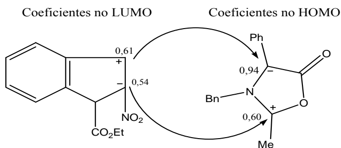
Esquema 3.6: Interação orbital entre o nitro-indol e a munchnona
