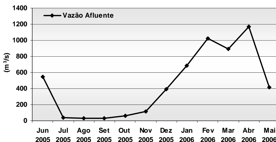
Figura 09: Gráfico da vazão afluente do reservatório da U.H.E. – Samuel entre os meses de junho de 2005 a maio de 2006.
