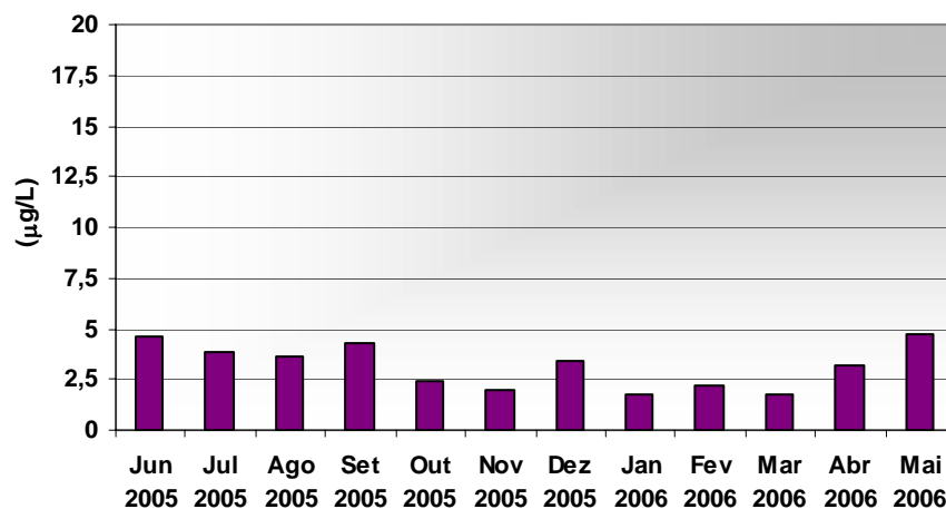
Figura 24: Variação temporal dos valores de pigmento total ( \mu\text{g/L} ) na estação M1 do reservatório da U.H.E. – Samuel (2005-2006).
