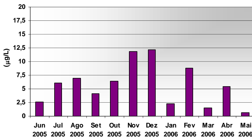
Figura 26: Variação temporal dos valores de pigmento total ( \mu\text{g/L} ) na estação M8 do reservatório da U.H.E. – Samuel (2005-2006).
