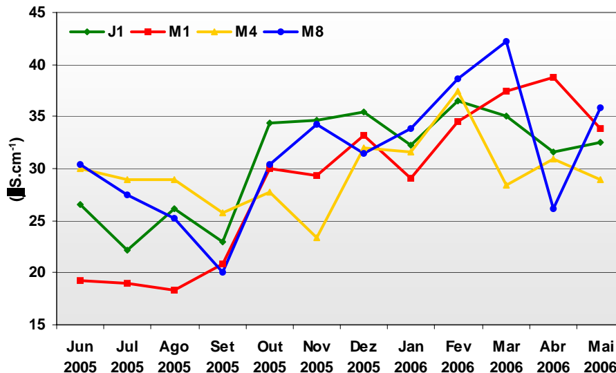
Figura 12: Variação temporal da condutividade elétrica ( \mu\text{S}/\text{cm}^3 ) na superfície da água das estações J1, M1, M4 e M8 do reservatório da U.H.E.–Samuel (2005-2006).
