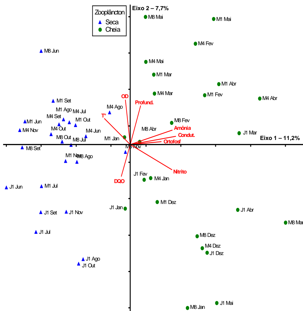
Figura 62: Análise de ACC entre a abundância do zooplâncton e as variáveis ambientais analisadas na UHE – Samuel.
