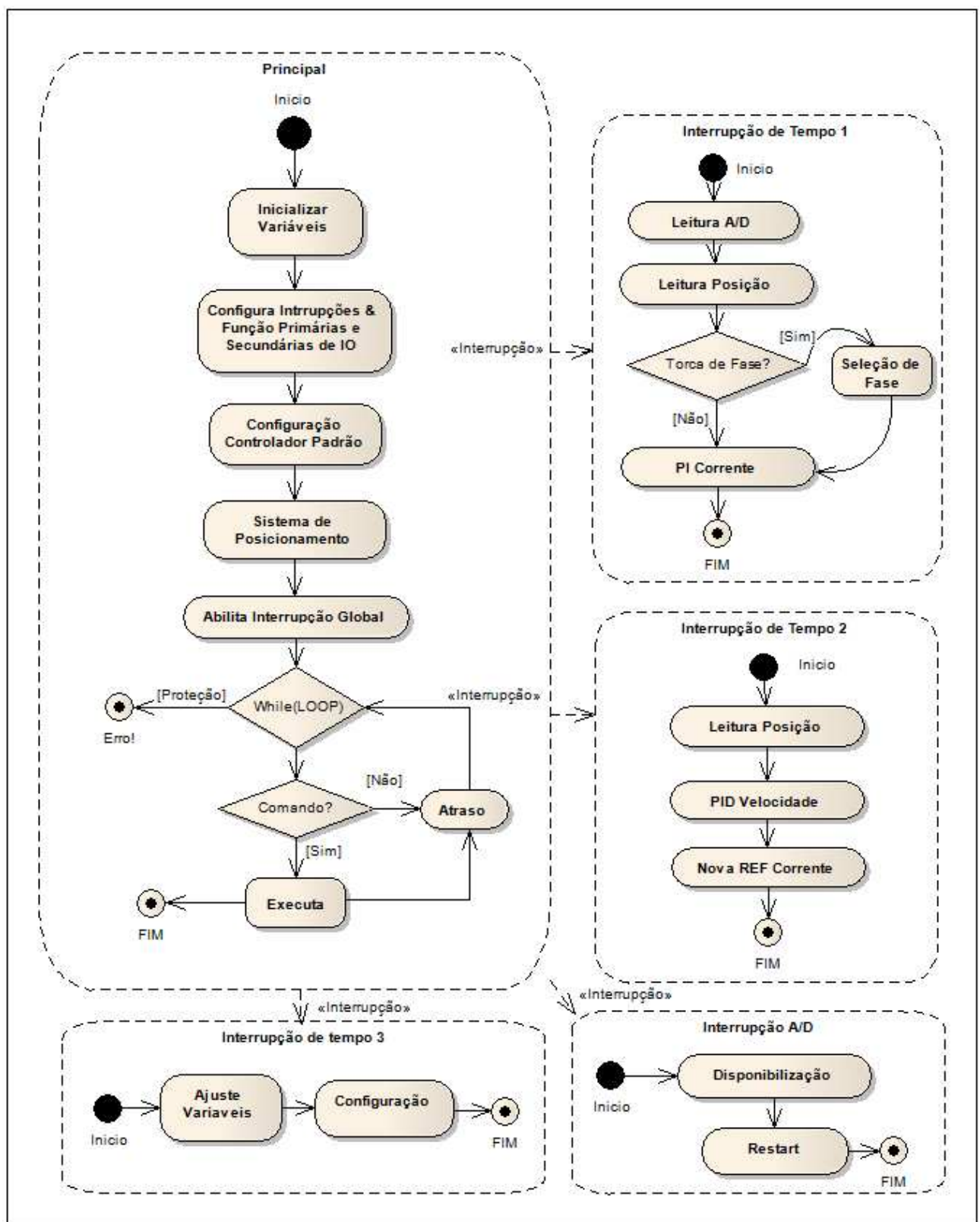
Figura 4.26: Diagrama de fluxo do software de controle.
