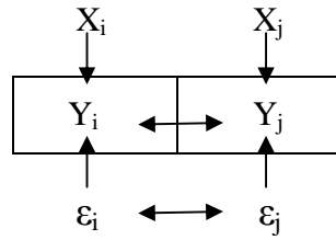
Figura 4. Representação esquemática do modelo SAC 11 .
