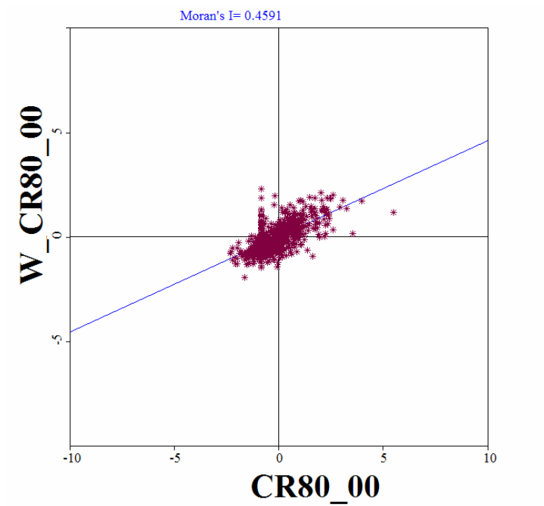
Figura 12. Gráfico de dispersão de Moran.
