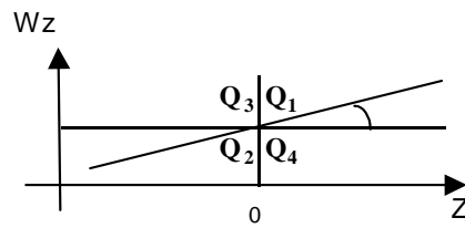
Figura 3. Diagrama de Moran.
