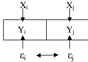
Figura 6. Representação esquemática do modelo SEM.
