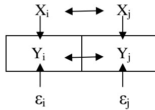
Figura 7. Representação esquemática do modelo SDM.
