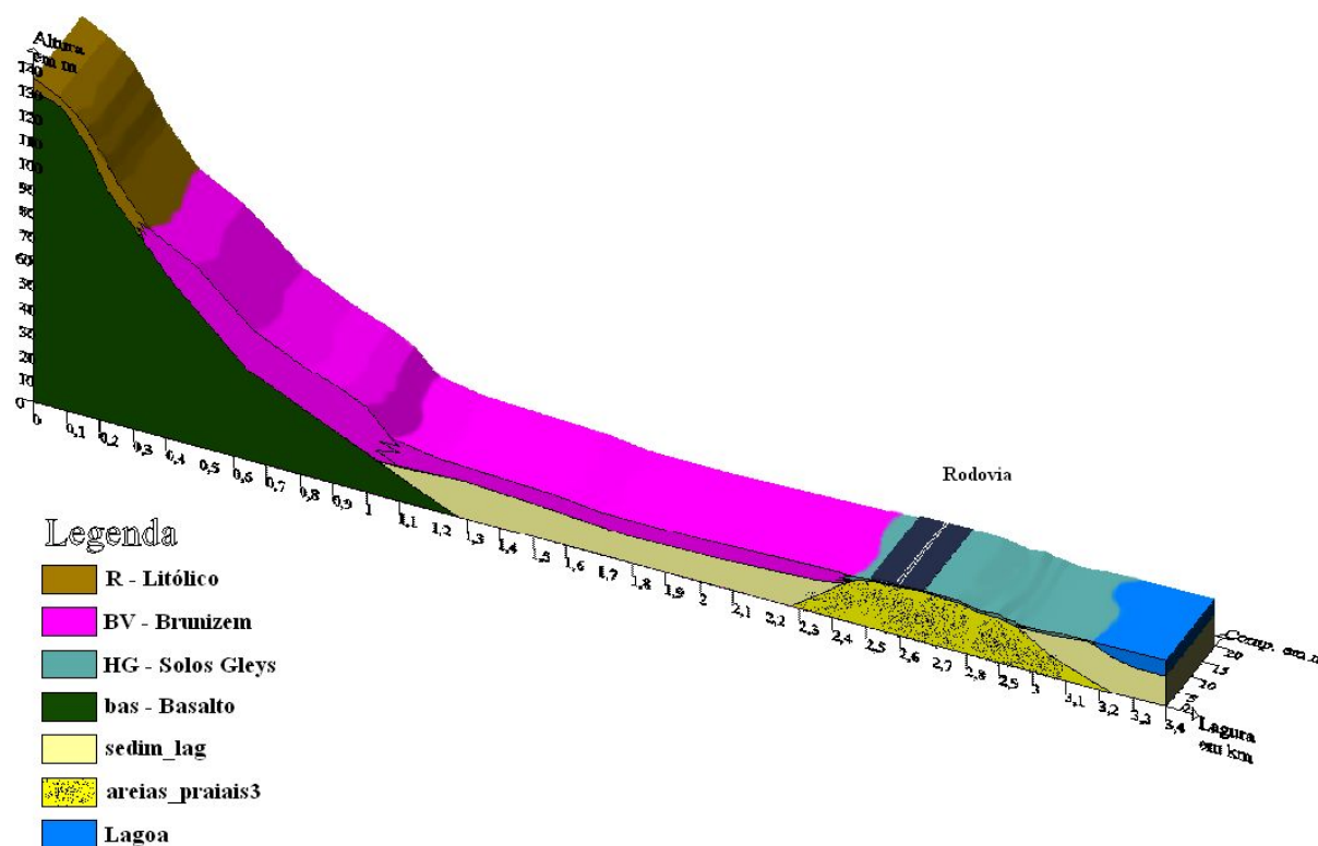
Figura 5.15: Corte no Morro do Túnel, lado sul do morro.
