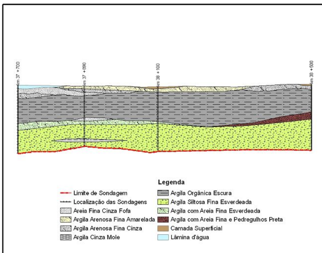
Figura 5.21: Representação do subsolo do Rio Três Forquilhas.
