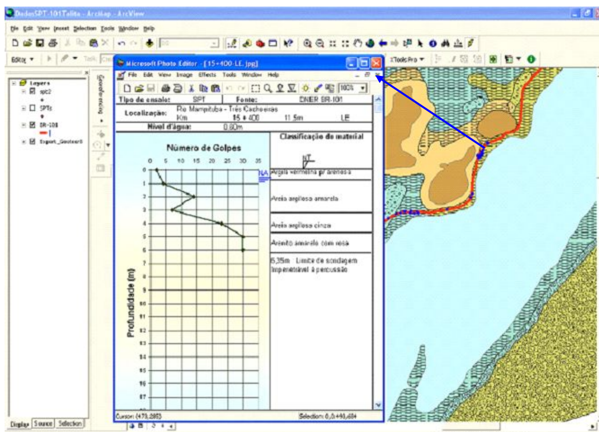
Figura 5.7: Visualização do acesso ao banco de dados em ambiente de SIG.
