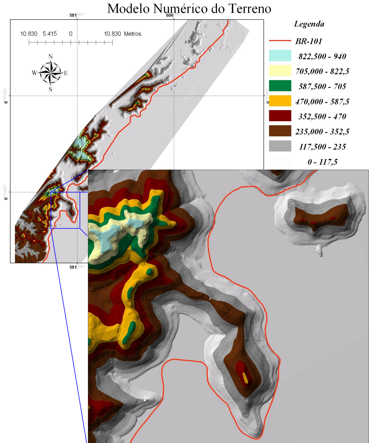
Figura 5.5: Modelo Numérico do Terreno da foz do rio Maquiné (em planta).
