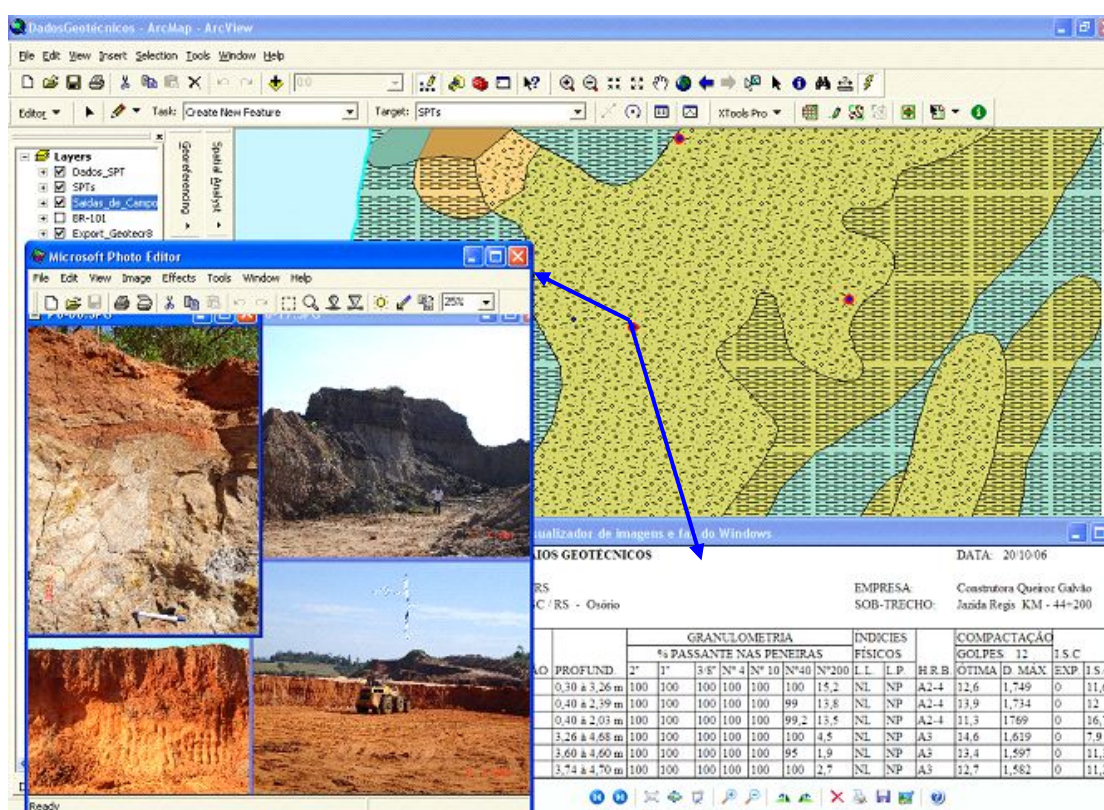
Figura 5.8: Dados geotécnicos das principais jazidas utilizadas na obra.
