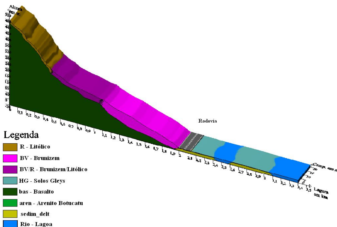
Figura 5.12: Corte no km 39+500 – solos litólicos e brunizems sobre material rochoso e solos gleys sobre depósitos de planície.
