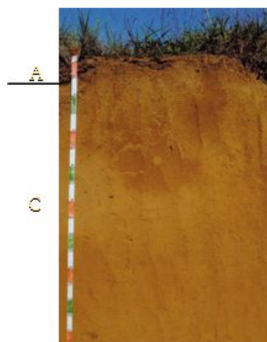
Figura 4.5: Perfil típico da unidade Osório (Streck et al. , 2002).
