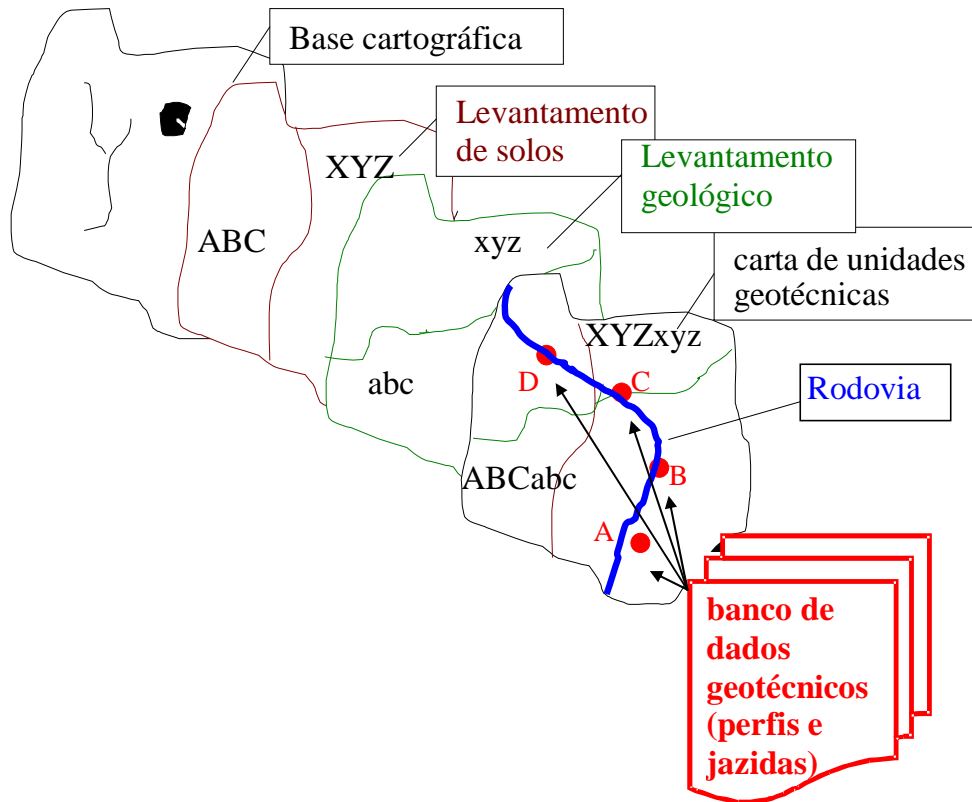
Figura 3.2: Esquema metodológico do mapeamento geotécnico aplicado a obras rodoviárias (modificado de Bastos et al. , 2006).
