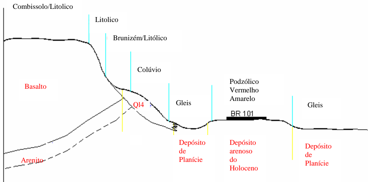
Figura 4.10: Topossequência típica – Seção à 4km antes de Terra de Areia, sentido Osório-Torres.
