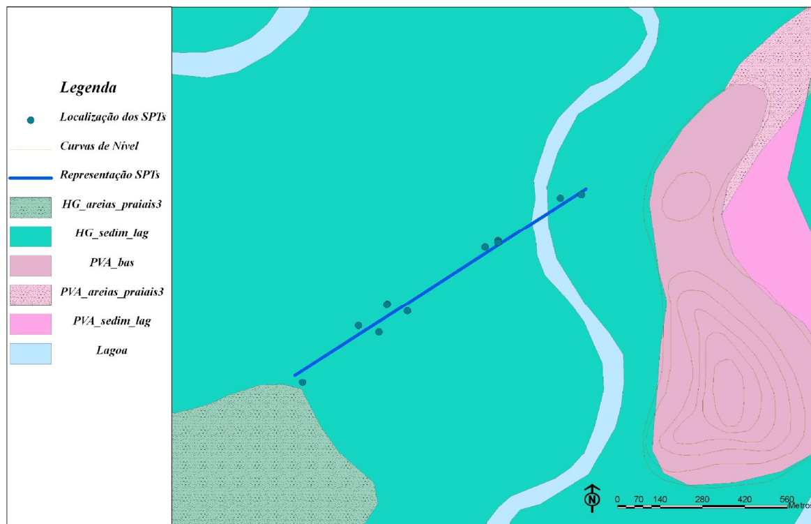
Figura 5.23: Localização dos dados de sondagens SPT e dos tipos de solos do delta do Rio Cardoso.
