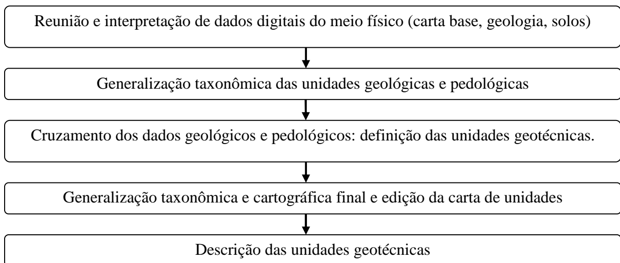
Figura 3.2: Esquema metodológico do mapeamento geotécnico aplicado a obras rodoviárias (modificado de Bastos et al. , 2006).
