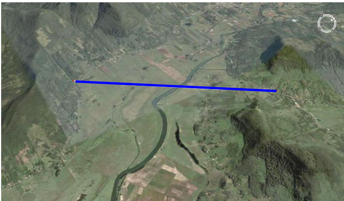
Figura 5.16: Visão geral do delta do Rio Maquine – Linha em branco: linha de sondagem (Google Earth, 2007).
