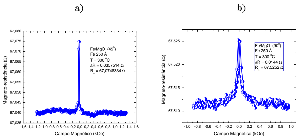
Figura 5.2 Resultado experimental da magneto-resistência para mostra de Fe/MgO (100): a) amostra rotacionada de 45^\circ , eixo fácil e b) rotação de 90^\circ , eixo duro.
