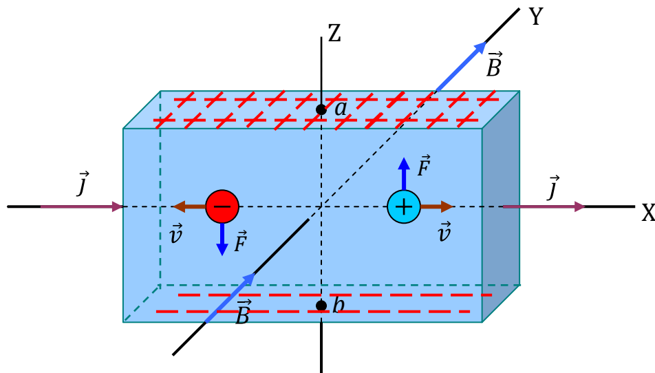
Figura 2.2 Ilustração do efeito Hall. Um campo magnético é aplicado numa barra de um semicondutor, percorrida por uma densidade de corrente elétrica \vec{j} . Quando \vec{j} estiver na direção de X e \vec{B} na direção de Y, todos os portadores de cargas positivas e negativas são defletidos para cima e para baixo na presença do campo magnético \vec{B} . A voltagem Hall ( V_H ) é medida entre os pontos a e b , no eixo Z.
