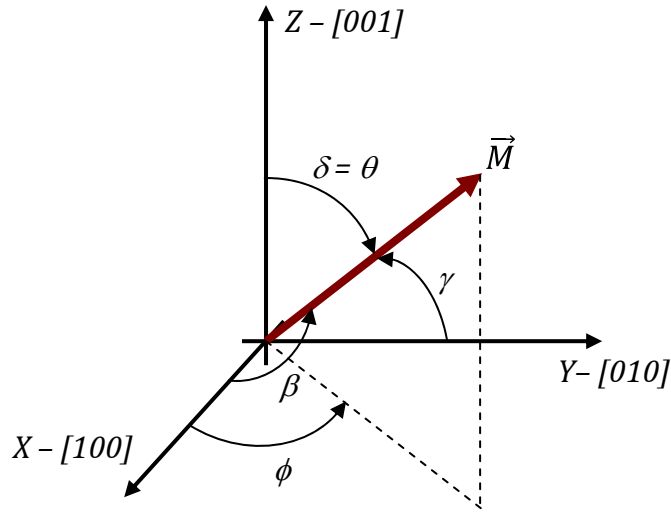
Figura 2.7 Sistema de eixos mostrando as coordenadas esféricas, os co-senos diretores da magnetização e os principais eixos de simetria de um cristal cúbico.
