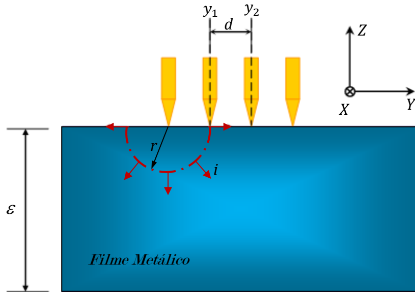
Figura 3.6 Ilustração geométrica da distribuição de corrente elétrica em 2D, no caso em que (\epsilon \gg d) .
