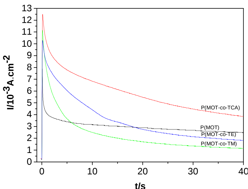
Figura 49: Cronoamperogramas da síntese para os polímeros PMOT-EQ, PMOT-co-TE-EQ, PMOT-co-TM-EQ e PMOT-co-ATC-EQ. Et = CV, Ea = Pt, Er = ECS. Eletrólito: NaClO 4 0,1 mol.L -1 /H 2 O:ACN (3:1). t = 40 s, Temperatura ambiente.
