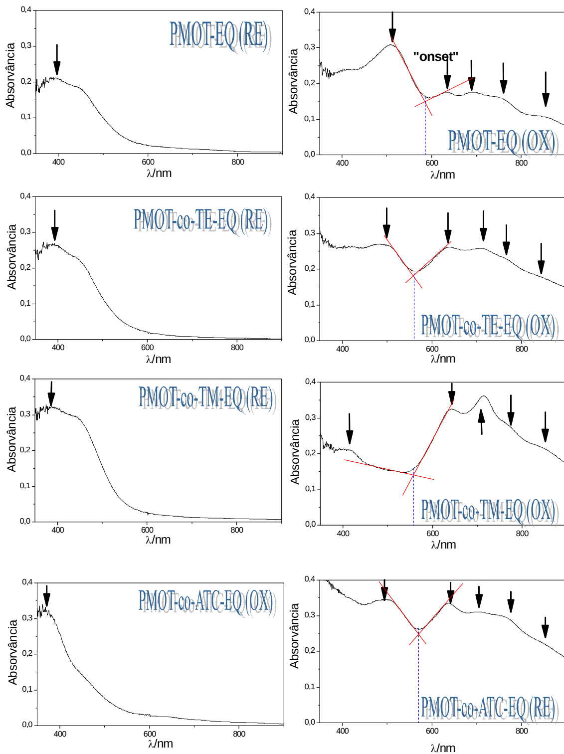
Figura 46: Espectro de UV-vis em acetonitrila para o polímero PMOT-EQ e copolímeros PMOT-co-TE-EQ, PMOT-co-TM-EQ e PMOT-co-ATC-EQ.
