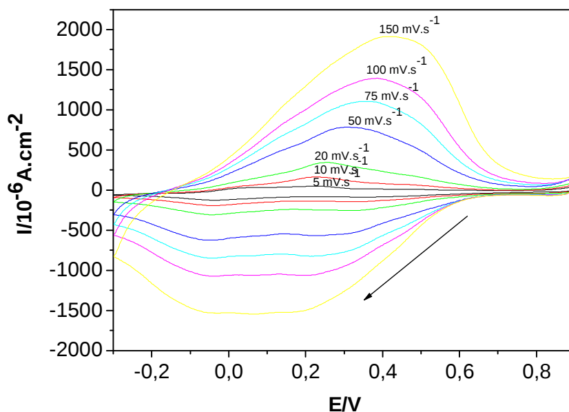
Figura 51: Curva de Voltametria Cíclica para o PMOT-co-TE-EQ. Et = CV, Ea = Pt, Er = ECS. Eletrólito: \text{NaClO}_4 0,1 mol.L -1 /H 2 O:ACN (3:1). Temperatura ambiente.
