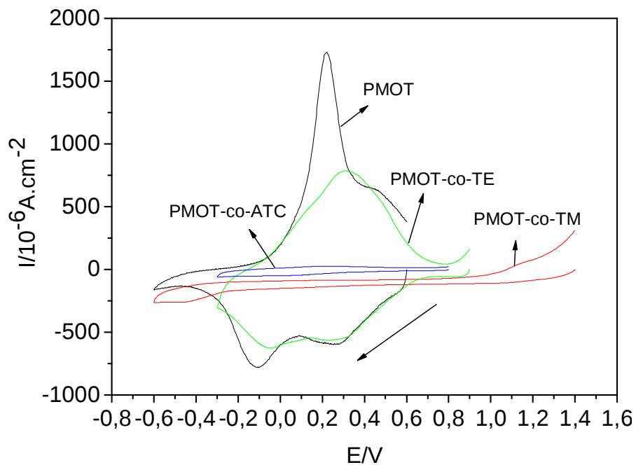
Figura 57: Comparação entre as curvas de voltametria cíclica para os polímeros a uma velocidade de varredura igual a 50 \text{ mV.s}^{-1} . Et = CV, Ea = Pt, Er = ECS. Eletrólito: \text{NaClO}_4 0,1 \text{ mol.L}^{-1}/\text{H}_2\text{O}:\text{ACN} (3:1). Temperatura ambiente.
