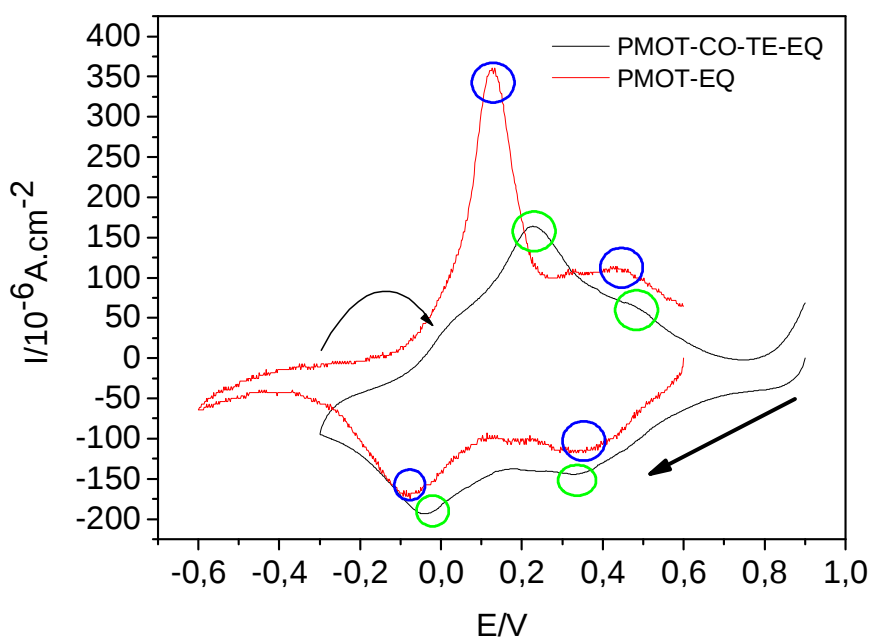
Figura 52: Curvas voltamétricas para os polímeros PMOT-EQ e PMOT-co-TE-EQ a 10 mV.s -1 . Círculos azuis – picos do PMOT-EQ; Círculos verdes – picos do PMOT-co-TE-EQ; Seta curva – Pico anódico irreversível presente no PMOT-co-TE-EQ até a velocidade de varredura de 10 mV.s -1 . Et = CV, Ea = Pt, Er = ECS. Eletrólito: \text{NaClO}_4 0,1 mol.L -1 /H 2 O:ACN (3:1). Temperatura ambiente.
