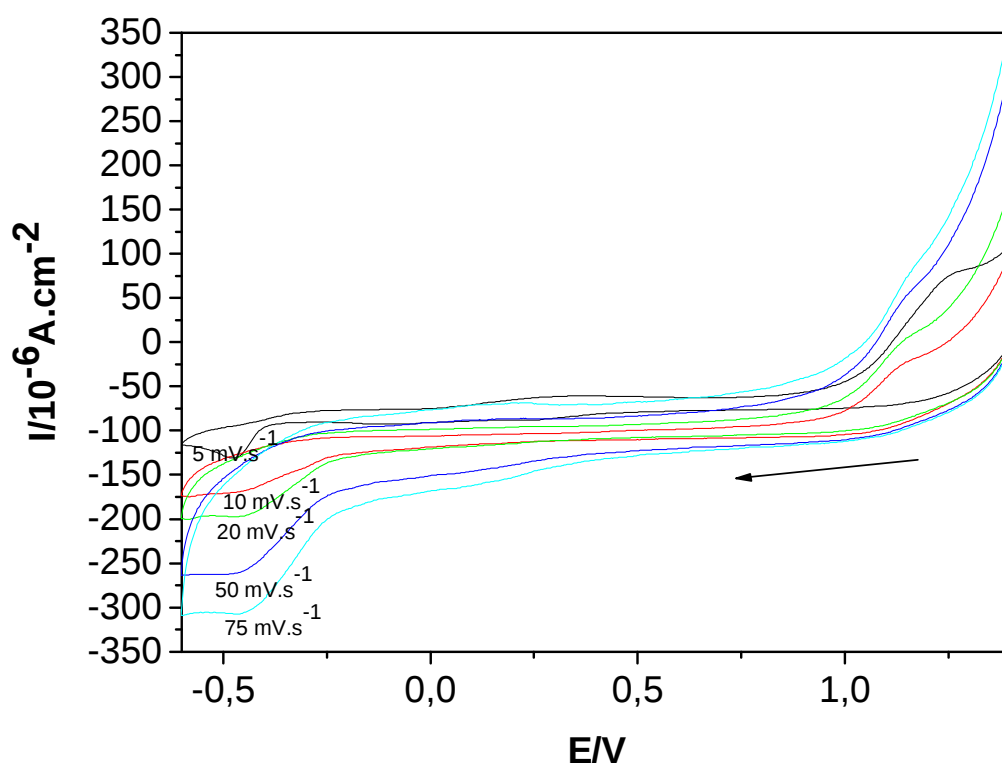
Figura 53: Curva de Voltametria Cíclica para o PMOT-co-TM-EQ. Et = CV, Ea = Pt, Er = ECS. Eletrólito: \text{NaClO}_4 0,1 \text{mol.L}^{-1} /H 2 O:ACN (3:1). Temperatura ambiente.
