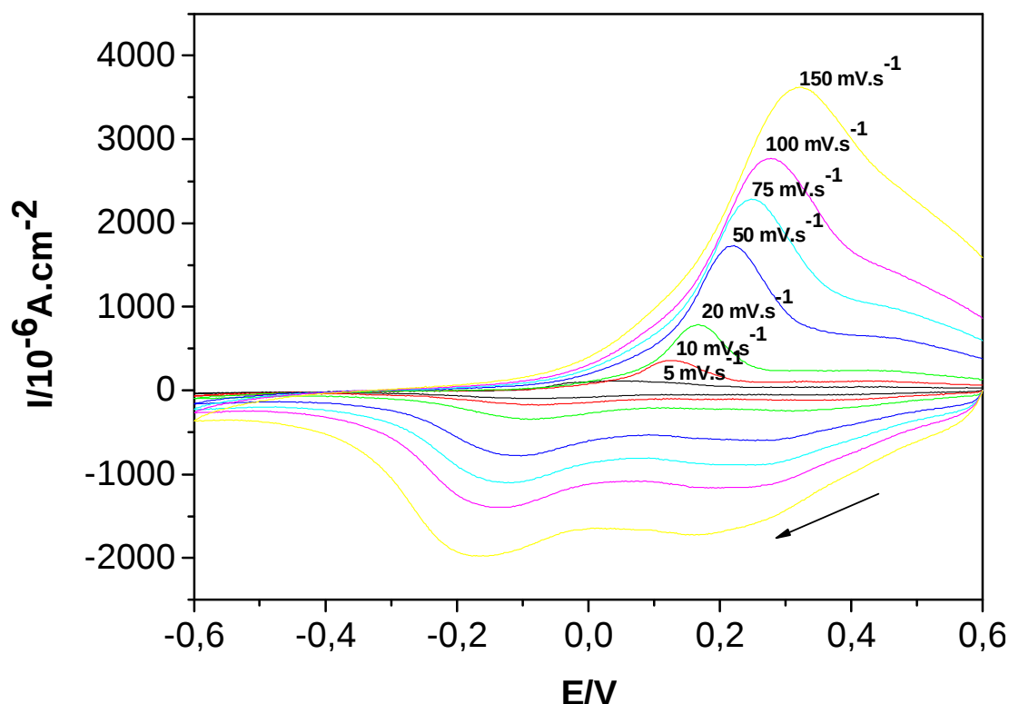
Figura 50: Curva de Voltametria Cíclica para o PMOT-EQ. Et = CV, Ea = Pt, Er = ECS. Eletrólito: \text{NaClO}_4 0,1 mol.L -1 /H 2 O:ACN (3:1). Temperatura ambiente.
