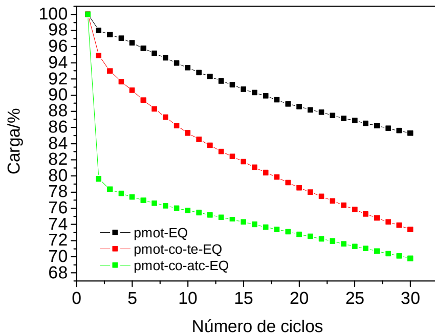
Figura 58: Perda de carga total em função do número de ciclos para os polímeros PMOT-EQ, PMOT-co-TE-EQ e PMOT-co-ATC-EQ. Et = CV, Ea = Pt, Er = ECS. Eletrólito: \text{NaClO}_4 0,1 \text{ mol.L}^{-1}/\text{H}_2\text{O}:\text{ACN} (3:1). Temperatura ambiente.
