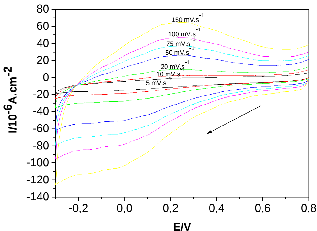
Figura 54: Curva de Voltametria Cíclica para o PMOT-co-ATC-EQ. Et = CV, Ea = Pt, Er = ECS. Eletrólito: NaClO 4 0,1 mol.L -1 /H 2 O:ACN (3:1). Temperatura ambiente.
